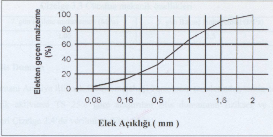
Şekil 3.1 Standart CEN kumu granülometri eğrisi
