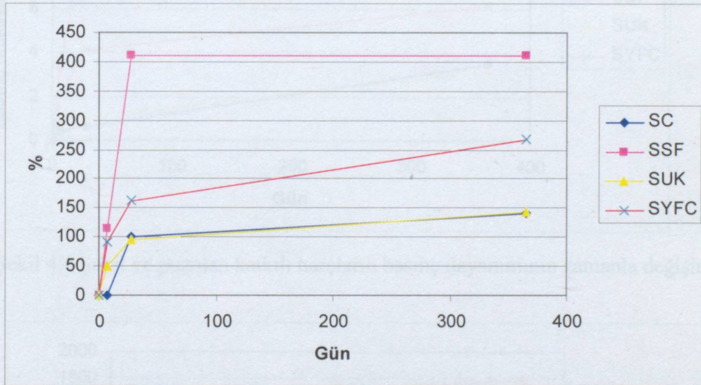
Şekil 4.3 Eğilme mukavemetinin bağıl değerinin zamanla değişimi
