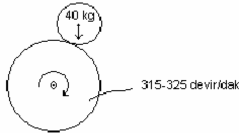
Şekil 3.5 Cilalanma deney düzeneğinin şematik gösterimi (Özen, 2004)
