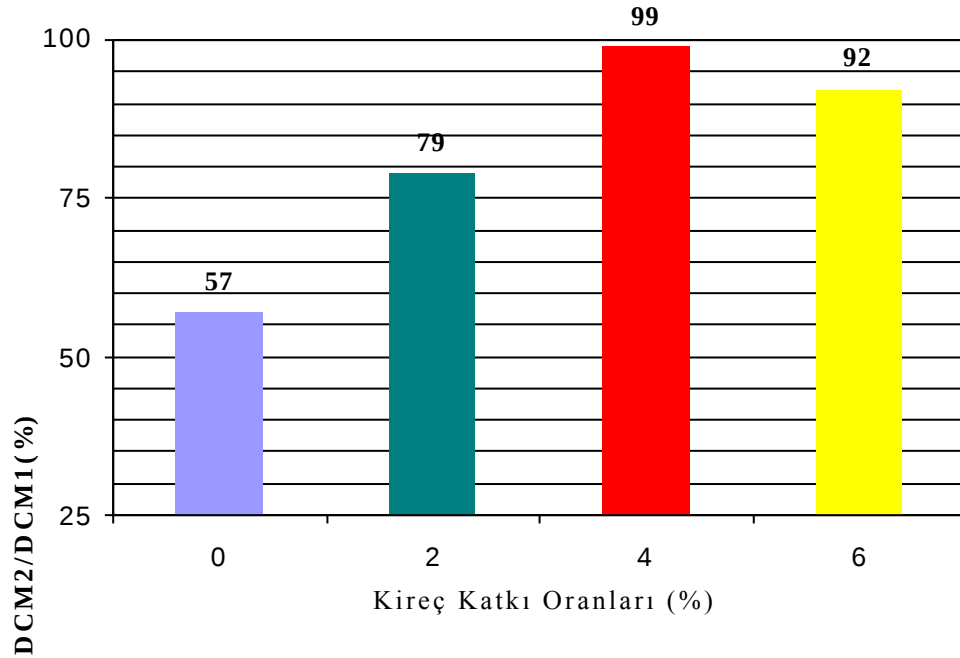
Şekil 8.8 Kireç katkı oranları- düşük sıcaklıktaki koşullu ve koşulsuz numunelerin dolaylı çekme mukavemeti değerlerinin oranları ilişkisi
