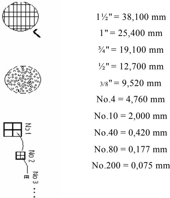
Şekil 3.1 Agreg, gradasyonları için kullanılan elek boyutları (Özen, 2004)
