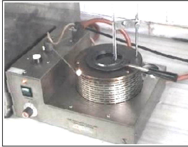
Şekil 3.17 Cleveland açık kap cihazı (Özen, 2005)
