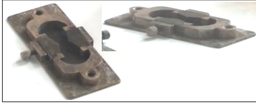
Şekil 3.13 Düktilite deney düzeneğinde kullanılan pirinç kalıpları (Özen, 2005)
