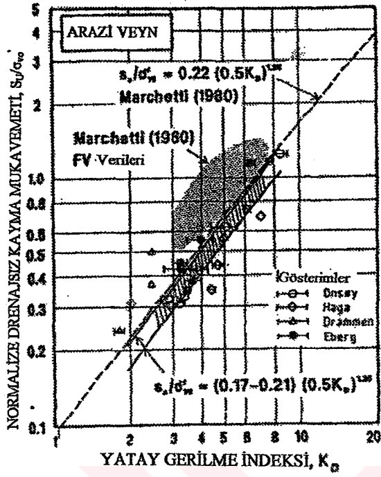
Şekil 2.34 S_u/\sigma'_{vo} vs K_0 (Lacasse ve Lunne, 1988)
