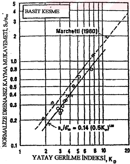
Şekil 2.36 S_u/\sigma'_{vo} vs K_0 (Lacasse ve Lunne, 1988)
