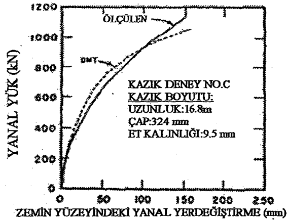
Şekil 2.42 Kazığın en üst noktasındaki yer değiştirmenin bulunan değeri:Deney C (Robertson vd., 1989b)
