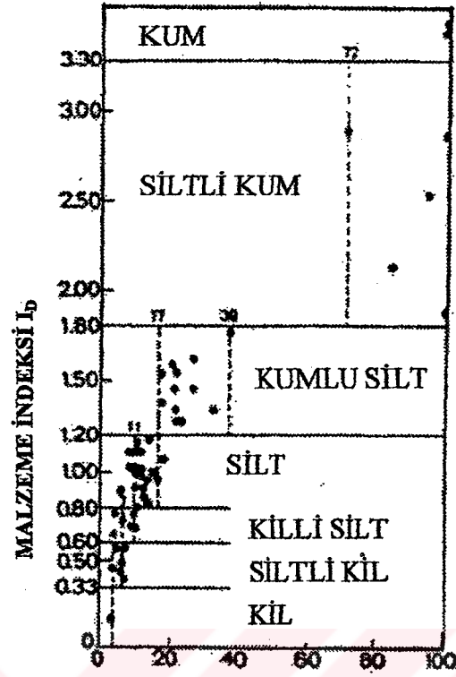
Şekil 2.18 Girişten 1 dak sonra I_D 'ye bağlı olarak artık boşluk suyu basıncının sönümlenmesi (Davidson ve Boghrat, 1983)
