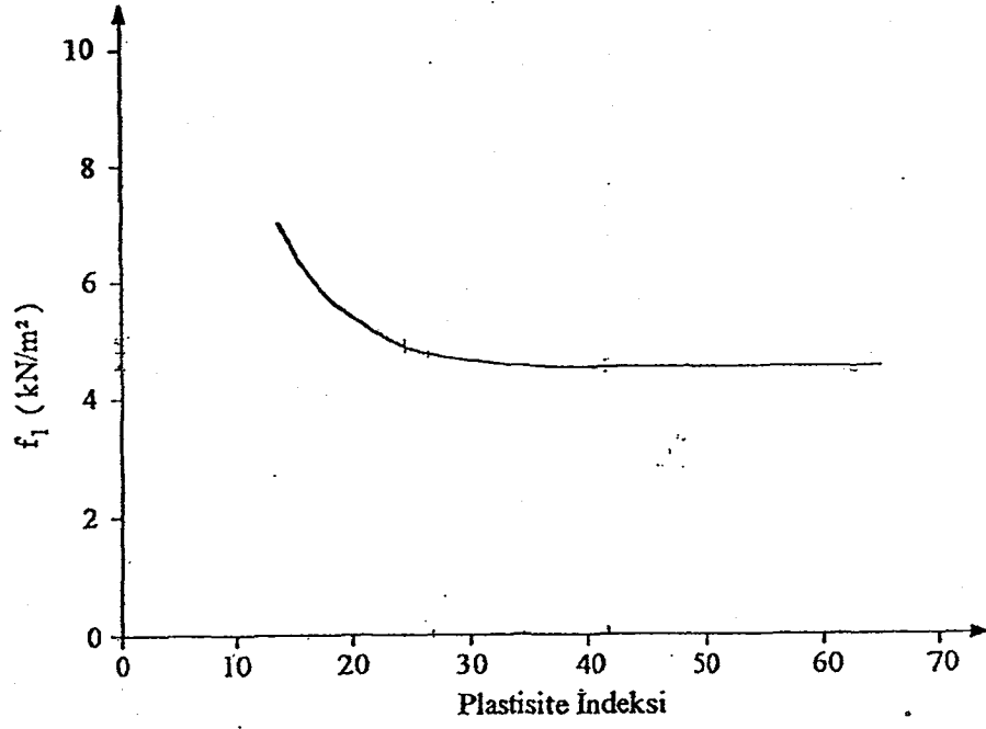
Şekil 3.4 f_1 = C_u/N değerinin plastisite indeksi ile değişimi (Stroud ve Butler, 1975)
