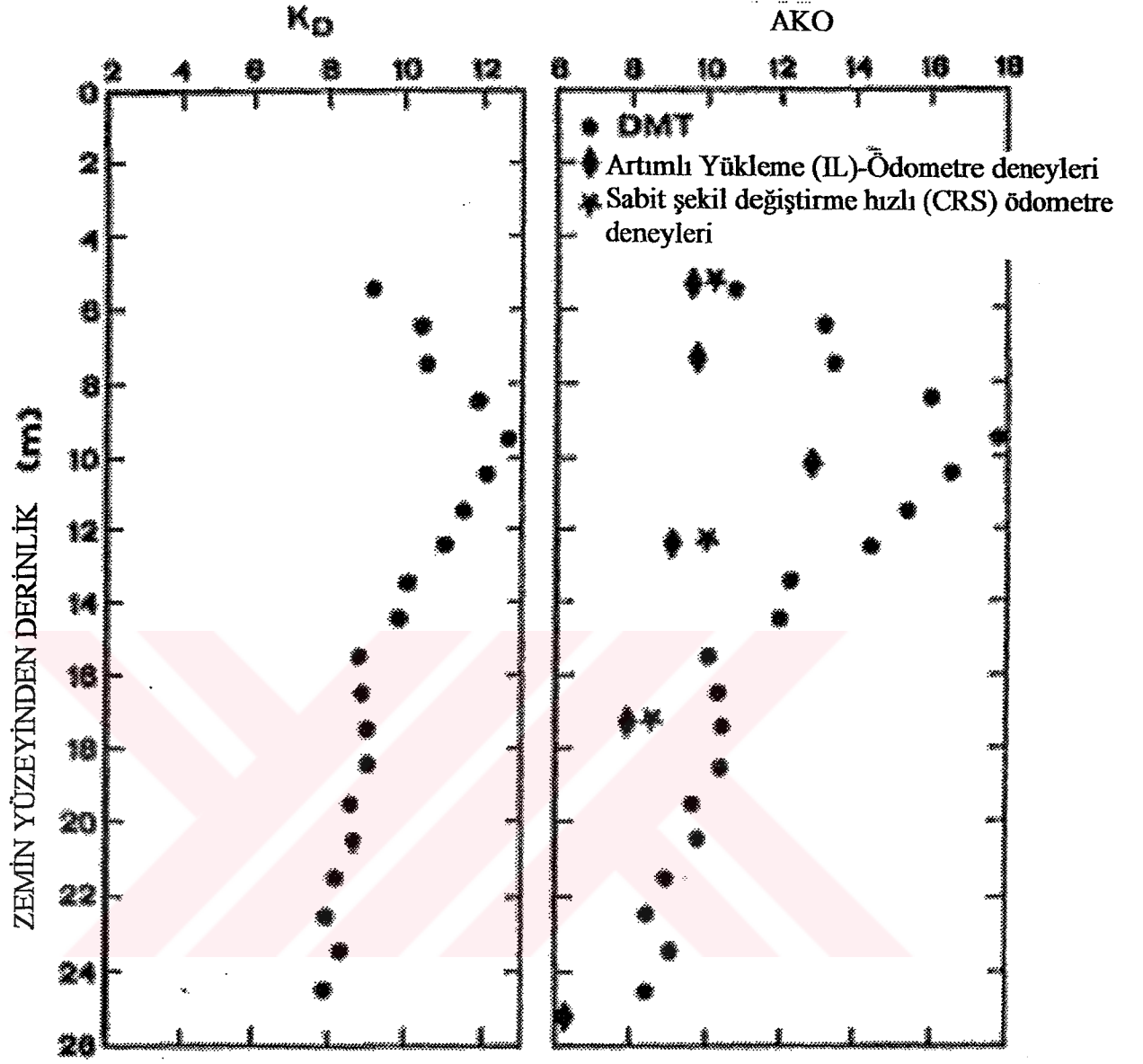
Şekil 5.2 K_D değişiminin AKO değişimi ile benzerliği (Jamolkowski vd., 1988)
