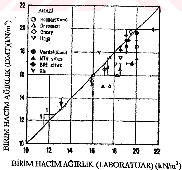
Şekil 2.21 Dilatometre deneyi parametrelerinden arazi birim hacim ağırlığının tahmini (Lacasse ve Lunne, 1988)
