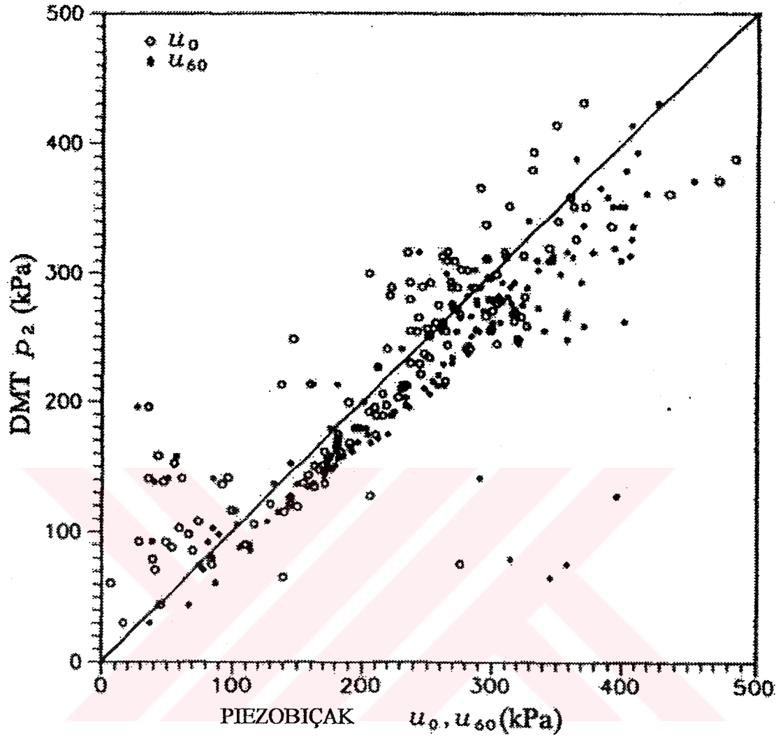
Şekil 2.13 Piezobıçak u_{artık} ile DMT p_2 arasındaki karşılaştırma (Lutenegger ve Kabir, 1988)
