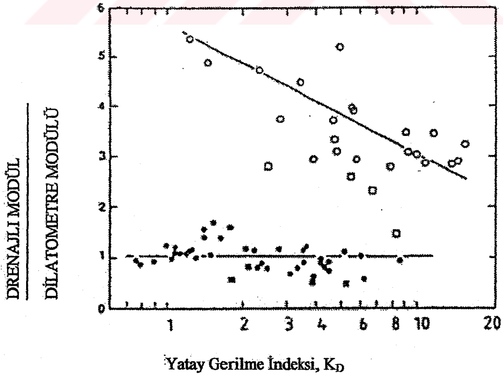
Şekil 2.26 Kumlar için, dilatometre deneyinden elde edilen drenajlı Young Modülünün değerlendirilmesi (Belloti vd., 1989)
