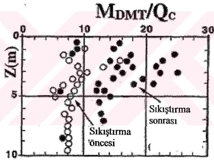
Şekil 5.9 Sıkıştırma öncesi ve sonrasında ölçülen koni uç direnci Q_c ile DMT sınırlanmış modülü M_{DMT} değişimi (Jendeby, 1992)
