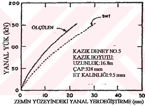
Şekil 2.41 Kazığın en üst noktasındaki yer değiştirmenin bulunan değeri:Deney 5 (Robertson vd., 1989b)
