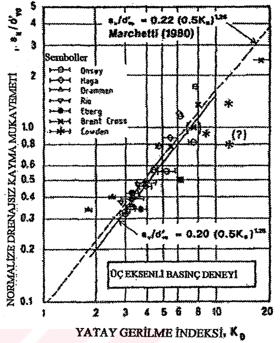
Şekil 2.35 S_u/\sigma'_{vo} vs K_0 (Lacasse ve Lunne, 1988)
