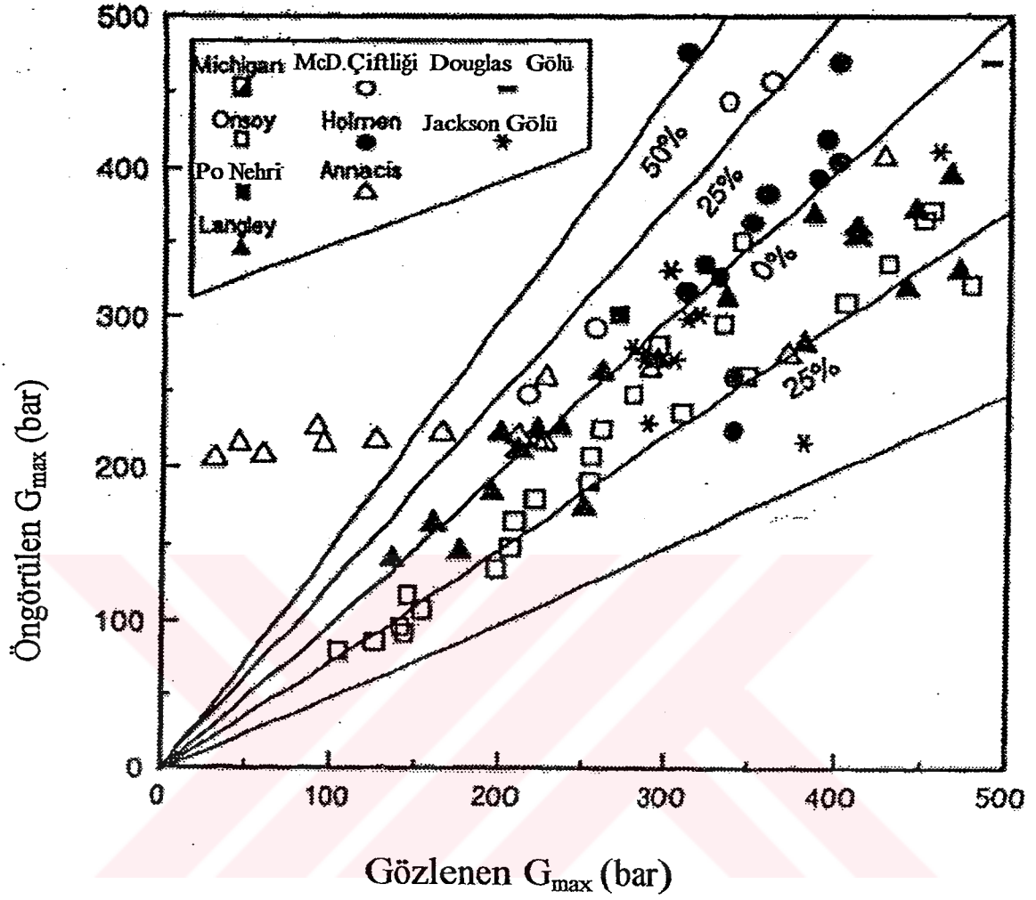
Şekil 2.29 Gözlenen G_{max} 'a karşılık öngörülen G_{max} (Hryciw, 1990)
