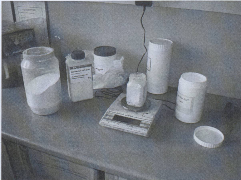
Şekil 8.1 Toz karışımının hassas terazide tartılarak hazırlanması
