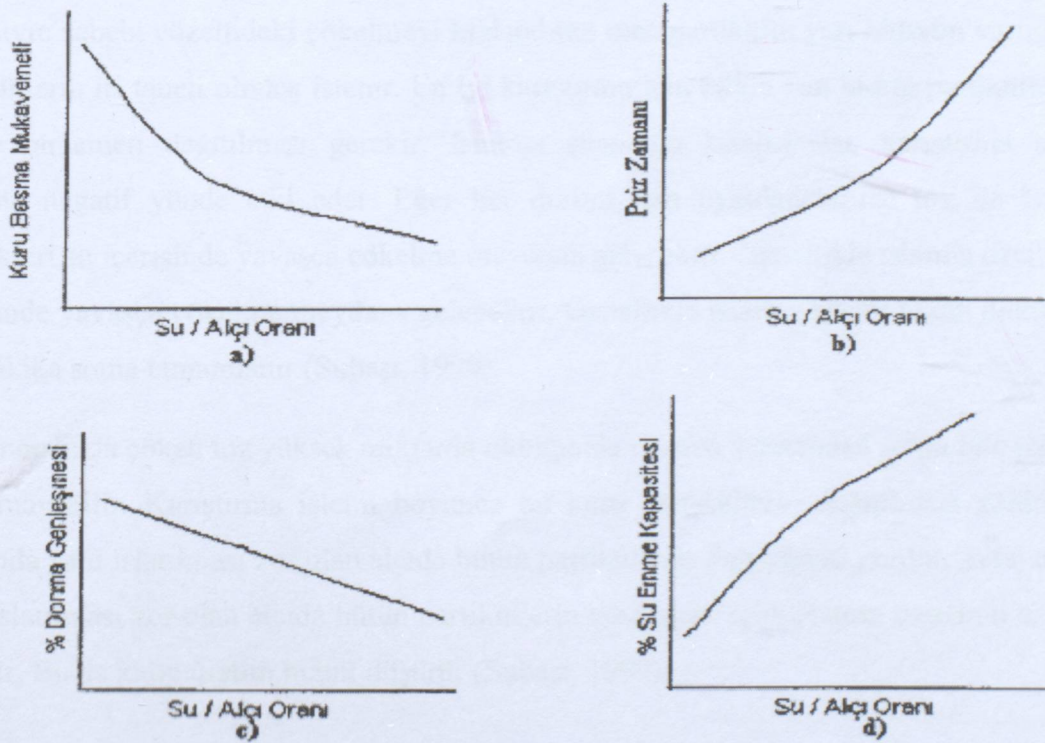
Şekil 6.4 Su /Alçı oranına bağılı olarak sırasıyla kuru basma mukavemeti, priz zamanı, % sertleşme genleşmesi ve % su emme kapasitesinin değışimi (Mahir, 1996)
