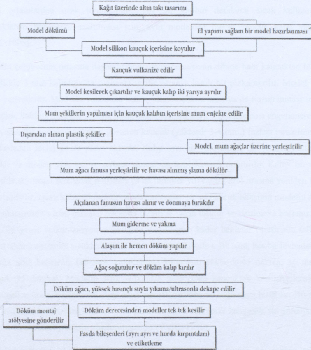
Şekil 4.2 Kuyumculukta dereceli hassas döküm işlem kademeleri (Wright, 1998).
