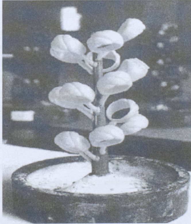
Şekil 4.4 Düzenlenmiş dereceli hassas döküm mum ağacı (WGC, 1995)
