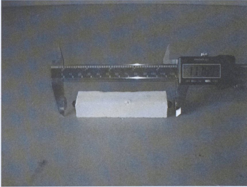
Şekil 8.5 Genleşme ölçümleri
