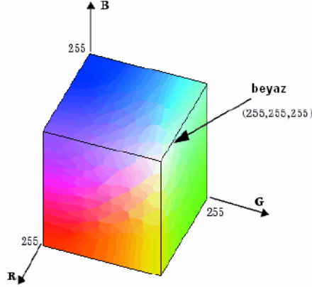
Şekil 2.1 RGB uzayı
