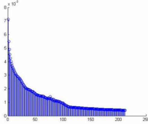
Şekil 8.7 İteratif eğitim
