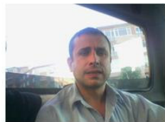
ycbcr ten
