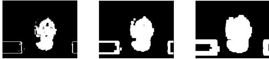
Şekil 2.5 Yayma
