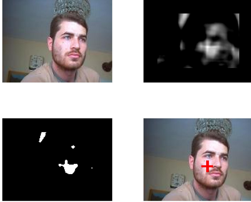
Şekil 3.2 Şablon eşleme
