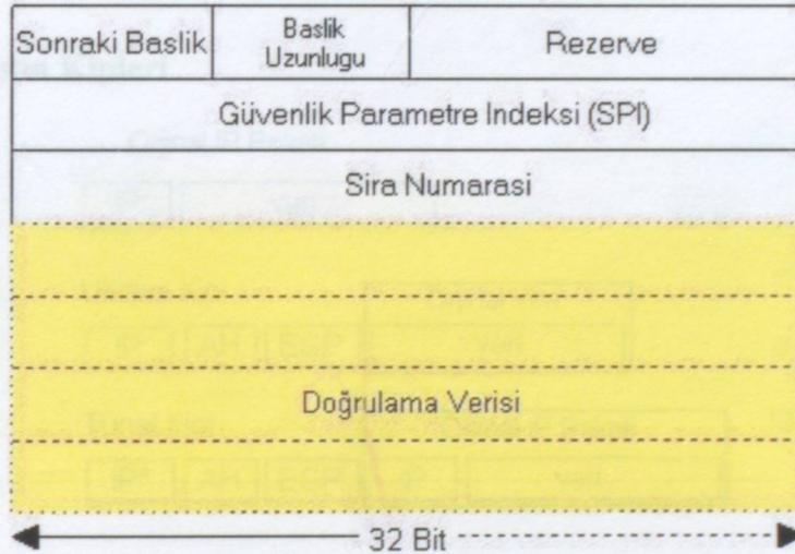
Şekil 8-6 Doğrulama başlığı formatı
