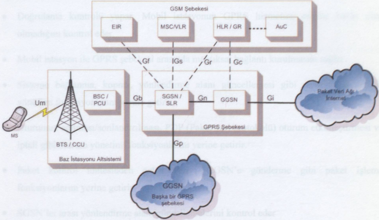
Şekil 4-1 GPRS Mimarisi
