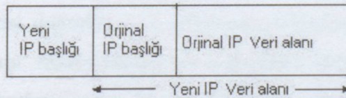
Şekil 8-4 Güvenli IP paketi
