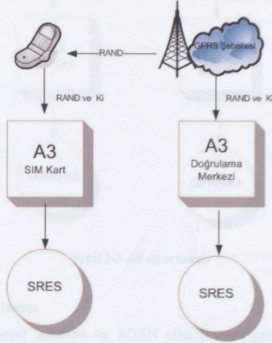
Şekil 7-2 A3 algoritması
