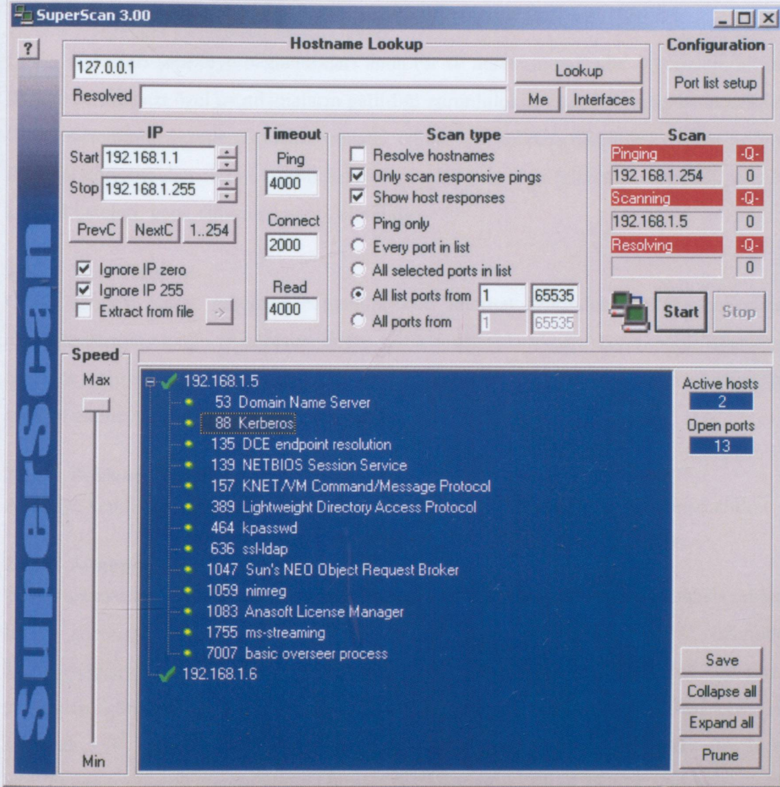
Şekil 2-4 SuperScan tarama sonucu
