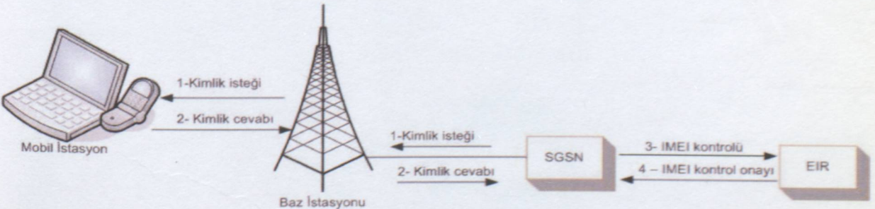
Şekil 7-7 kimlik doğrulama prosedürü
