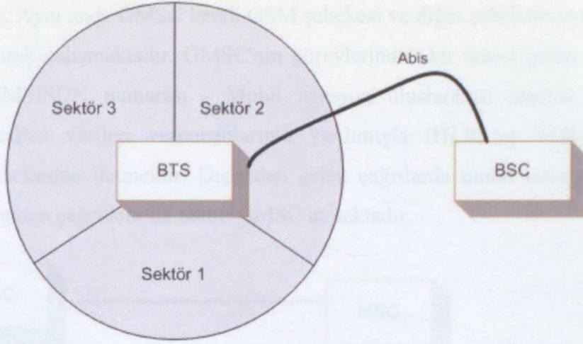
Şekil 3-3 120 Derece sektörleme
