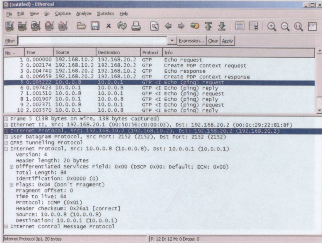
Şekil 14-2 SGSN ve GGSN arasındaki trafiğin analizi
