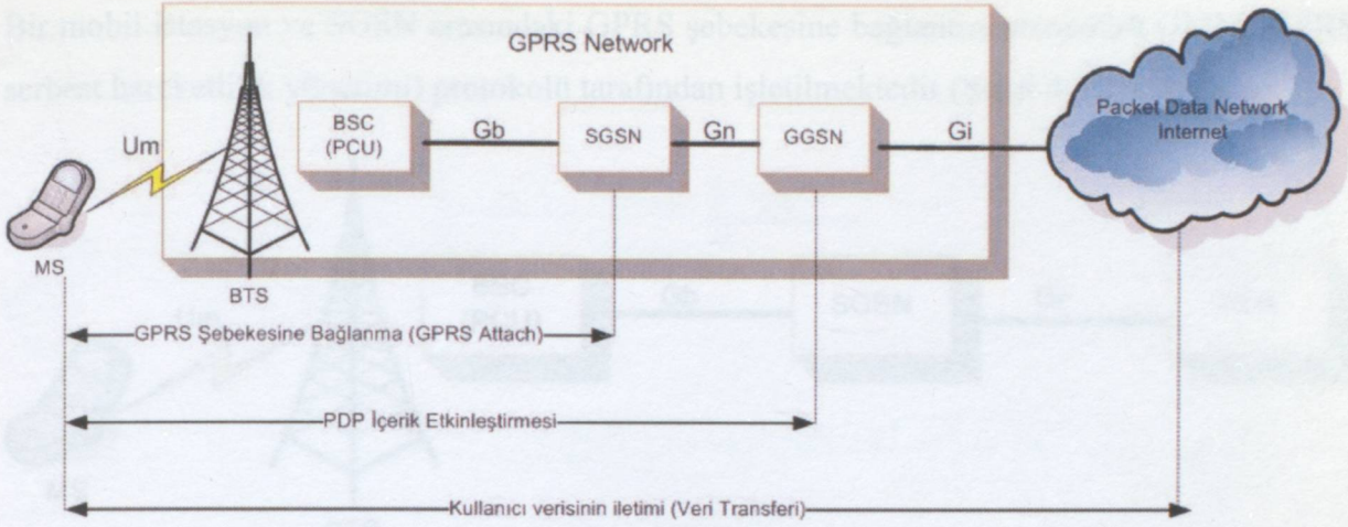
Şekil 4-2 GPRS prosedürleri
