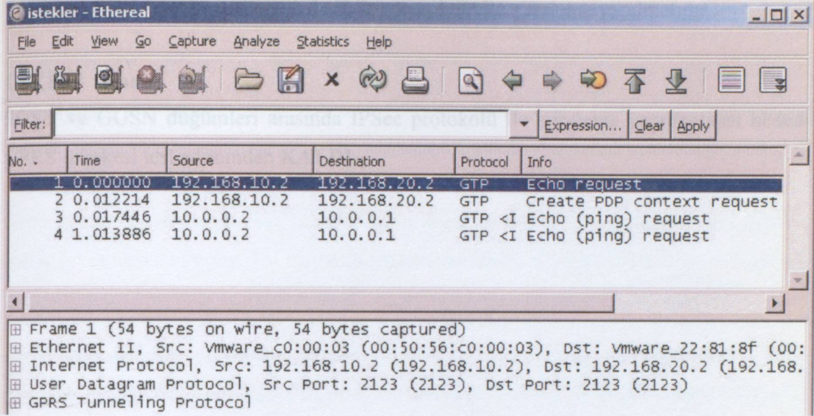
Şekil 14-15 PDP içerik etkinleştirmesine ait GTP paketleri
