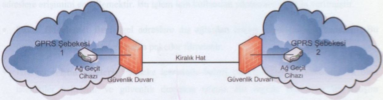
Şekil 9-1 Doğrudan bağlantı
