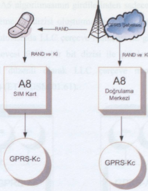
Şekil 7-3 A8 algoritması
