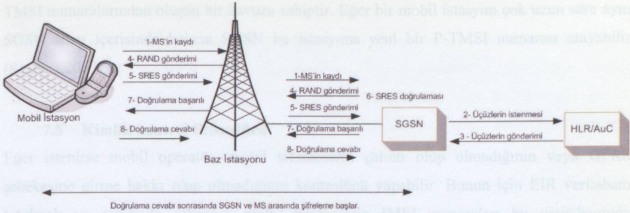
Şekil 7-6 Şifreleme prosedürü
