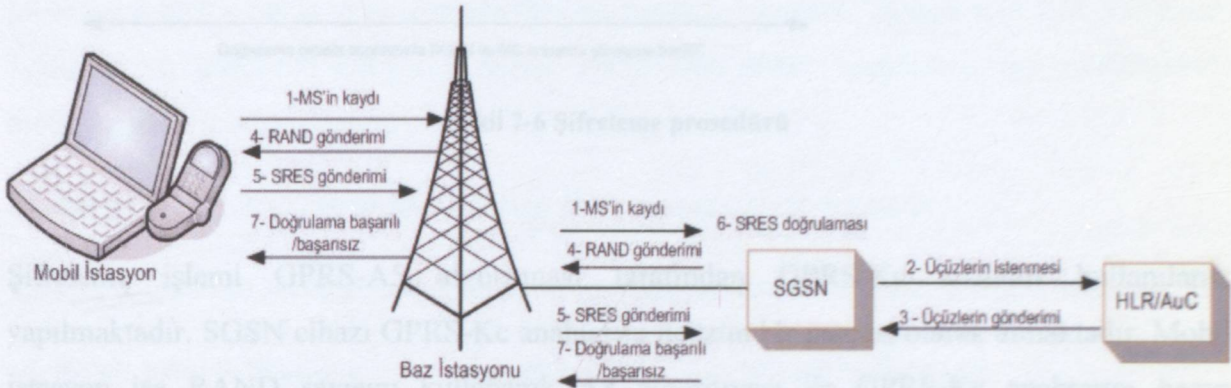
Şekil 7-5 Doğrulama prosedürü
