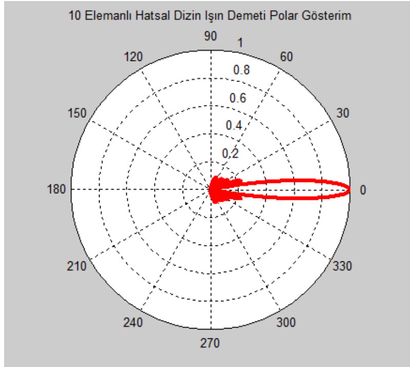
Şekil 2. 15 10 elemanlı hatsal dizin ışın demeti polar gösterim
