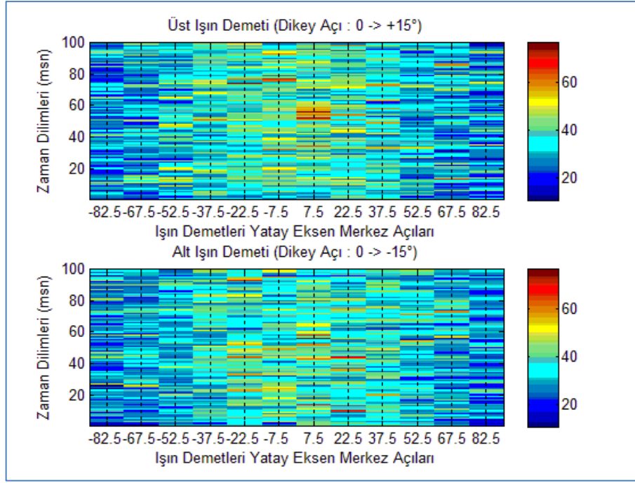
Şekil 4. 12 SGO = -14.5 dB için zaman alanı ışın demetlemesiyle hedef tespiti
