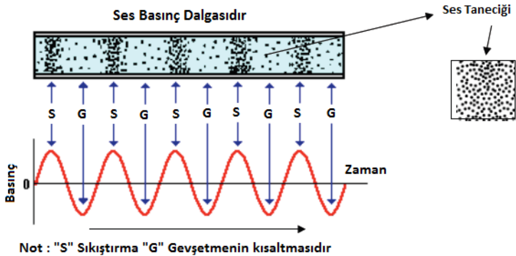
Şekil 2. 1 Sesin oluşumu
