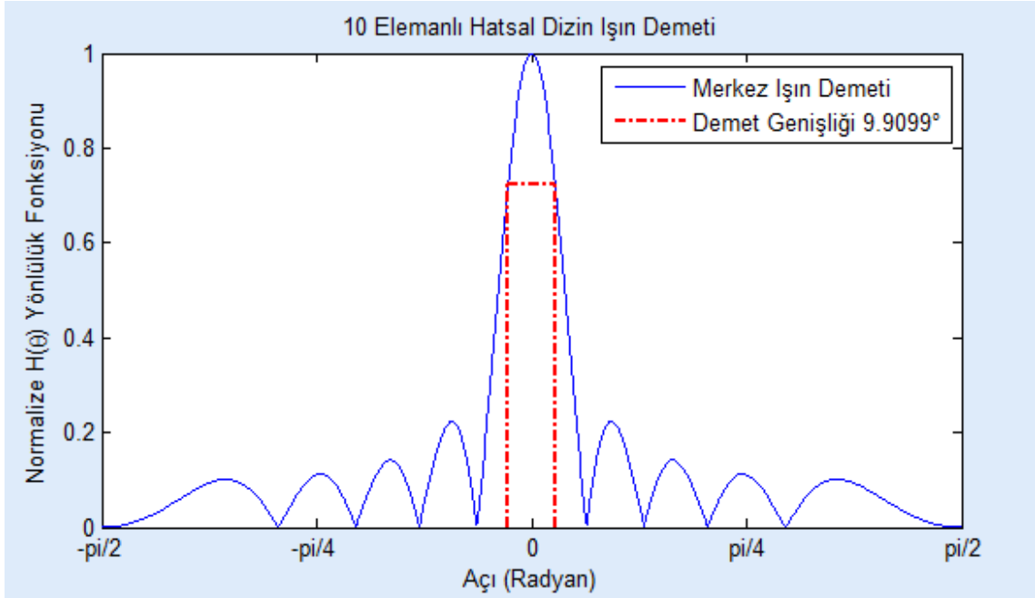
Şekil 2. 14 10 elemanlı hatsal dizin ışın demeti genişliği
