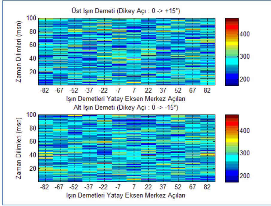
Şekil 4. 17 SGO = -26.5 dB için FFT ile frekans alanı ışın demetlemesiyle hedef tespiti
