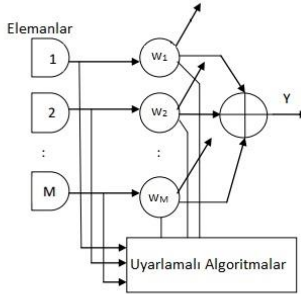
Şekil 3. 1 Uyarlamalı ışın demetleyicisi genel yapı
