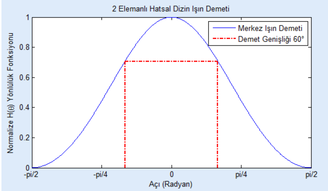
Şekil 2. 10 2 elemanlı hatsal dizin ışın demeti genişliği
