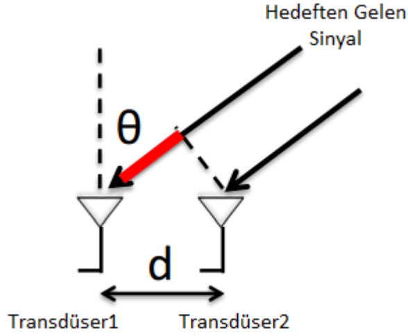
Şekil 2. 6 Hedeften yayılan sinyallerin transdüser \theta açısıyla gelişi
