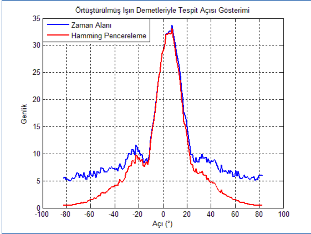
Şekil 4. 20 SGO = 0 dB zaman alanı için örtüşürülmüş ışın demetleri grafiği
