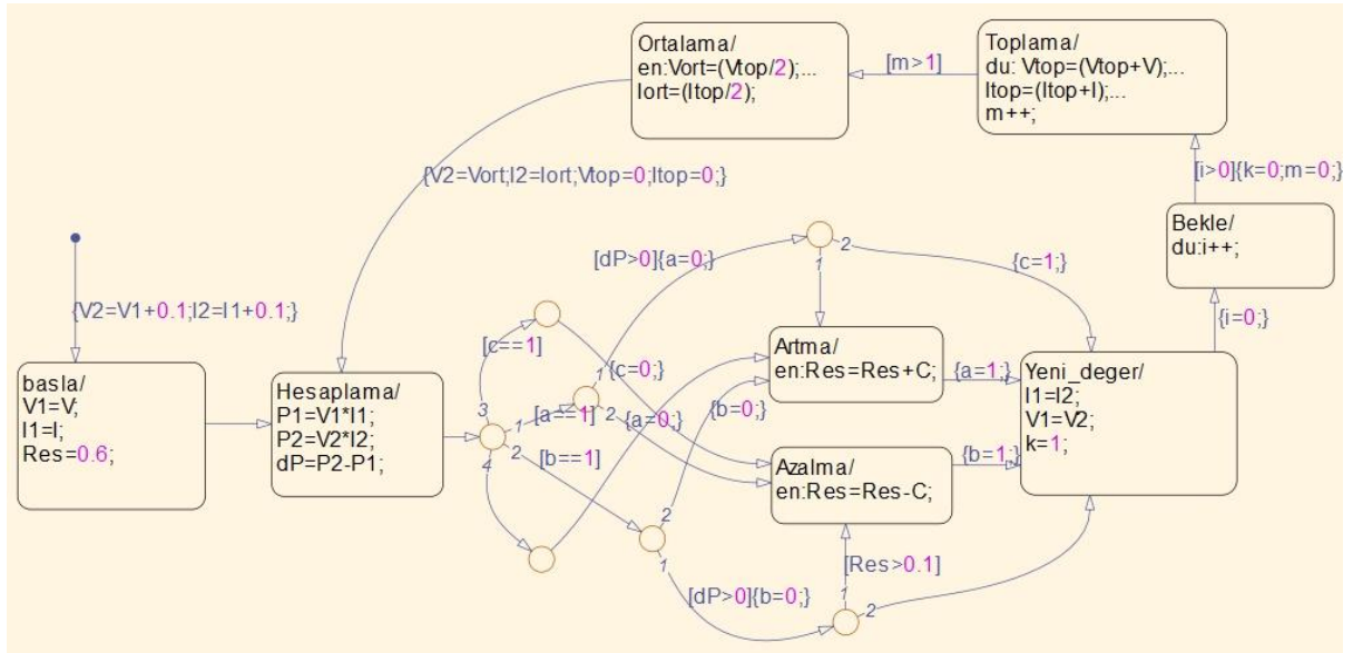
Şekil 4. 16 P&O algoritması Stateflow şeması
