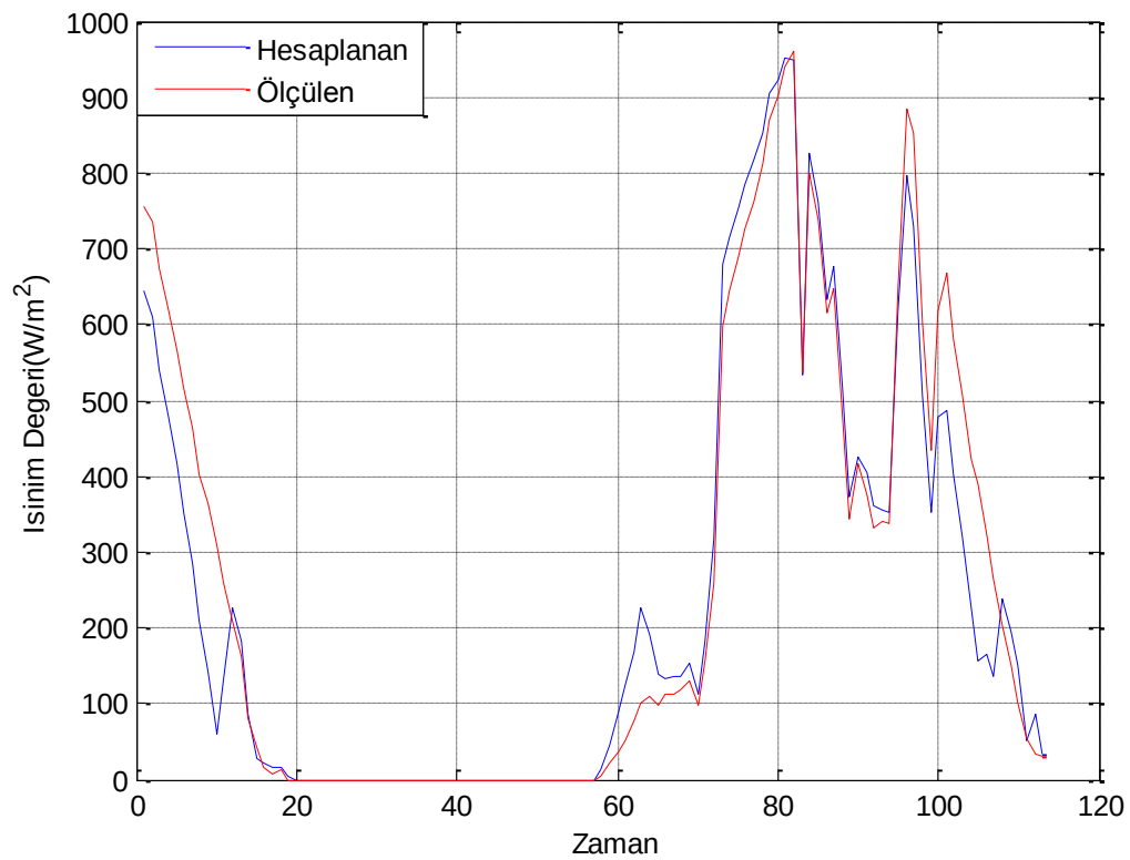
Şekil 4. 6 Eğimli yüzeye gelen ışıınımın gerçek ortam şartlarında ölçülen değeriyle karşılaştıırılması
