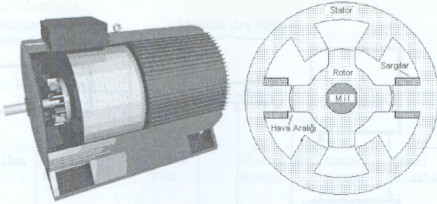
Şekil 2.11 Basit bir jeneratör ve stator-rotor aksamı (Güney, 2001)
