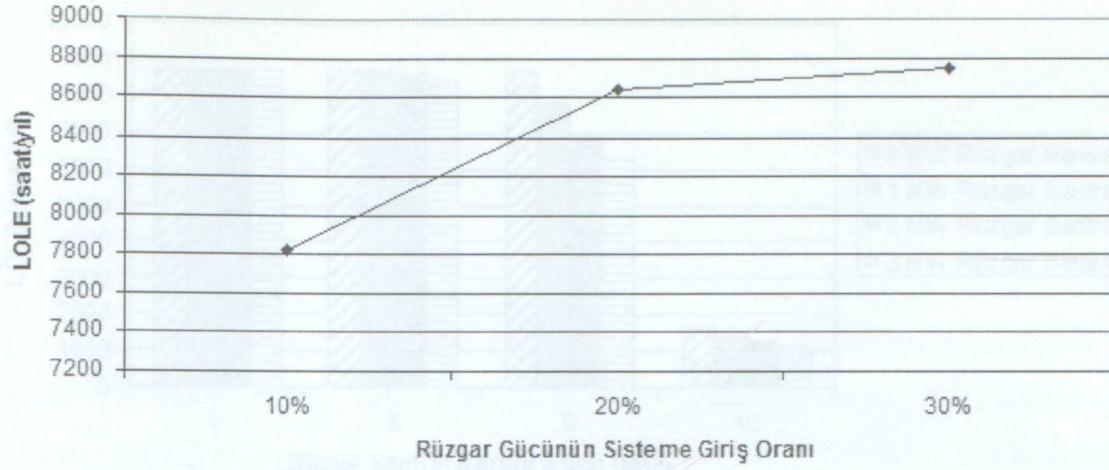
Şekil 5.13 LOLE'nin şebeke giriş oranlarına göre değişimi
