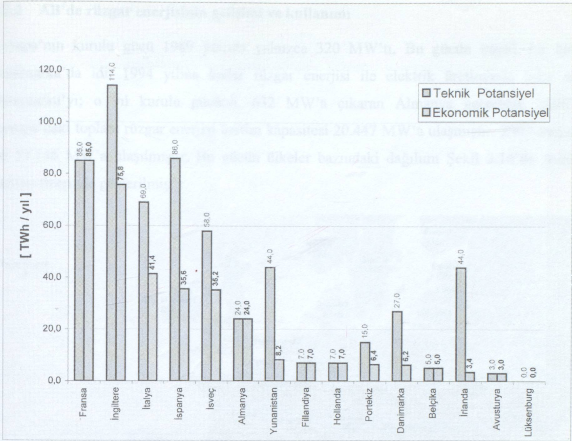
Şekil 3.13 AB rüzgar potansiyeli (Akalin, 2005b)
