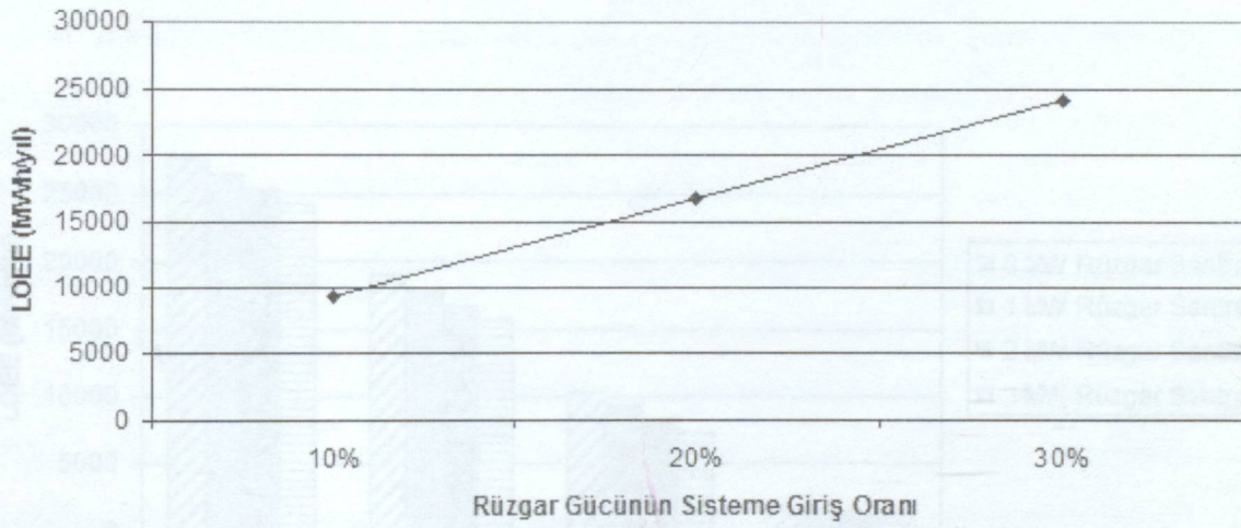
Şekil 5.14 LOEE'nin şebeke giriş oranlarına göre değişimi
