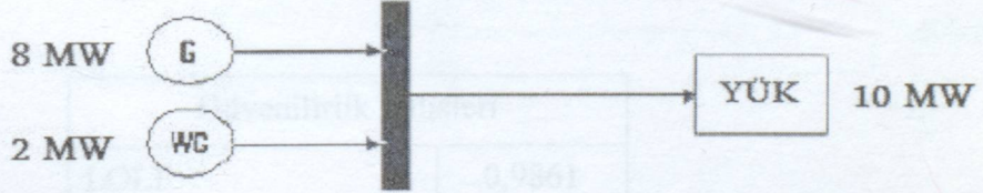
Şekil 5.9 Şebekeye giriş oranının % 20 olduğu durum
