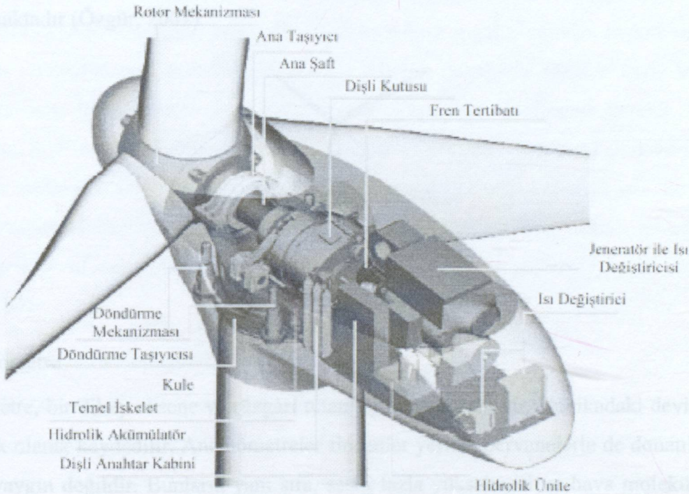
Şekil 2.9 Bir rüzgar türbini üzerindeki ekipmanlar ve konumları
