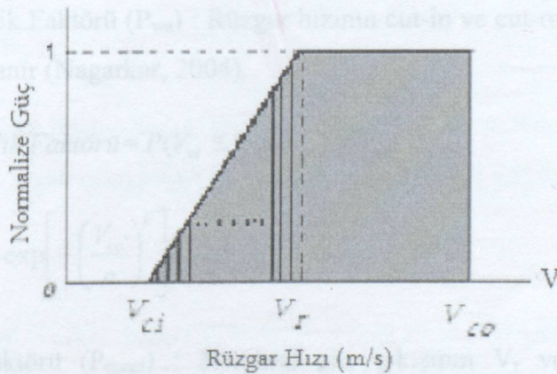
Şekil 4.5 Yaklaşık güç çıkış eğrisi
