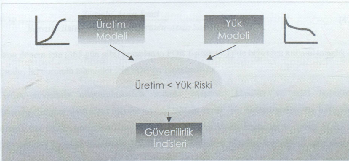
Şekil 4.3 Üretim güvenilirliği modelinin elemanları
