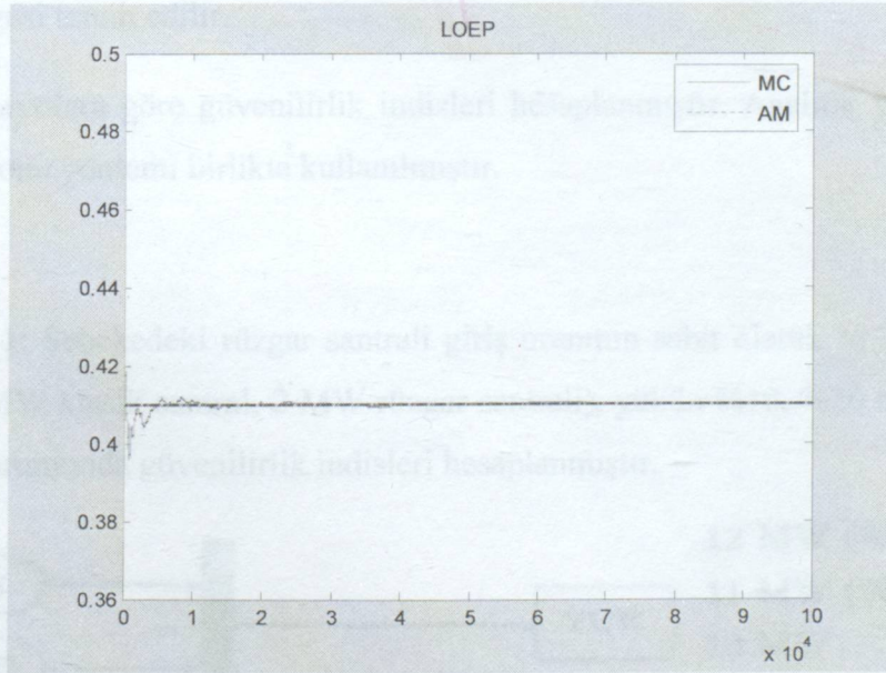
Şekil 4.15 LOEP indisinin Monte Carlo simülasyonu
