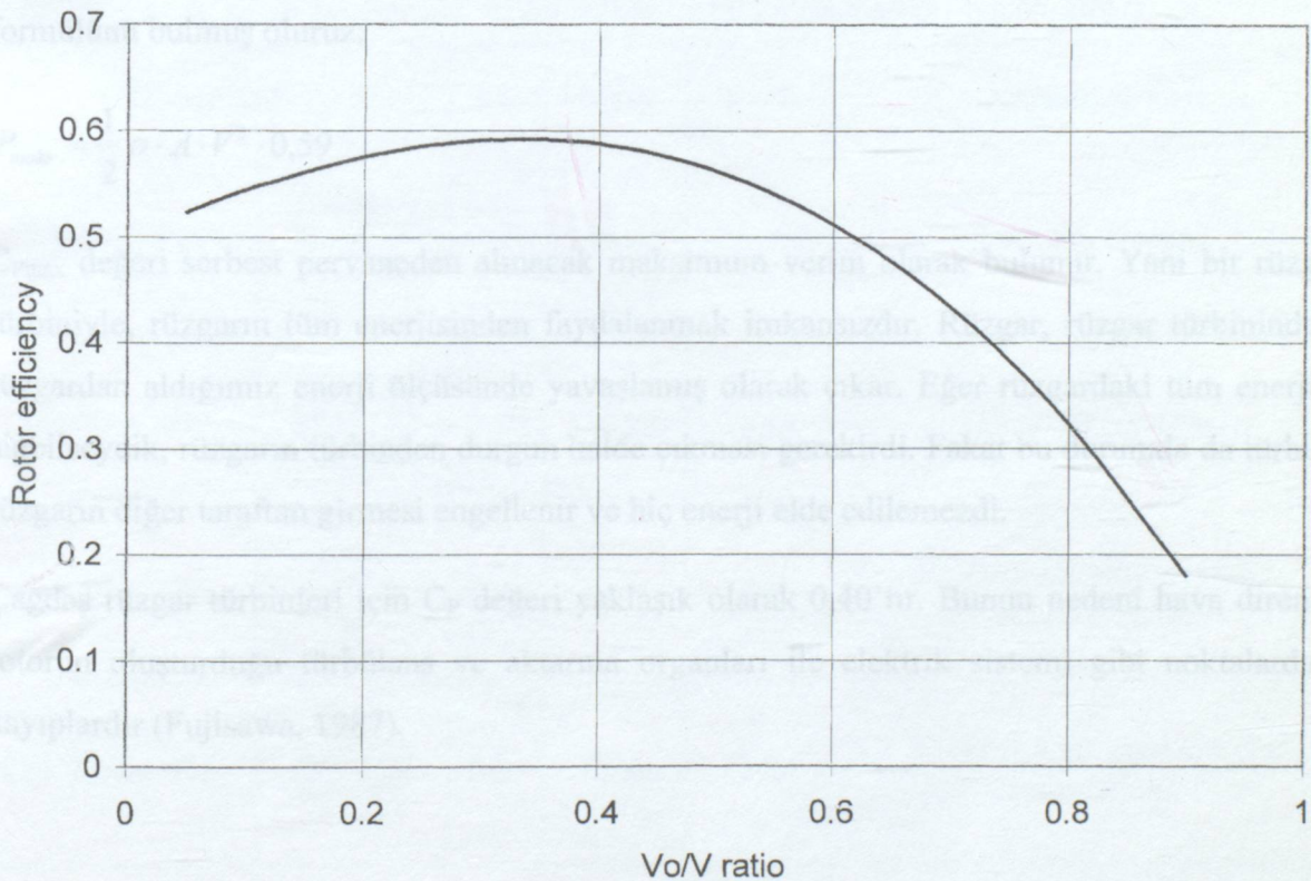
Şekil 2.4 C_p - V_0/V değişimi (Betz, 1994)
