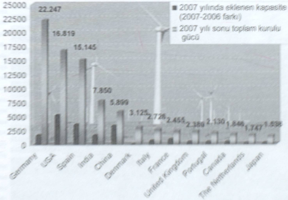
Şekil 3.6 2007'de kurulan rüzgar güçleri ve yıl sonu rüzgar kurulu gücü (WWEA, 2008)
