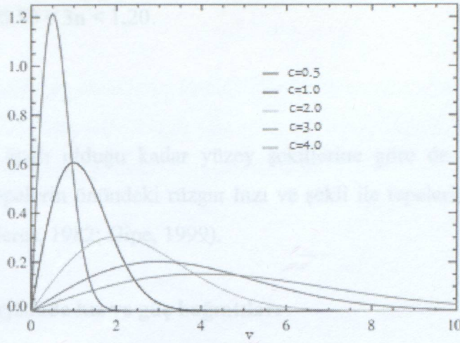
Şekil 2.2 Rayleigh dağılımına c parametresinin değişiminin etkisi
