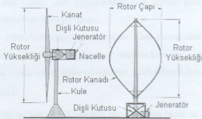
Şekil 2.6 Yatay ve dikey eksenli rüzgar türbinleri (Şen, 2003)
