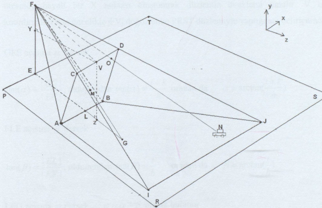
Şekil 5.2 Geometrik düzeltme hesaplaması
