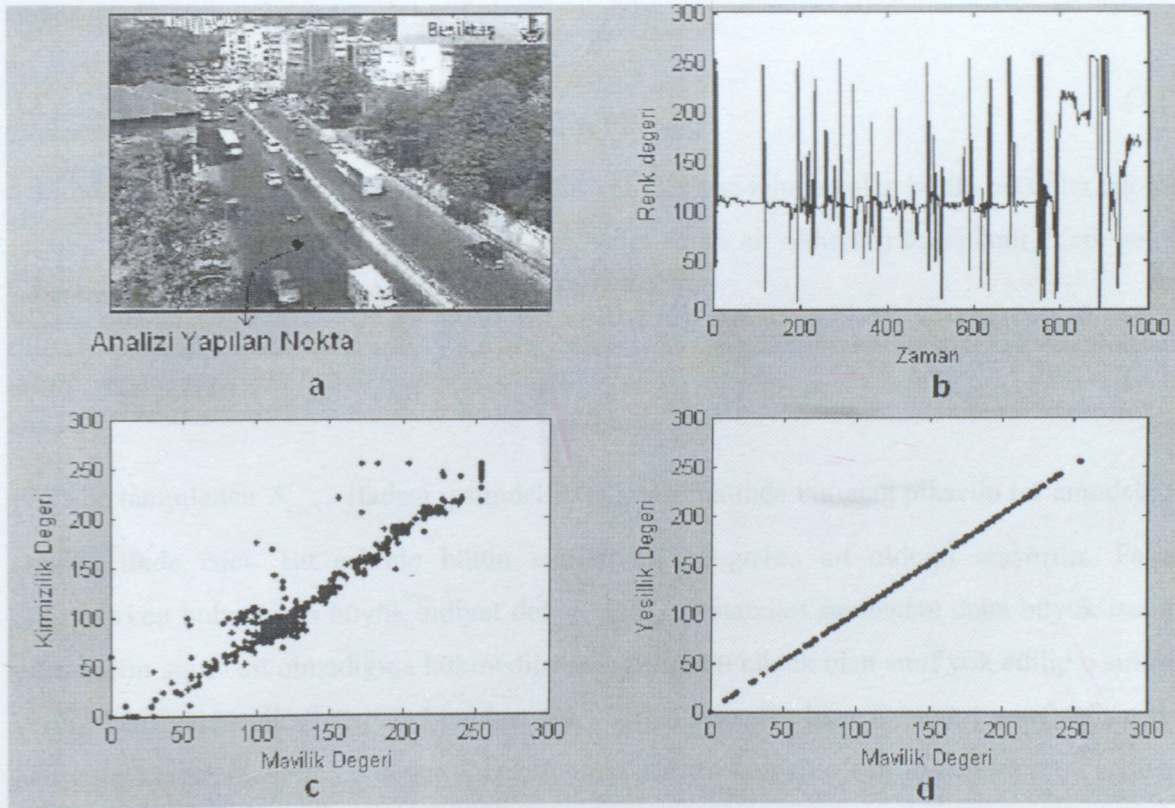
Şekil 7.3 a)Analizi yapılan nokta b)Bu noktanın zamana bağlı ışık şiddeti c)Bu noktanın kırmızı-mavi ekseninde aldığı değerler d)Bu noktanın yeşil-mavi ekseninde aldığı değerler
