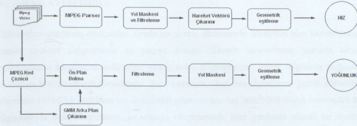
Şekil 2.1 Önerilen sistemin akış şeması
