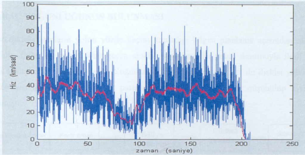
Şekil 6.2 Anlık hız ve 2 saniye periyotlu zaman dilimi ortalama hız
