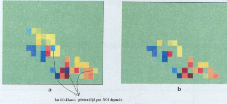
Şekil 4.3 a)Süzgeçten önceki MV b)Süzgeçten sonraki MV
