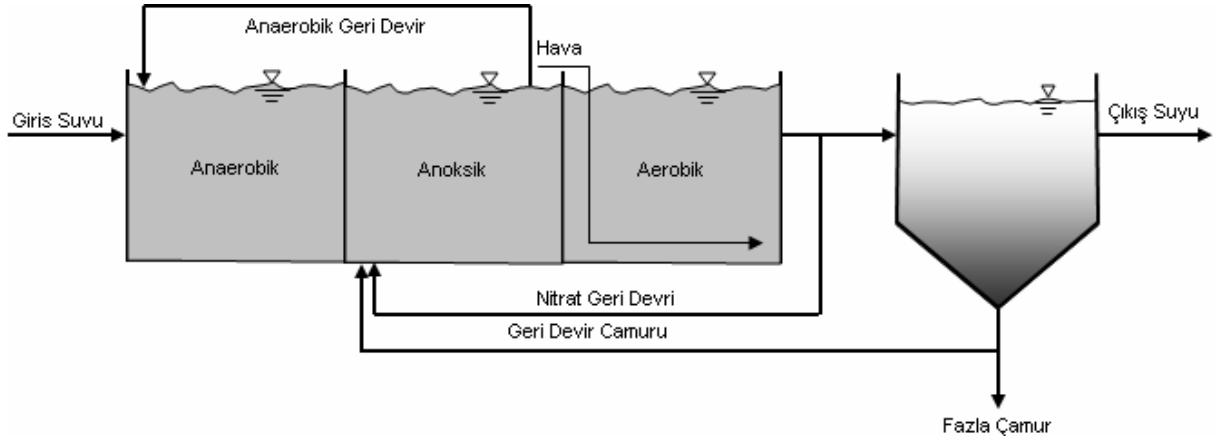
Şekil 4.10 UCT prosesinin şematik görünümü [16].
