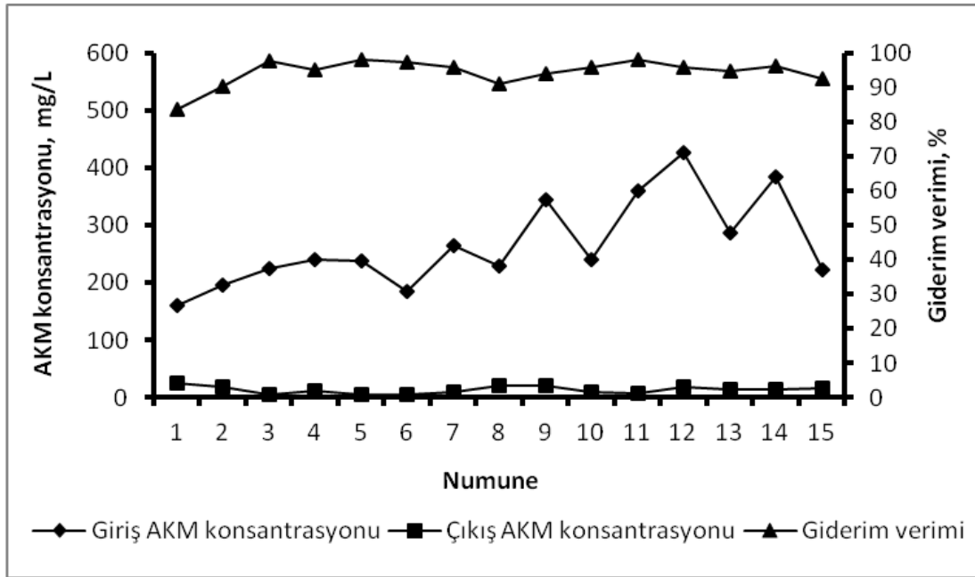
Şekil 7.1 Yeni geliştirilen modifiye beş kademeli Bardenpho prosesinde giriş-çıkış AKM konsantrasyonları ve giderim verimleri.
