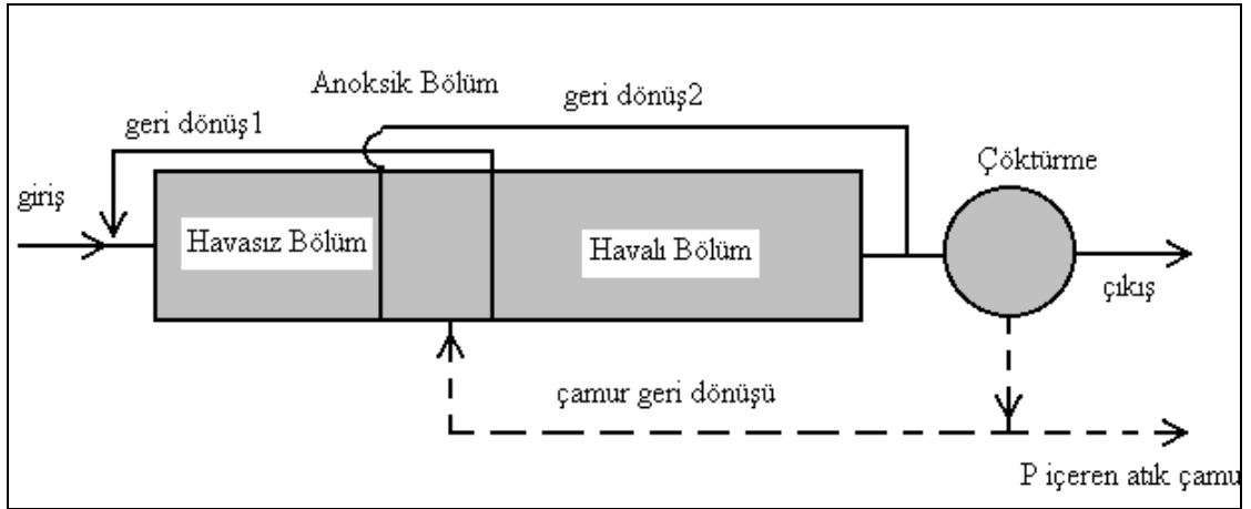
Şekil 4.11 VIP prosesinin şematik görünümü [16].
