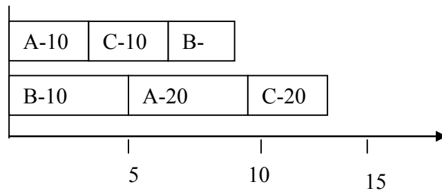
Şekil 3.9 Atama tablosu 7
