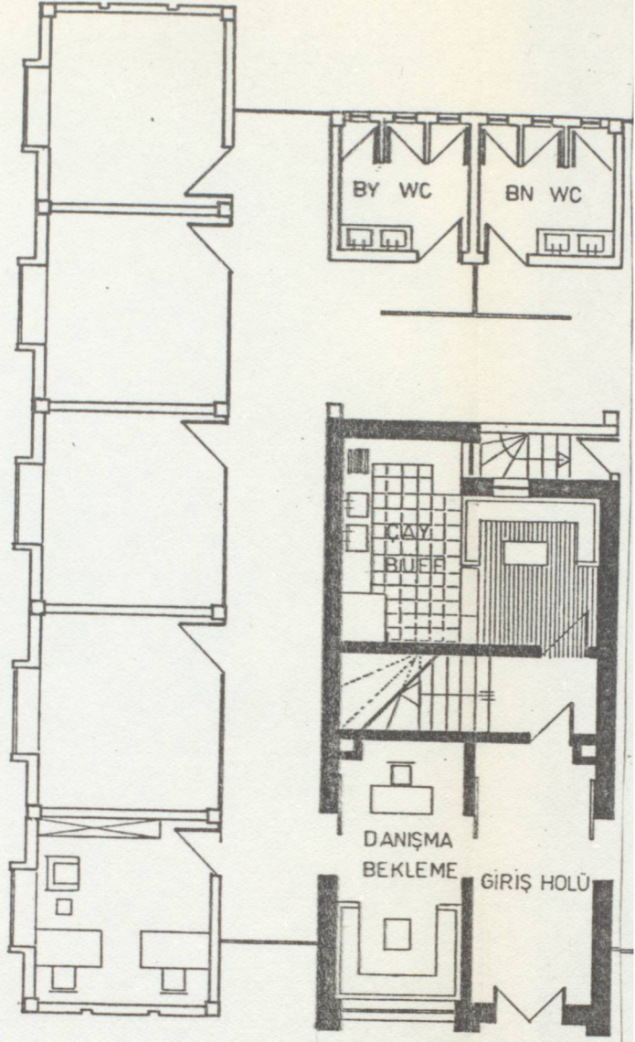
GİRİŞ KATI PLANI Ö: 1/100
