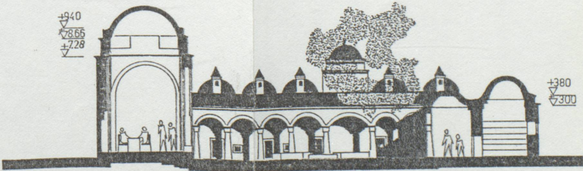
PEYKLER MEDRESESİ: KÜTÜPHANE
