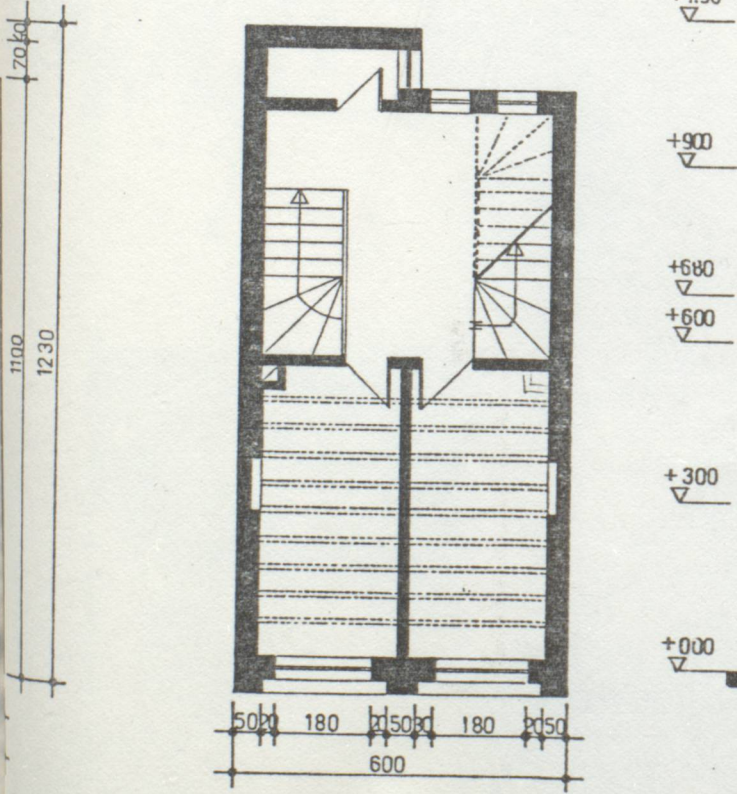
NORMAL KAT RÖLÖVESİ Ö: 1/100
