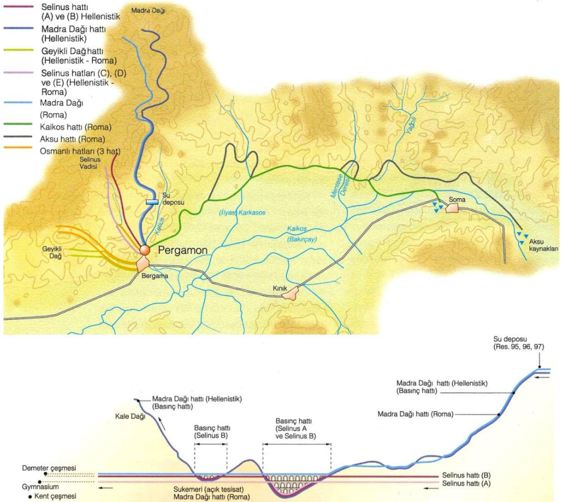
Şekil 5.8 Pergamon Su Dağıtım Şebekesinin Genel Plan ve Kesiti (Radt, 2002: 148)
