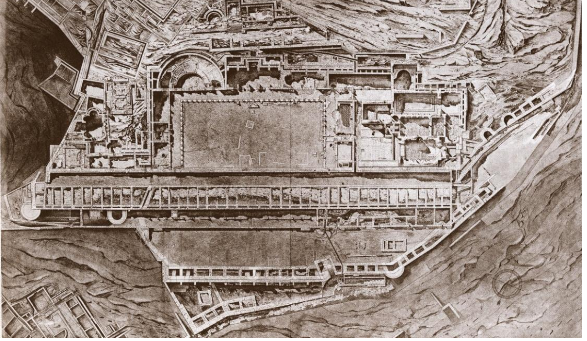
Şekil 5.13 Büyük Gymnasion ve Hera Tapınağı'nın Temel Planı (Radt, 2002: 113)
