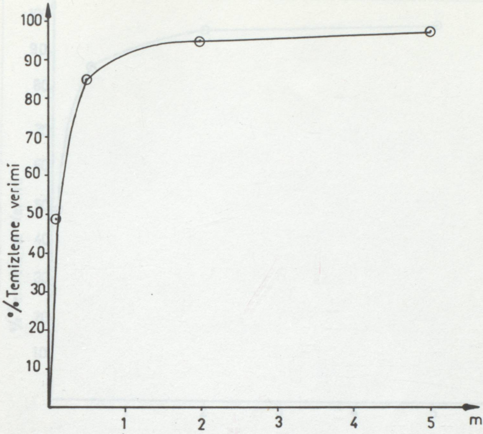
ŞEKİL 3.12.3. 50 mg/l'nin TEMİZLEME VERİMİ GRAFİĞİ
