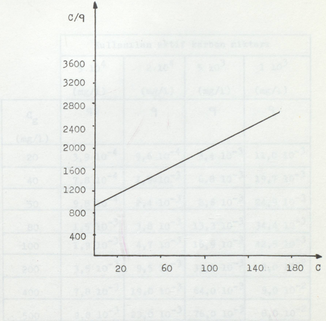
ŞEKİL 3.10.8 500 mg/l İÇİN LANGMUIR İZOTERMİ
