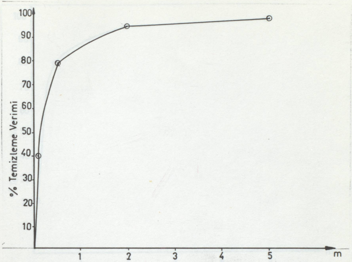
ŞEKİL 3.12.6 200 mg/l'nin TEMİZLEME VERİMİ GRAFİĞİ
