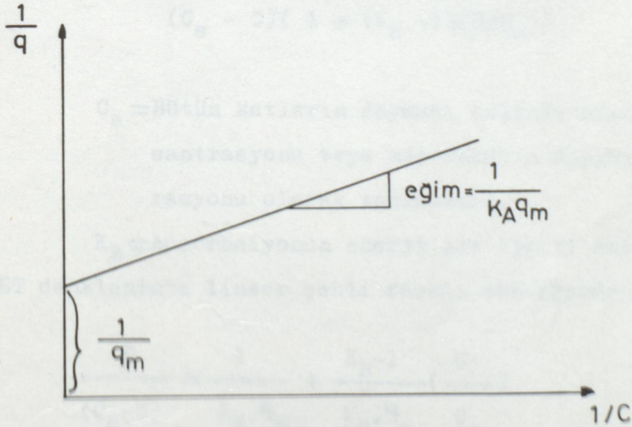
Sekil 2.3.8.1. LANGMUIR ADSORBSİYON İZOTERMLERİNİN LINEER ŞEKİLLERİ
