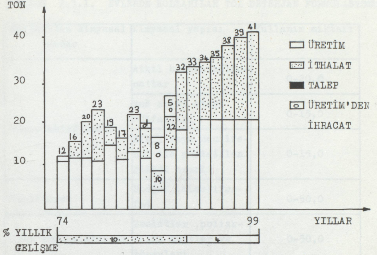
ŞEKİL 2.1.2 ALKİL BENZENLERİN TÜRKİYEDEKİ TÜKETİMİ
