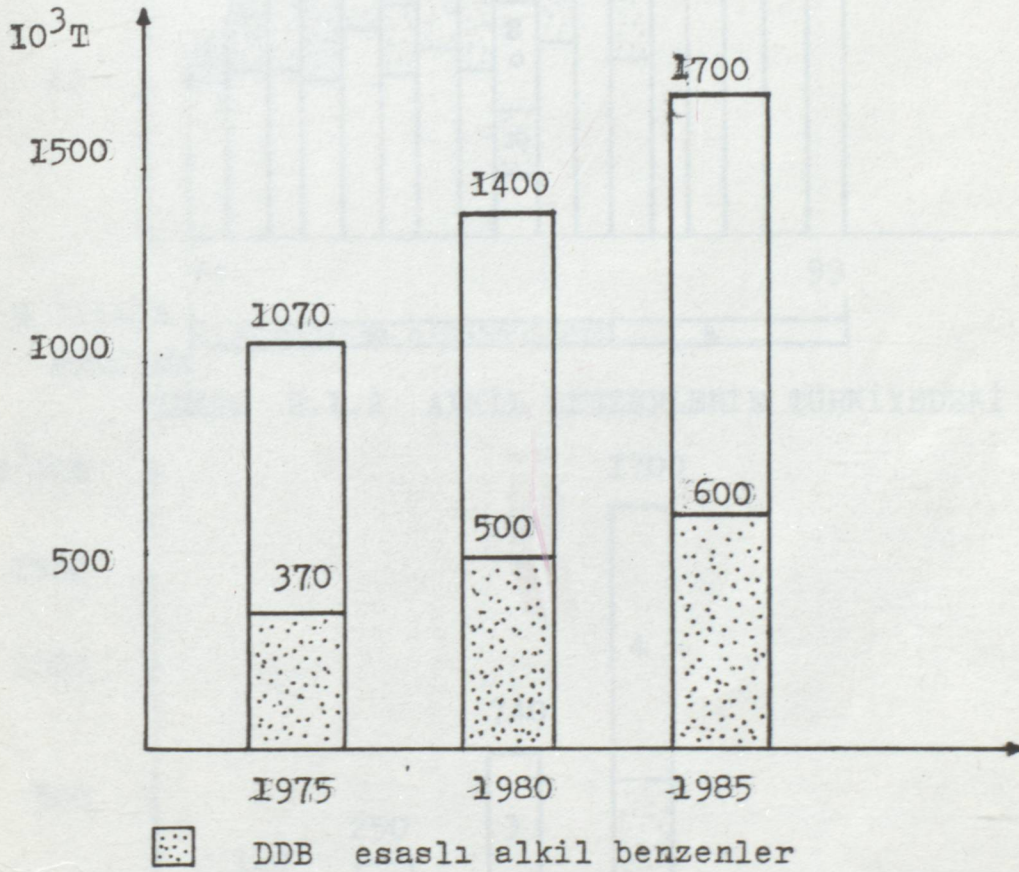
ŞEKİL 2.1.1. ALKİL BENZENLERİN DÜNYADAKİ ÜRETİMİ
