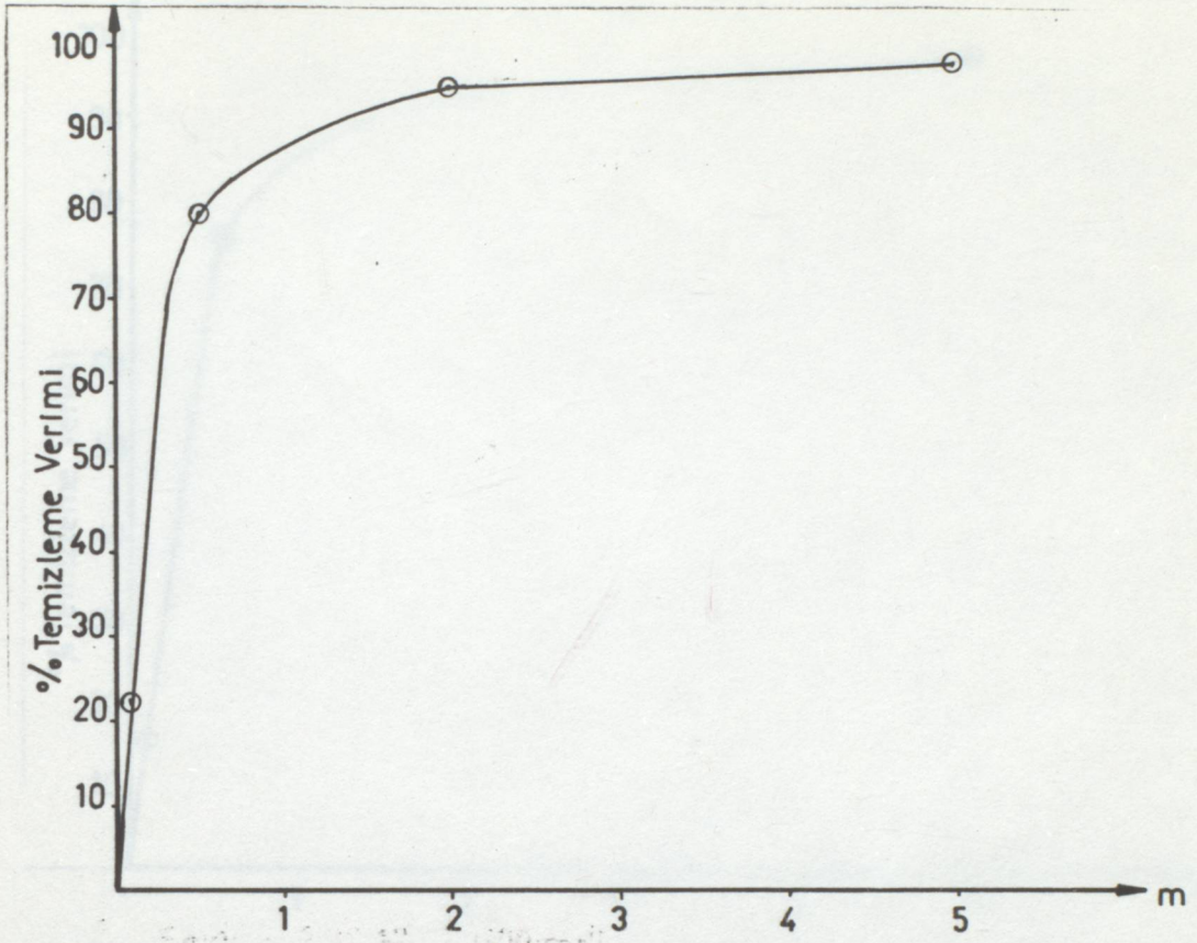
ŞEKİL 3.12.7. 400 mg/l'nin TEMİZLEME VERİMİ GRAFIGİ
