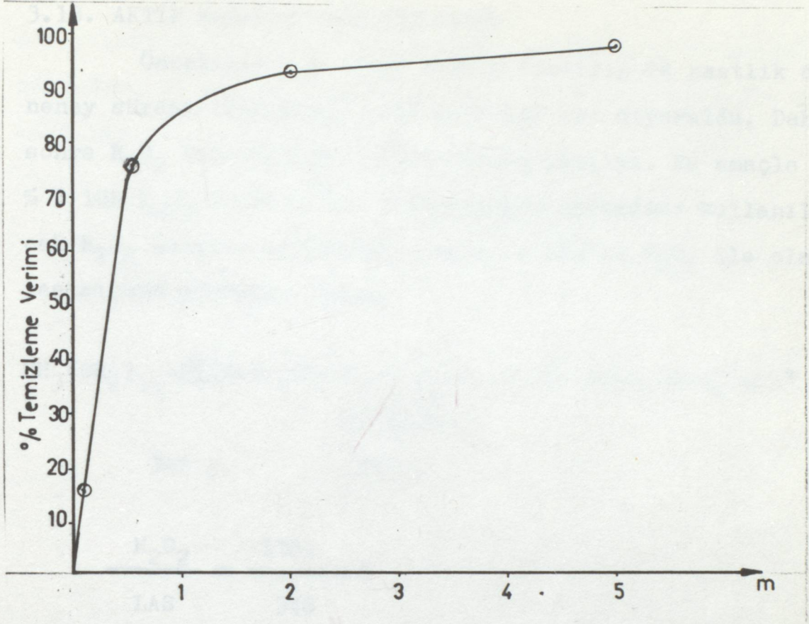
ŞEKİL 3.12.8. 500 mg/l'nin TEMİZLEME VERİMİ GRAFİĞİ
