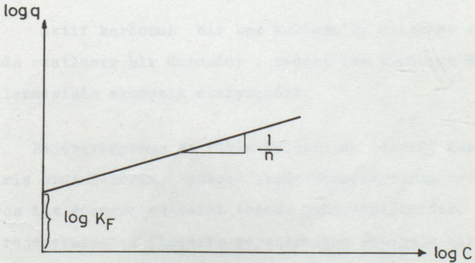
Şekil 2.3.8.3 Lineerleştirilmiş Freundlich Adsorbsiyon İzotermi
