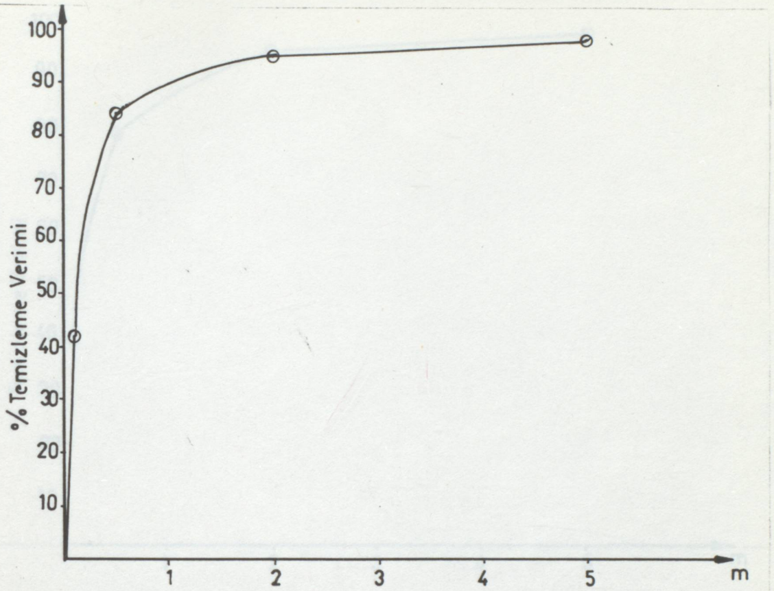
ŞEKİL 3.12.5. 100 mg/l'nin TEMİZLEME VERİMİ GRAFİĞİ
