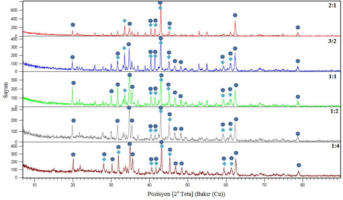
Şekil 6. 25 Termal metot ile 1000°C ve 240 dakikada üretilen ürünlerin XRD paternleri
