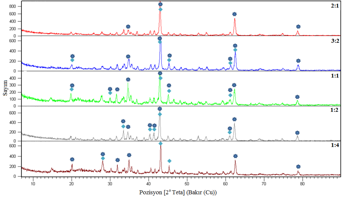
Şekil 6. 23 Termal metot ile 1000°C ve 30 dakikada üretilen ürünlerin XRD paternleri
