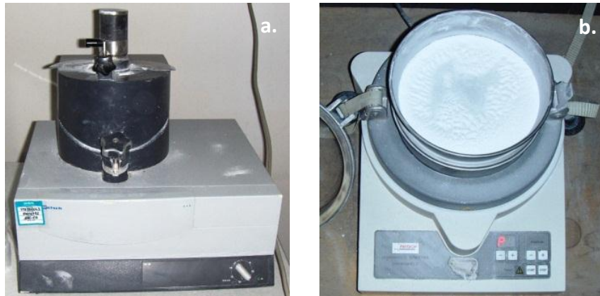
Şekil 5. 1 Kullanılan ekipmanlar, a. Retsch marka agat havan, b. Fritsch marka elek
