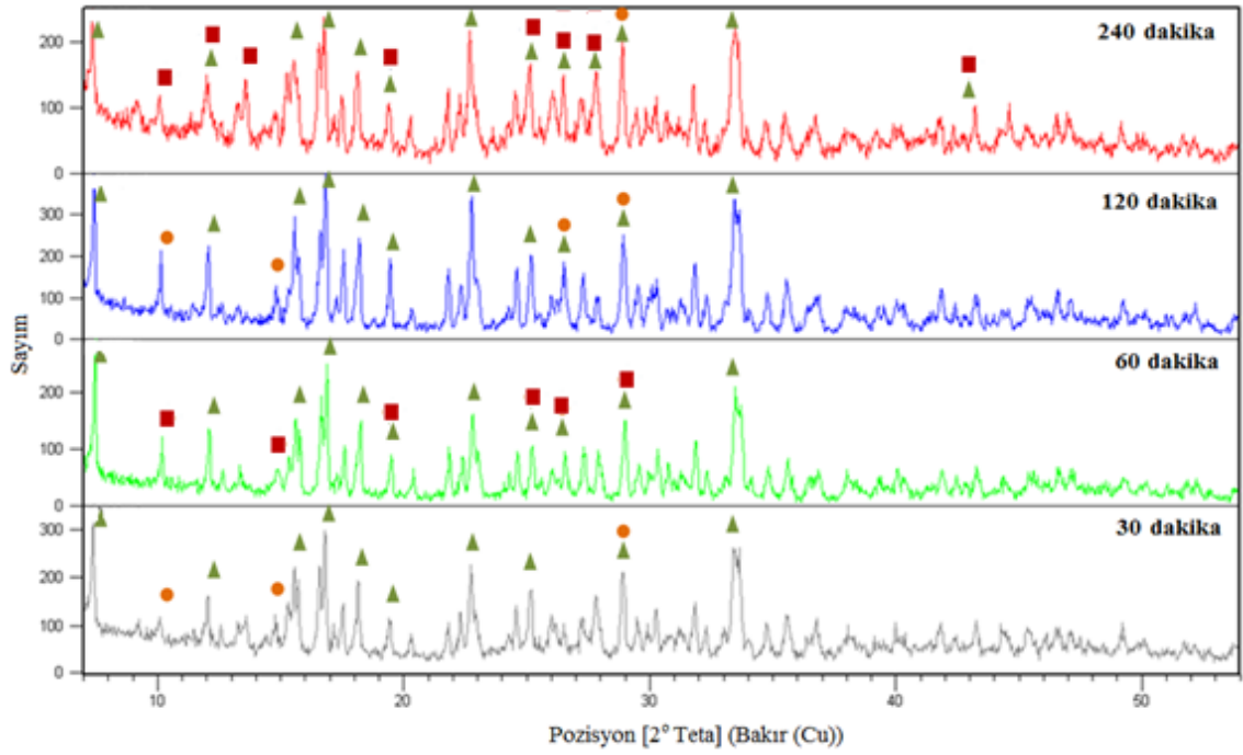
Şekil 6. 5 Hidrotermal metot ile 80°C' de sentezlenen ürünlerin XRD paternleri ▲-01-076-540, ●-01-070-1902, ■-01-073-0638
