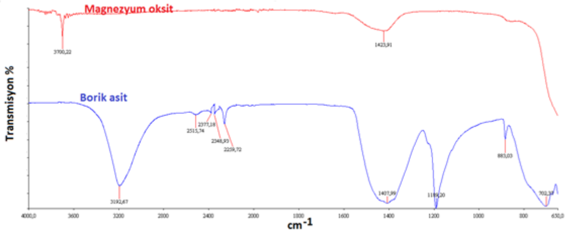
Şekil 6. 2 Kullanılan hammaddelerin FT-IR spektrumu
