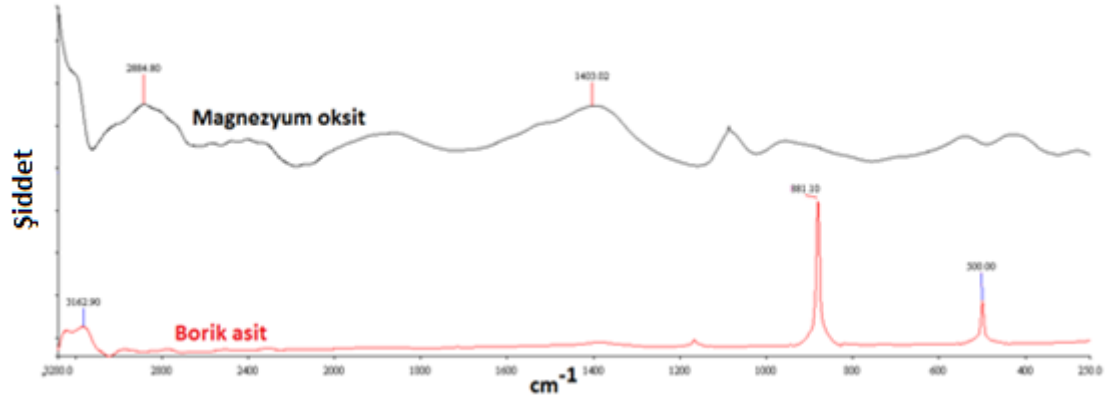
Şekil 6. 3 Kullanılan hammaddelerin Raman spektrumu
