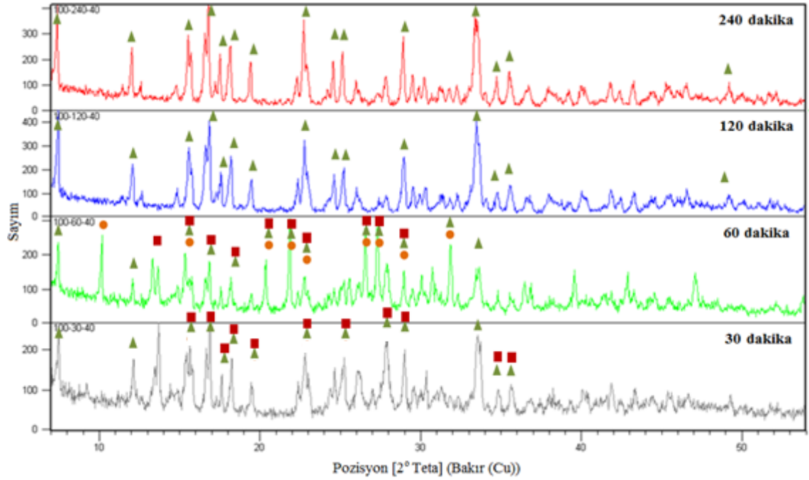
Şekil 6. 7 Hidrotermal metot ile 100°C' de sentezlenen ürünlerin XRD paternleri
