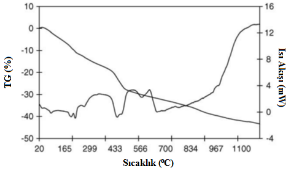
Şekil 4. 4 Sentezlenen numunenin termogravimetrik analizi [6]
