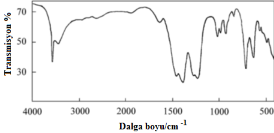
Şekil 4. 3 Sentezlenen numunenin FT-IR spektrumu [5]
