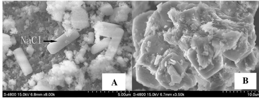
Şekil 4. 7 a. Sinterleme öncesi 120 saat malle öğütülen numune, b. Sinterleme sonrası 120 saat malle öğütülen numune [10]
