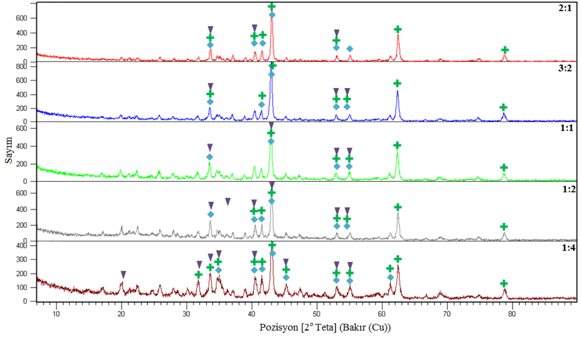
Şekil 6. 21 Termal metot ile 900°C ve 60 dakikada üretilen ürünlerin XRD paternleri
