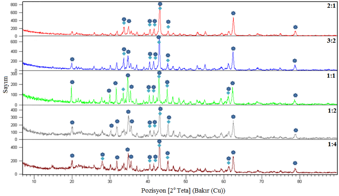
Şekil 6. 24 Termal metot ile 1000°C ve 60 dakikada üretilen ürünlerin XRD paternleri
