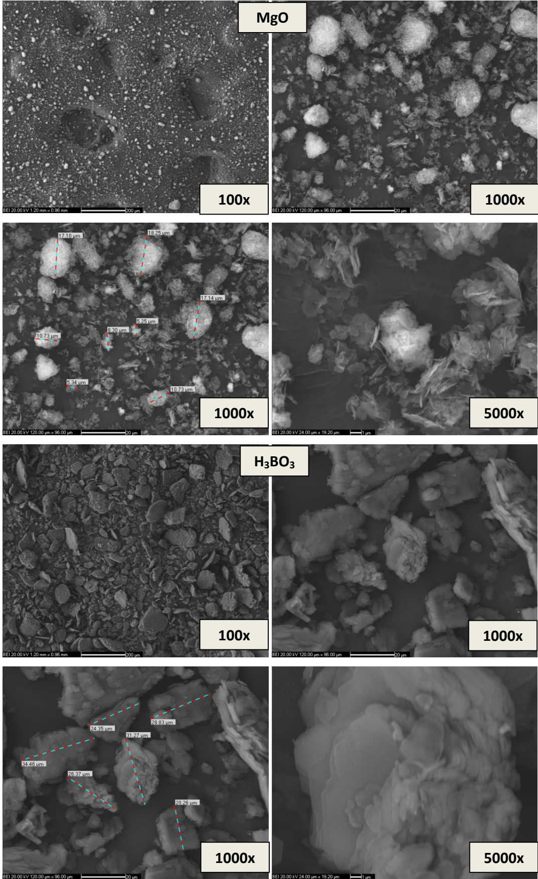
Şekil 6. 4 Kullanılan hammaddelerin SEM yüzey görüntüleri
