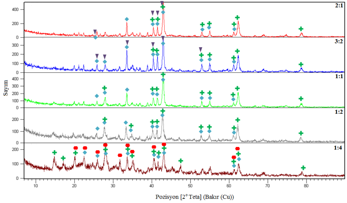
Şekil 6. 19 Termal metot ile 800°C ve 240 dakikada üretilen ürünlerin XRD paternleri
