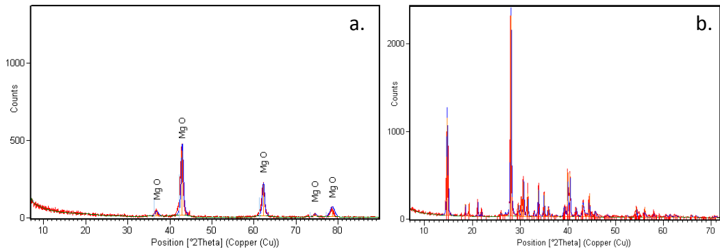
Şekil 6. 1 Kullanılan hammaddelerin XRD paternleri; a. MgO, b. H 3 BO 3
