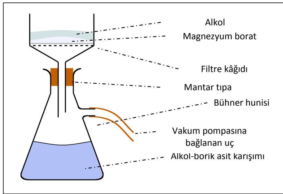
Şekil 5. 5 Hidrotermal reaksiyon sonrası ürün yıkama şematik gösterimi
