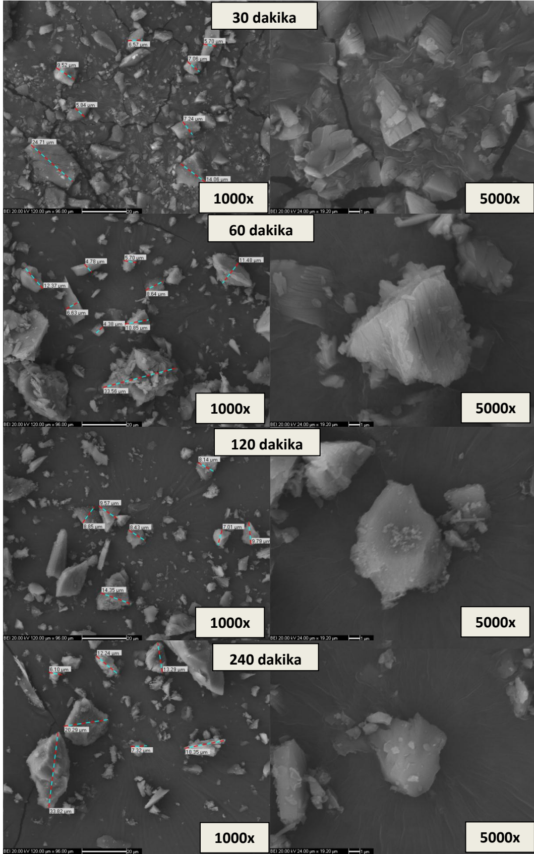
Şekil 6. 15 Hidrotermal metot ile 90°C' de sentezlenen ürünlerin SEM yüzey görüntüleri
