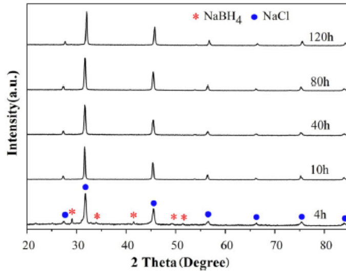
Şekil 4. 6 Mil ile öğütme işlem süresine göre XRD spektrumları [10]
