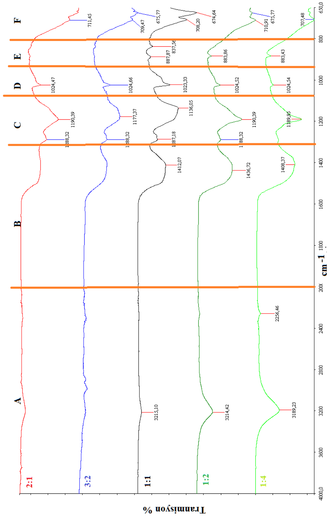
Şekil 6. 33 Termal metotla 1000°C ve 60 dakikada üretilen ürünlerin FT-IR spektrumları
