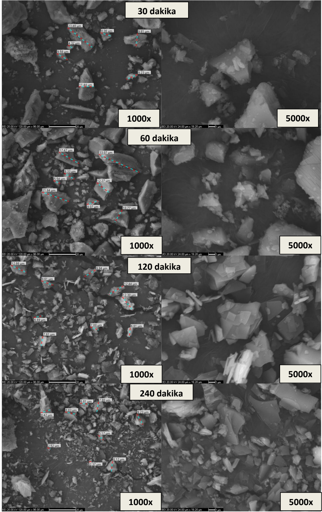
Şekil 6. 16 Hidrotermal metotla 100°C' de sentezlenen ürünlerin SEM yüzey görüntüleri
