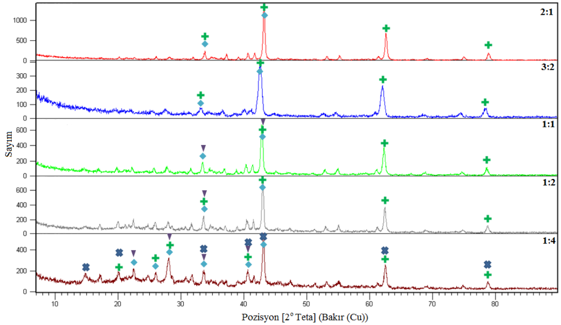
Şekil 6. 20 Termal metot ile 900°C ve 30 dakikada üretilen ürünlerin XRD paternleri
