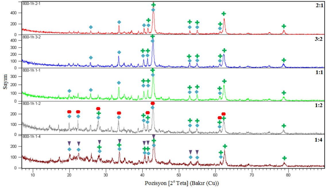
Şekil 6. 18 Termal metot ile 800°C ve 60 dakikada üretilen ürünlerin XRD paternleri
