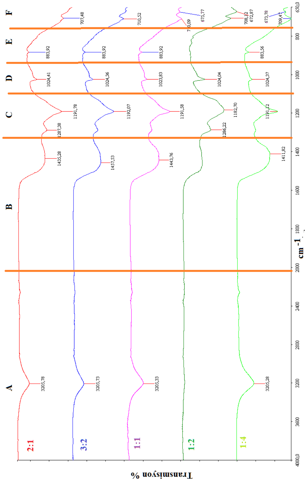
Şekil 6. 32 Termal metotla 1000°C ve 30 dakikada üretilen ürünlerin FT-IR spektrumları
