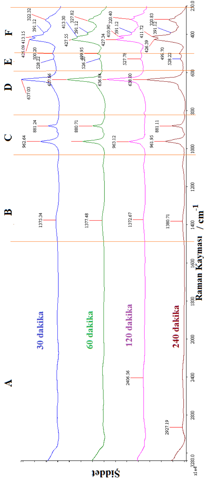
Şekil 6. 11 Hidrotermal metot ile 80^{\circ}\text{C} ' de sentezlenen ürünlerin Raman spektrumları
