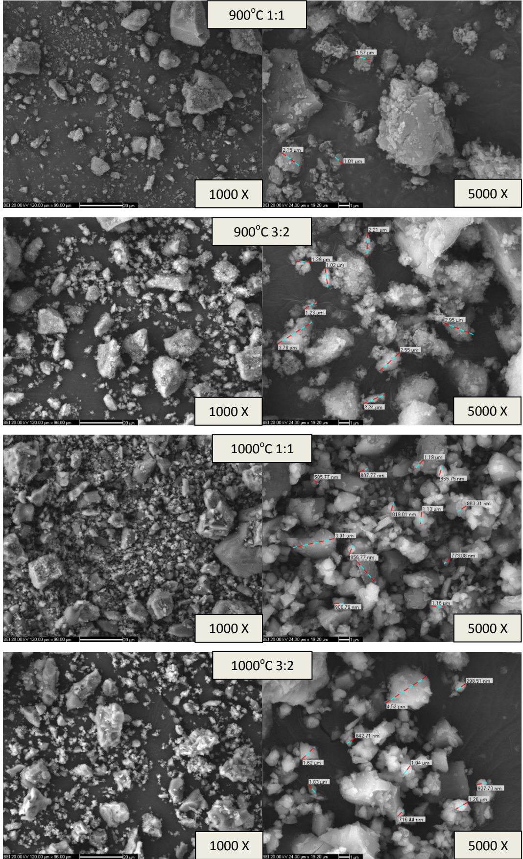
Şekil 6. 45 900-1000°C'de 3:2-1:1 oranları için 240 dakikada SEM yüzey görüntüleri
