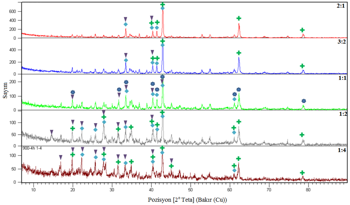
Şekil 6. 22 Termal metot ile 900°C ve 240 dakikada üretilen ürünlerin XRD paternleri
