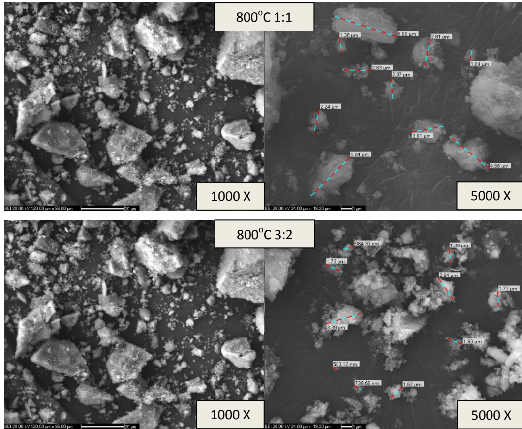
Şekil 6. 44 800°C'de 3:2-1:1 oranları için 240 dakikada SEM yüzey görüntüleri
