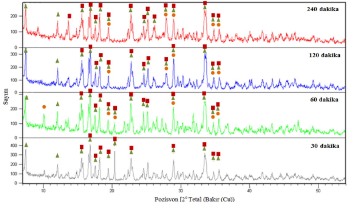
Şekil 6. 6 Hidrotermal metot ile 90°C' de sentezlenen ürünlerin XRD paternleri
