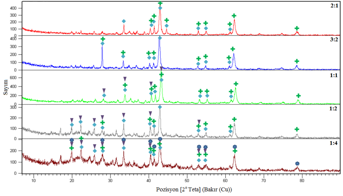
Şekil 6. 17 Termal metot ile 800°C ve 30 dakikada üretilen ürünlerin XRD paternleri
