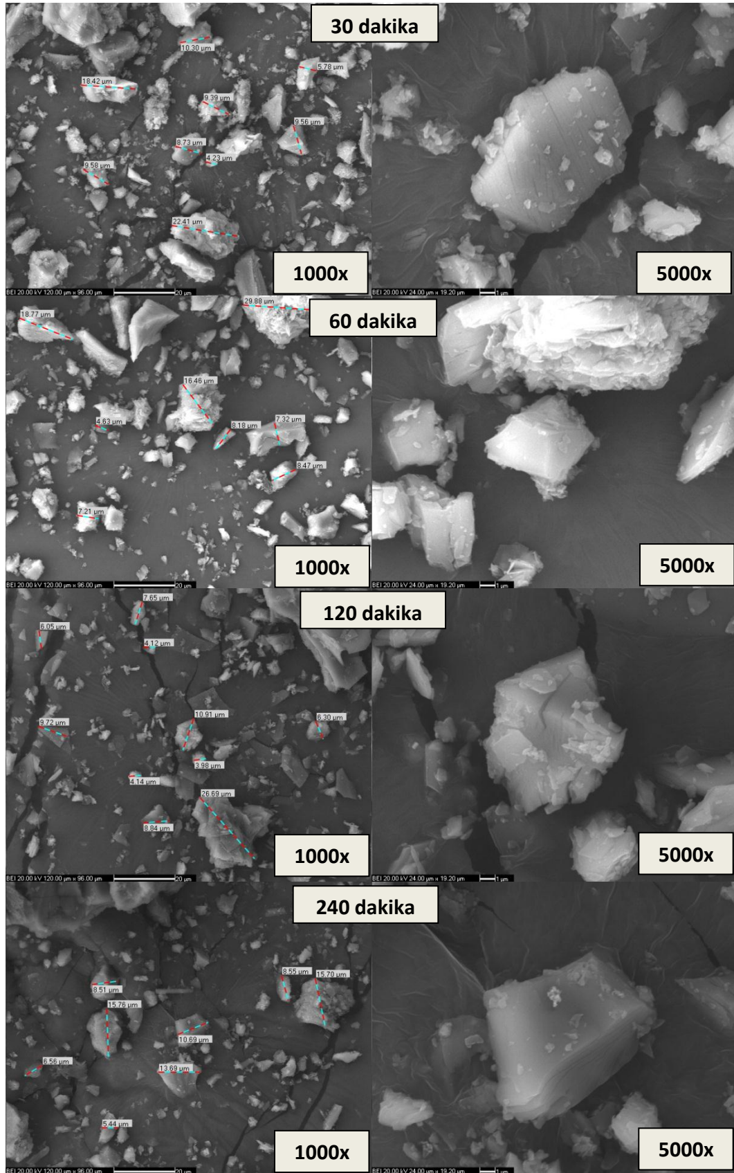
Şekil 6. 14 Hidrotermal metot ile 80°C' de sentezlenen ürünlerin SEM yüzey görüntüleri
