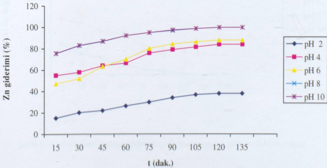
Şekil 8.2 10 g/l pelet kullanıldığında sudaki çinkonun % uzaklaşması
