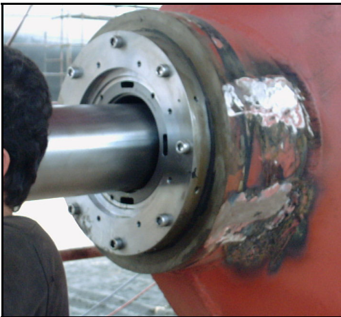
Şekil 4.19 Şaftın sürülmesi.
