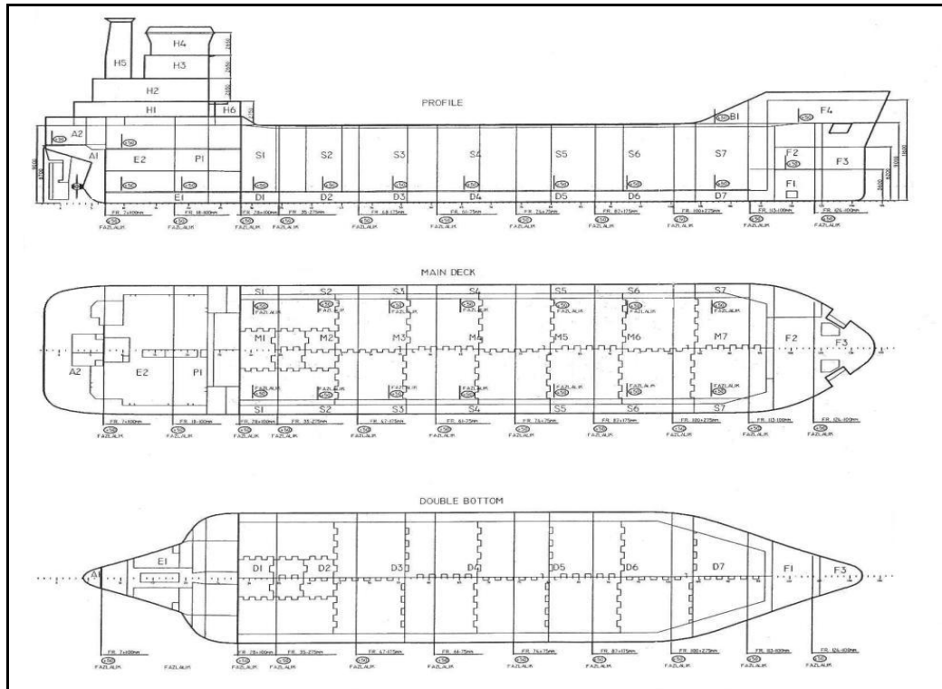
Şekil 6.42 Blokların montaj sırasını ve yapısını gösteren bir strateji planı.
