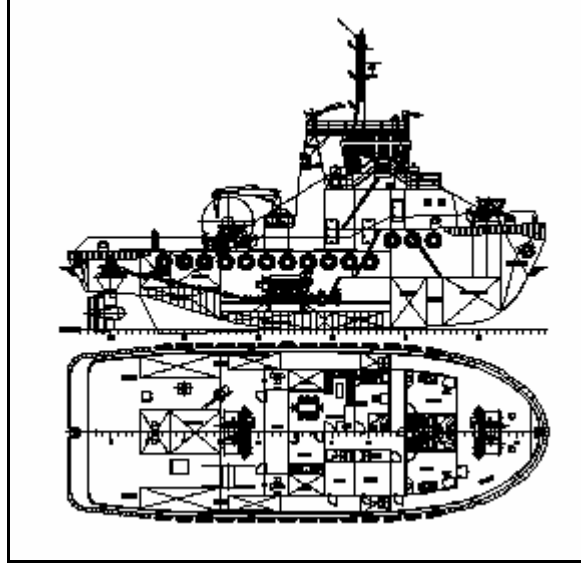
Şekil 3.7 Romorkör formunun profil ve güverte kesit görünümü.
