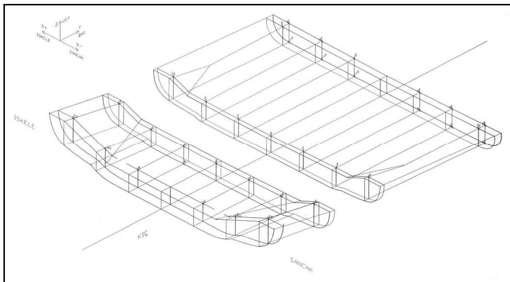
Şekil 6.43 Double bottom blok kızak montaj krokisi.
