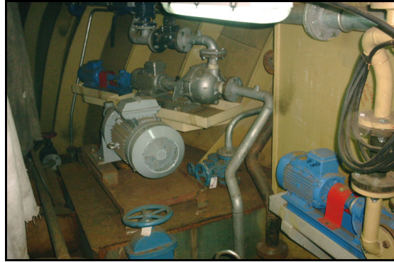
Şekil 4.11 Yakıt transfer pompaları.
