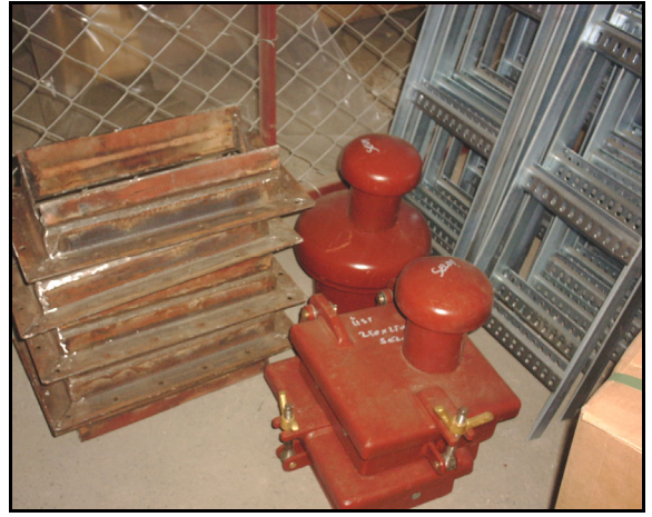
Şekil 6.18 Mantarbaşların muhafaza edilmesi.
