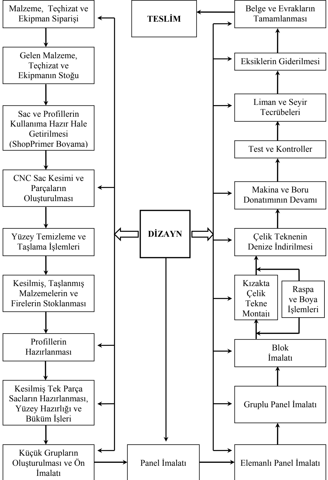
Şekil 6.22 Gemi inşaatında üretim akışı.
