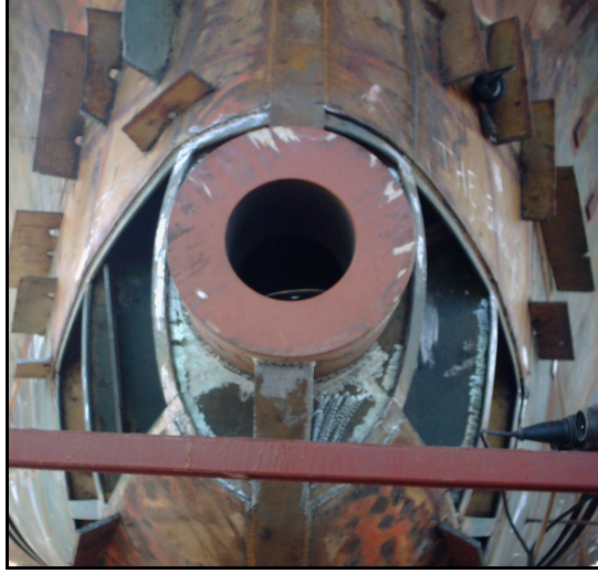
Şekil 4.17 Şaft bosaı montajı.
