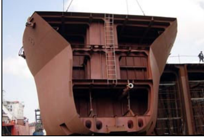
Şekil 6.44 Bloğun kızak eğimine uygun olarak kaldırılması. [15]
