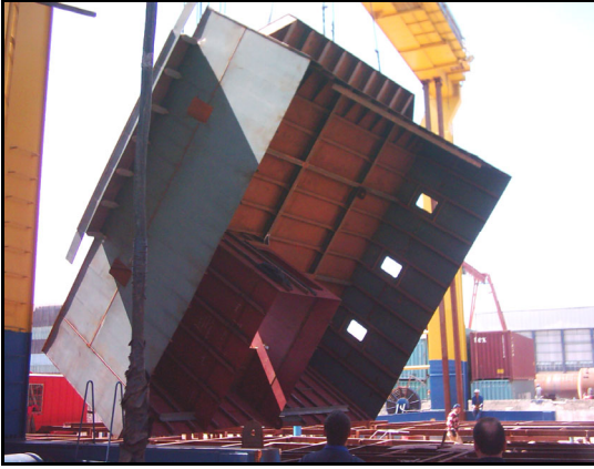
Şekil 4.5 Bloğun montaj için kaldırılması.
