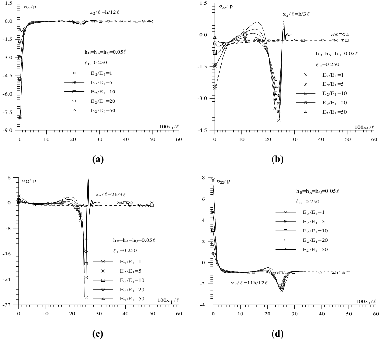
Şekil 2.19 Farklı E_2/E_1 oranları için \sigma_{22}/p gerilmesinin farklı kesitlerde x_1/\ell ye göre grafikleri.
