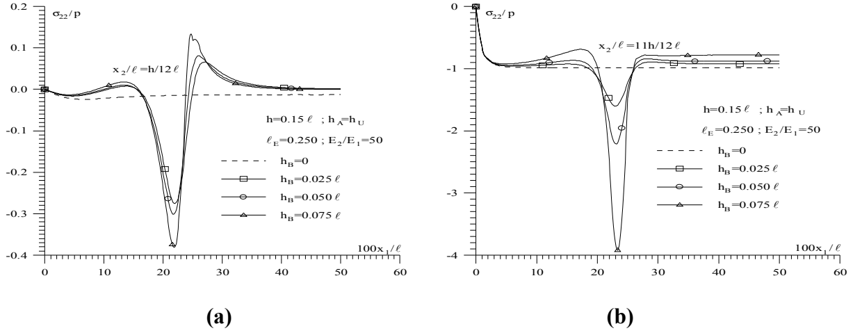
Şekil 2.37 Farklı h_B değeri için \sigma_{22}/p gerilmesinin farklı kesitlerde x_1/\ell ye göre grafikleri.
