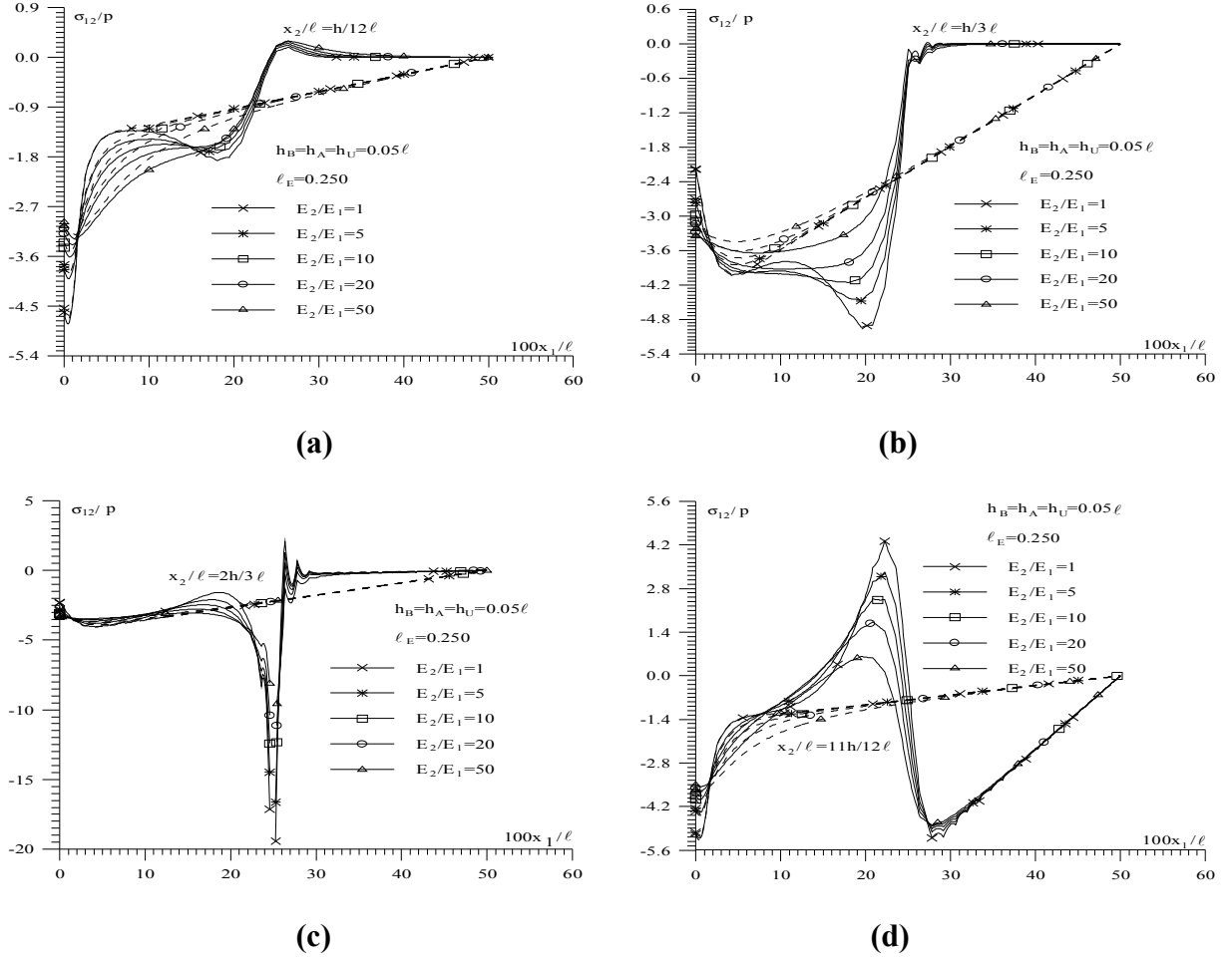
Şekil 2.20 Farklı E_2/E_1 oranları için \sigma_{12}/p gerilmesinin farklı kesitlerde x_1/l ye göre grafikleri.
