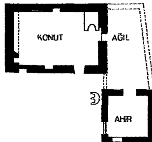
Şekil 3.15 Nohurlu Türkmenlerinde konut ve eklentileri (Eruzun, 1980)
