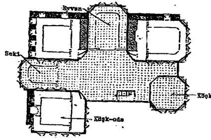
Şekil 4.8 Taselya’da, Ambelakia kasabasında 18. yüzyıldan kalma ev (Eldem, 1973)
