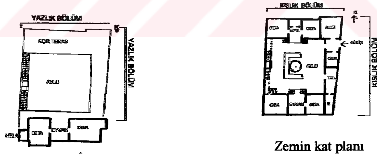
Şekil 6.2 Akyüzler Evinde "yazlık ve kışlık bölüm"
