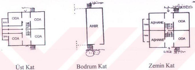
Şekil 6.120 Yusuf Çakır Evinde (konağında) katların kullanımı (Simetri iki ev)
