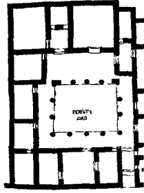
Şekil 3.10 Priene. Peristil ve normal avlulu bir konut (Helenistik devir) (Naumann,1991)
