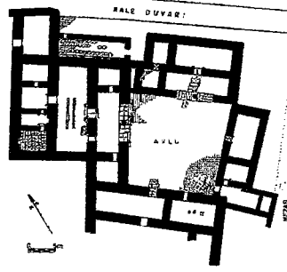
Şekil 3.13 Zincirli. Yukarı Saray (M.Ö. 700) (Naumann, 1991)
