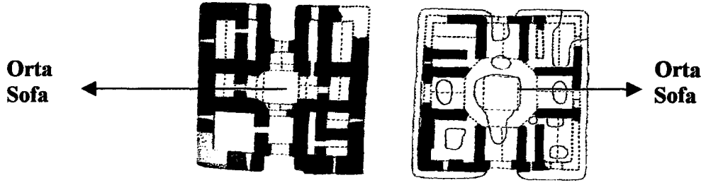
Şekil 3.16 Termez. 12-13 yüzyıllarında bir konutun alt ve üst kat planları (Cezar, 1977)
