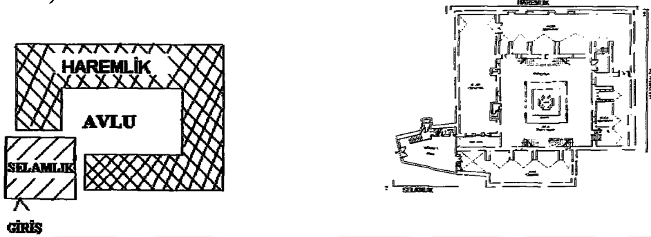
Şekil 6.22 Şahap Bakır Evinde “harem ve selamlık” bölümü
