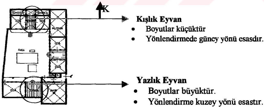
Şekil 6.13 Hacı İmam Demirkol Evinde yazlık ve kışlık eyvanlar (Akkoyunlu ,1989)
