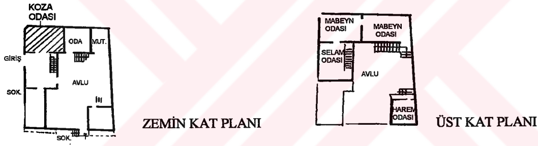
Şekil 6.80 Muradiye mah. no :1'de koza odası
