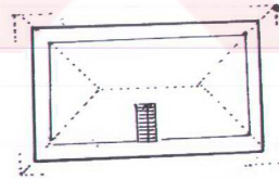
Şekil 6.124 Yukarı Kışla Köyünde evin çatı katı kullanımı
