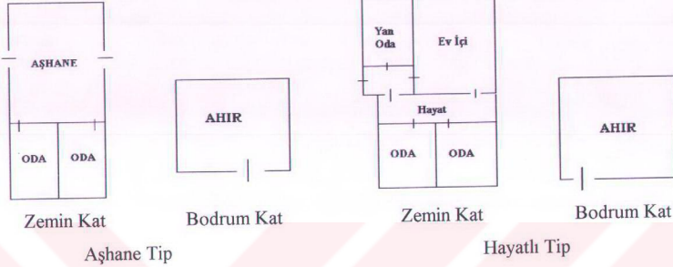
Şekil 6.118 Doğu Karadeniz Evinde plan tipleri
