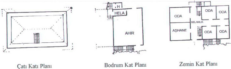
Şekil 6.121 Yukarı Kışla köyü no:171'de evin bölümleri
