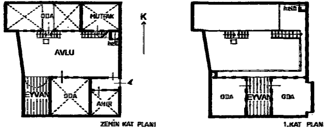
Şekil 6.1 Ömer Göncü Evinde "avlu" ve "eyvan"
