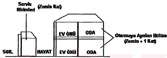
Şekil 6.74 Muğla Evinde katların kullanım durumu
