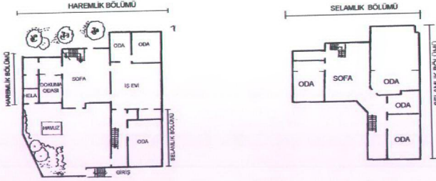
Şekil 6.112 Latifoğlu Konağında harem ve selamlık bölümü
