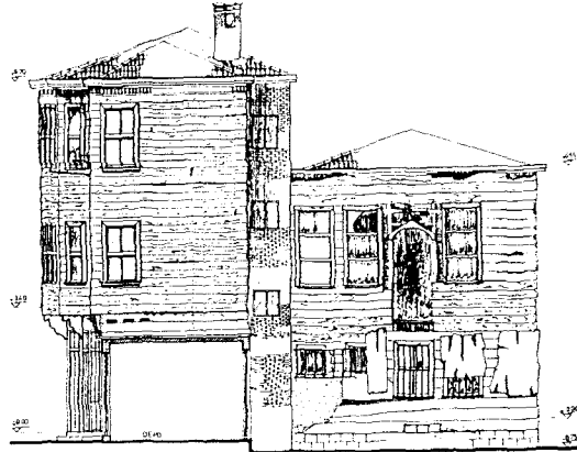
Ç.82-Sağ görünüş
