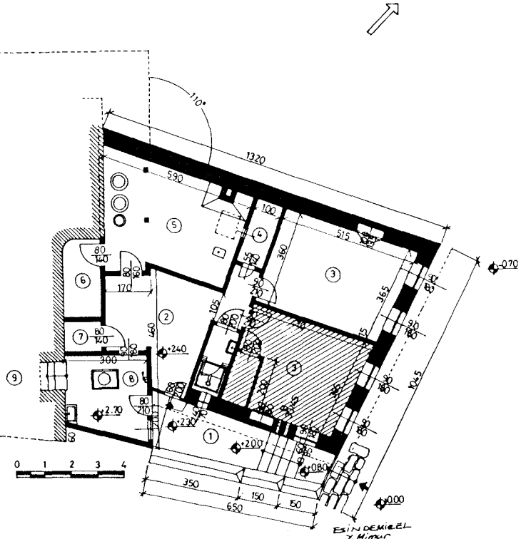
Ç.70-Alt kat planı
