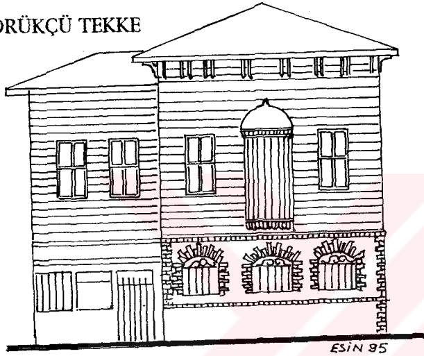
Ç.79-Ön görünüş (E. Demirel)
