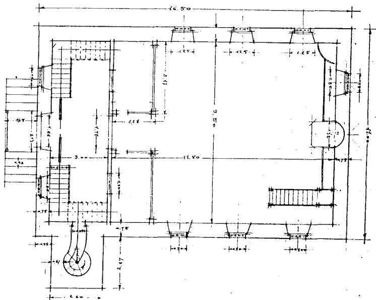
Ç.142-Yuşa Tekkesi plan (İst. Vak. Böl. Md. Ar.)
