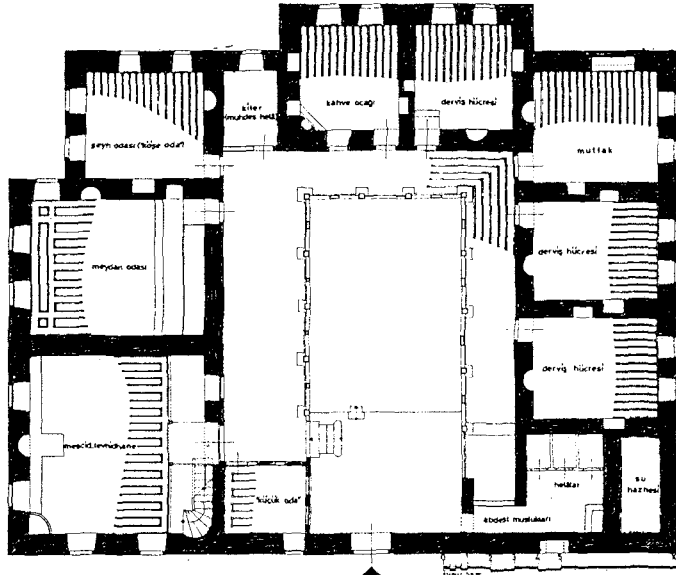
Ç.120-Tahir Ağa Tekkesi plan (DB.İst. Ans.)
