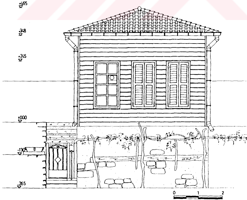
Ç.55-Efganiler Tekkesi köşk sohbethaneninin görünüşü (Y.T.Ü'den)
