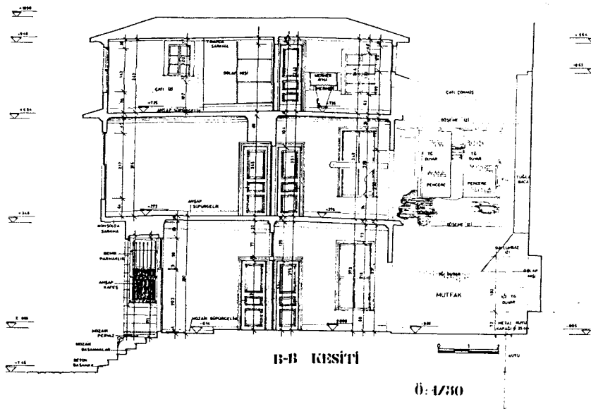
Ç.132-Hacı Beşir Ağa Tekkesi Meşrutası kesit (C. Ertem'den)
