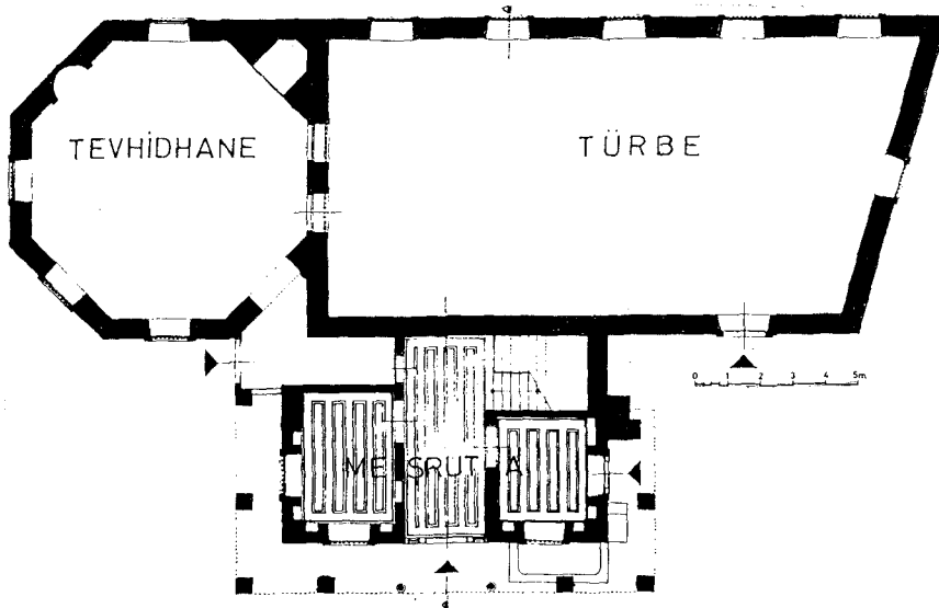
Ç.112-Ataullah Ef. Tekkesi plan
