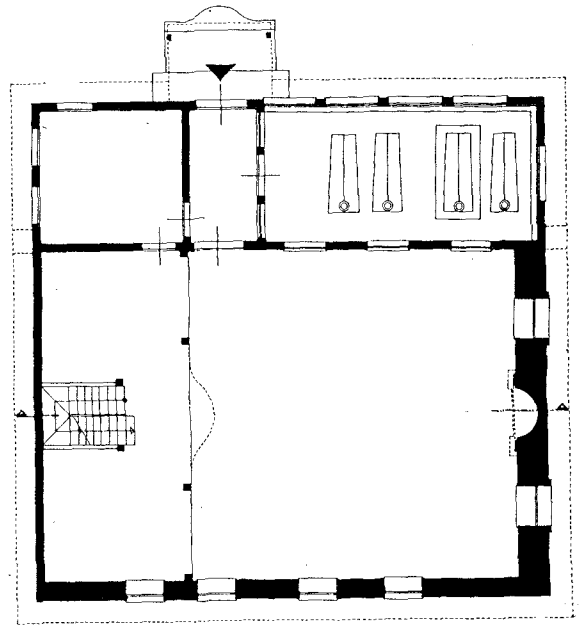
Ç.109-Ekmel Tekkesi plan (İst. Vak. Böl. Md. Ar.)
