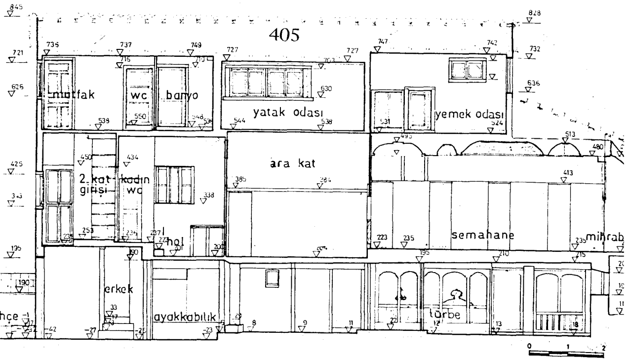
Çürüklük Tekkesi Rölövesi
