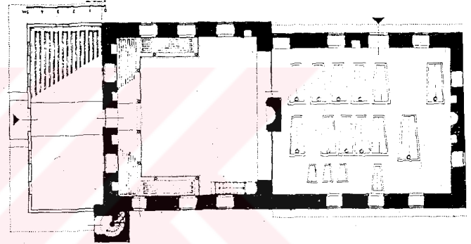
Ç.111-Saçlı Emir Osman Tekkesi plan (B. Tanman'dan)
