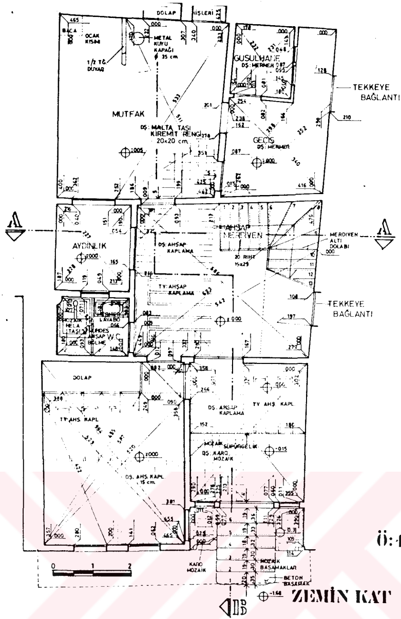
Ç.131-Hacı Beşir Ağa Tekkesi Meşrutası plan (C. Ertem'den)
