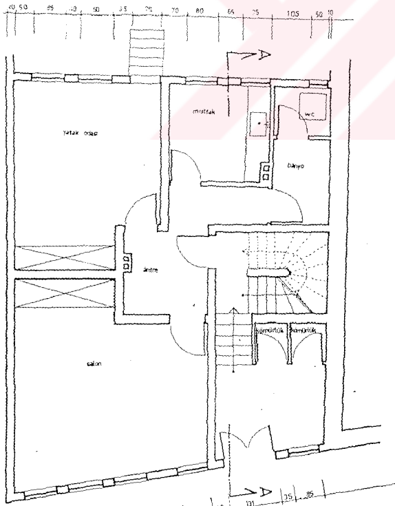
GİRİŞ PLANI Ö.1/50
