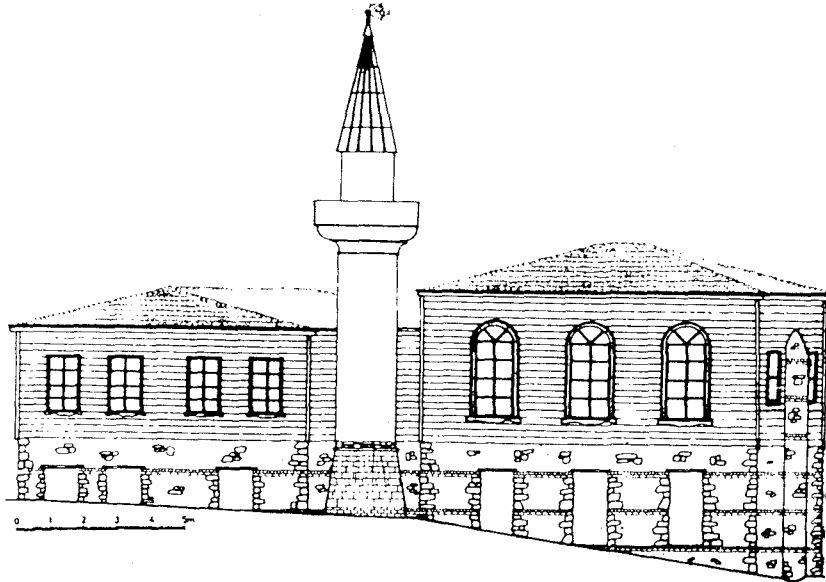
Ç.147-Restitüsyon görünüşü (M.S.Ü'den)
