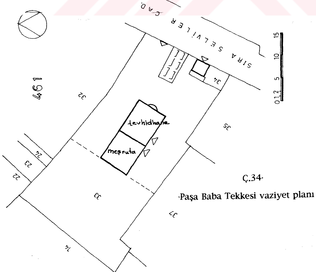
Ç.33-Yavaşca Mehmet Ef. Tekkesi vaziyet planı
