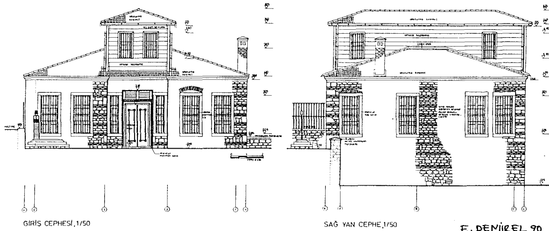
Ç.124-Ön görünüş
