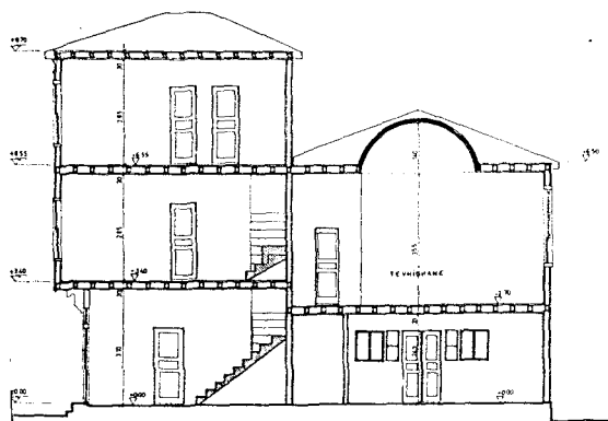
A.A KESİTİ 1/50
