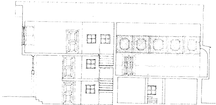
Tevhidhaneden Geçen Kesit
