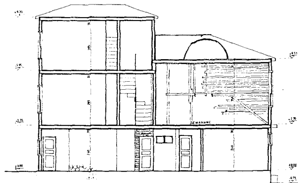
B-B KESTİTİ 1/50
