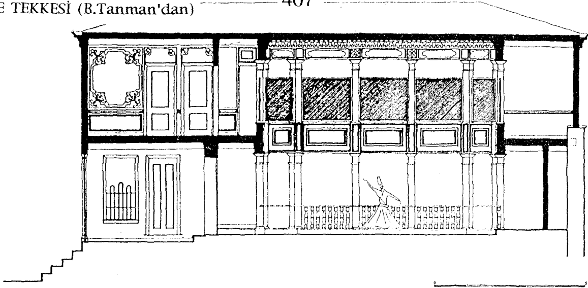
Ç.89-Tevhidhane Kesiti
