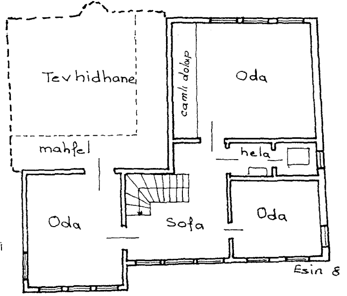
Ç.102-Kılıçcı Tekkesi 1. kat krokisi
