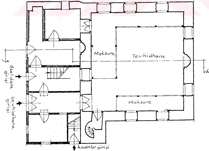
Ç.144-Zemin kat planı
