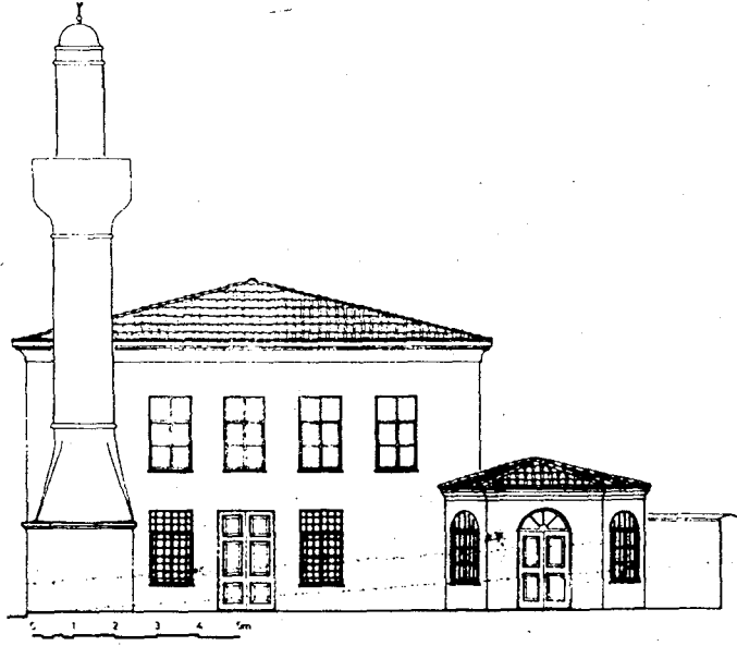
Ç.145-Görünüş
