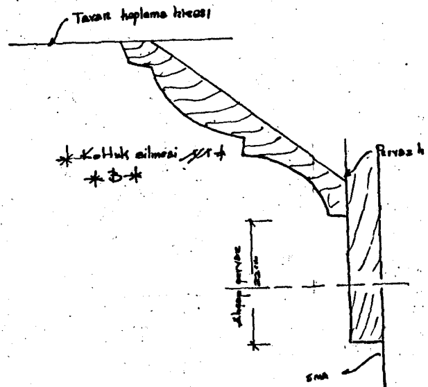
154- Koltuk altı silmesi ve pasa detayı,
