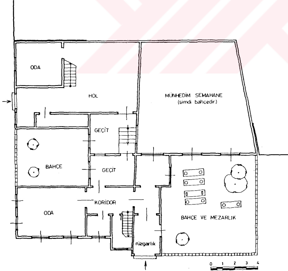
Ç.103-Zıbnı Şerif Tekkesi zemin kat planı yıkılmadan önce (M. Rona'dan)
