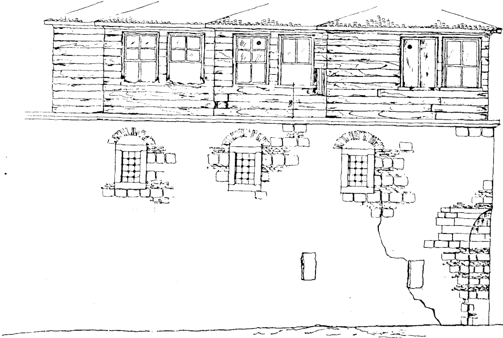
Ç.149-Ahşap meşruta görünüş (rölöve)
