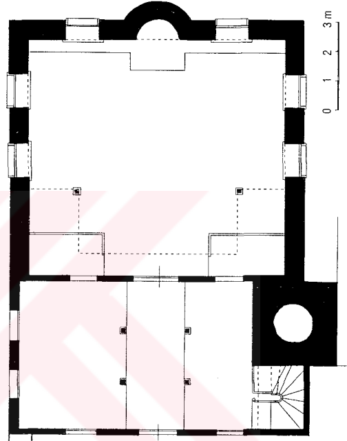
Ç.141-Akarca Tekkesi plan
