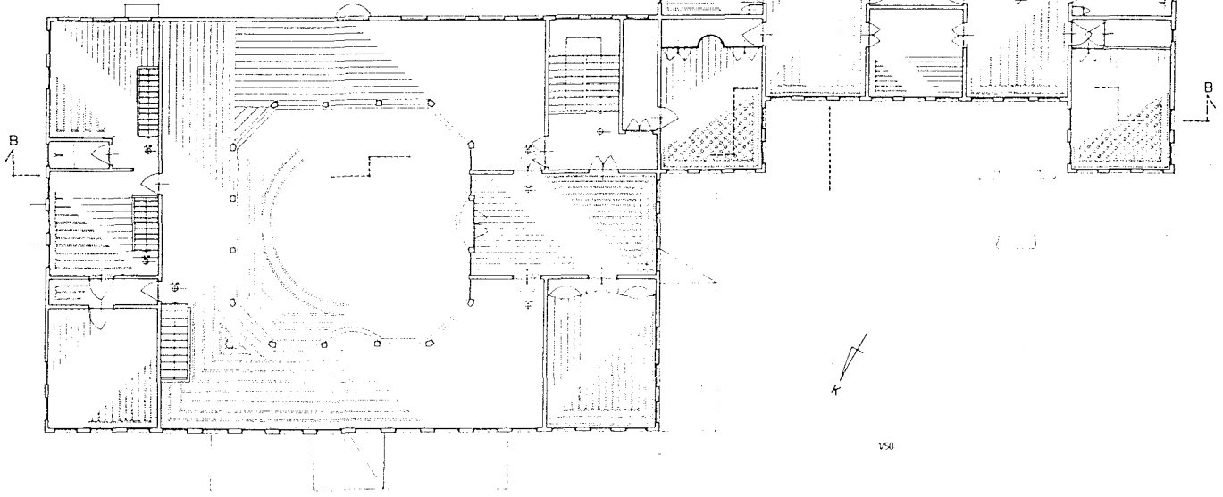
Ç.57-Kasımpaşa Mevlevihanesi birinci kat planı
