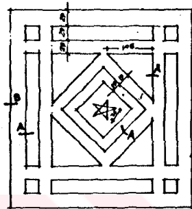
Ç.152-Ahşap oda plan-kesit-görünüş (restorasyon)
