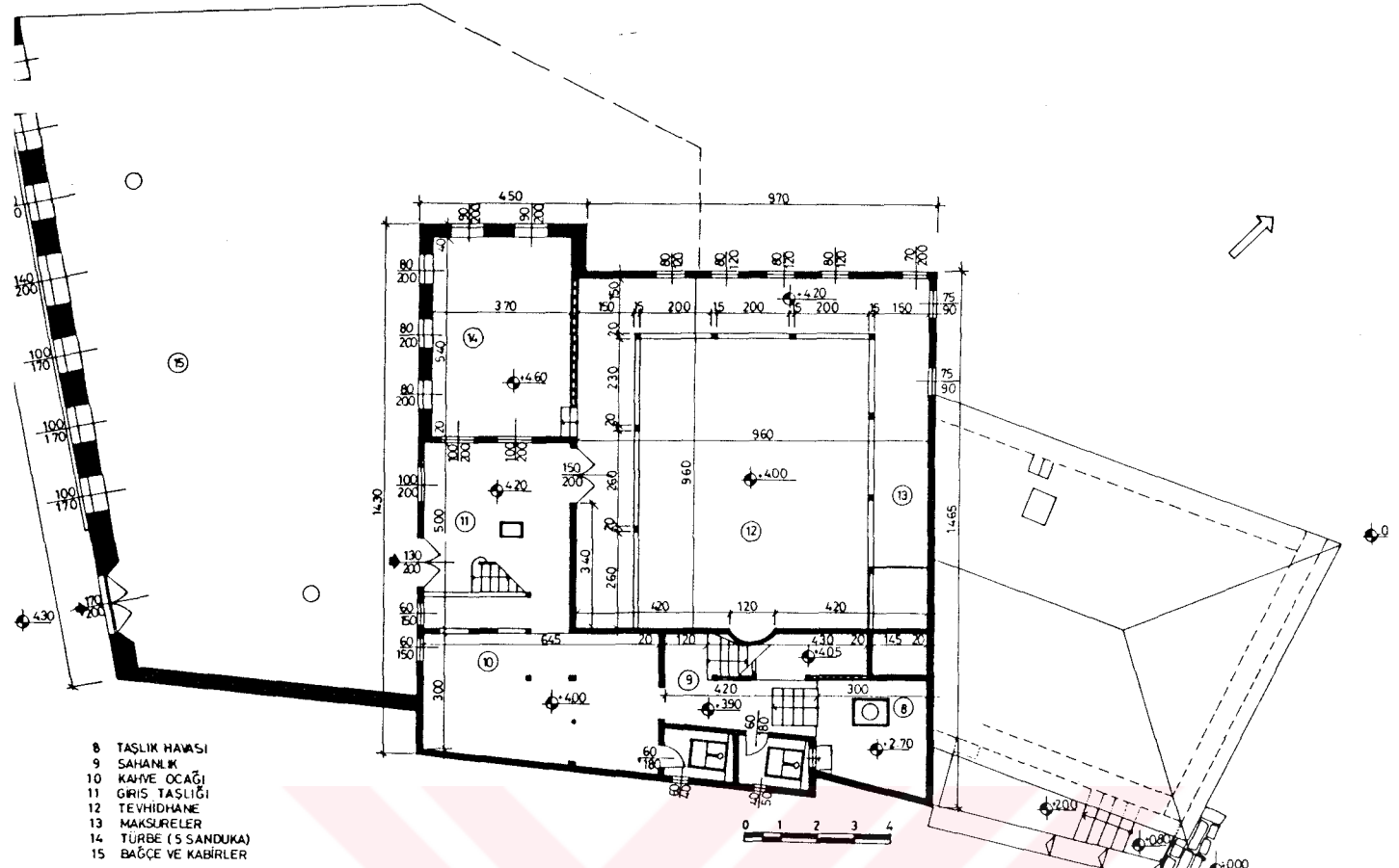
Ç.69-Zemin kat planı
