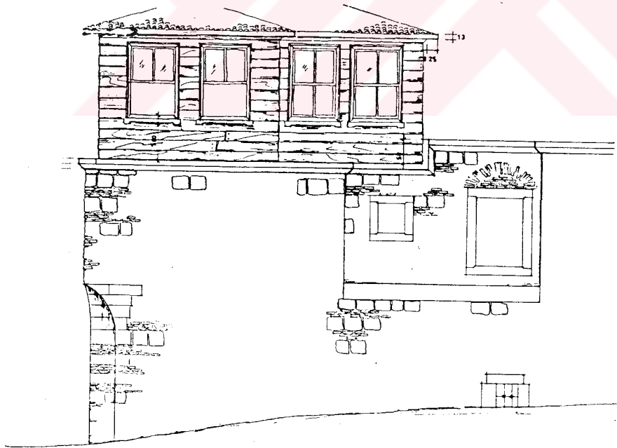
Ç.151-Görünüş (rölöve)
