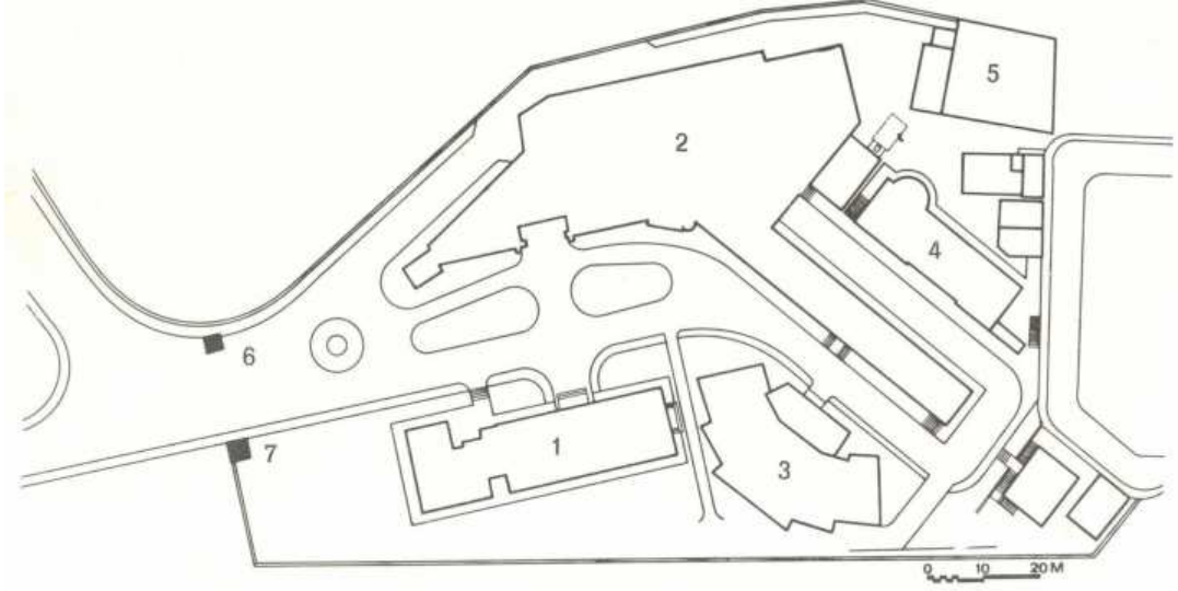
Şekil 3.109 Yıldız Çini Fabrika-i Hümayunu'nun mevcut yerleşim planı (Küçükerman, 1987b)
