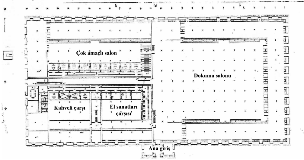
Şekil 3.55 Feshane-i Âmire'nin mevcut durum planı (Tomur Atagök Arşivi, 2000)
