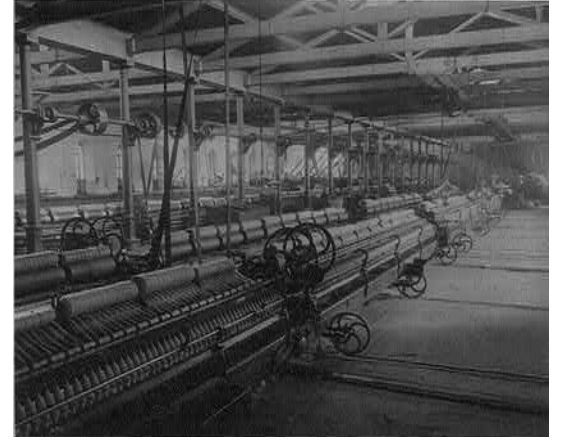
Şekil 3.39 ve Şekil 3.40 Feshane-i Âmire'deki iplik eğirme makineleri (II. Abdülhamit Albümü, 1880-1893, 11911/47-48) [2]
