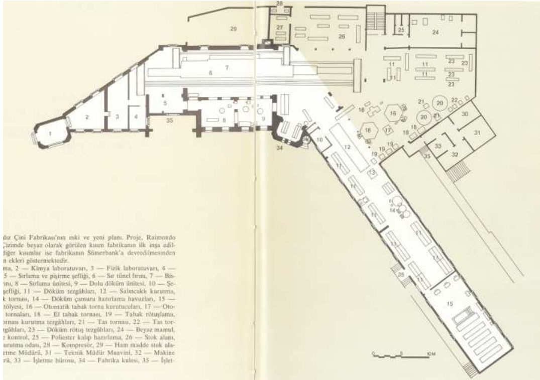
Şekil 3.112 Yıldız Çini Fabrika-i Hümayunu’nun işletme binasının planı (Küçükerman, 1987b)
