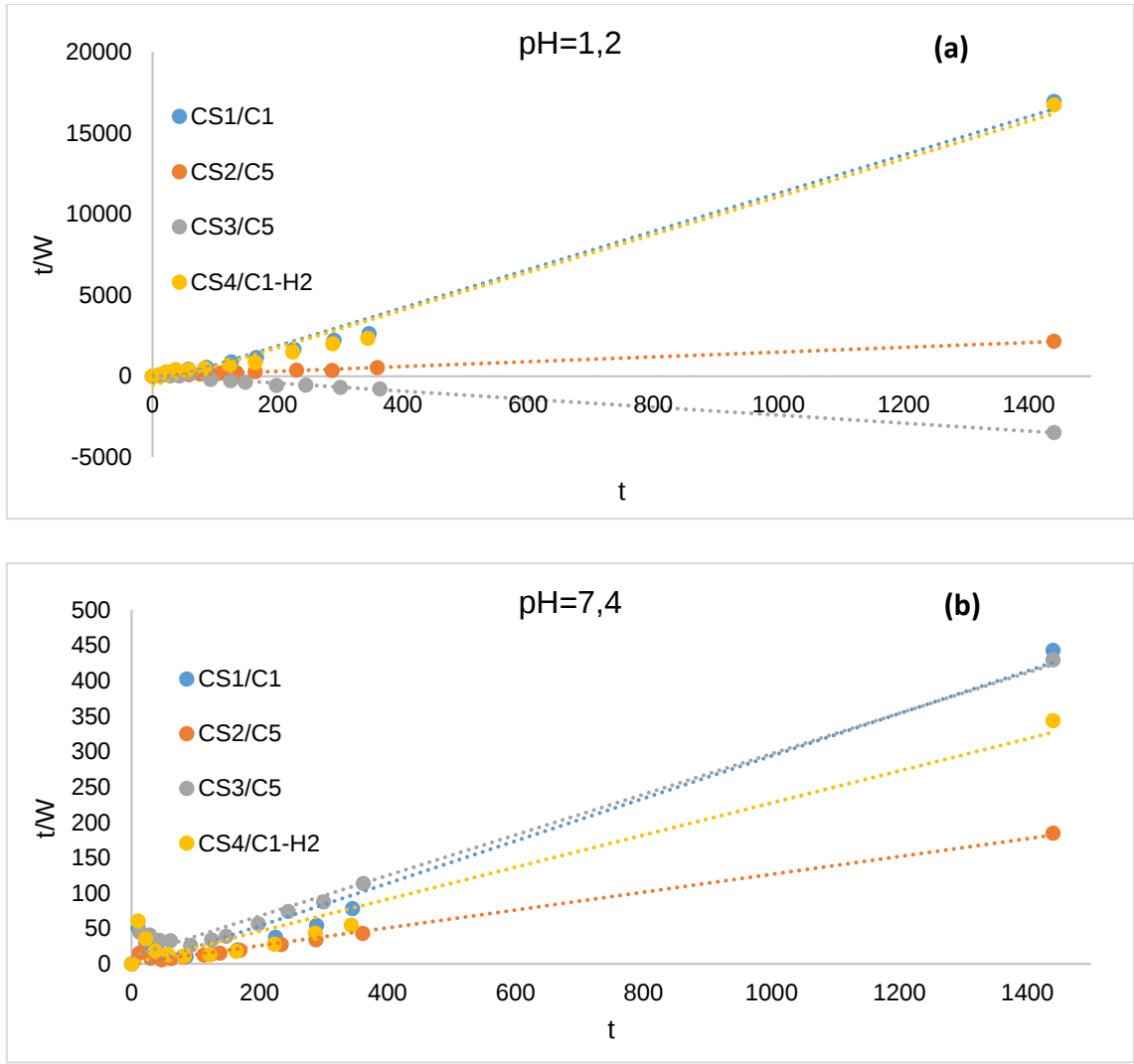
Şeki 7.20 Çekirdek-kabuk hidrojel kürelerin ikinci-derece kinetik verilerinden çizilen grafikler ( t/W 'ye karşı t ) (a) pH=1,2, (b) pH=7,4
