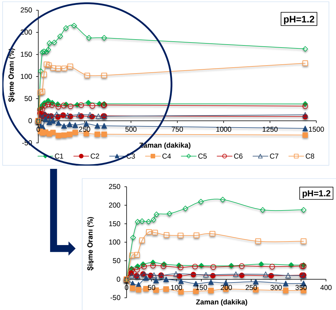
Şekil 7.9 Hidrojel kürelerin sentetik mide sıvısı ortamındaki dinamik şişme sonuçları
