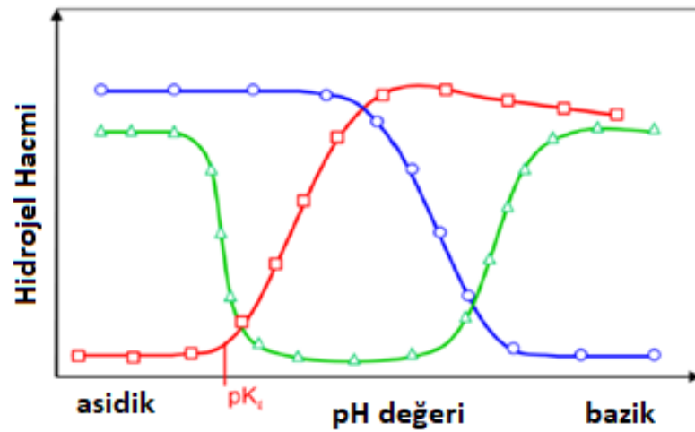
Şekil 2.7 pH duyarlı hidrojellerin hacim-faz geçişleri; kırmızı: anyonik/asidik hidrojel, mavi: katyonik/bazık hidrojel, yeşil: amfifilik hidrojel göstermektedir [119]
