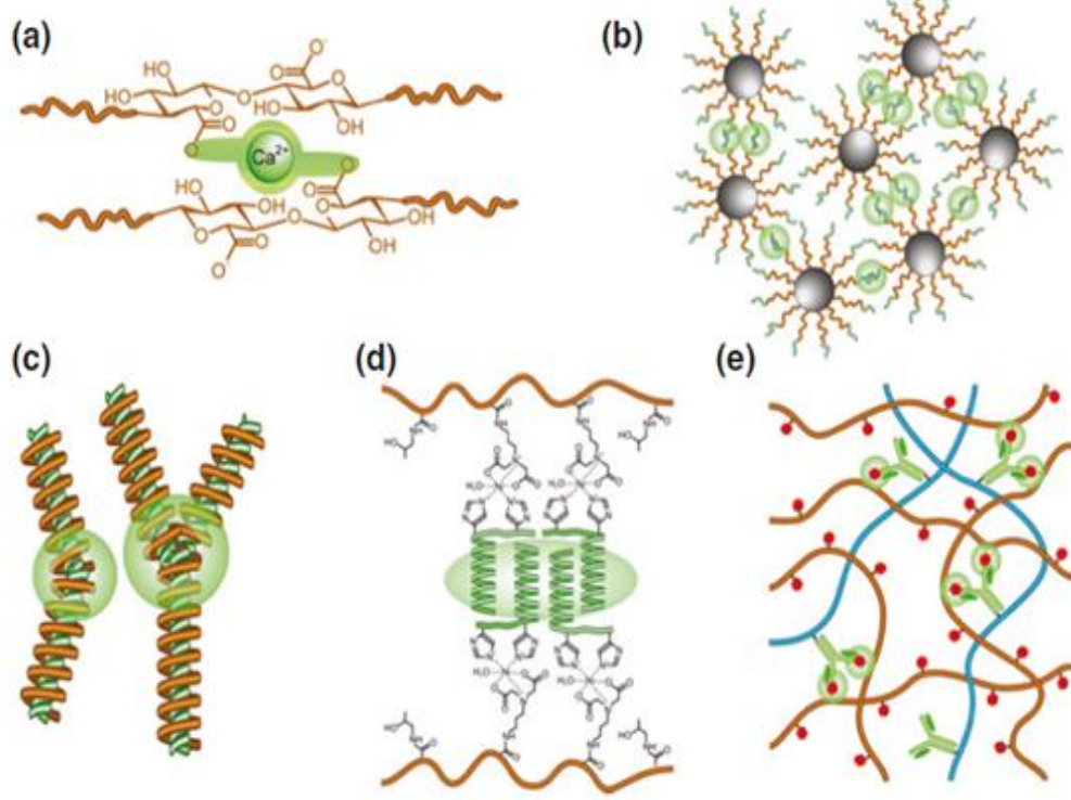
Şekil 2.2 Fiziksel çapraz bağlı hidrojellerin oluşumu için uygulanan yöntemlerin şematik gösterimi. a) iyonik etkileşimler, b) hidrofobik etkileşimler, c) stereokompleks oluşumu, d) sarmal sarmal etkileşimleri, e) özel moleküler tanıma (specific molecular recognition) [47]
