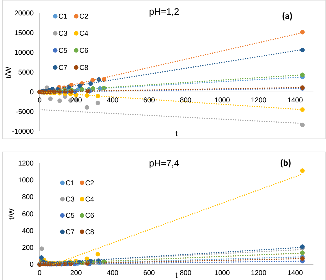
Şeki 7.18 Hidrojel kürlerin ikinci-derece kinetik verilerinden çizilen grafikler ( t/W 'ye karşı t ) (a) pH=1,2, (b) pH=7,4
