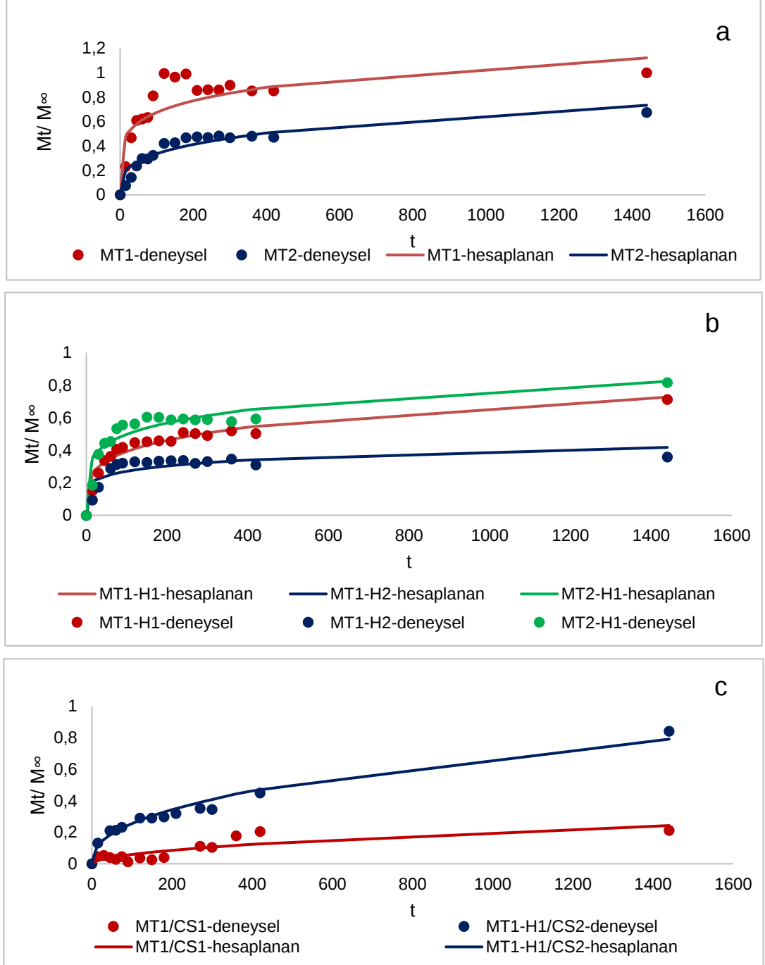
Şekil 7.27 Hidrojel kürelerin deneysel ve KormeyerPeppas modeli ile hesaplanan M_t / M_{\infty} değerlerinin zamana karşı karşılaştırmalı grafikleri (pH=7,4) a) Tuz etkisi, b) HAP etkisi, c)Çekirdek-kabuk etkisi
