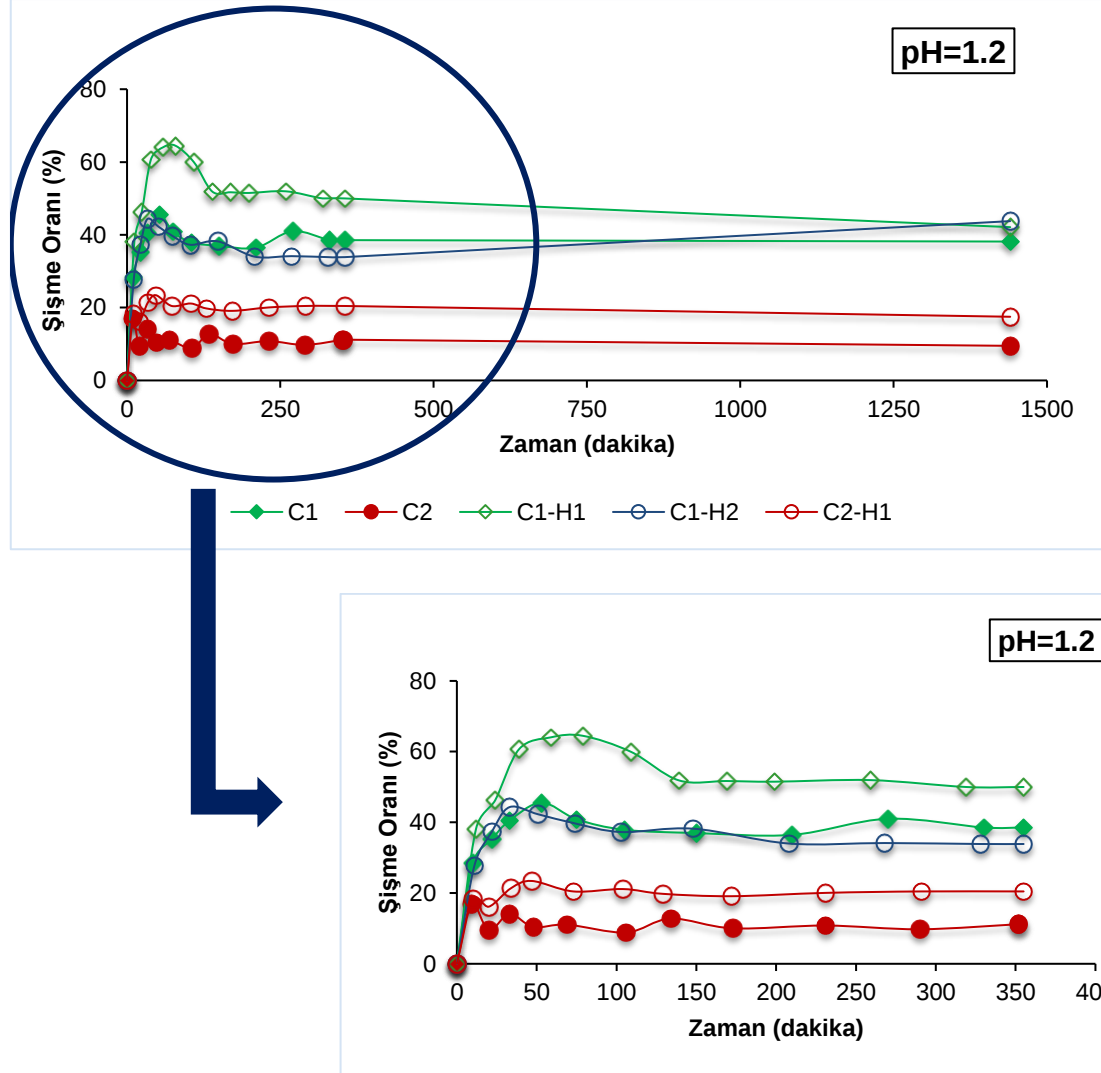
Şekil 7.11 HAP katkılı hidrojel kürelerin sentetik mide sıvısı ortamındaki dinamik şişme sonuçları
