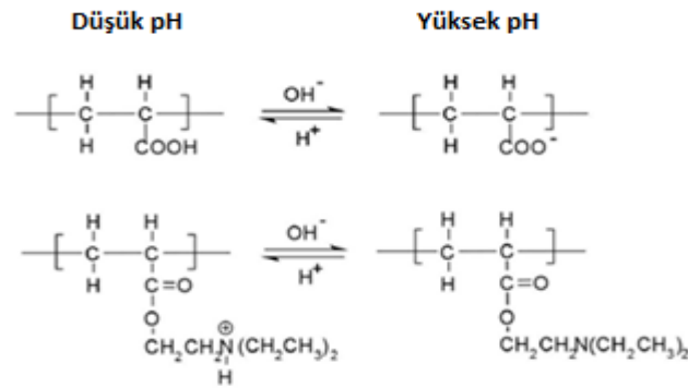
Şekil 2.6 Anyonik ve katyonik polielektrolitlerin ve pH'a bağlı iyonlaşma süreci [109]
