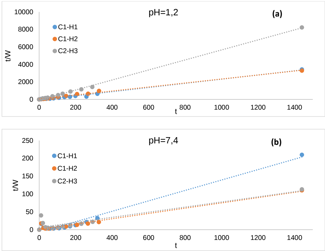
Şeki 7.19 Hidroksiapatit katkılı hidrojel kürlerin ikinci-derece kinetik verilerinden çizilen grafikler ( t/W 'ye karşı t ) (a) pH=1,2 , (b) pH=7,4
