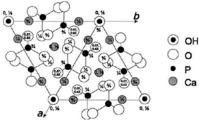
Şekil 6.3 Hidroksiapatitin c ekseninde doğrultusunda ideal kristalize yapısı [226]
