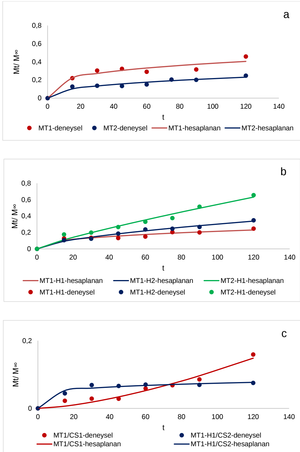
Şekil 7.26 Hidrojel kürelerin deneysel ve KormeyerPeppas modeli ile hesaplanan M_t / M_\infty değerlerinin zamana karşı karşılaştırmalı grafikleri (pH=1,2) a) Tuz etkisi, b) HAP etkisi, c)Çekirdek-kabuk etkisi
