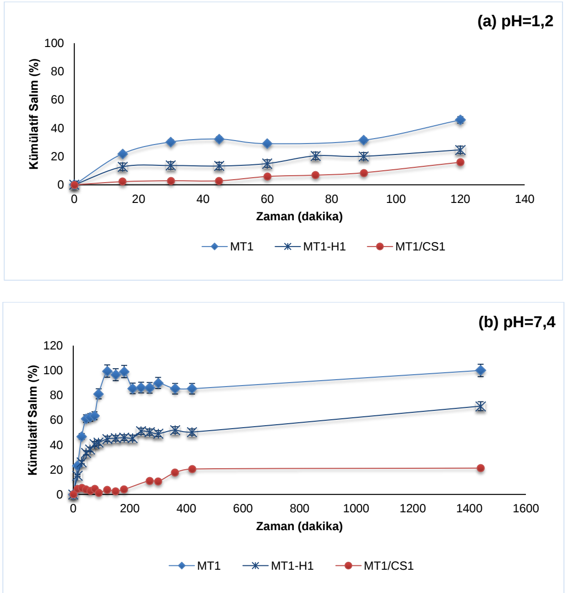
Şekil 7.23 Çekirdek-kabuk ve HAP katkılı hidrojel kürelerin salım eğrileri a) pH=1,2, b) pH=7,4
