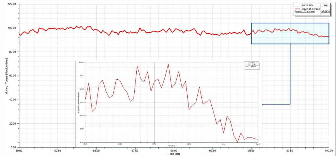
Şekil B. 33 40 oluklu rotoruna 18° kaykısı açısı uygulanmış modele ait moment değişimi
