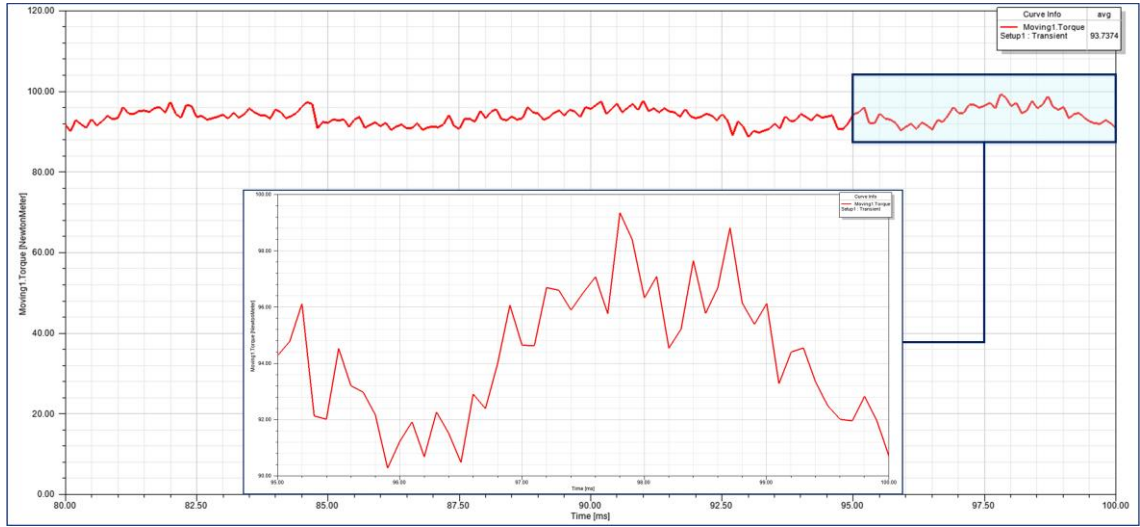
Şekil B. 28 38 oluklu rotoruna 20° kaykısı açısı uygulanmış modele ait moment değişimi
