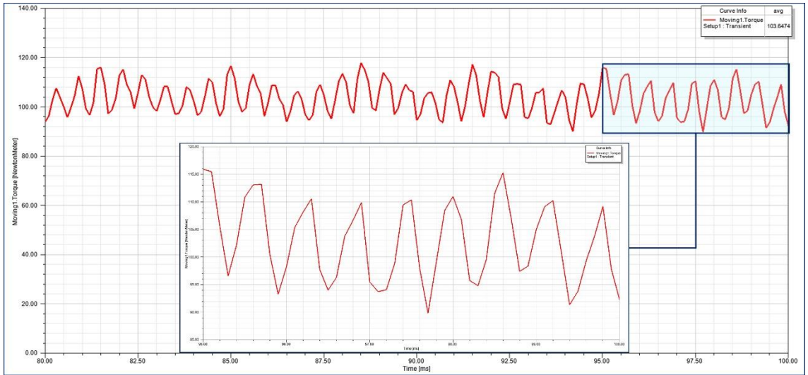
Şekil B. 37 42 oluklu rotoruna 10° kaykı açısı uygulanmış modele ait moment değişimi
