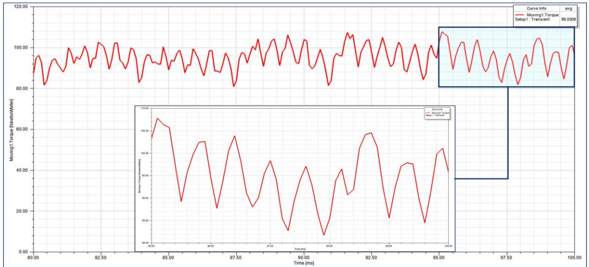
Şekil B. 9 30 oluklu rotoruna 15° kaykısı açısı uygulanmış modele ait moment değişimi
