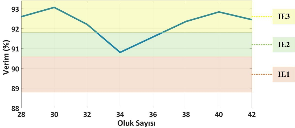
Şekil 4. 1 Farklı oluk sayılarına göre tasarlanan EAAM’lerden elde edilen verimler
