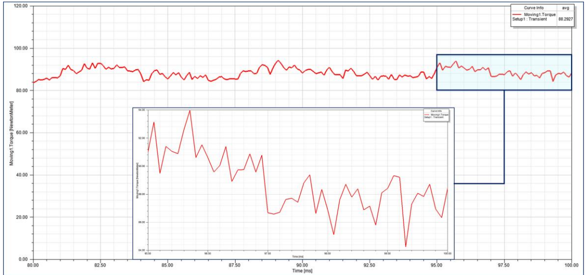
Şekil B. 15 32 oluklu rotoruna 20° kaykısı açısı uygulanmış modele ait moment değişimi
