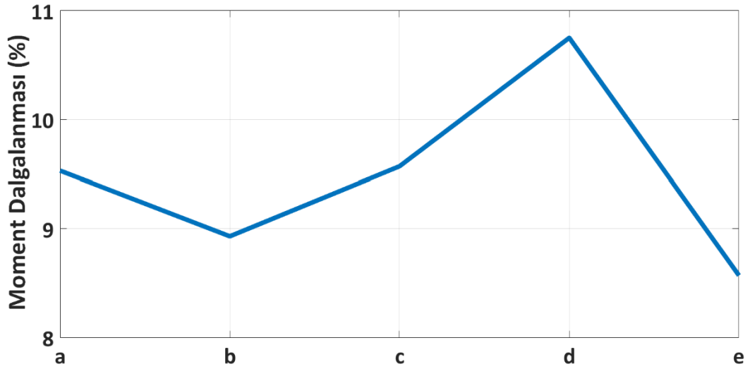
Şekil 4. 28 YMK malzeme uygulanan EAAM'nin moment dalgalanması grafiği
