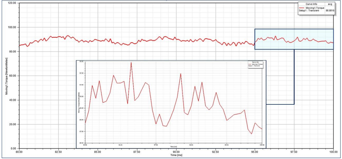
Şekil B. 22 34 oluklu rotoruna 21,17^\circ kaykısı açısı uygulanmış modele ait moment değişimi
