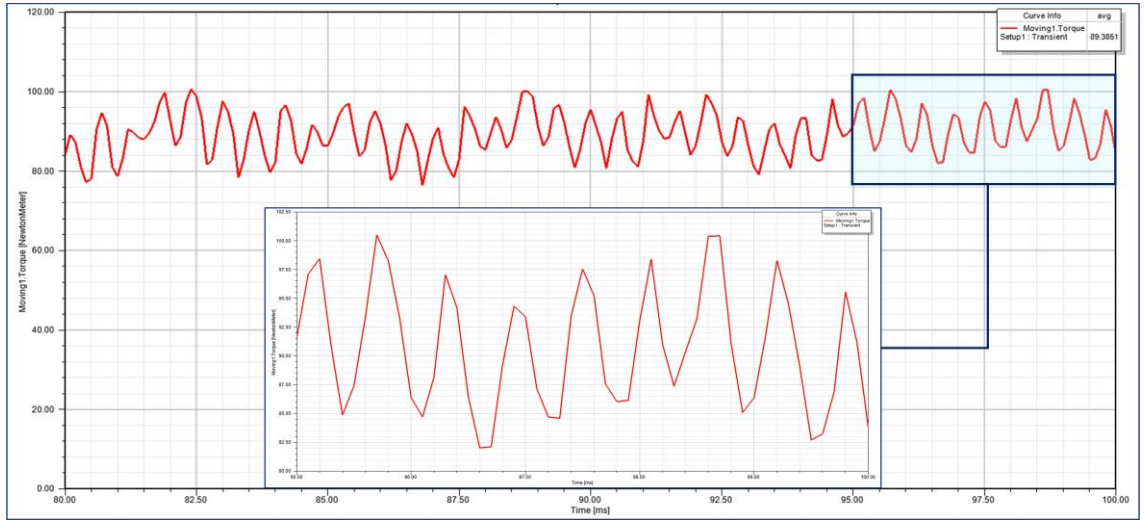
Şekil B. 8 30 oluklu rotoruna 12° kaykısı açısı uygulanmış modele ait moment değişimi
