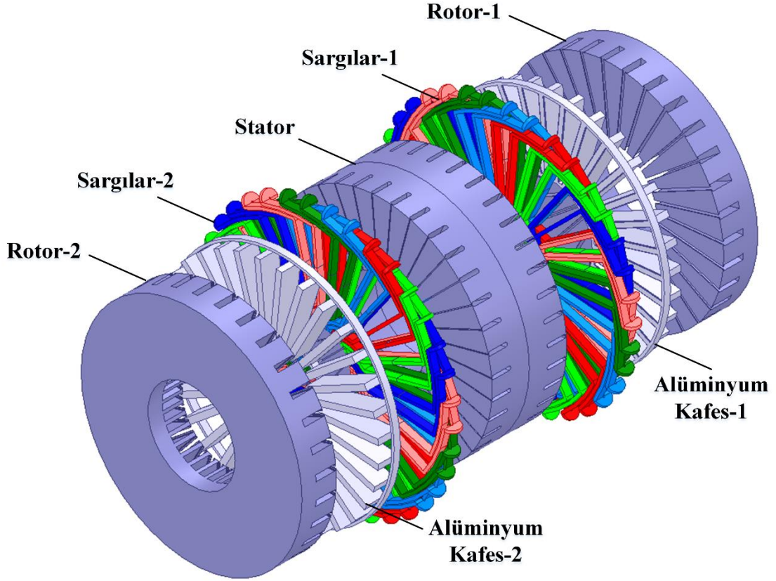
Şekil 2. 3 TSÇR Yapısı
