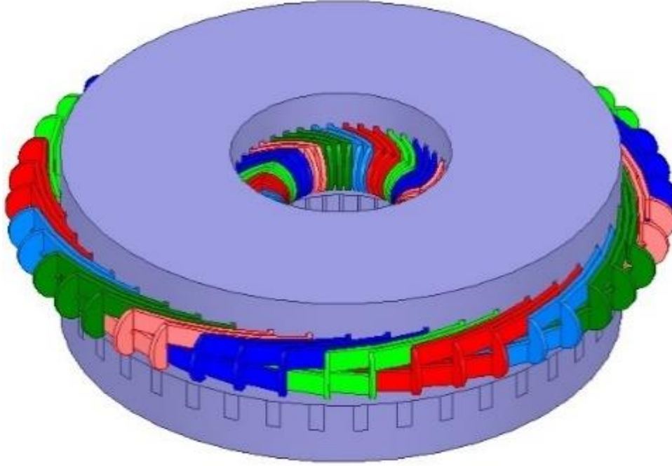
Şekil 3. 2 EAAM model geometrisi
