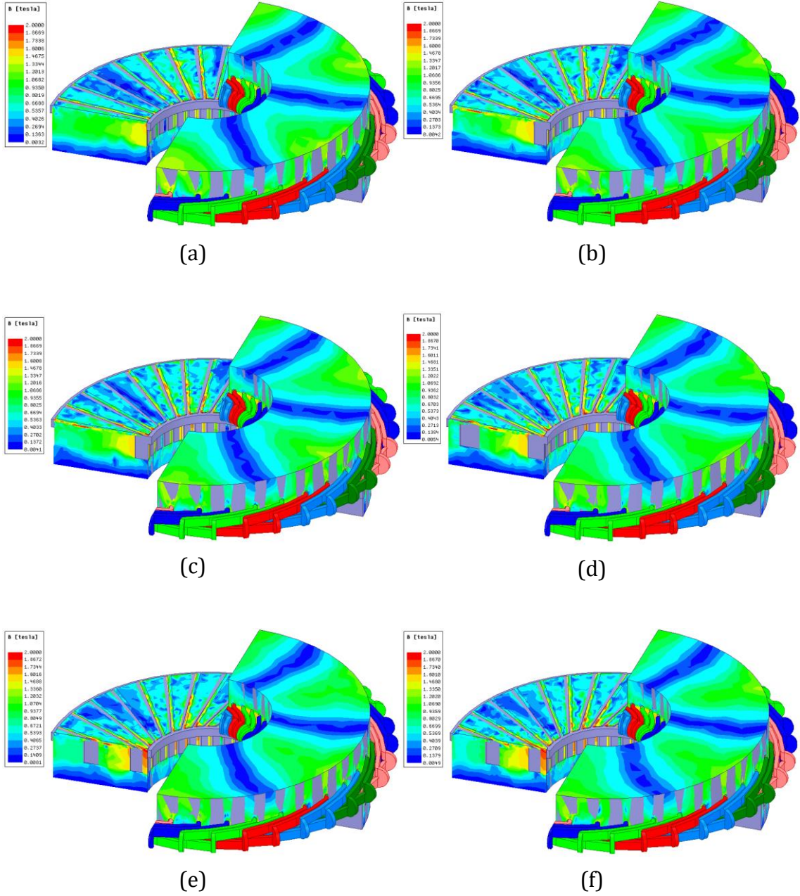
Şekil 4. 14 34 oluklu EAAM analizlerinden elde edilen manyetik akı yoğunluğu dağılımları (a) Kaykı açısı uygulanmamış model, (b) 10° kaykı açısı uygulanmış model, (c) 10,58° kaykı açısı uygulanmış model, (d) 15° kaykı açısı uygulanmış model, (e) 20° kaykı açısı uygulanmış model, (f) 21,17° kaykı açısı uygulanmış model
