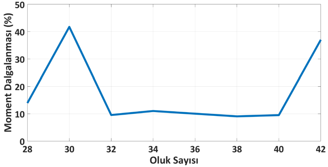
Şekil 4. 2 Farklı oluk sayılarına göre tasarlanan EAAM'lerin moment dalgalanması grafiği
