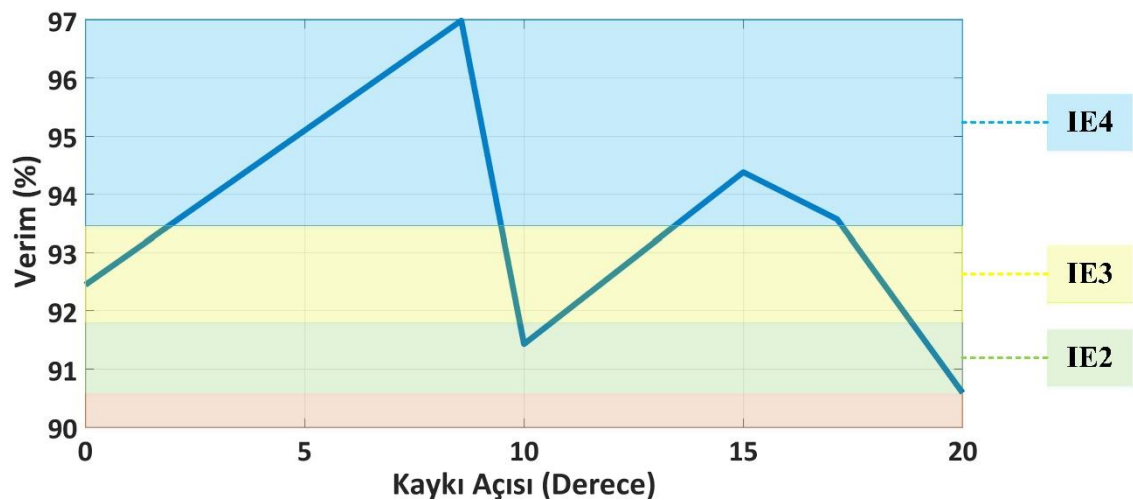
Şekil 4. 21 42 oluklu EAAM'nin kaykırı açısı analizlerinden elde edilen verim değerleri
