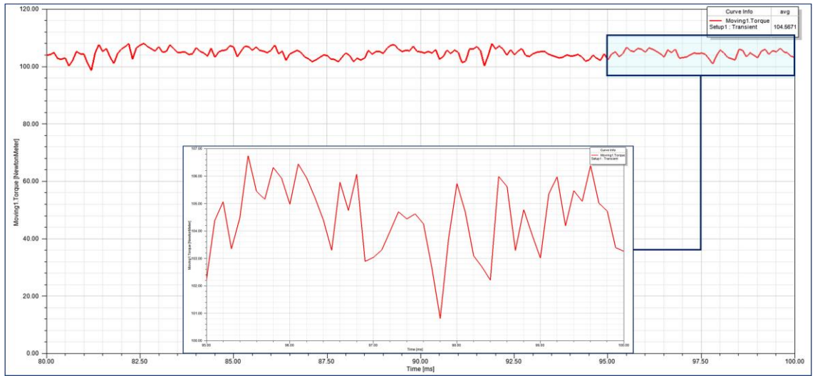
Şekil B. 23 38 oluklu rotoruna kaykısı açısı uygulanmamış modele ait moment değişimi
