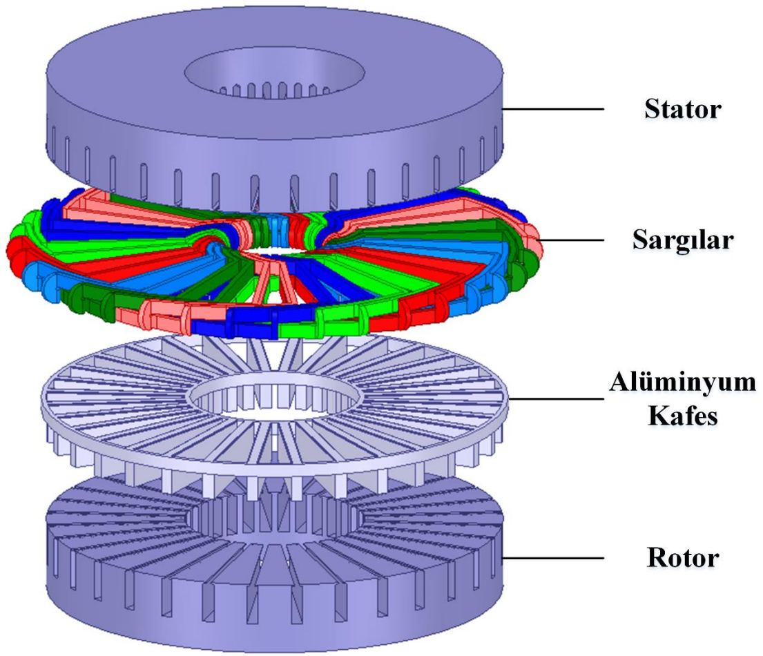
Şekil 2. 1 TSTR Yapısı
