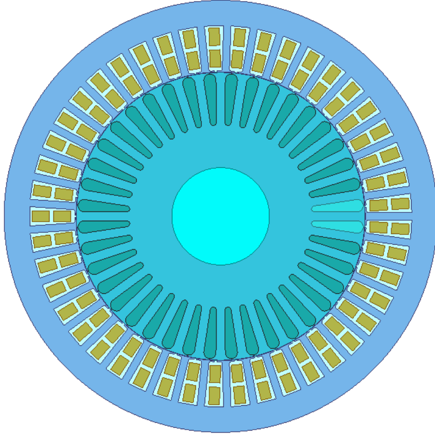
Şekil 3. 1 RAAM model geometrisi
