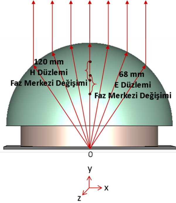
Şekil 5.7 Lens antenin faz merkezi değişimi
