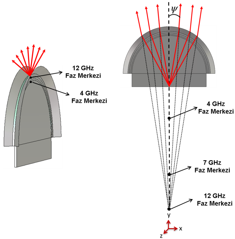
Şekil 6.9 Düzlemsel lens antenin frekansa bağlı faz merkezi aralığı (a) E Düzlem (b) H Düzlem
