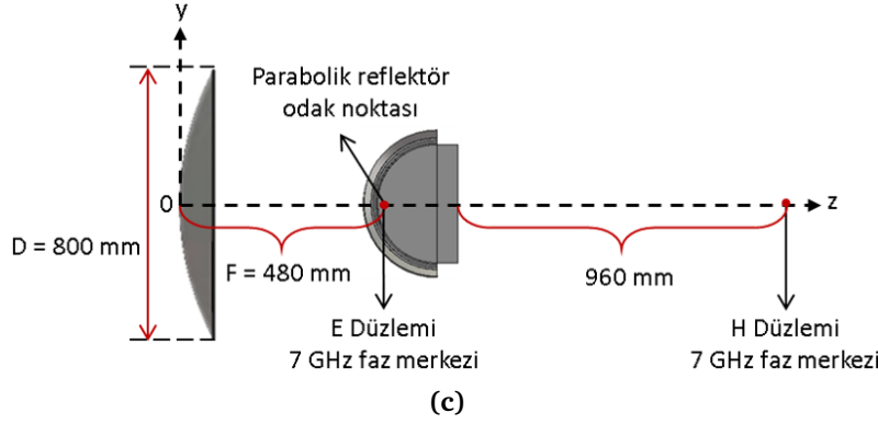
Şekil 6.10 Düzlemsel lens antenin reflektör beslemesi olarak kullanıldığı dört senaryo (a) 7 GHz'deki E düzlemi faz merkezi, F/D=2.5 ile reflektör odağına, (b) 7 GHz'deki H düzlemi faz merkezi, F/D=2.5 ile reflektör odağına, (c) 7 GHz'deki E düzlem faz merkezi, F/D=0.6 ile parabolik reflektörün odağına yerleştirilir.
