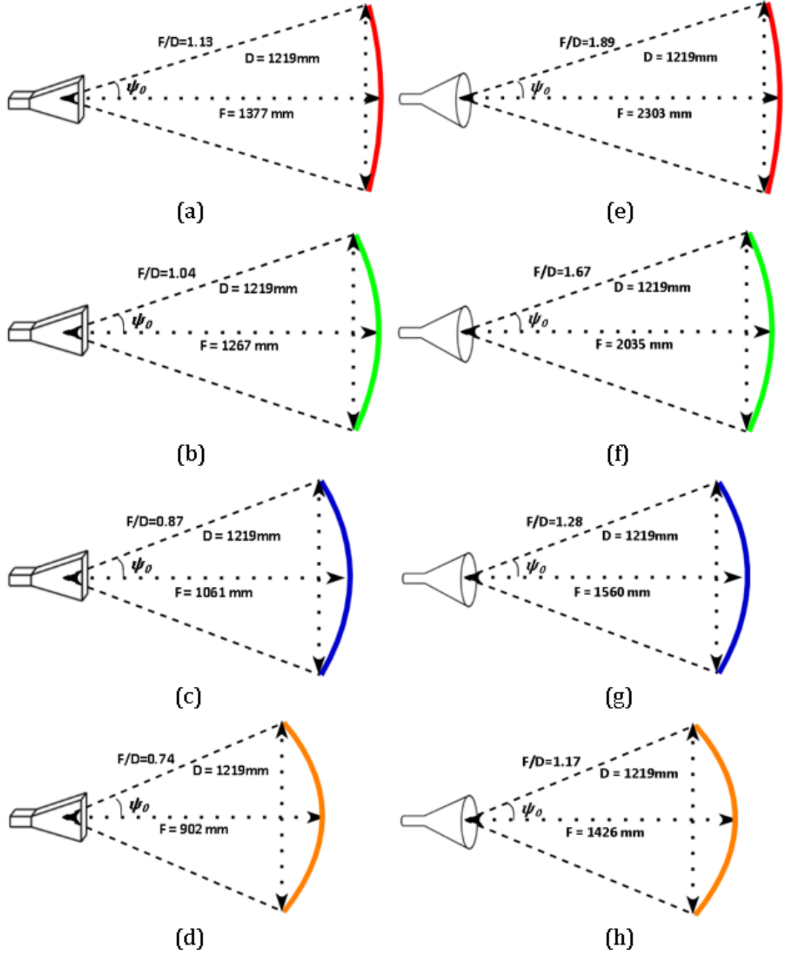
Şekil 4.4 Piramit (a, b, c, d) ve konik (e, f, g, h) horn antenlerle beslenmiş kenar azalması değeri (a, e) 8 dB (b, f) 10 dB (c, g) 15 dB (d, h) 20 dB olan reflektör antenler [53]
