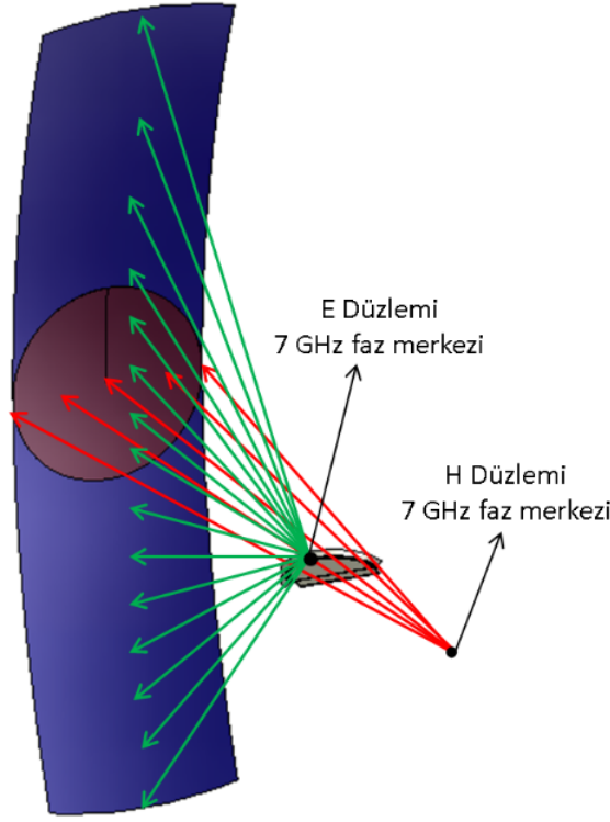
Şekil 6.35 Düzlemsel lens anten beslemeli şekillendirilmiş reflektör yapısı
