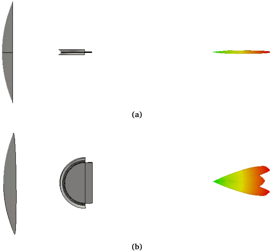
Şekil 6.21 F/D=0.6 Düzlemsel Lens Anten Beslemeli Reflektörün 3 Boyutlu Işınım Örüntüsü (a) E düzlemi (b) H düzlemi
