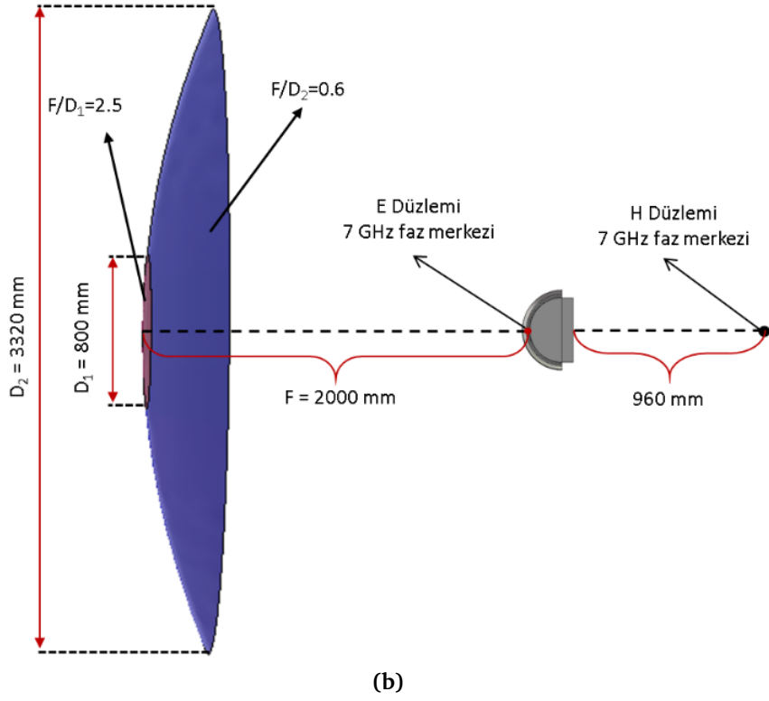
Şekil 6.32 Düzlemsel lens anten beslemesi kullanılarak tasarlanan reflektör yapısı (a) E-düzlemi ve (b) H-düzlemi
