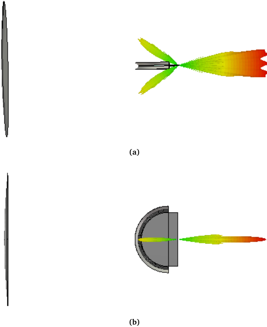
Şekil 6.18 F/D = 2.5 düzlemsel lens anten beslemeli reflektörün 3 boyutlu ışıma örüntüsü (a) E düzlemi (b) H düzlemi
