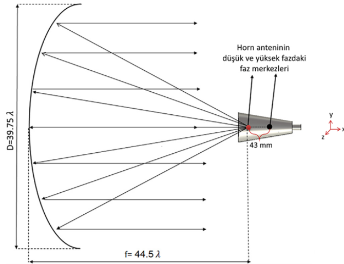
Şekil 4.10 Oluklu horn tarafından beslenen parabolik reflektör anten [60]
