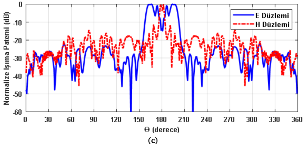
Şekil 6.20 F/D=0.6 düzlemsel lens anten beslemeli reflektöre ait E ve H düzlemi normalize ışınım paternleri (a)4 GHz, (b)7 GHz ve (c)12 GHz
