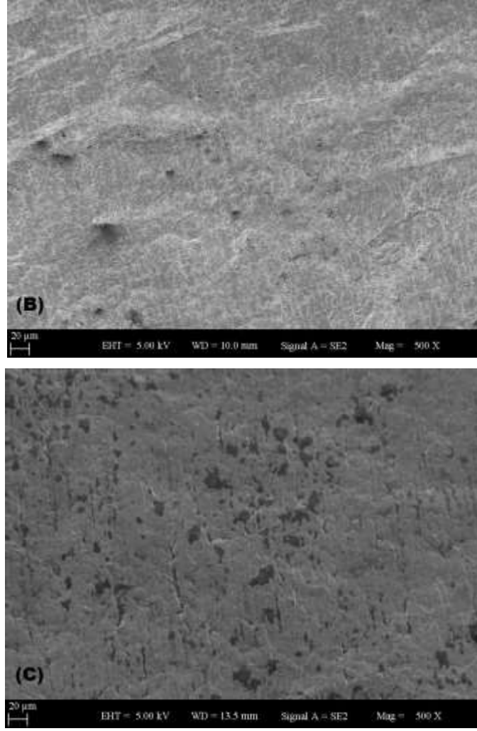
Şekil 7.5 Bindirme birleştirme yöntemiyle azot gazı kullanılarak sert lehimlenmiş bakır borulara ait ısı tesiri altında kalan bölgenin yüzey görüntüleri A-650°C, B-750°C, C-800°C (devamı)
