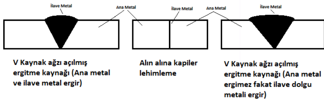
Şekil 3.1 Ergitme Kaynağı, Kapiler Lehimleme ve Lehim Kaynağı birleştirme şekillerinin şematik gösterimi [14]
