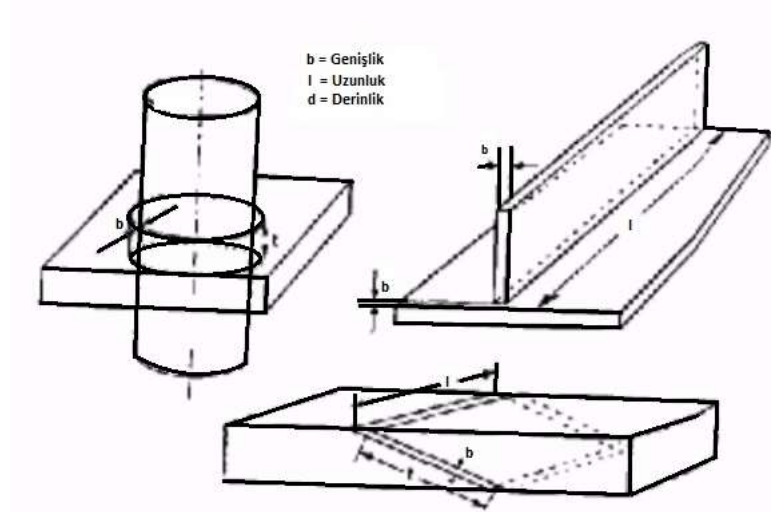
Şekil 3.5 Lehimleme aralığının boyutları [20]
