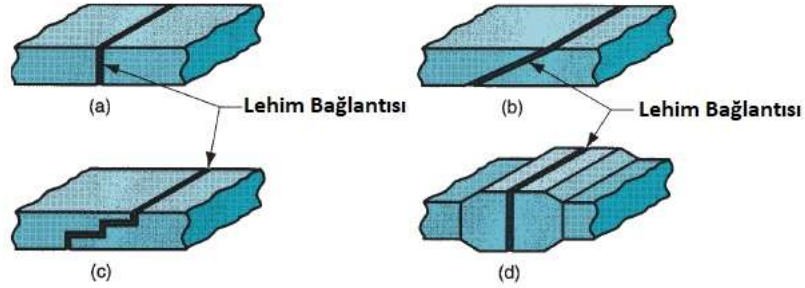
Şekil 3.17 (a) Geleneksel alın alına lehimleme ve uygulamaları: (b) Eğik alın alına bağlantı, (c) kademeli alın alına bağlantı, (d) bağlantı noktasındaki parçanın kesitinin artması [29]
