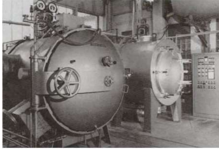
Şekil 3.10 Vakum ortamında sert lehimleme iin kullanılan fırınlar [16]
