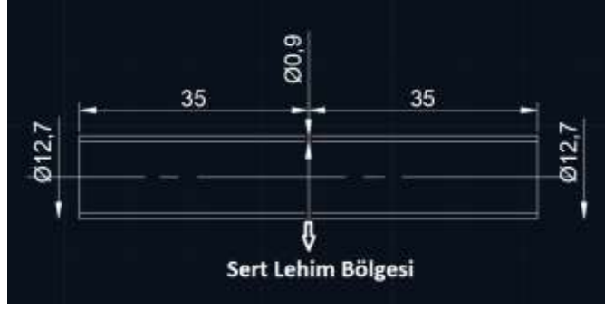
Şekil 6.2 Alın altına yöntemiyle sert lehimlenmiş bakır boru numune boyutları
