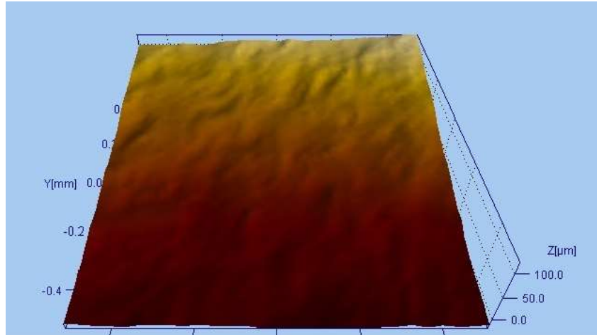
Şekil 7.11 Azot gazı kullanılmadan sert lehimlenmiş numuneye ait yüzey görünümü
