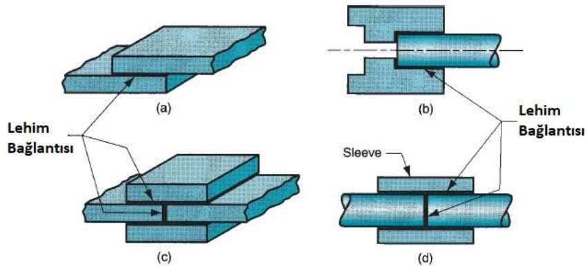
Şekil 3.18 (a) Geleneksel bindirme bağlantısı ve uygulamaları: (b) silindirik parçalar, (c) sandviç parçalar ve (d) Alın alına bağlantının bindirme bağlantıya dönüştürülmesi için ek parça kullanılması [29]
