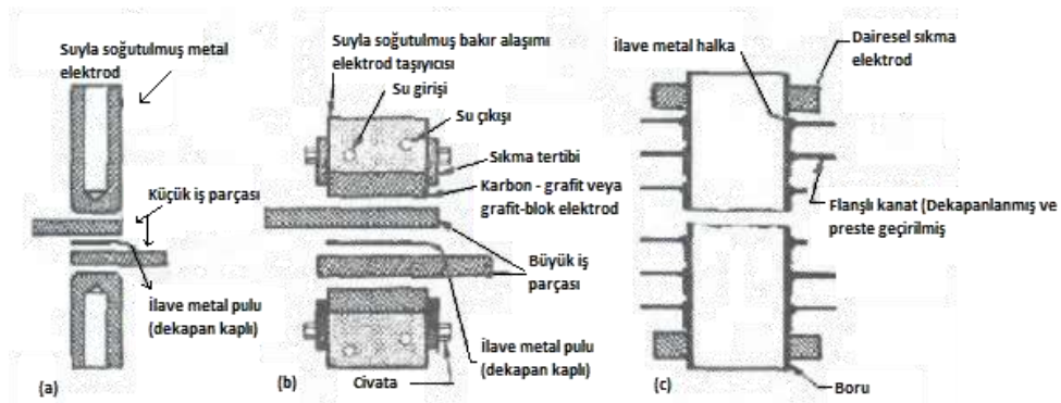
Şekil 3.14 Direnç sert lehimlemesi için tertipler: (a) Karşılıklı suyla soğutulmuş metal elektrotlar (normal direnç kaynağı tipi) kullanan küçük yassı parçalar; (b) suyla soğutulmuş bakır alaşımından taşıyıcılara bağlanmış karşılıklı karbon blok elektrotları kullanan büyük yassı parçalar, (c) dairesel olarak kavrayan elektrotların kullanıldığı boruya kanat sert lehimlenmesi [22]
