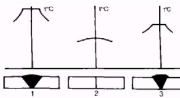
Şekil 3.4 Eritme kaynağı, lehim kaynağı ve kapiler lehimleme için ağızların şekli ve sıcaklık dağılımları 1) Eritme kaynağı 2) Kapiler lehimleme 3) Lehim kaynağı [20]
