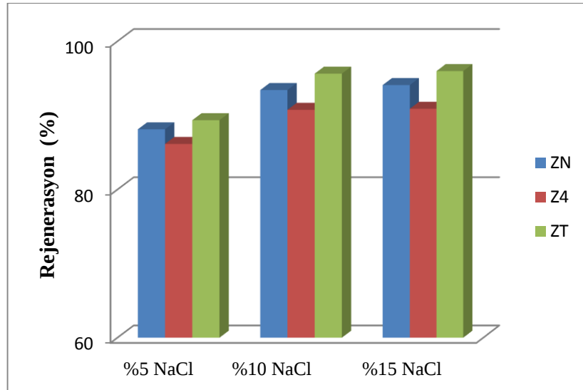
Şekil 8.33 Zeolit numunelerinin farklı rejenerant oranlarına göre rejenerasyon verimleri
