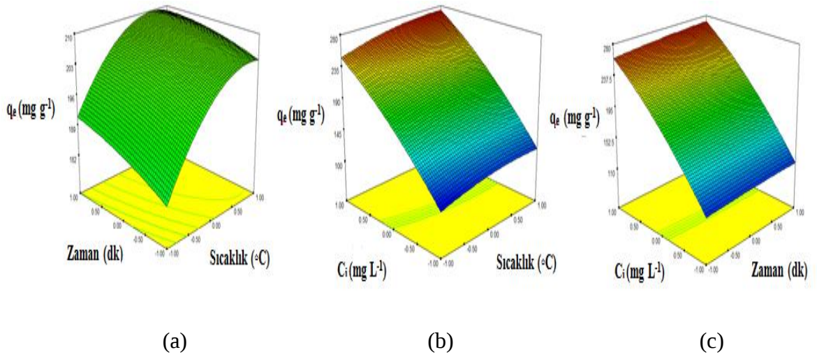
Şekil 8.27 ZT adsorbantı ile Pb(II) giderim kapasitesine parametrelerin etkisine ait cevap yüzey grafikleri (a) sıcaklık ve zaman etkisi (b) sıcaklık ve konsantrasyon (c) zaman ve konsantrasyon
