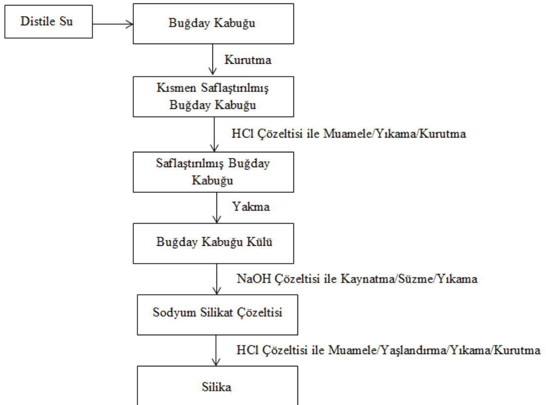
Şekil 7.1 Buğday kabuğundan silika üretimi akım şeması
