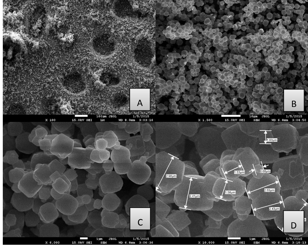
Şekil 8.9 Z 40 numunesinin SEM görüntüleri (a) X 100, (b) X 1500, (c) X 6000, (d) X 10000
