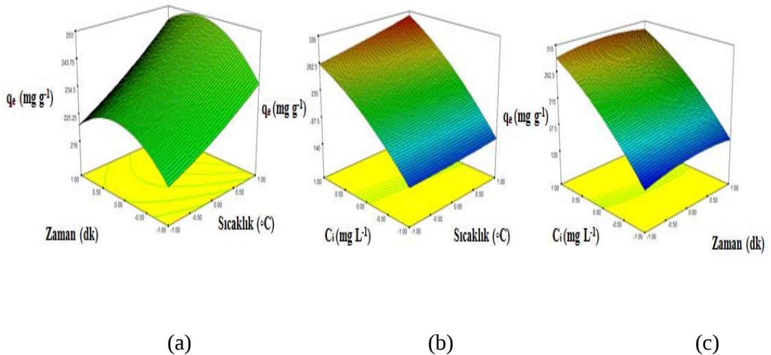
Şekil 8.26 ZN adsorbantı ile Pb(II) giderim kapasitesine parametrelerin etkisine ait cevap yüzey grafikleri (a) sıcaklık ve zaman etkisi (b) sıcaklık ve konsantrasyon (c) zaman ve konsantrasyon
