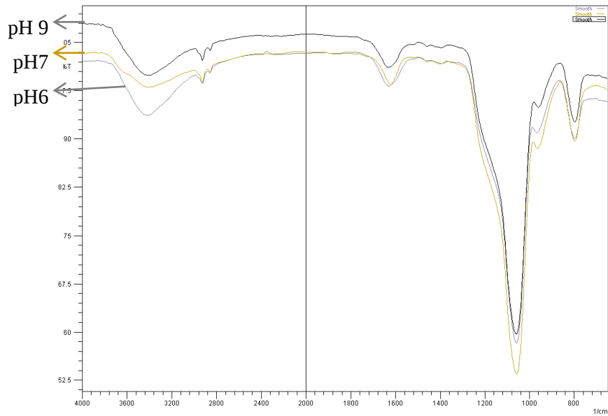
Şekil 8.3 Silika aerogel numunelerinin FT-IR spektrumu
