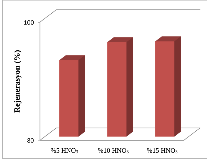
Şekil 8.39 Silika aerjel numunesinin farklı rejenerant oranlarına göre rejenerasyon verimleri
