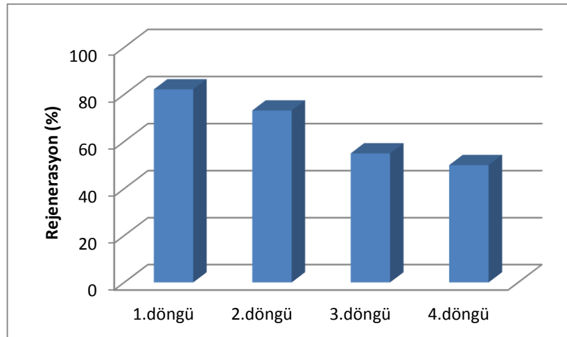
Şekil 8.40 Silika aerjel numunesinin rejenerasyon yüzdeleri
