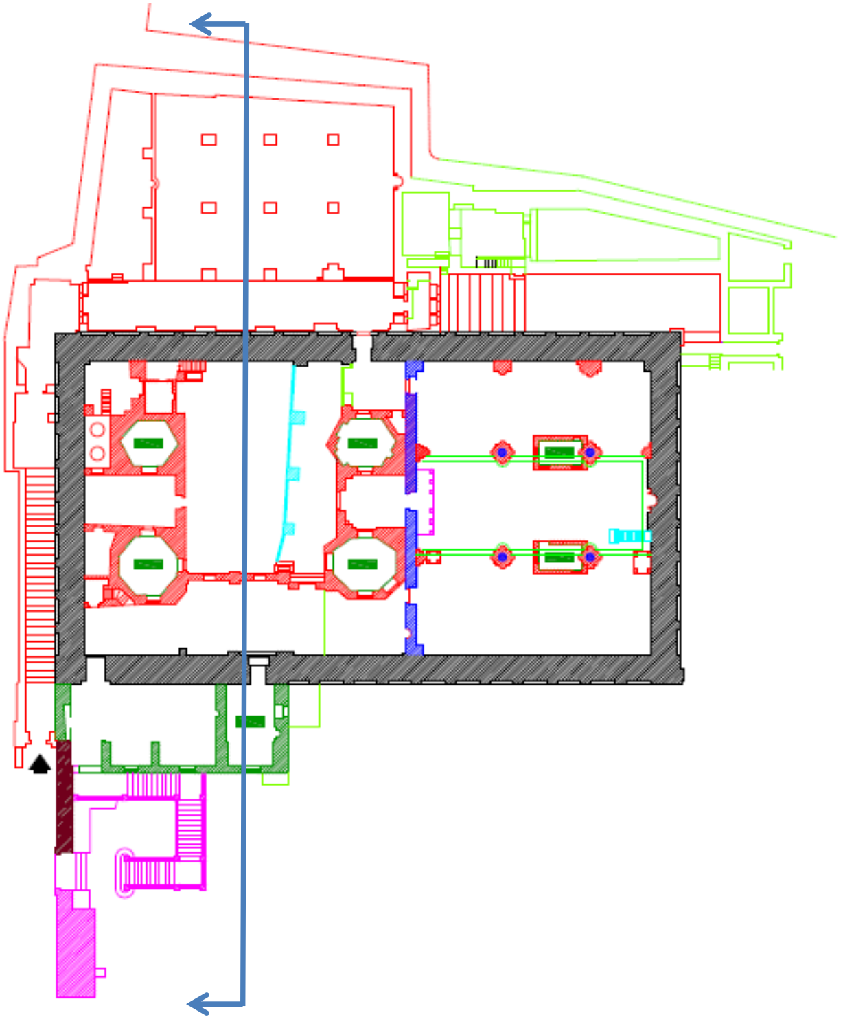
Şekil 2.86 (a) İsraili Döneminde, El-Harem El-İbrahimi'nin Planı, (Al-Shweiky, 2014), (b) İsrail Döneminde, El-Harem El-İbrahimi'nin Kesitleri, (Al-Shweiky, 2014)
