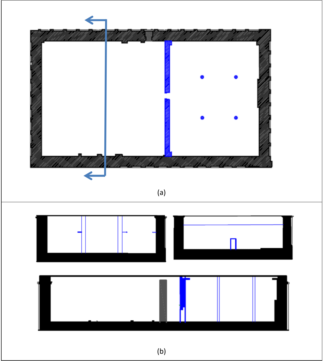
Şekil 2.24 (a) Emeviler Döneminde El-Harem El-İbrahimi'nin Planı, (Al-Shweiky, 2015), (b) Emeviler Döneminde El-Harem El-İbrahimi'nin Kesitleri, (Al-Shweiky, 2015)
