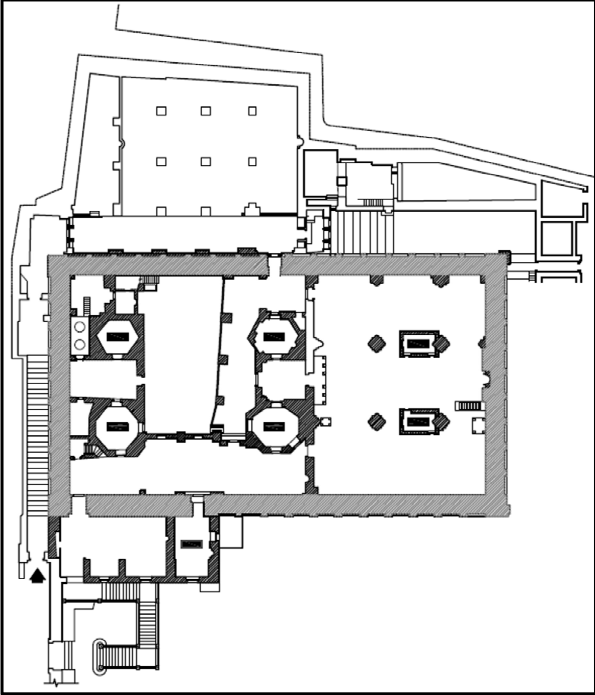
Şekil 3.6 El-Harem El-İbrahimi'nin Planı, (HRC [24], 2003)
