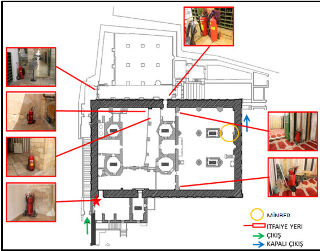
Şekil 4.5 El-Harem El-İbrahimi Yapısında Yangın Çıkması Durumunda Kullanılabilecek Ekipmanlar (Al-Shweiky, 2015)
