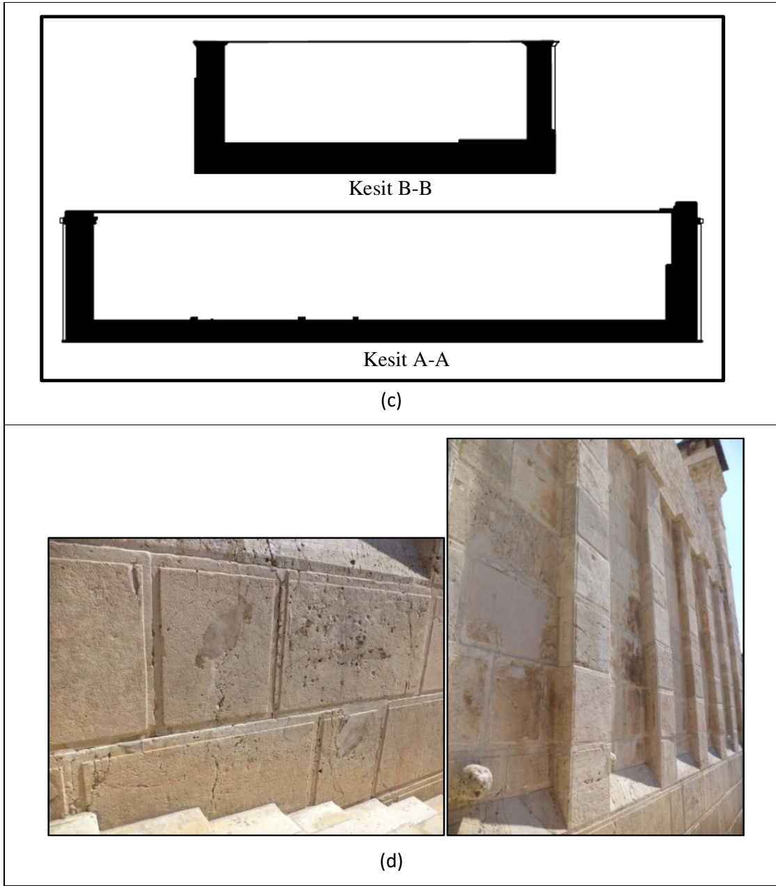
Şekil 2.16 (a) Romalılar Döneminde Mağara ve Sur Planı, (Düzenleme: Al-Shweiky, 2014), (b) Romalılar Döneminde Sur Planı, (Al-Shweiky, 2014), (c) Romalılar Döneminde Sur Kesitleri, (Al-Shweiky, 2014 ), (d) Herod Tarafından İnşa Ettirilen Sur Duvarları, (Al-Shweiky, 2013) (Devam)
