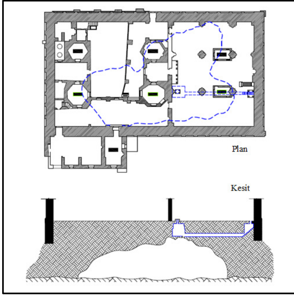
Şekil 2.52 (a) Mağara Planı (Vincent [157]), Mağara Üst Katı, (URL [120]), (b) Mağara Planı ve Kesti, (Al-Shweiky, 2015) (Devam)
