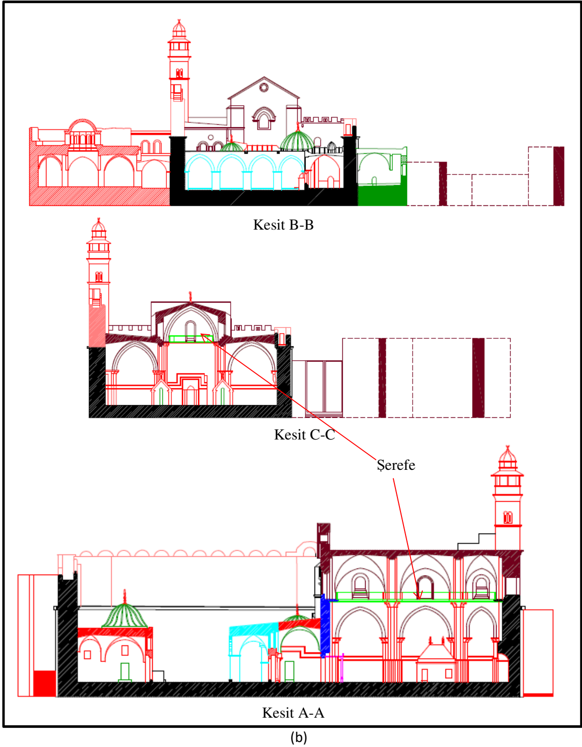
Şekil 2.57 (a) Birinci Osmanlı Döneminde, El- Harem El-İbrahimi'nin Planı, (Al-Shweiky, 2014), (b) Birinci Osmanlı Döneminde, El-Harem El-İbrahimi'nin Kesitleri, (Al-Shweiky, 2014) (Devam)
