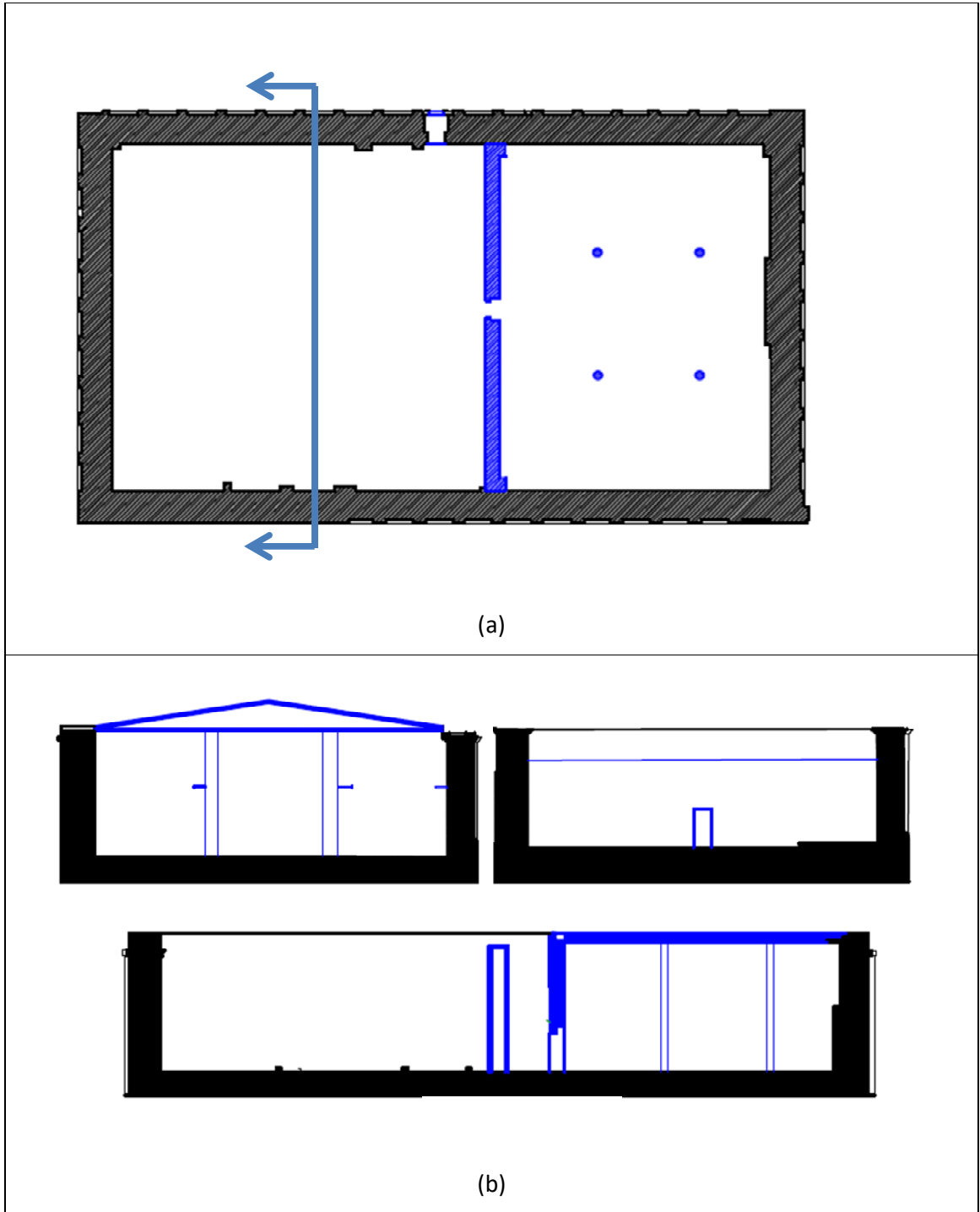
Şekil 2.20 (a) Bizanslılar Döneminde Yapının Planı, (Al-Shweiky, 2015), (b) Bizanslılar Döneminde Yapının Kesitleri, (Al-Shweiky, 2015)
