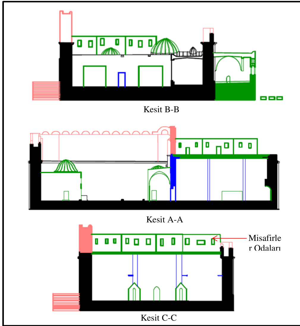
Şekil 2.27 (a) Fatımiler Döneminde El-Harem El-İbrahimi'nin Planı, (Al-Shweiky, 2014), (b) Fatımiler Döneminde El-Harem El-İbrahimi'nin Kesitleri, (Al-Shweiky, 2014)
