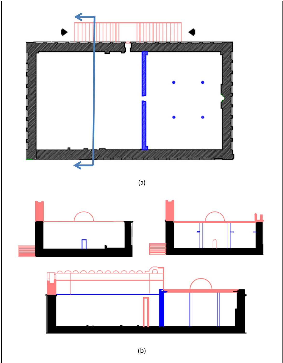
Şekil 2.25 (a) Abbasiler Döneminde El-Harem El-İbrahimi'nin Planı, (Al-Shweiky, 2014), (b) Abbasiler Döneminde El-Harem El-İbrahimi'nin Kesitleri, (Al-Shweiky, 2014)
