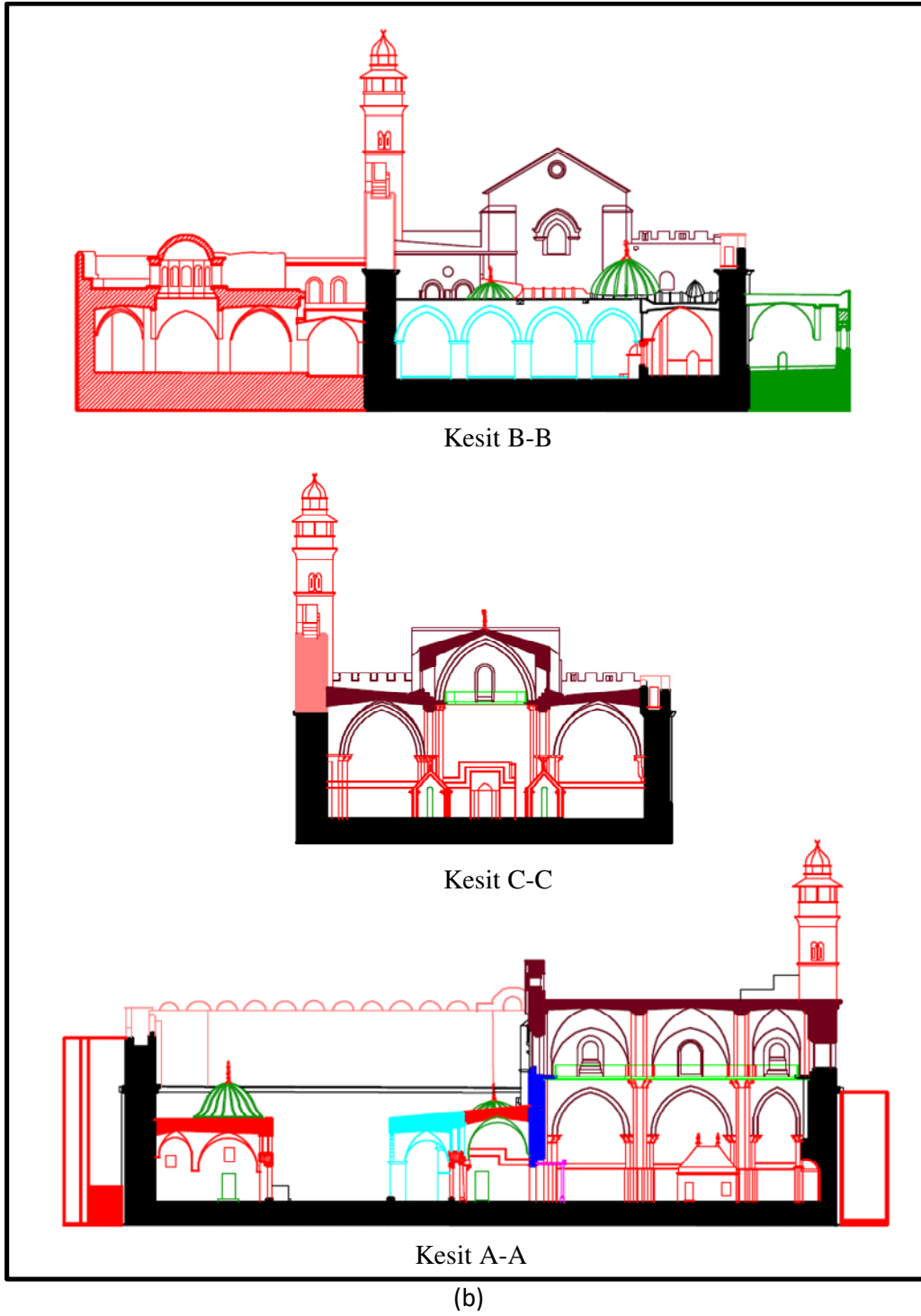
Şekil 2.83 (a) Ürdün Döneminde, El-Harem El-İbrahimi'nin Planı, (Al-Shweiky, 2014), (b) Ürdün Döneminde, El-Harem El-İbrahimi'nin Kesitleri, (Al-Shweiky, 2014) (Devam)
