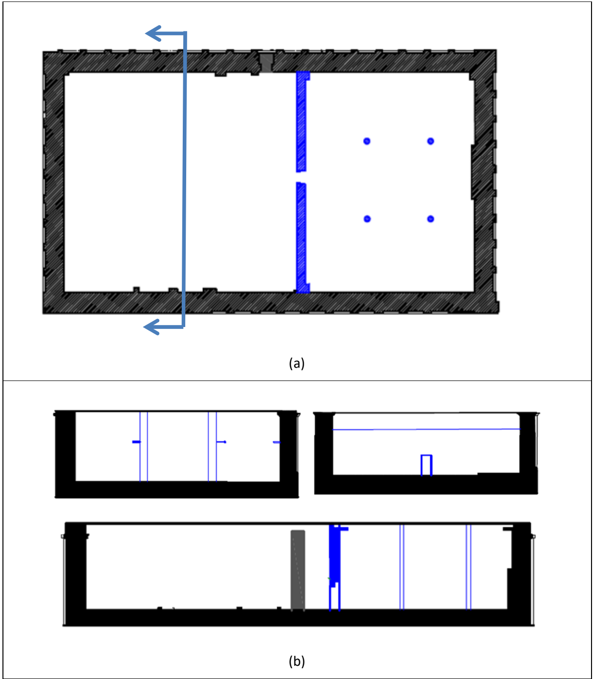
Şekil 2.23 (a) Dört Halife Döneminde El-Harem El-İbrahimi'nin Planı, (Al-Shweiky, 2015), (b) Dört Halife Döneminde El-Harem El-İbrahimi'nin Kesitleri, (Al-Shweiky, 2015)
