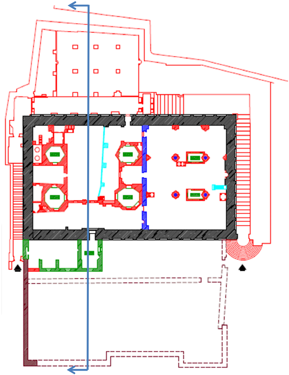
Şekil 2.51 (a) Memluklar Döneminde, El-Harem El-İbrahimi'nin Planı, (Al-Shweiky, 2014), (b) Memluklar Döneminde, El-Harem El-İbrahimi'nin Kesitleri, (Al-Shweiky, 2014)
