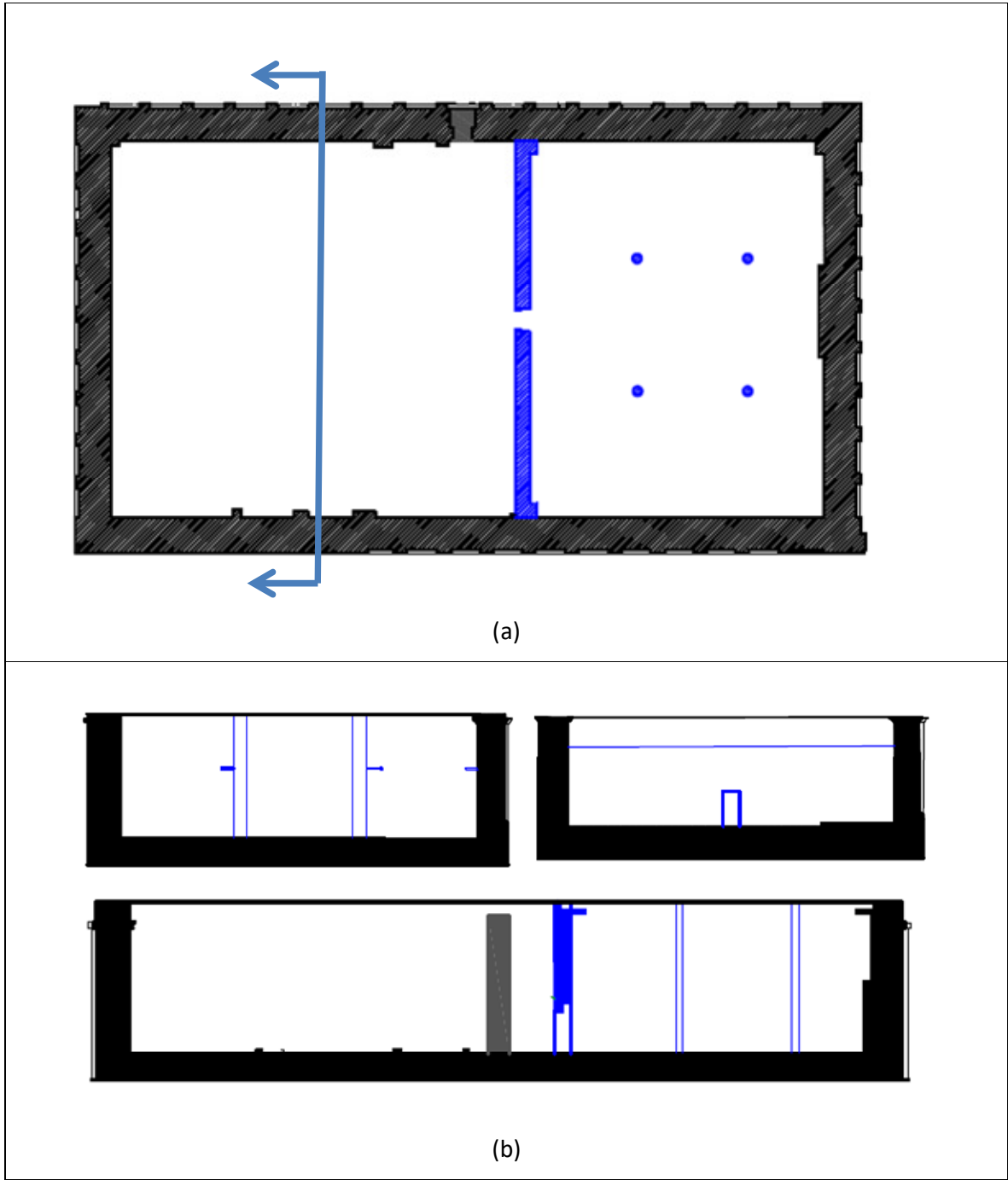
Şekil 2.21 (a) Sasaniler Döneminde Yapının Planı, (Al-Shweiky, 2015) (b) Sasaniler Döneminde Yapının Kesitleri, (Al-Shweiky, 2015)
