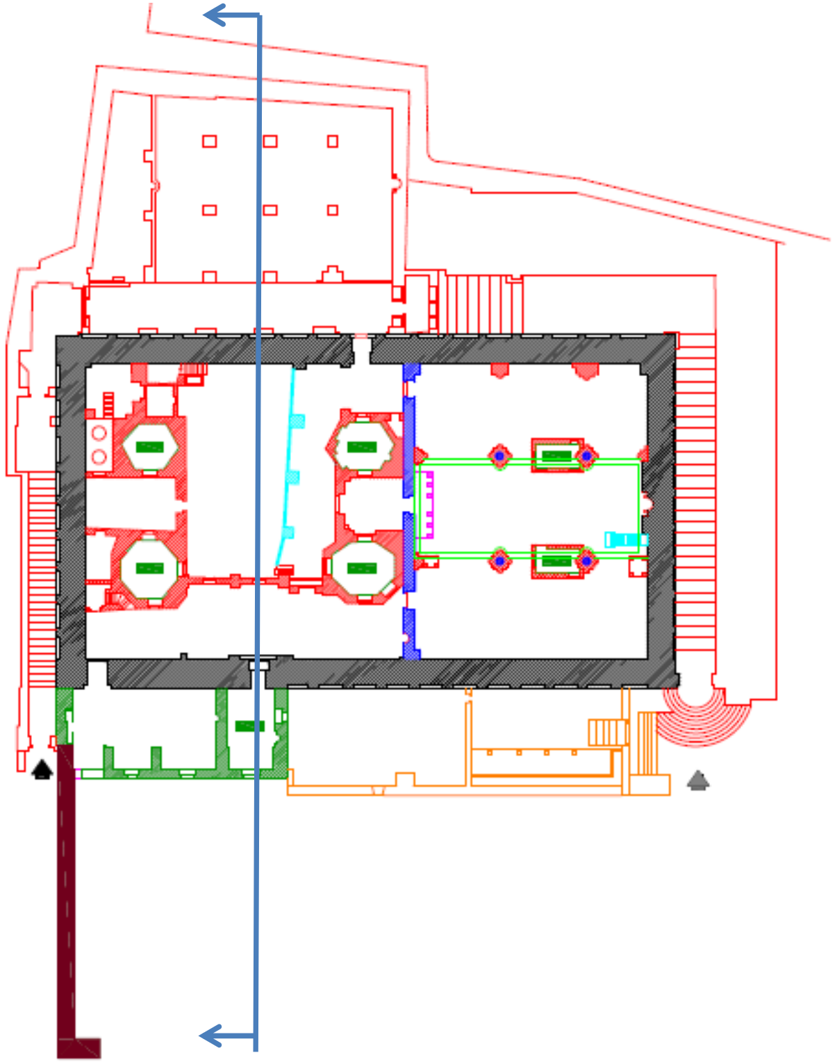
Şekil 2.75 (a) İngiliz Mandası Döneminde, El-Harem El-İbrahimi'nin Planı, (Al-Shweiky, 2014), (b) İngiliz Mandası Döneminde, El-Harem El-İbrahimi'nin Kesitleri, (Al-Shweiky, 2014)
