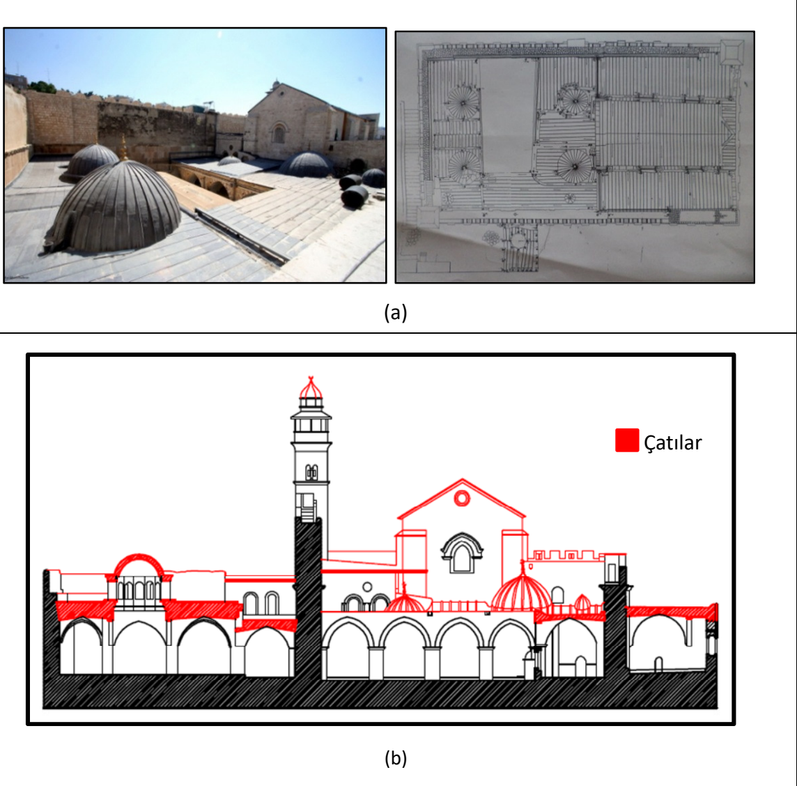
Şekil 3.24 (a) El-Harem El-İbrahimi'nin Çatıları ve Kurşun Levhalar Planı, (URL [133]), (El-Avkaf), (b) El-Harem El-İbrahimi'nin Çatıların Kesiti, (Al-Shweiky, 2013)
