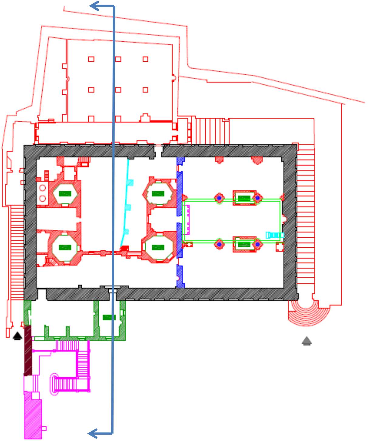
Şekil 2.83 (a) Ürdün Döneminde, El-Harem El-İbrahimi'nin Planı, (Al-Shweiky, 2014), (b) Ürdün Döneminde, El-Harem El-İbrahimi'nin Kesitleri, (Al-Shweiky, 2014)
