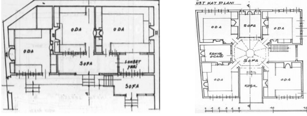
Şekil 5.13 Çankırı geleneksel konutlarının iç ve orta sofalı planları [139]
