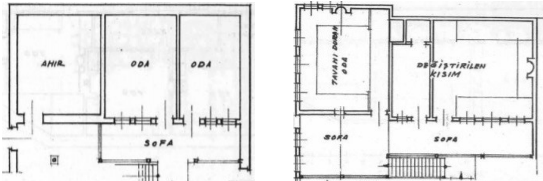
Şekil 5.12 Çankırı geleneksel konutları dış sofalı plan tipleri [139]
