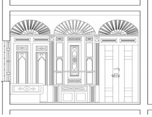
Şekil 3.51 Osman Çavuş evinin yüklük ve şerbetliği [84]
