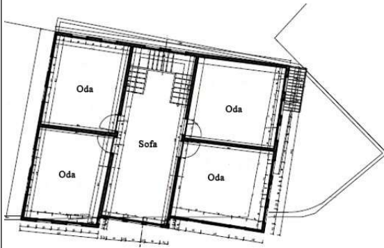
Giriş: Su Deposu Caddesi 5.b- Zemin kat planı
