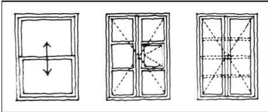
Şekil 2.33 Geleneksel Türk evindeki pencere açılış yönleri [18]
