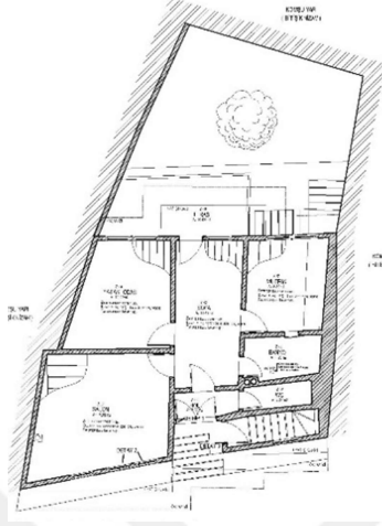
Giriş: Buğdaypazarı Mahallesi 72.a- Zemin kat planı
