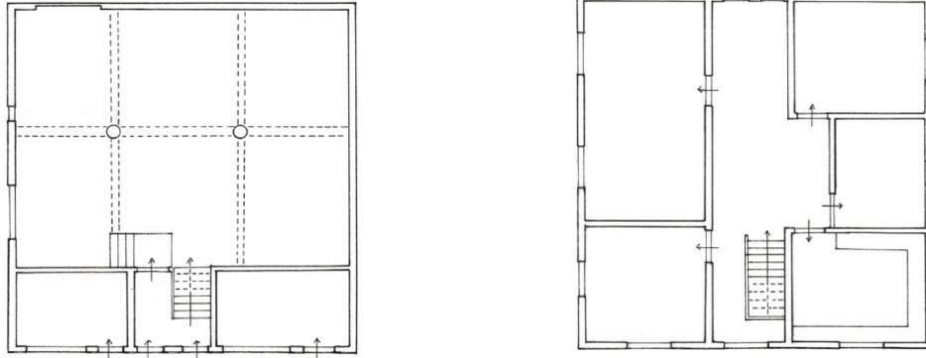
Şekil 4.101 Etnografya Müzesi'nin alt ve üst katların iç sofalı plan tipleri [132]
