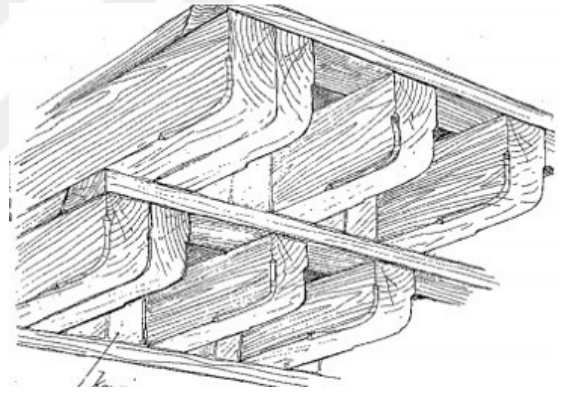
Şekil 3.19 Üst katı destekleyen çıkma taşıyıcıları [70]
