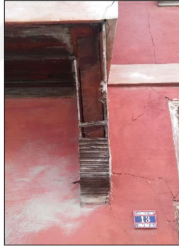
75.b- Kıvrımlı ahşap payandalar
