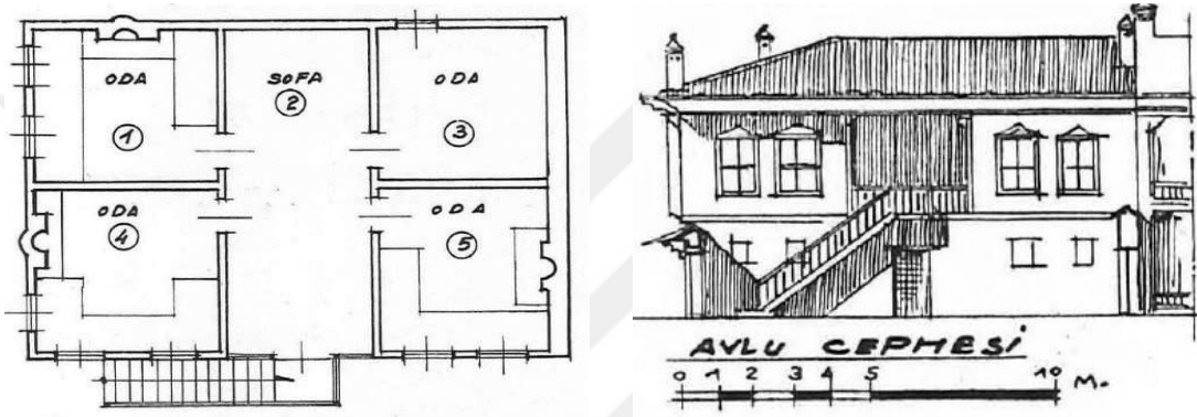
Şekil 3.38 Bezginoglu konutu planı ve cephe biçimlenişi [76]
