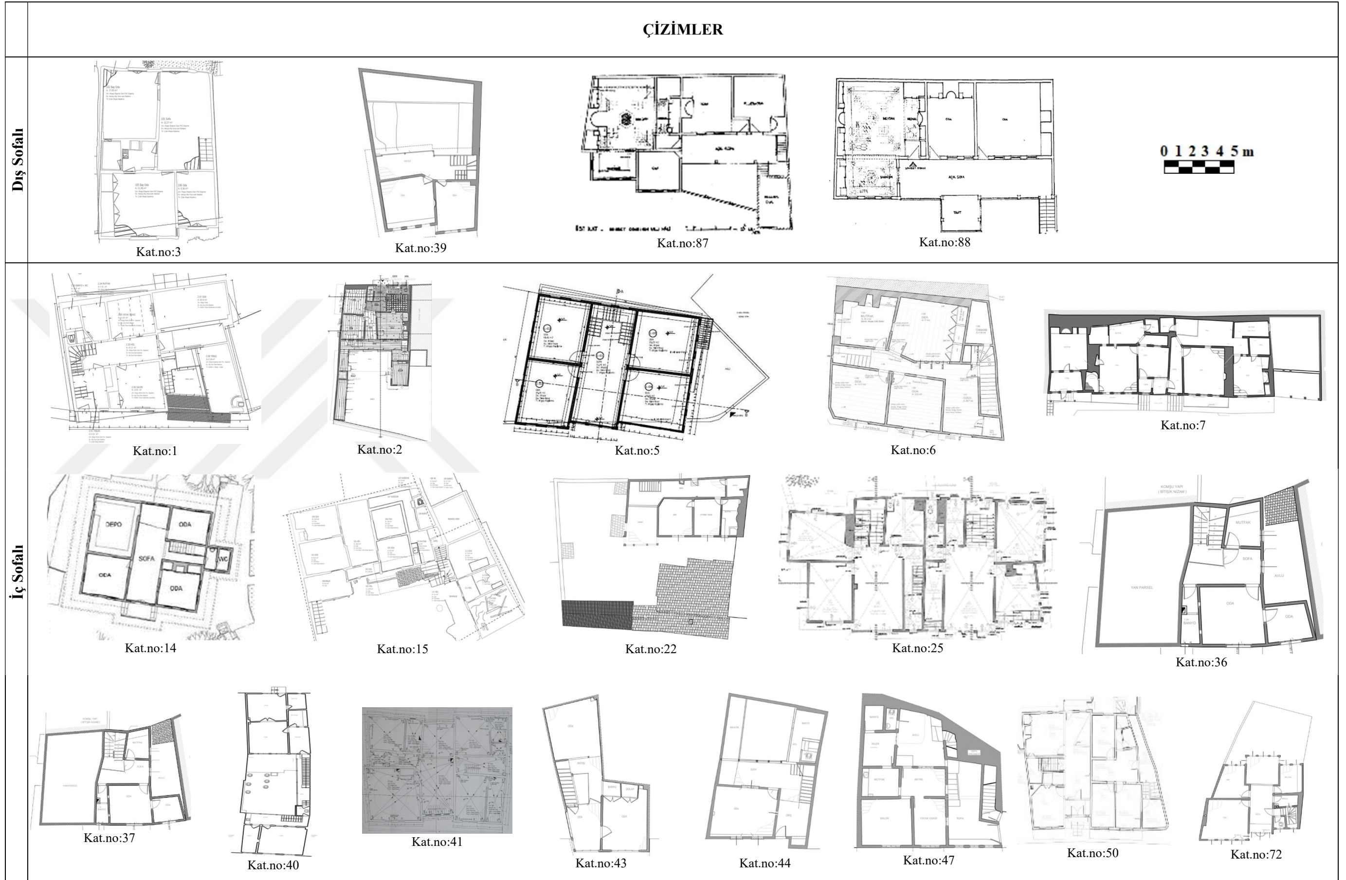
Şekil 5.15 Çankırı merkez ilçe geleneksel konutlarının plan tiplerinin tipolojisi
