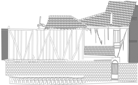
15.ı- C – C kesiti
