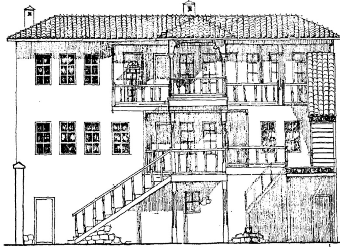
88.b- Doğu görünüşü [130]
