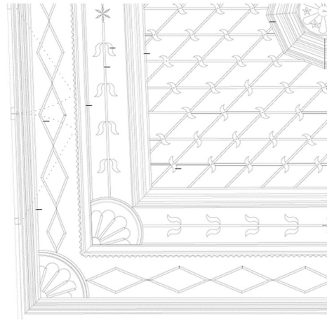
3.p- Çıtakâri tekniğinde yapılan ahşap çıtalı köşeleri bitkisel bezemeli tavan görünüşü
