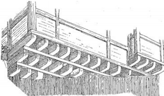
Şekil 3.20 Üst katı destekleyen çıkma taşıyıcıları [70]
