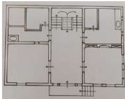
Şekil 6.2 Atkaracalar İlçesi Rifat Ulusoy konutunun iç sofalı plan tipi [131]
