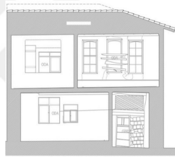
39.h- B-B kesiti
