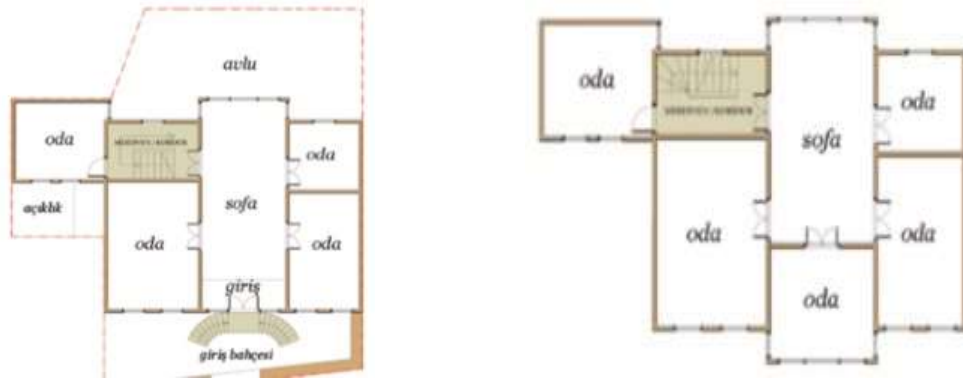
Şekil 3.16 Birlik Sokak 3 No'lu konutun zemin ve birinci katın iç sofalı plan tipi [71]
