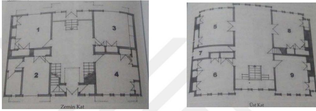
Şekil 5.14 Misafir evi zemin kat ve üst kat planları [144]
