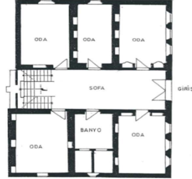
Şekil 6.3 Nevşehir geleneksel konutu iç sofalı plan tipi [91]
