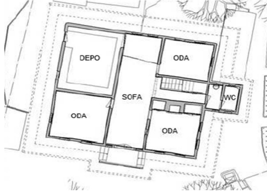
Şekil 6.1 Merkez İlçe katalog no:14'ün konutun iç sofalı plan tipi [129]
