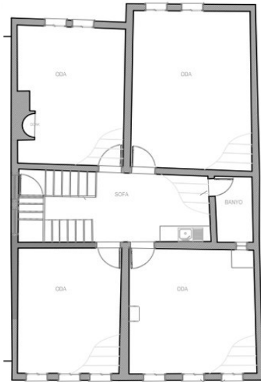
46.c- Birinci kat planı
