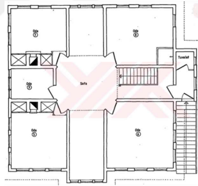
Şekil 4.110 Fişek Ali konağının alt ve üst katların iç sofalı plan tipleri [133]
