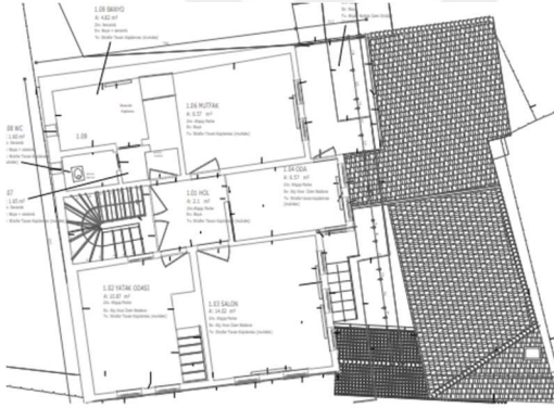
1.c- Birinci kat planı
