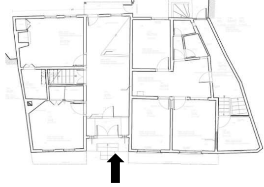
Giriş: Uzunyol Caddesi 50.b- Zemin kat planı
