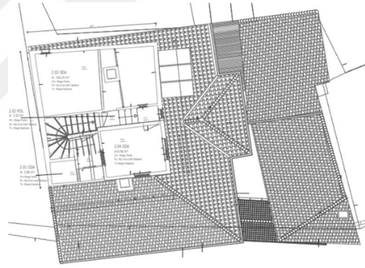
1.d- Çatı katı planı
