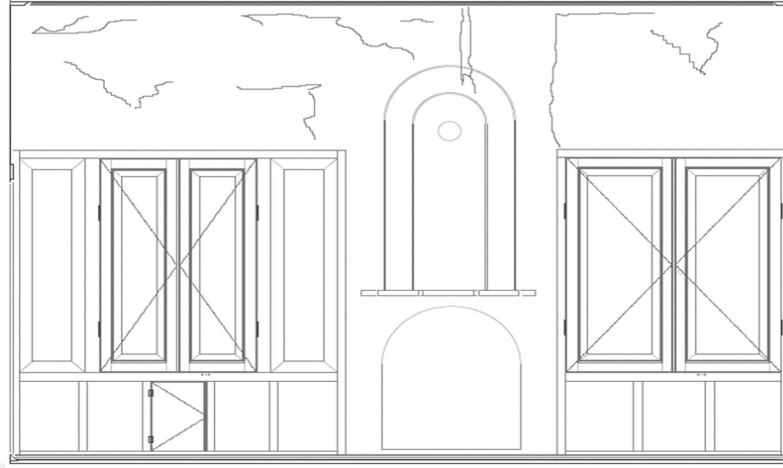
14.g- Ocak, şerbetlik ve dolap görünüşü
