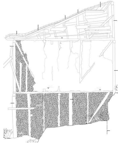
3.h- Güneydoğu görünüşü
