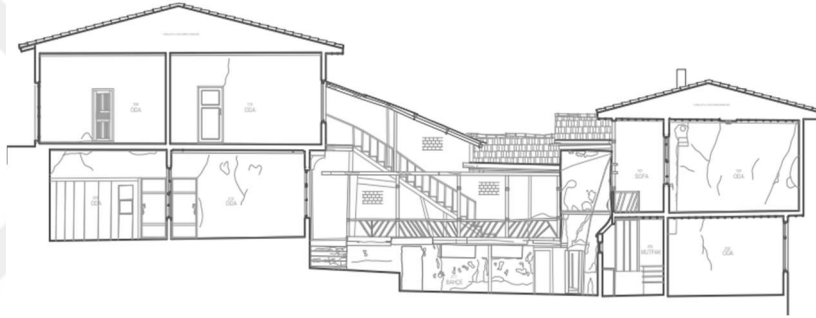
40.i- C-C kesiti
