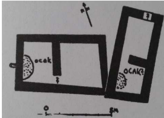
Şekil 2.8 Hitit evi planı görünüşü [29]
