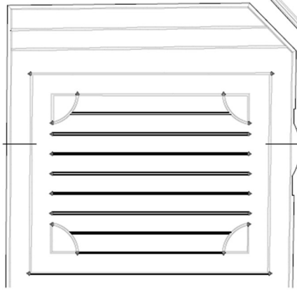
47.m- Ahşap çıtalı tavandan görünüş 0 20 40 60 80 100 cm
