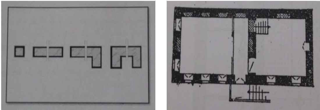
Şekil 2.19 Sofasız plan tipleri [24] [34]
