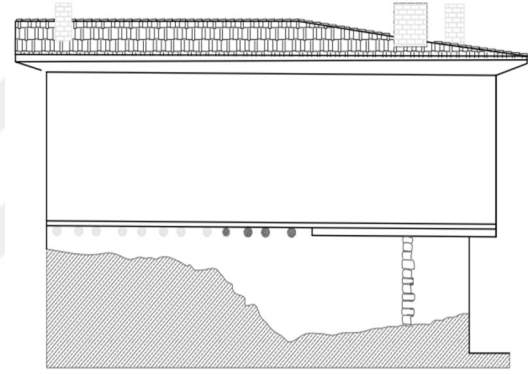
6.f- Kuzey görünüşü
