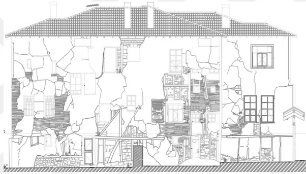
25.f- D-D kesiti
