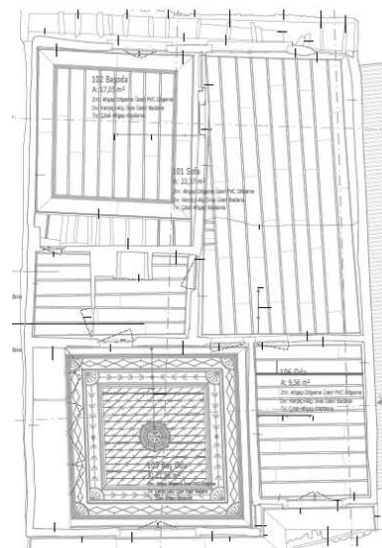
3.d- Birinci kat tavan planı
