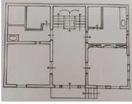
Şekil 4.102 Rıfat Ulusoy konutu alt ve üst katlarının iç sofalı plan tipleri [131]
