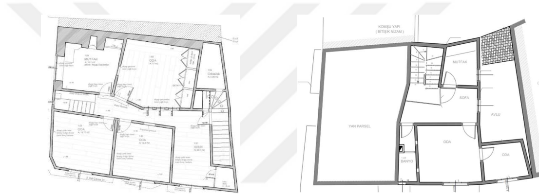
Şekil 5.8 Merkez İlçe katalog no:6 ve 36'nın konutun iç sofalı plan tipleri
