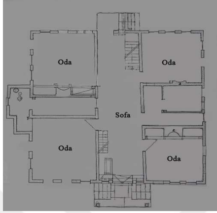
55.a- Zemin kat planı
