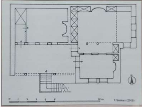
Şekil 4.154. Amir–Mahir Güney ve Fadik–Zuhre konutlarının iç sofa plan tipleri [137]
