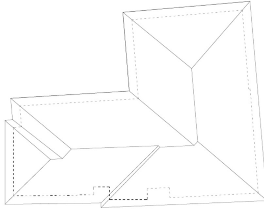
8.c- Çatı planı
