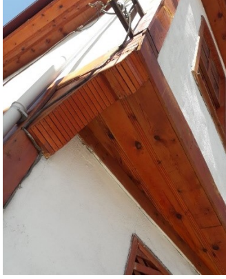
39.ö- Gönye çıkmadan diğer görünüş
