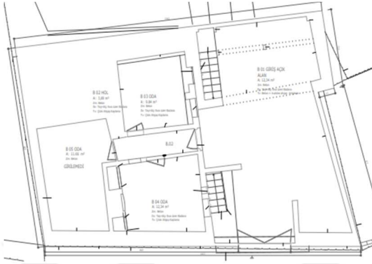
1.a- Bodrum kat planı
