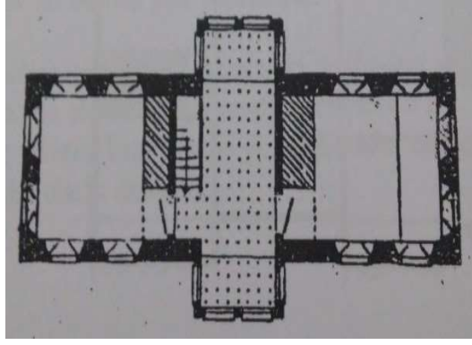
Şekil 2.22 Konya Meram'da bir konutun iç sofalı plan tipi [34]
