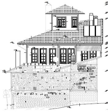
1.i- Kuzey görünüşü 0 1 2 3 4 5 metre
