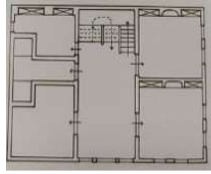
Şekil 4.102 Rıfat Ulusoy konutu alt ve üst katlarının iç sofalı plan tipleri [131]
