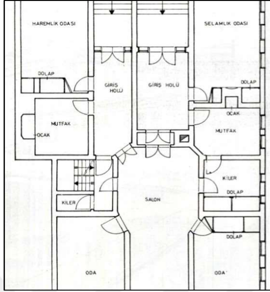
Şekil 3.84 Mütevellioğlu Mesrur Bey konutu zemin kat planı [98]
