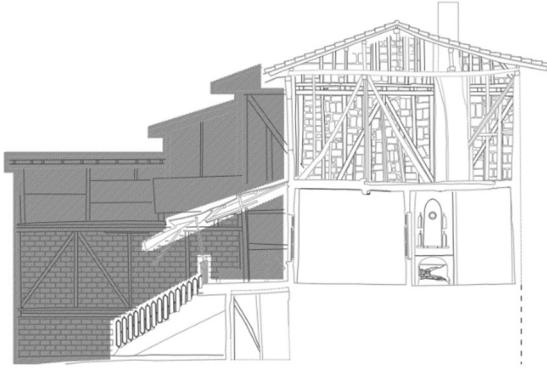
15.g- A-A kesiti
