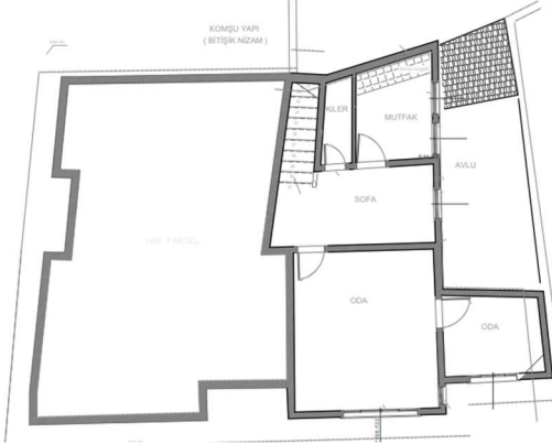
37.c- İkinci kat planı
