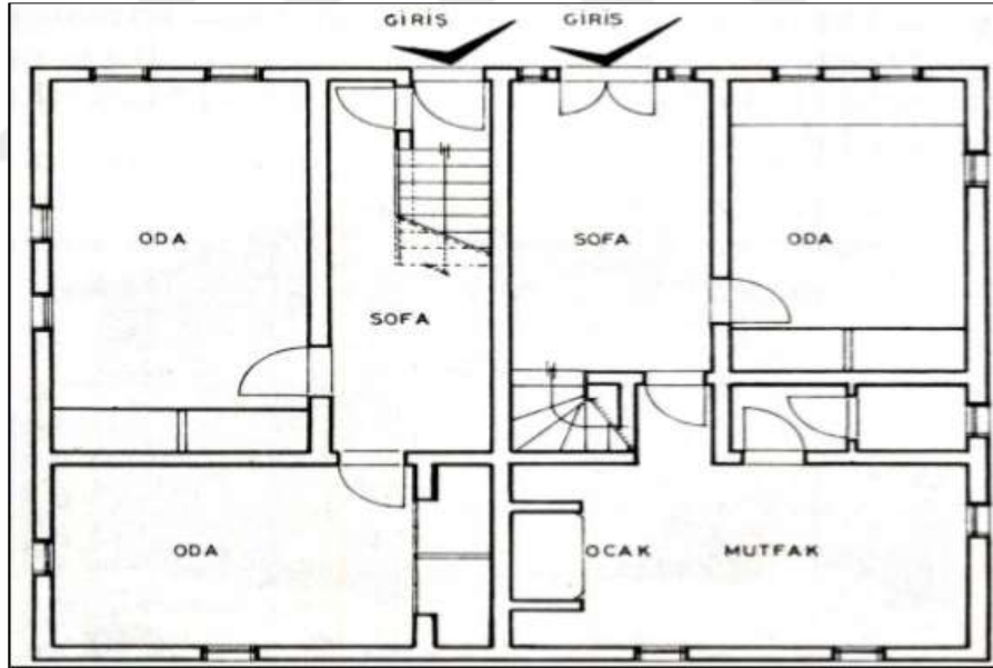
Şekil 3.85 Akaylar konağı zemin kat planı [98]
