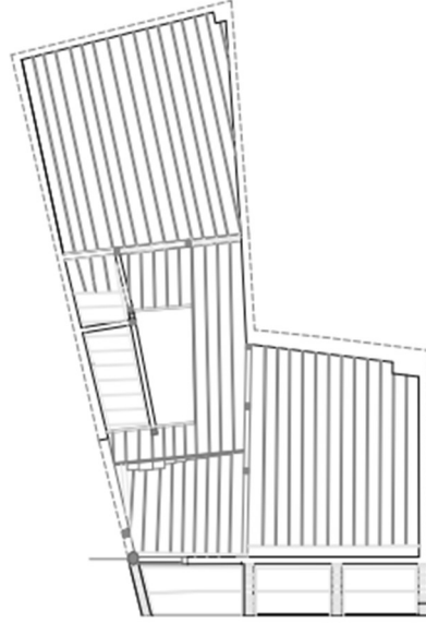
43.d- Zemin kat tavan planı
