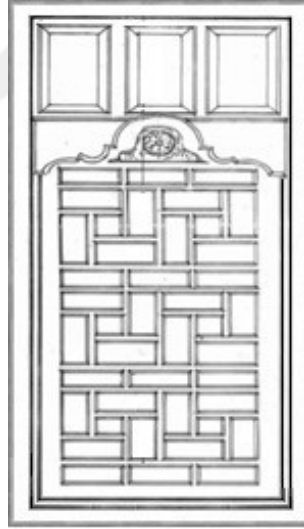
Şekil 5.6 Kündekâri tekniğinde yapılan giriş kapısı [139]
