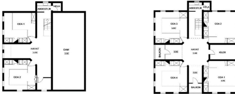
Şekil 4.123 KaraMustafagil konutunun alt ve üst kat iç sofalı plan tipleri [134]
