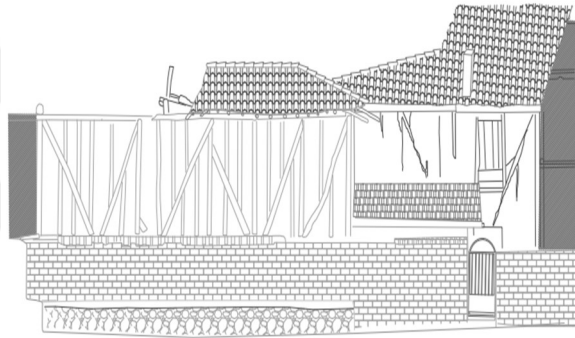
10.i- C-C kesiti
