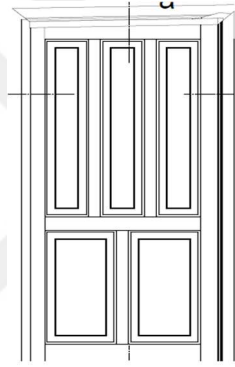
43.j- Giriş kapısından görünüş
