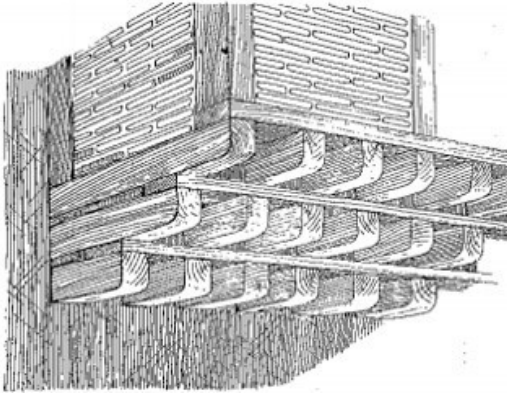
Şekil 3.19 Üst katı destekleyen çıkma taşıyıcıları [70]
