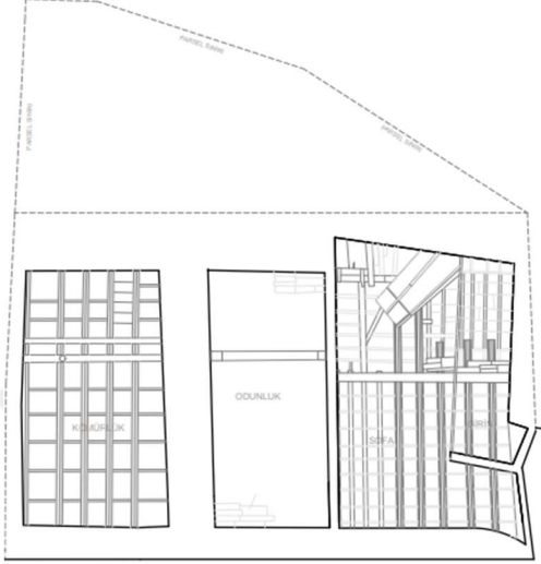
47.d- Bodrum kat tavan planı
