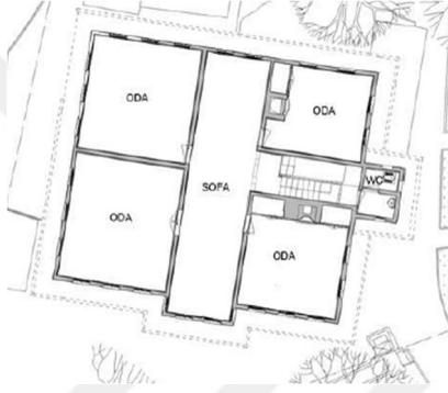
14.c- Birinci kat planı [129]
