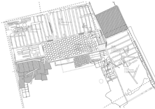
10.c- İkinci kat planı
