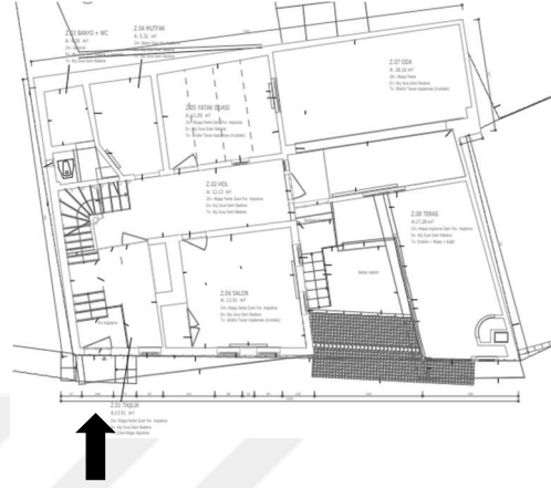
Giriş: Şehit Alparslan Bayram Sk. 1.b- Zemin kat planı
