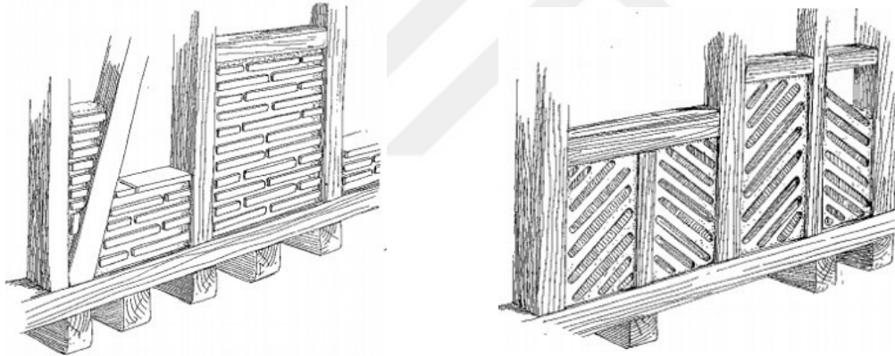
Şekil 3.17 Ahşap çatkı arası kerpiç ve tuğla dolgu [70]
