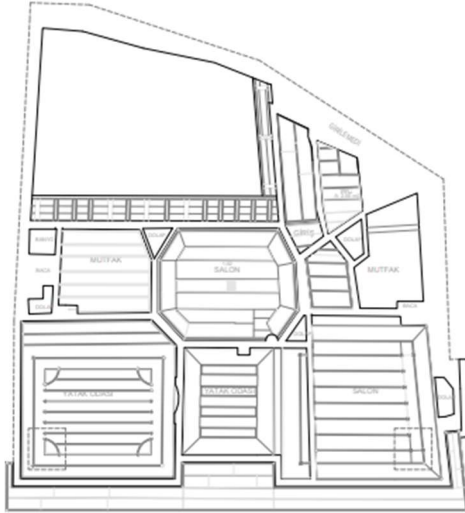
47.f- Birinci kat tavan planı
