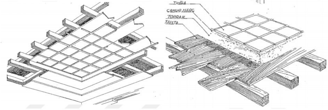
Şekil 3.22 Taban ve tavanların görünüşleri [70]
