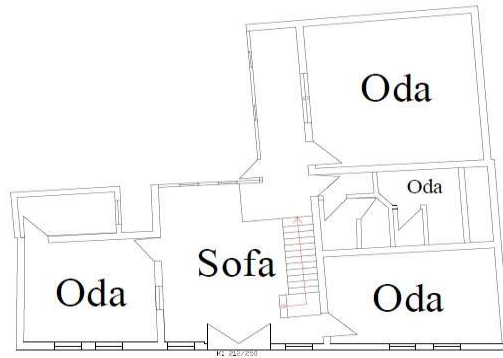
Şekil 5.9 Merkez İlçe katalog no:8'in konutun ters L sofalı plan tipi
