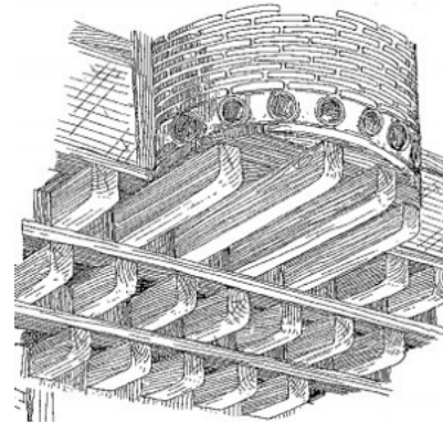
Şekil 3.20 Üst katı destekleyen çıkma taşıyıcıları [70]
