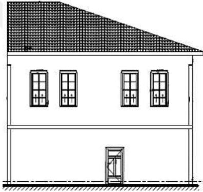
5.g- Batı görünüşü
