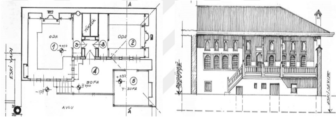
Şekil 3.34 Tekkeli Hoca konutunun planı ve cephe görünüşü [76]
