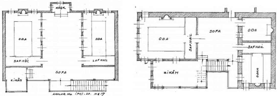
Şekil 3.15 Akalar Mahallesi İpci Sokak no 17’deki konutun dış sofalı plan tipi ile Halıcı İbrahim konutunun iç sofalı plan tipi [70]
