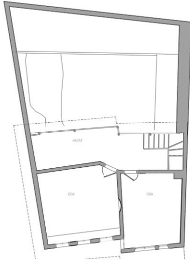
39.c- Birinci kat döşeme planı
