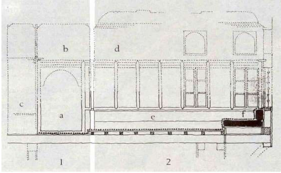
Şekil 2.30 Türk evinde döşeme ve duvar karakteristiği [17]
