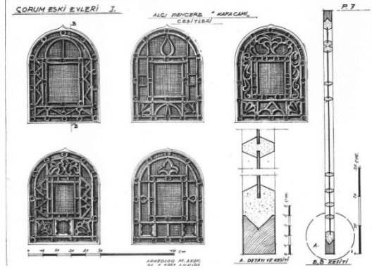
Şekil 3.35 Tekkeli Hoca konutu tepe pencereleri [76] [77]
