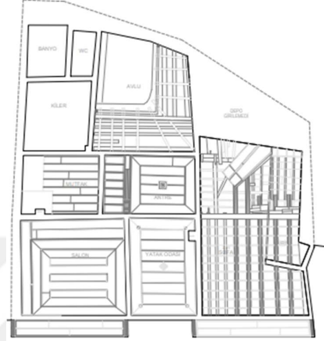
47.e- Zemin kat tavan planı
