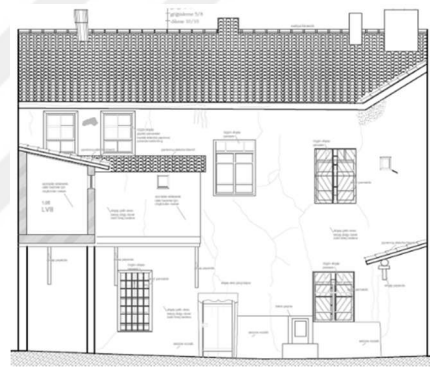
30.d- Kuzey görünüşü
