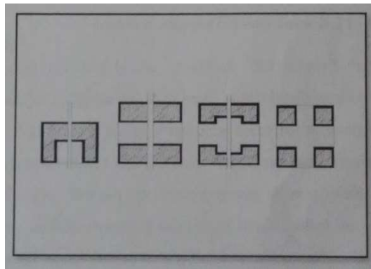
Şekil 2.21 İç sofalı plan tipi [24]
