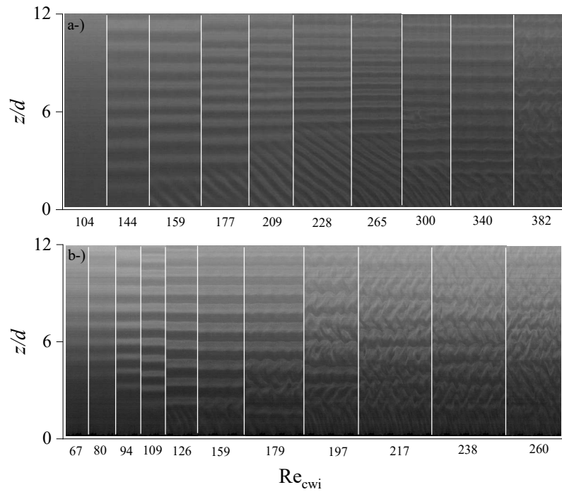
Şekil 8. 9 Xanthan çözeltisinin aynı yöne dönme koşullarında oluşan akış yapıları (a) n=0,50 ve (b) n=0,39 ( \eta=0,643 ).
