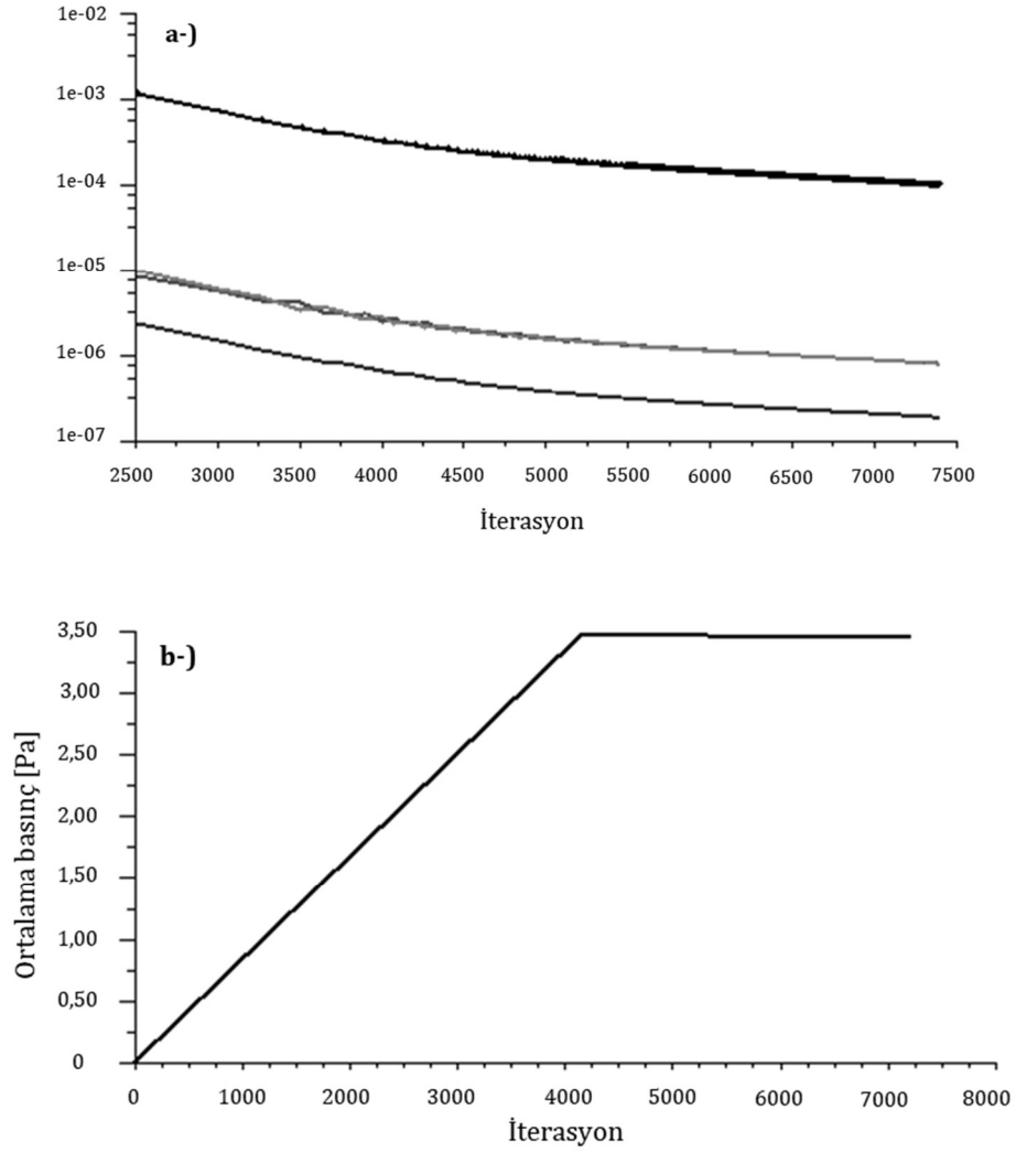
Şekil 7. 5 Simülasyon işlemi içerisinde gerçekleşen bir yakınsama örneği.
