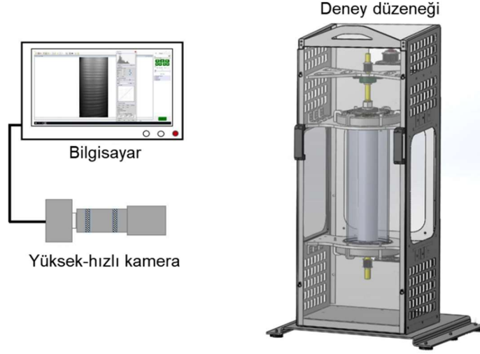
Şekil 2. 1 Deney düzeneğinin şematik görünümü.
