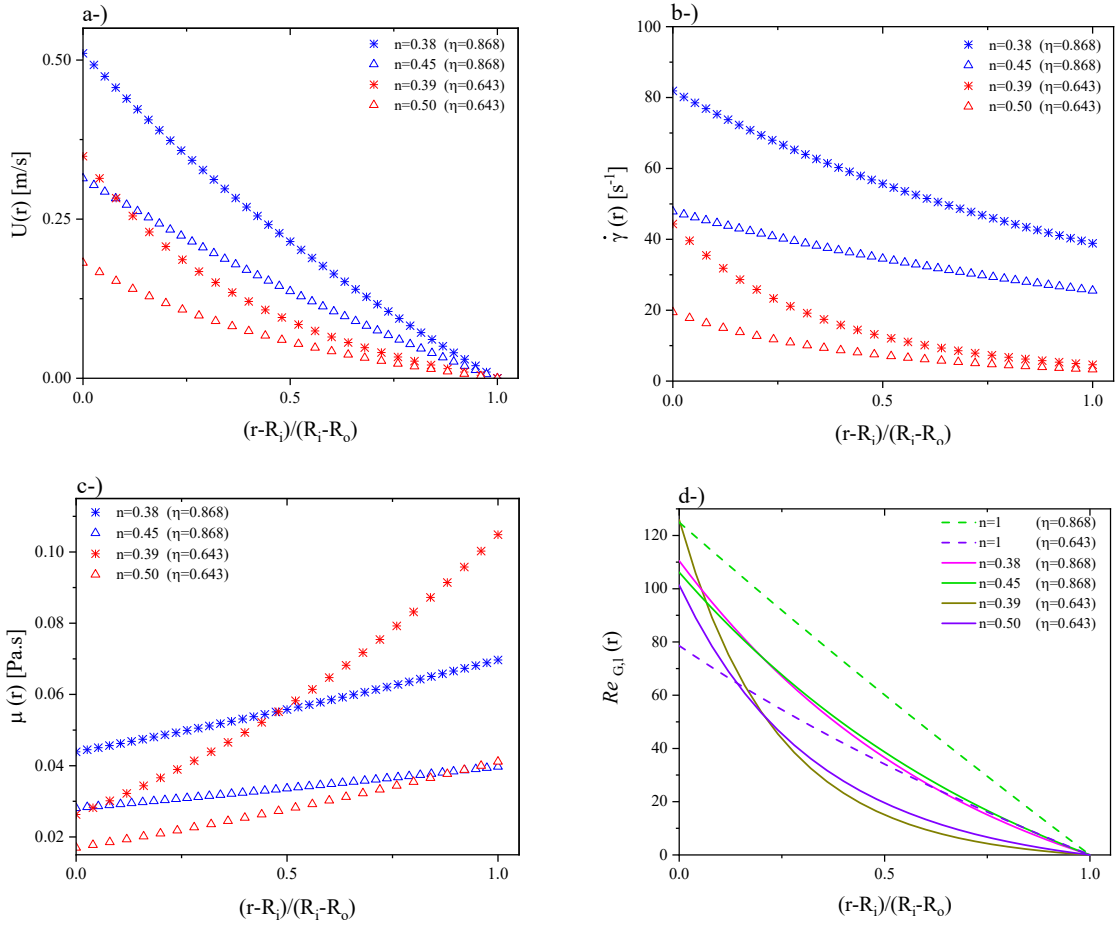
Şekil 3. 5 Hız, kayma hızı, viskozite ve Re_{G,l} profilleri, TVF kritik geçiş değerine karşılık gelen silindirler arasındaki mesafe boyutsuz tanımlanmıştır.
