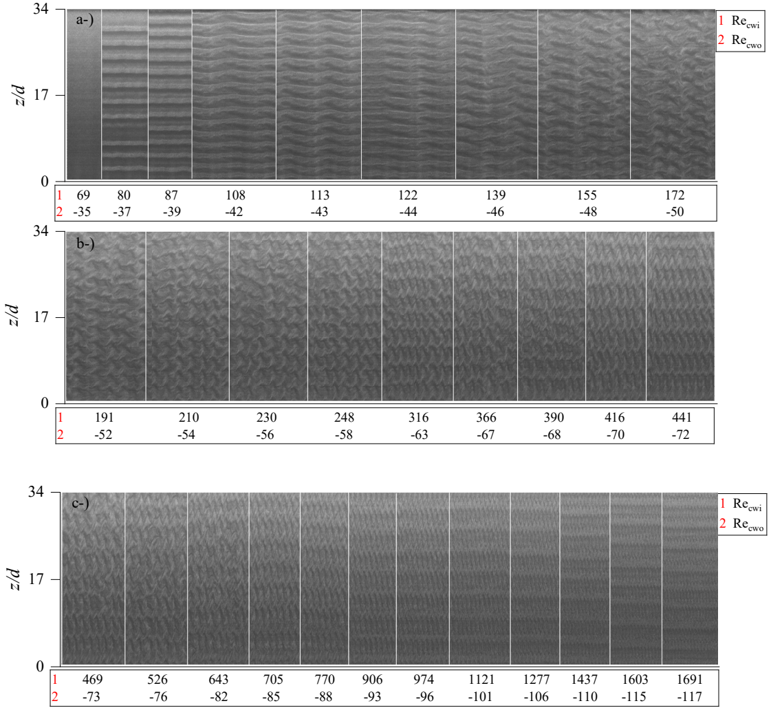
Şekil 4. 29 Farklı Re_{cw} değerlerinde %0,1 xanthan çözeltisi için uzay-zaman grafiği (zıt yön).
