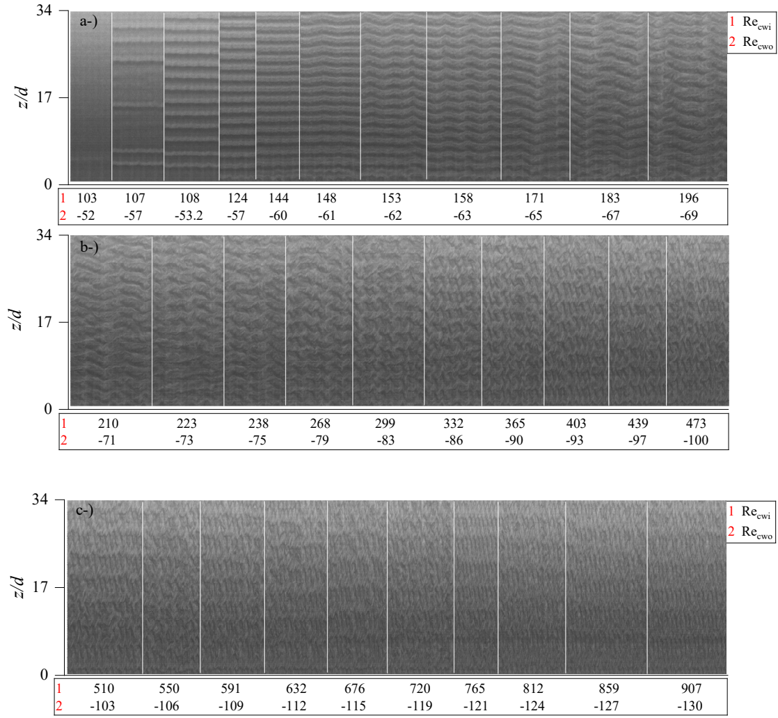
Şekil 4. 28 Farklı Re_{cw} değerlerinde %0,2 xanthan çözeltisi için uzay-zaman grafiği (zıt yön).
