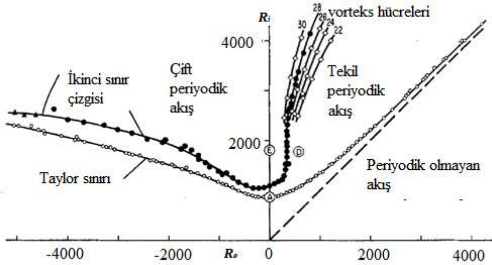
Şekil 1.6 Dairesel Couette akışının rejim geçiş sınırları [5].
