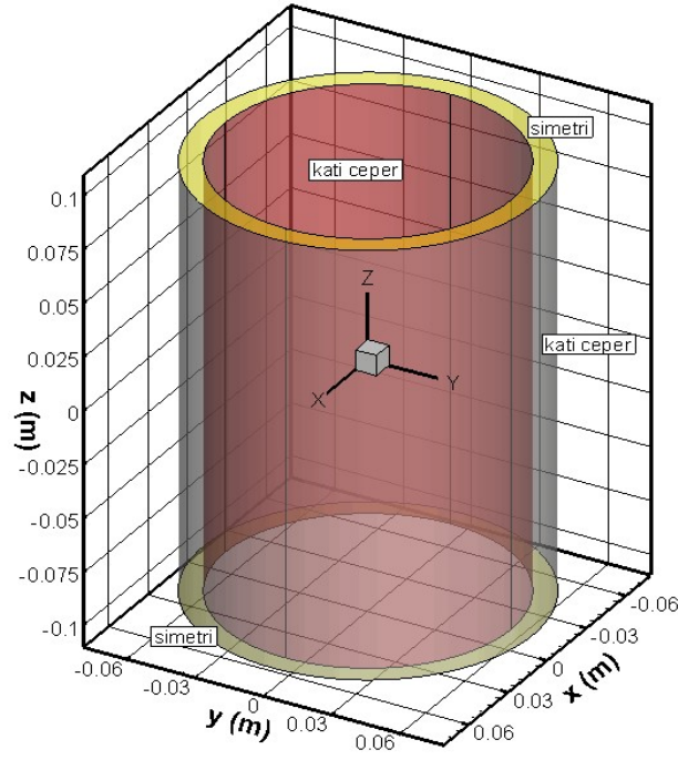
Şekil 7. 4 Çalışma bölgesi ve sınır şartları.
