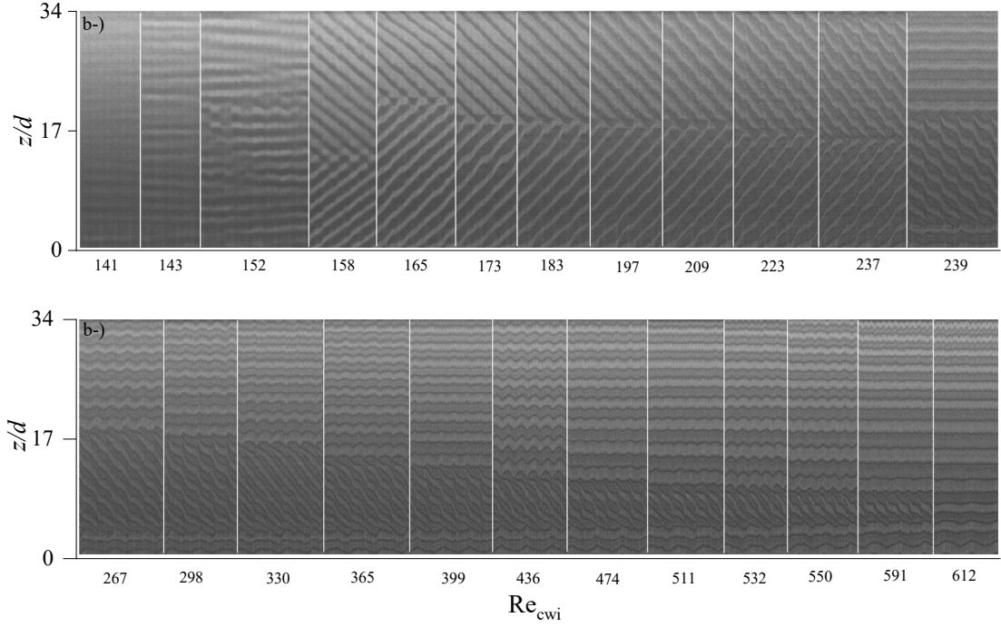
Şekil 8. 10 Xanthan çözeltisinin aynı yöne dönme koşullarında oluşan akış yapıları (a) n=0,45 ve (b) n=0,33 ( \eta=0,868 ).
