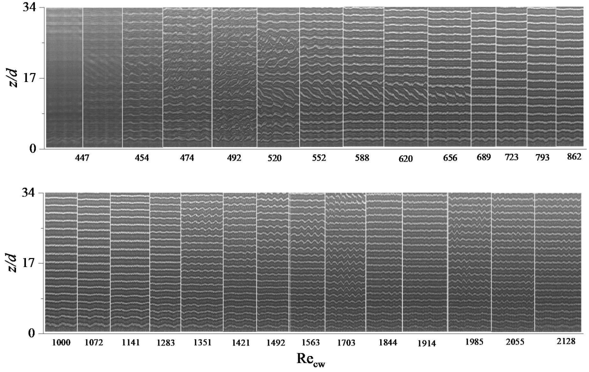
Şekil 4. 7 Farklı Re_{cw} değerlerinde gliserin akışkanına ait uzay-zaman grafiği ( \omega_o=43,5\text{rpm} ).
