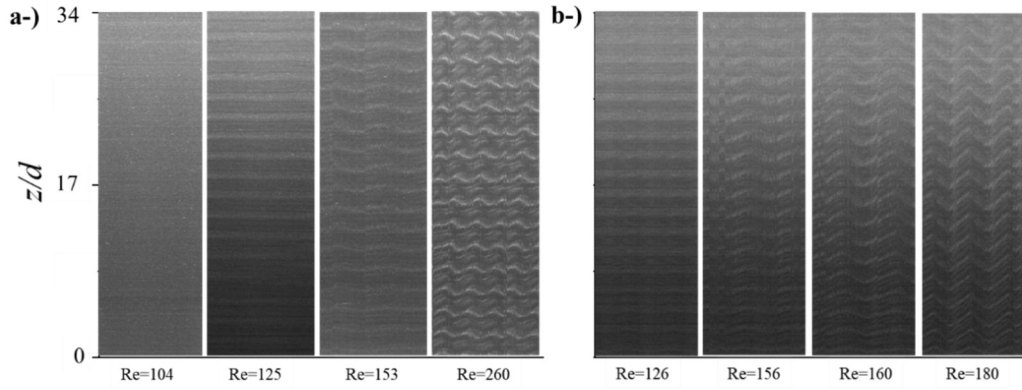
Şekil 8. 2 Farklı gliserin konsantrasyonlarda ortaya çıkan akış yapıları a-) %60 b-) %75.
