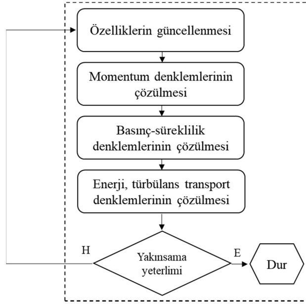
Şekil 7. 1 Segregated çözüm yöntem aşamalarının şematik gösterimi.
