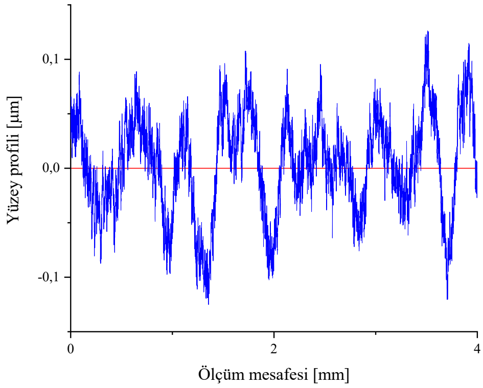
Şekil 2. 13 Normal yüzeyin profili.
