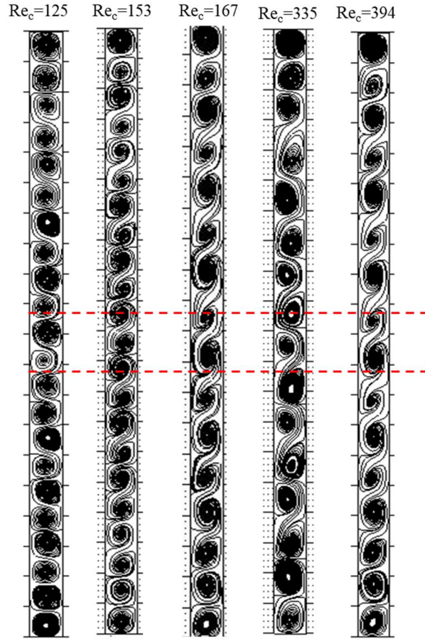
Şekil 7. 9 Gliserin akışkanına ait akım çizgilerinin boşluktaki dağılımı.
