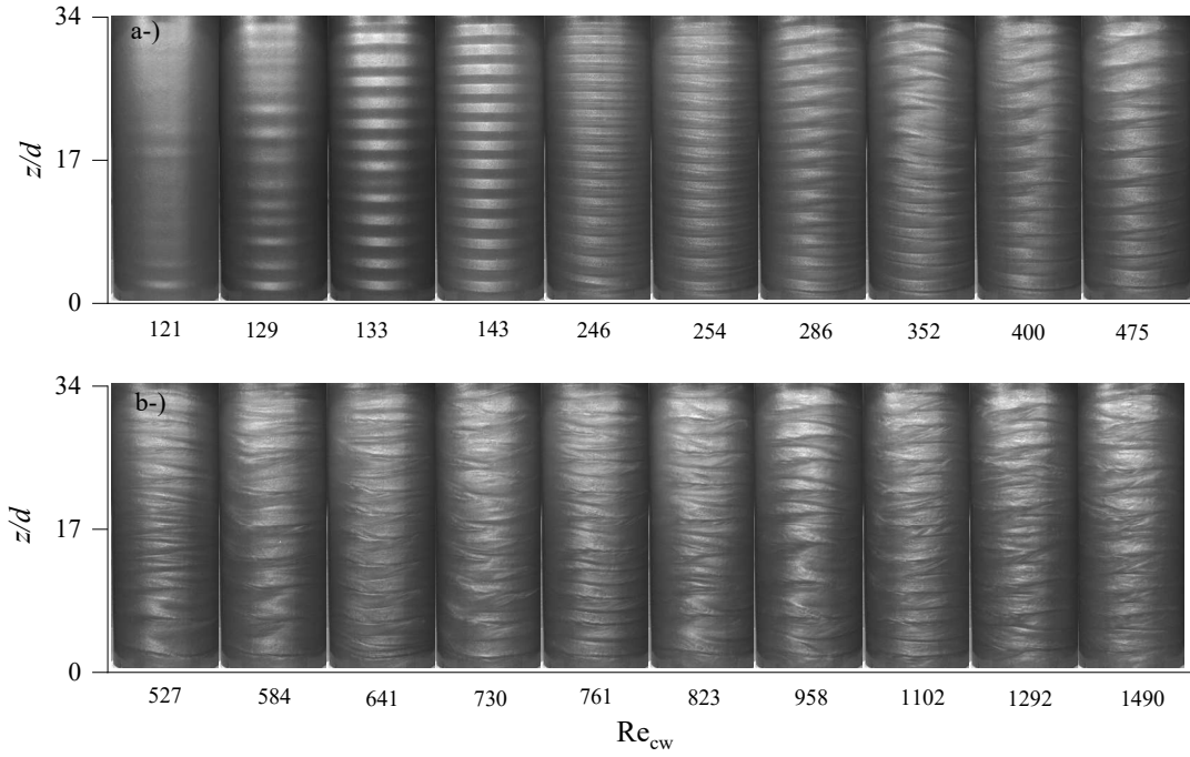
Şekil 5. 8 Farklı Re_{cw} değerlerinde %0,2 xanthan çözeltisi için akış yapılarının anlık görüntüleri.
