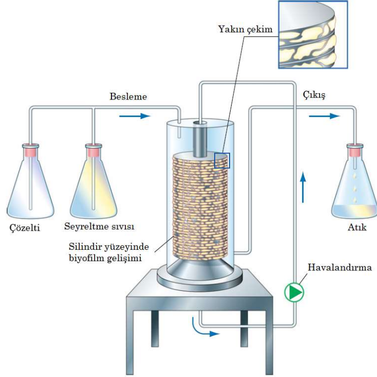
Şekil 1.10 Biyofilm ayrıştırılmasında kullanılan TC reaktörü [72].
