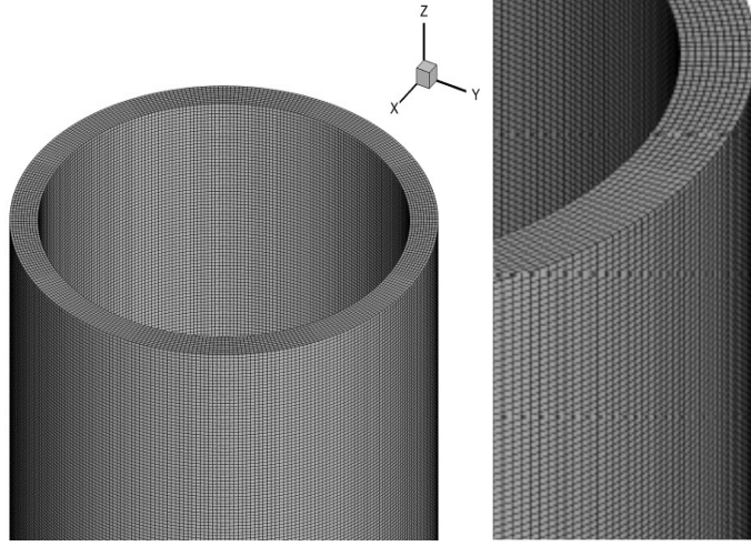
Şekil 7. 6 Nümerik alışmalarda kullanılan ağ yapısının görünümü.
