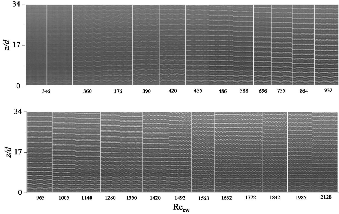
Şekil 4. 6 Farklı Re_{cw} değerlerinde gliserin akışkanına ait uzay-zaman grafiği ( \omega_o=33\text{rpm} ).
