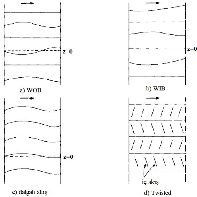
Şekil 4. 1 Iooss (1986) tarafından yapılan çalışmada incelenen akış yapılarının şematik görünümü [123].
