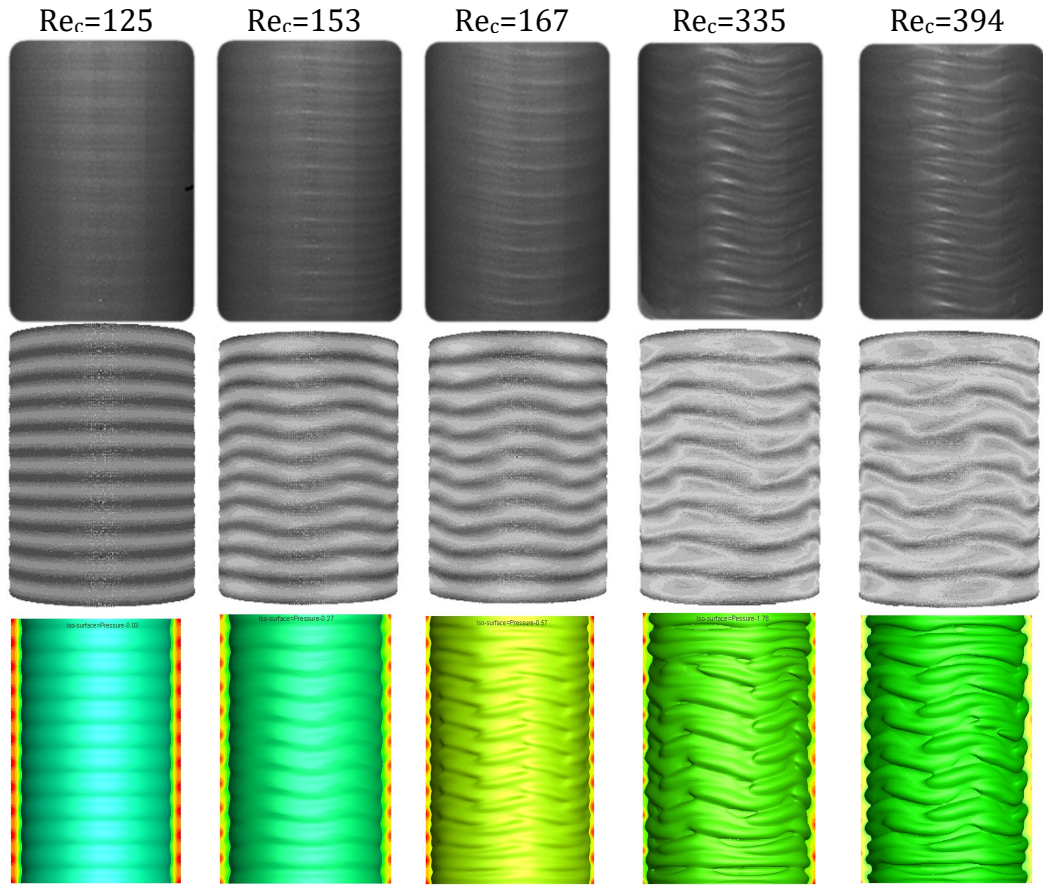
Şekil 7. 8 Gliserin çözeltisinin akış yapılarının deneysel, nümerik akış yapıları ve eş basınç çizgileri.
