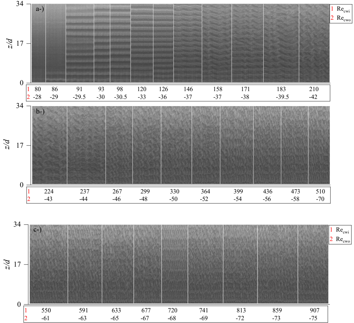
Şekil 4. 26 Farklı Re_{cw} değerlerinde %0,2 xanthan çözeltisi için uzay-zaman grafiği (zıt yön).
