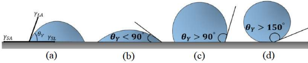
Şekil 5. 2 (a) Temas açısının şematik olarak görünümü, (b) hidrofilik, (c) hidrofobik, (d) süperhidrofobik yüzey.
