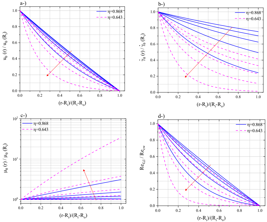
Şekil 3. 2 İki farklı yarıçap oranında n = 1, 0,8, 0,6, 0,4, 0,2 için normleştirilmiş hız, kayma hızı, viskozite ve Re_{G,l} profillerinin karşılaştırılması. Kırmızı ok n ’nin azalan değerlerini göstermektedir.
