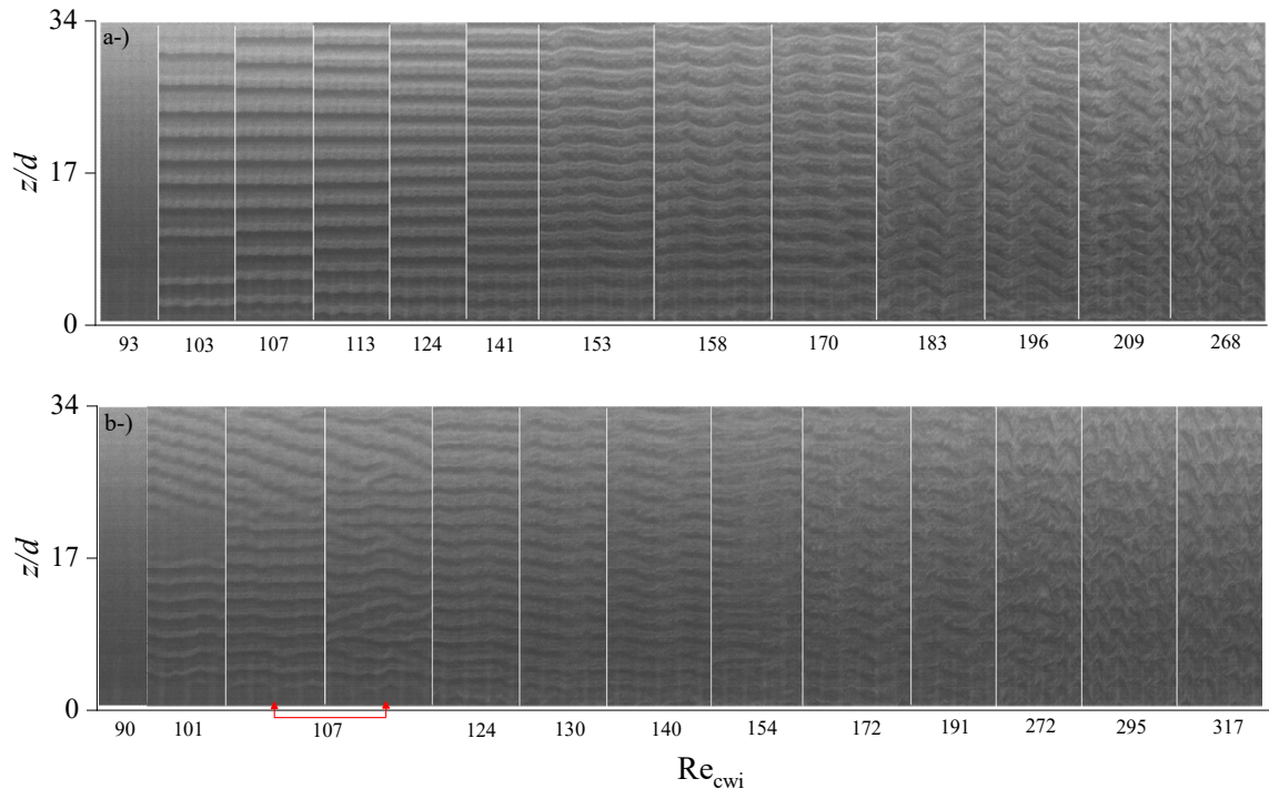
Şekil 8. 12 Xanthan çözeltisinin zıt yöne dönme koşullarında oluşan akış yapıları (a) n=0,33 ve (b) n=0,45 ( \eta=0.868 ).
