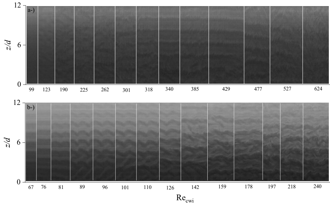
Şekil 8. 11 Xanthan çözeltisinin zıt yöne dönme koşullarında oluşan akış yapıları (a) n=0,50 and (b) n=0,39 ( \eta=0,643 ).
