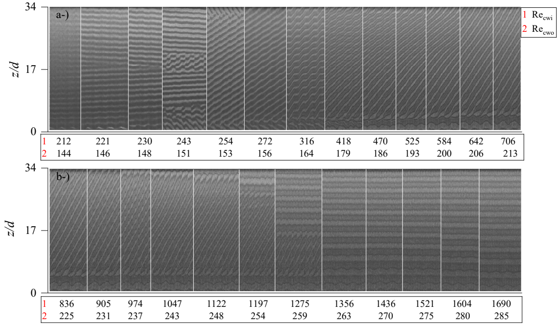
Şekil 4. 23 Farklı Re_{cw} değerlerinde %0,1 xanthan çözeltisi için uzay-zaman grafiği.
