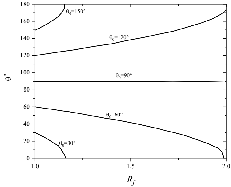
Şekil 5. 4 Temas açısının yüzey pürüzlülük ve görünen temas açısına bağlı olarak değişimi [166].
