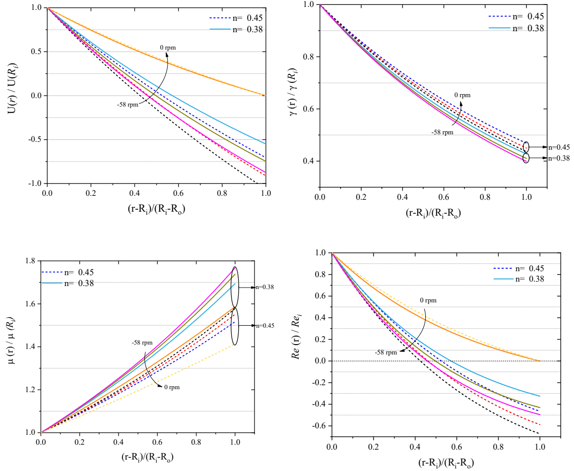
Şekil 4. 24 Silindirler arasındaki boşlukta zıt yöne dönme sonucunda hız, kayma hızı, viskozite ve Re_{G,l} değişimleri.
