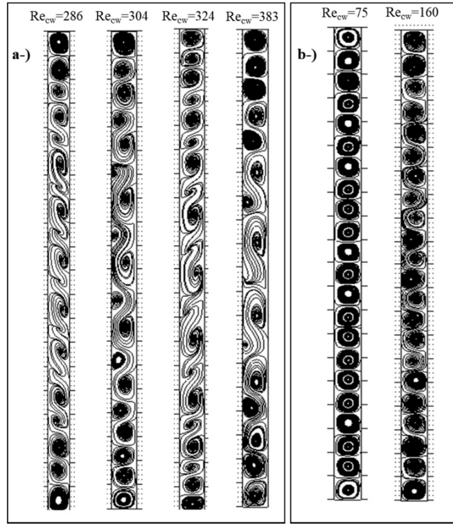
Şekil 7. 15 a-) %0,01 ve b-) %0,02 carbopol çözeltisine ait akım çizgilerinin boşluktaki dağılımı.
