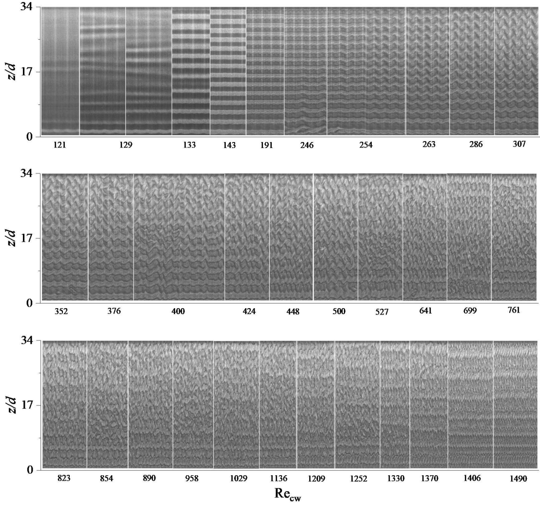
Şekil 5. 9 Farklı Re_{cw} değerlerinde %0,2 xanthan çözeltisi için uzay-zaman grafiği.
