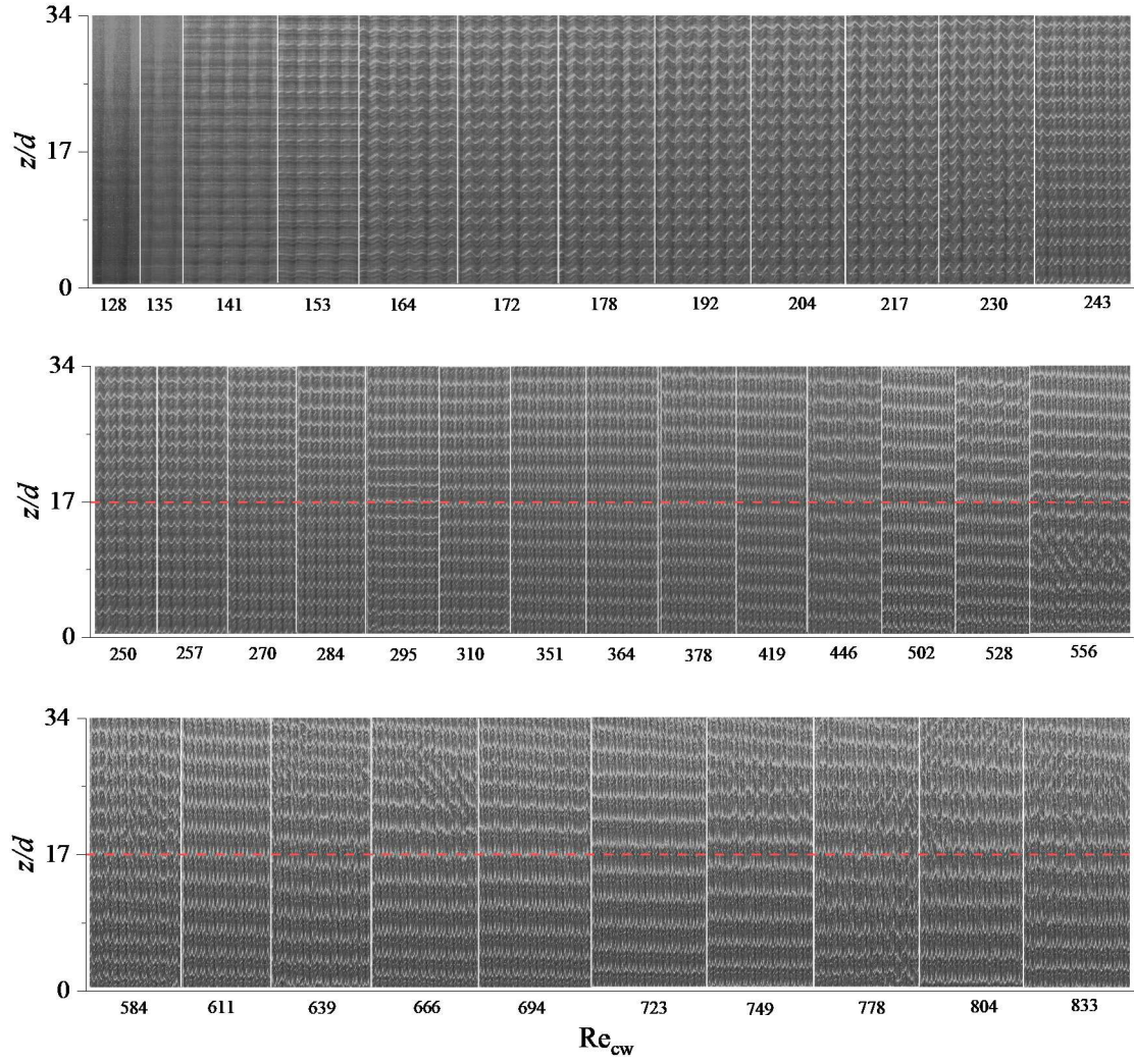
Şekil 5. 6 Farklı Re_{cw} değerlerinde %75 gliserin çözeltisi için uzay-zaman grafiği.
