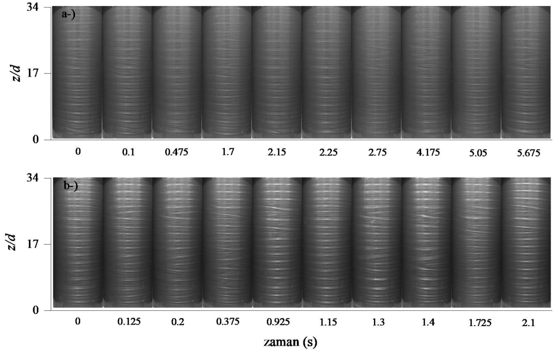
Şekil 4. 5 Zamana bağlı olarak gliserin akışkanının anlık görüntülerin değişimi a-) Re_{cwi}=390 , Re_{cwo}=283 b-) Re_{cwi}=520 , Re_{cwo}=373 .
