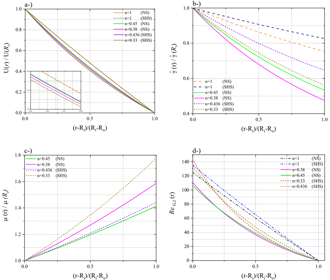
Şekil 5. 7 Hız, kayma-hızı viskozite ve lokal Reynolds profilinin boyutsuz olarak değişimi.
