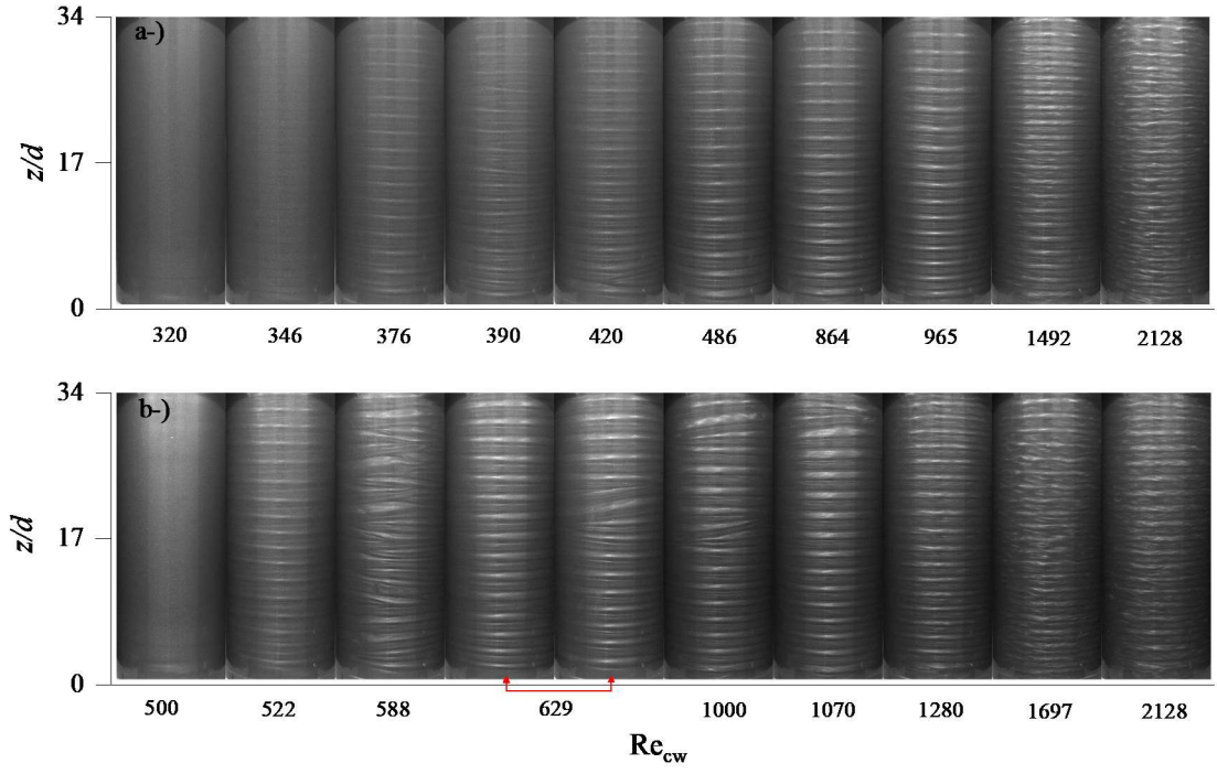
Şekil 4. 4 Farklı Re_{cw} değerlerinde gliserin akışkanına ait akış yapılarının anlık görüntüleri.
