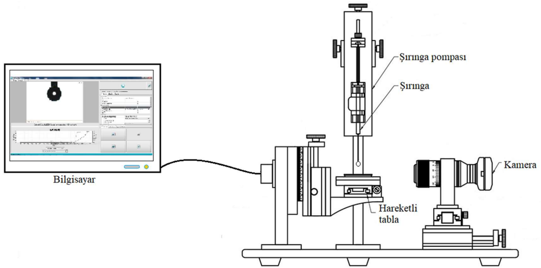
Şekil 2. 3 Temas açısı ölçüm cihazının şematik gösterimi.
