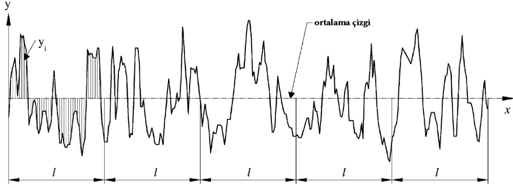
Şekil 2. 11 Aritmetik ortalama yükseklik (Ra) [95].
