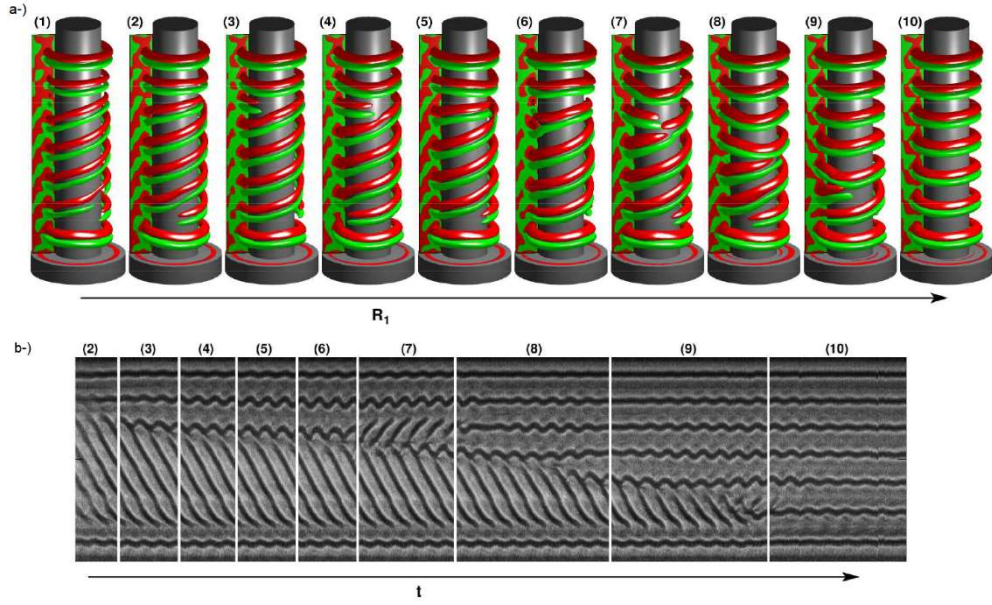
Şekil 1.8 wSVF akışından TVF akışına geçiş a) simülasyon b) deneysel sonuçlar [40].
