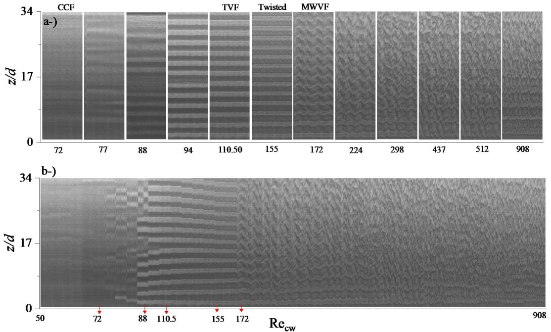
Şekil 3. 9 Farklı Re_{cw} değerlerinde %0,2 xanthan çözeltisi için uzay-zaman grafiği.
