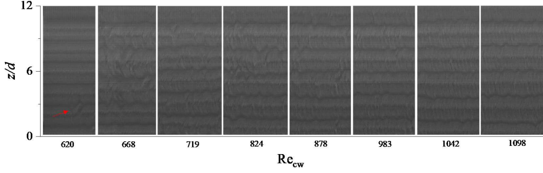
Şekil 3. 11 Farklı Re_{cw} değerlerinde %0,2 xanthan çözeltisi için uzay-zaman grafiği ( \eta=0,643 ).
