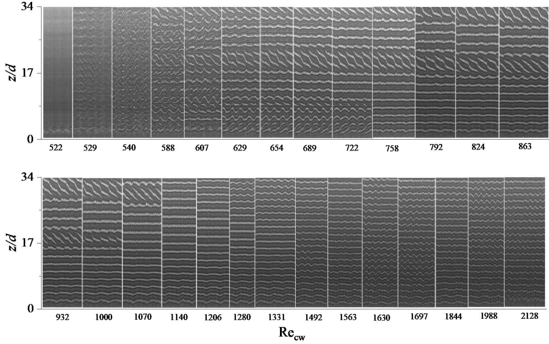
Şekil 4. 9 Farklı Re_{cw} değerlerinde gliserin akışkanına ait uzay-zaman grafiği ( \omega_o=53\text{rpm} ).
