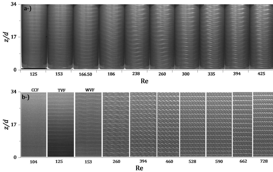
Şekil 3. 3 %75 gliserin çözeltisine ait akış yapılarının a) anlık ve b)uzay zaman grafikleri ile gösterimi.
