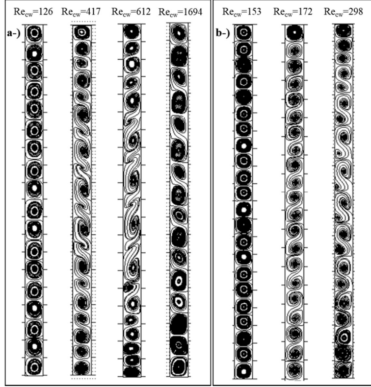
Şekil 7. 12 a-) %0,1 ve b-) %0,2 XG çözeltisine ait akım çizgilerinin boşluktaki dağılımı.
