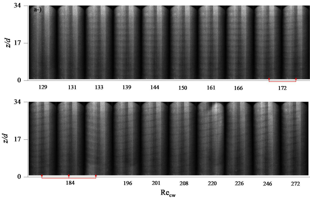
Şekil 6. 3 Farklı Re_{cw} değerlerinde %0,01 carbopol çözeltisine ait anlık görüntüler.
