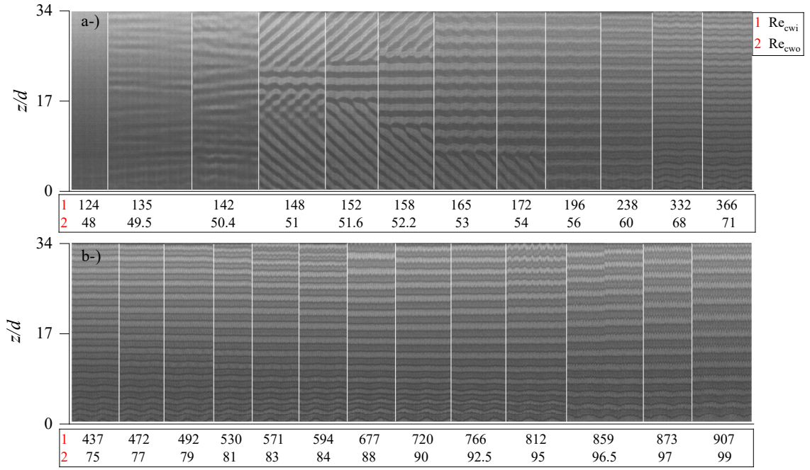
Şekil 4. 19 Farklı Re_{cw} değerlerinde %0,2 xanthan çözeltisi için uzay-zaman grafiği.
