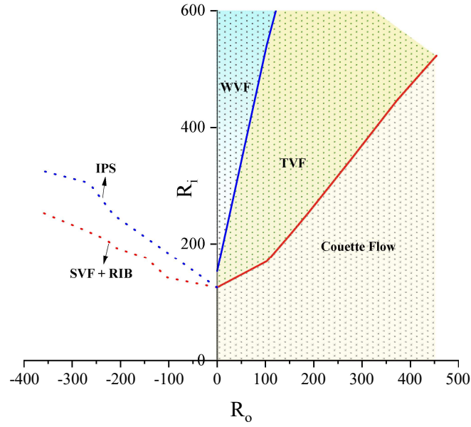
Şekil 8. 7 TC-UV reaktöründe ortaya çıkan akış yapılarının kritik sınır değerleri ( \eta=0,868 ).
