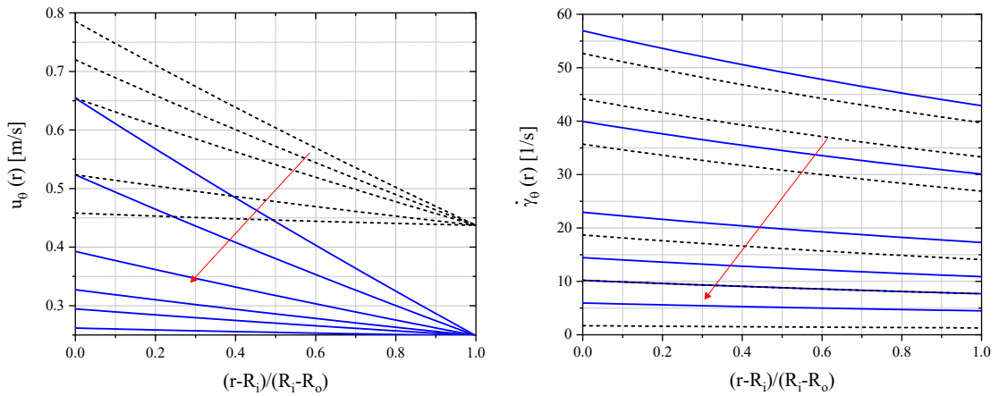
Şekil 4. 3 Hız ve kayma hızının iç silindirin dönme hızına bağlı olarak değişimi (kırmızı ok dış silindirin dönme hızının azalma yönünü göstermektedir).
