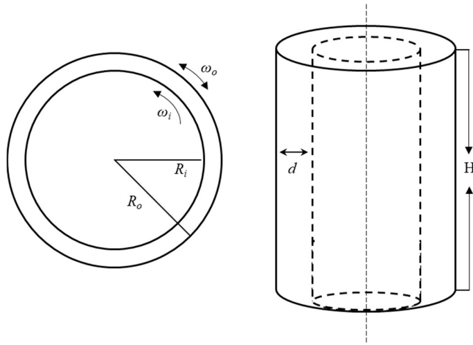
Şekil 1.1 Klasik TC düzeneği.
