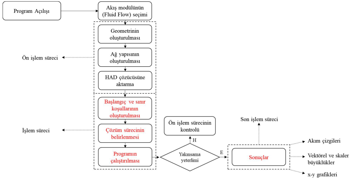
Şekil 7. 2 ANSYS CFX için genel çözüm sürecinin akış şeması.
