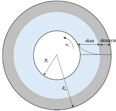
Şekil 6.2 TC deney düzeneği içerisindeki akan ve akmayan bölgelerin şematik gösterimi.
