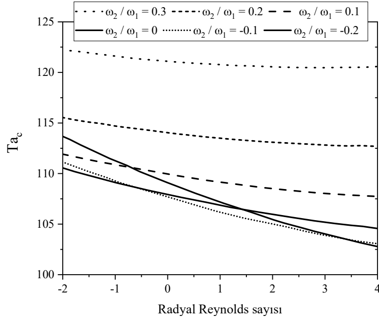
Şekil 4. 32 Radyal Reynolds sayısı ve silindirlerin dönme oranının ( \omega_2/\omega_1 ) kritik Taylor sayısı üzerindeki etkisi [140].
