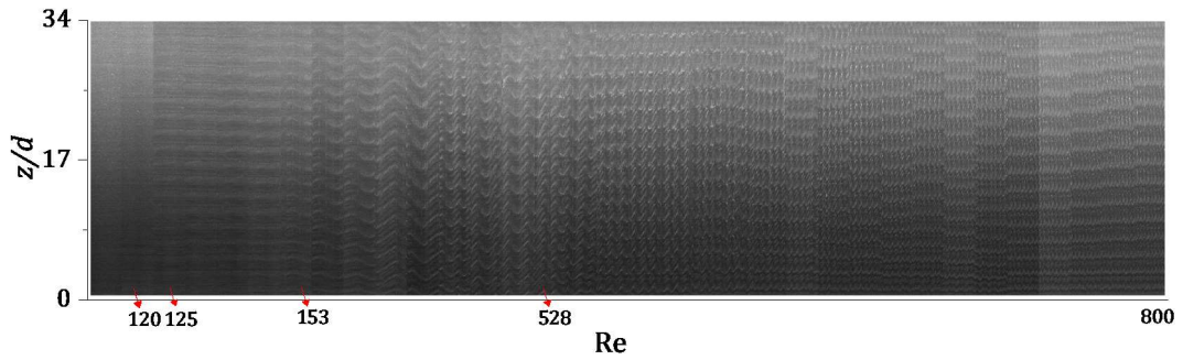
Şekil 3. 4 %75 gliserin çözeltisinin TC deney düzeneği içerisindeki akış yapılarının iç silindirin dönme hızına bağlı olarak dönüşümü.
