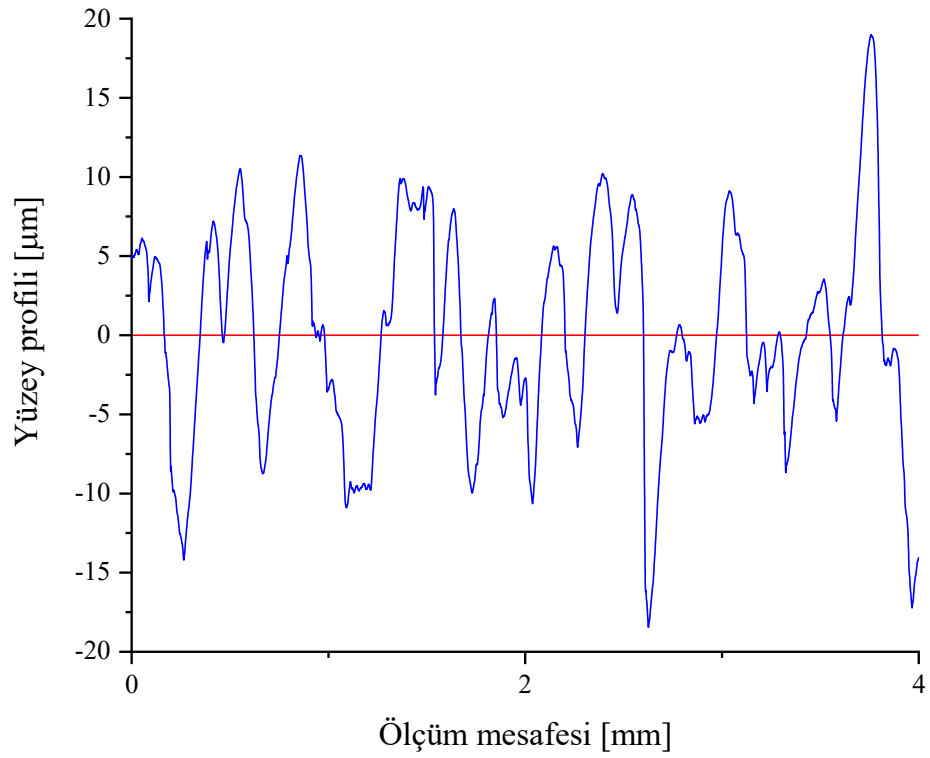
Şekil 2. 14 Hidrofobik yüzeyin profili.
