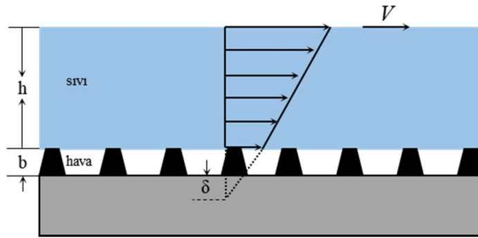
Şekil 2. 7 Couette akışının süperhidrofobik yüzey üzerindeki temsili.
