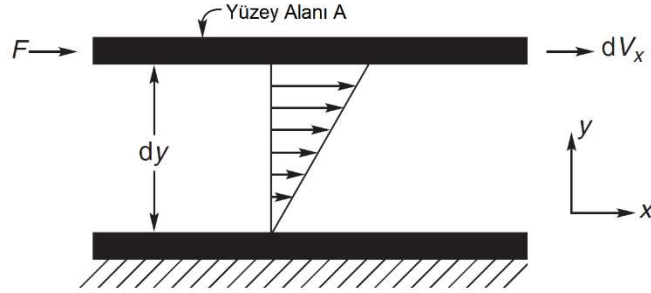
Şekil 1.5 Tek yönlü kayma akışının şematik gösterimi.
