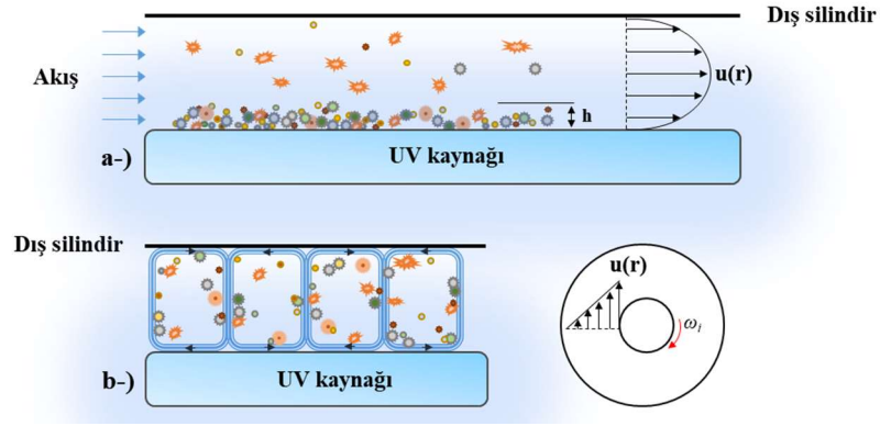
Şekil 8. 5 İstenmeyen türlerin taşınımının şematik gösterimi a-) C.UV b-) TC-UV.
