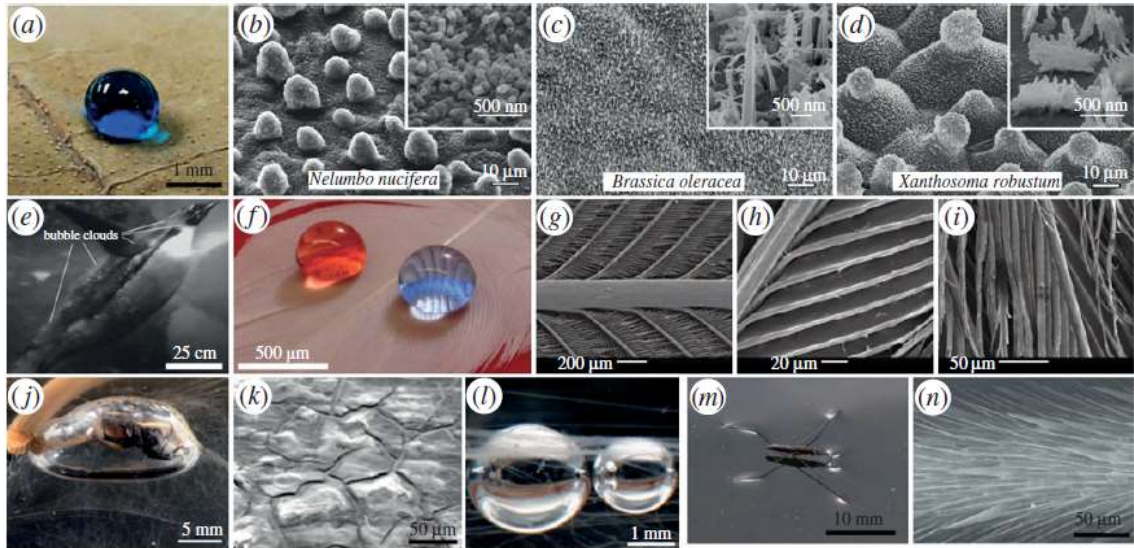
Şekil 5. 3 Doğada bulunan bazı süperhidrofobik yüzeyler.
