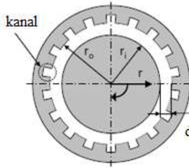
Şekil 1.7 Dış silindir üzerinde açılan kanallar [23].
