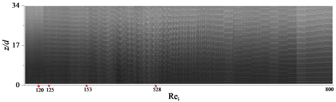
řekil 8. 8 Gliserin zeltisinin farklı Reynolds sayılarındaki uzay zaman grafięi.
