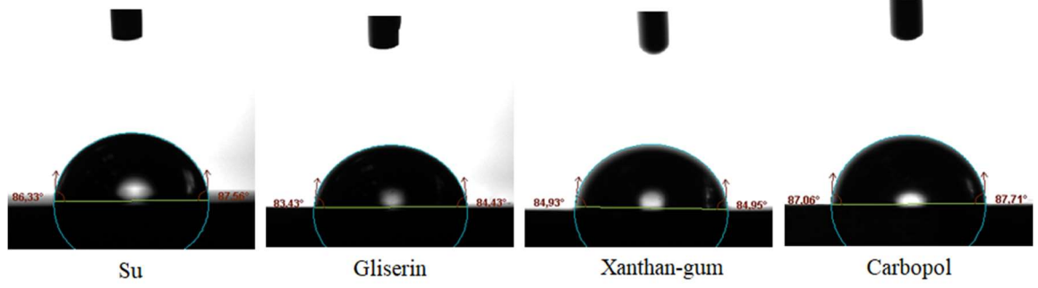
Şekil 2. 5 Normal yüzey ile akışkan temas açıları.
