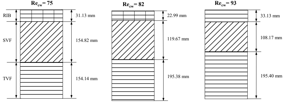
Şekil 3. 8 %0,1 xanthan çözeltisi için CCF ile TVF geçişi sırasında görülen akış yapılarının şematik görünüşü.
