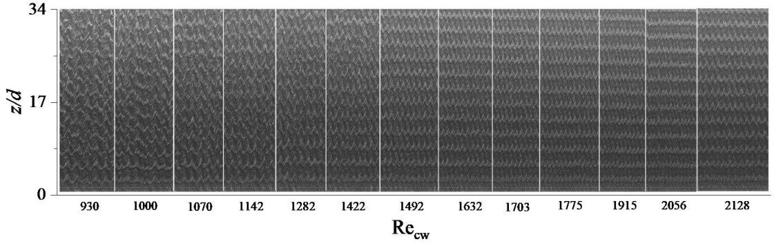
Şekil 4. 12 Farklı Re_{cw} değerlerinde gliserin akışkanına ait uzay-zaman grafiği ( \omega_o=-27 rpm).
