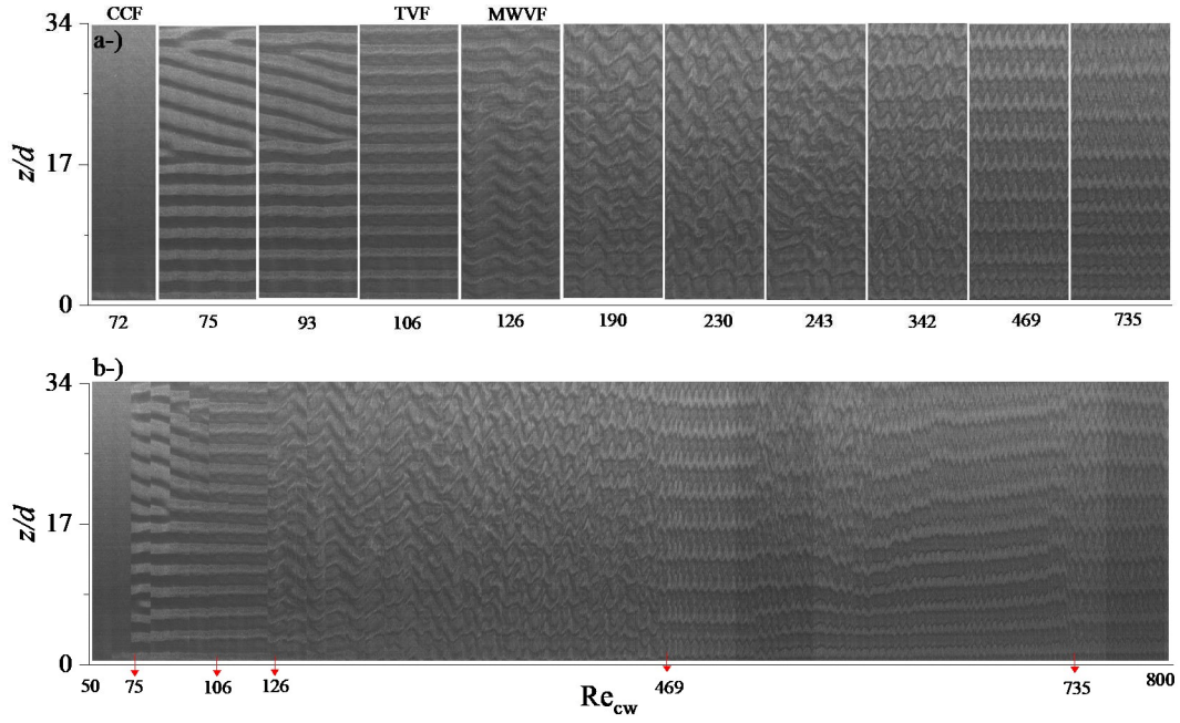
Şekil 3. 7 Farklı Re_{cw} değerlerinde %0,1 xanthan çözeltisi için uzay-zaman grafiği.
