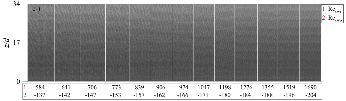
Şekil 4. 31 Farklı Re_{cw} değerlerinde %0,1 xanthan çözeltisi için uzay-zaman grafiği (zıt yön).
