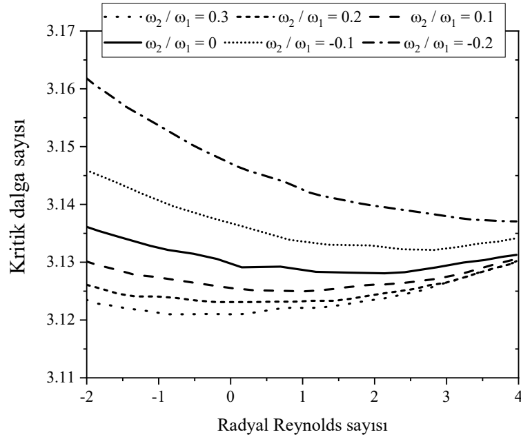
Şekil 4. 33 Radyal Reynolds sayısı ve silindirlerin dönme oranının ( \omega_2/\omega_1 ) kritik dalga sayısı üzerindeki etkisi [140].
