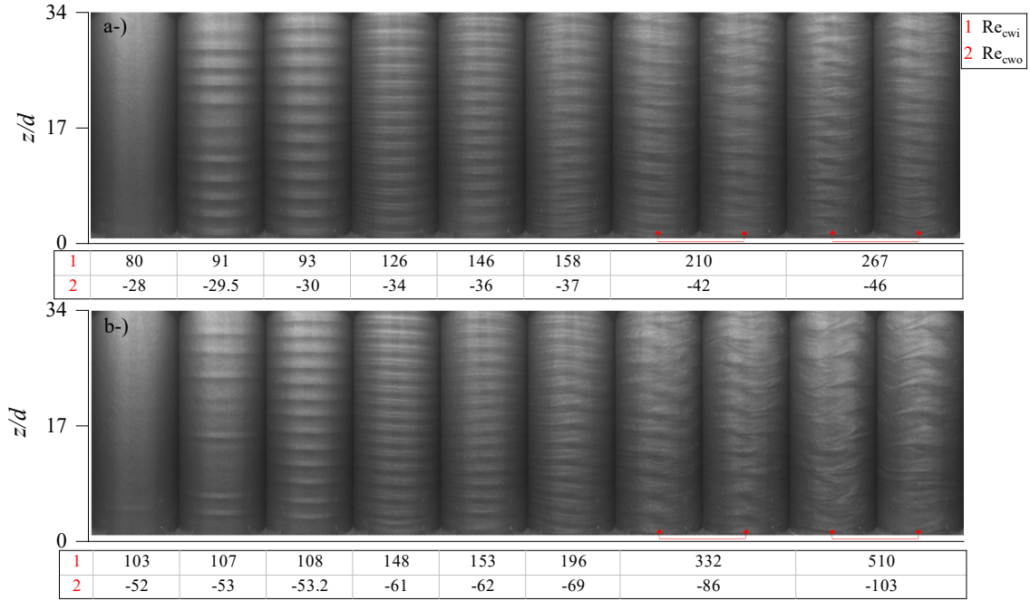
Şekil 4. 25 Farklı Re_{cw} değerlerinde %0,2 xanthan çözeltisi için akış yapılarının anlık görüntüleri (zıt yön).
