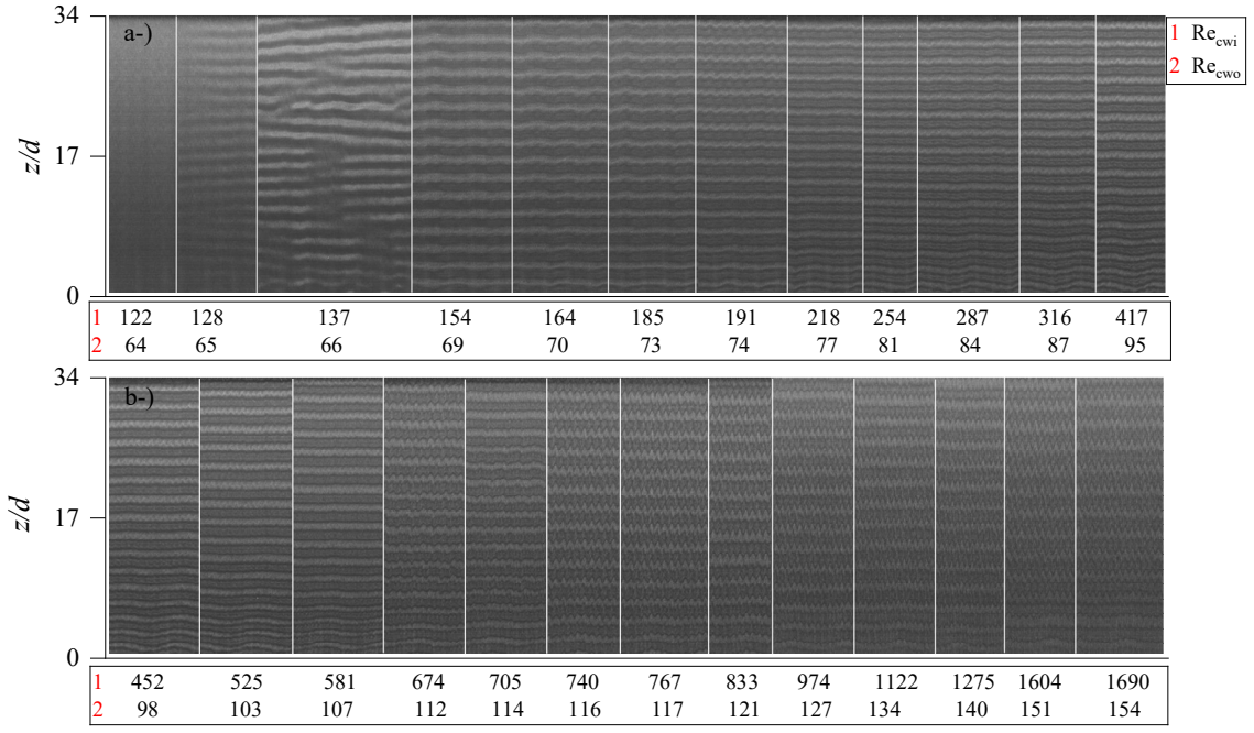
Şekil 4. 21 Farklı Re_{cw} değerlerinde %0,1 xanthan çözeltisi için uzay-zaman grafiği.
