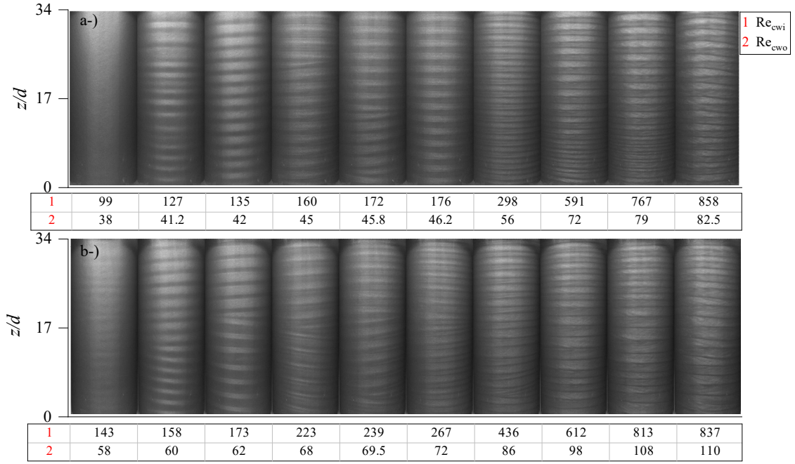
Şekil 4. 16 Farklı Re_{cw} değerlerinde %0,2 xanthan çözeltisi için akış yapılarının anlık görüntüleri.
