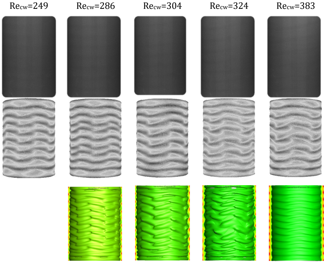
Şekil 7. 13 %0,01 carbopol çözeltisinin akış yapılarının deneysel, nümerik akış yapıları ve eş basınç çizgileri.
