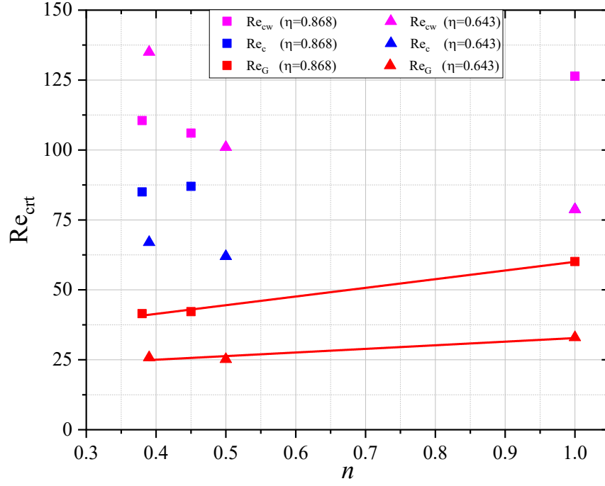
Şekil 3. 13 Farklı shear-thinning indeks ve yarıçap oranları için TVF akışına geçişi tanımlayan kritik Reynolds değerlerinin karşılaştırılması.
