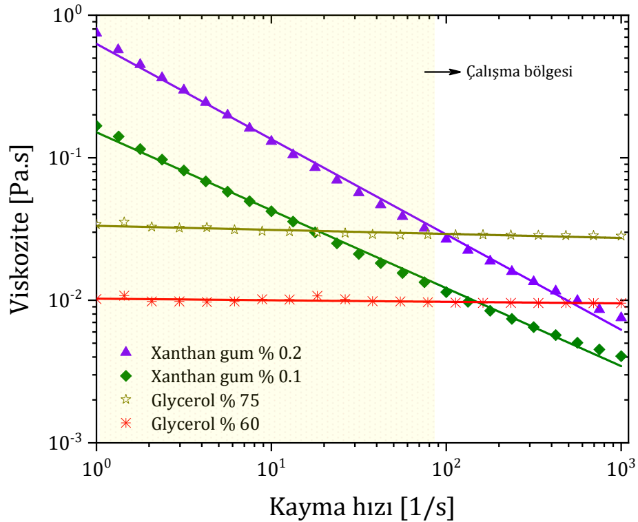
Şekil 3. 1 Deneyel çalışmalarda kullanılan akışkanlara ait reolojik özellikleri.
