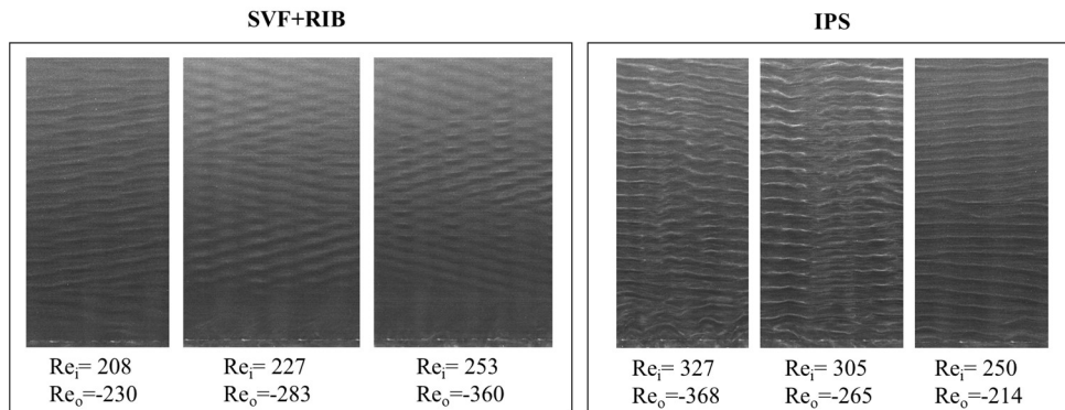
Şekil 8. 6 Zıt yöne dönme koşullarında ortaya çıkan akış yapıları.
