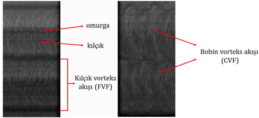
Şekil 3. 12 Yeni akış yapılarının büyütülmüş görüntüsü.
