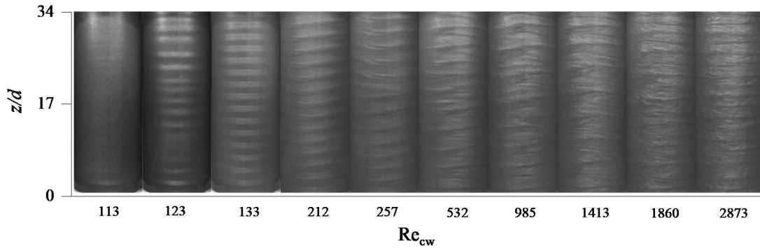
Şekil 5. 10 Farklı Re_{cw} değerlerinde %0,1 xanthan çözeltisi için akış yapılarının anlık görüntüleri.
