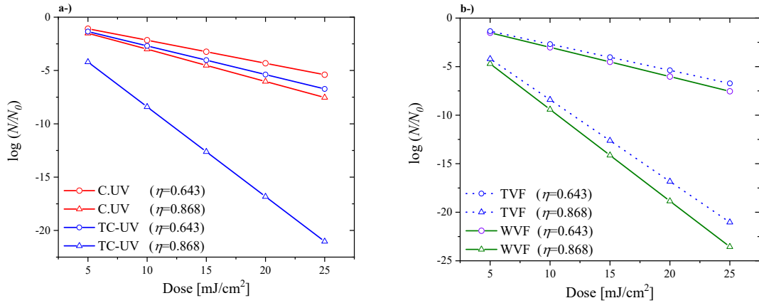
Şekil 8. 4 E. coli inaktivasyon verimliliği a-) C.UV ve TC-UV rektörleri b-) TC-UV reaktörü içerisindeki farklı akış yapıları.
