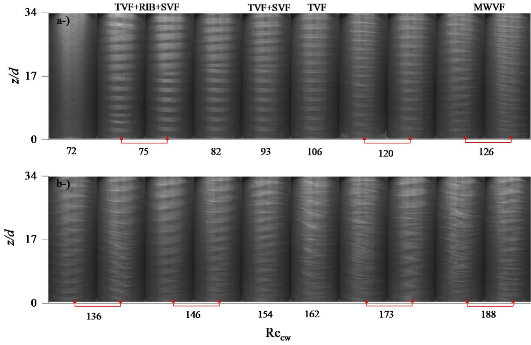
Şekil 3. 6 Farklı Re_{cw} değerlerinde %0,1 xanthan çözeltisi için akış yapılarının anlık görüntüleri.
