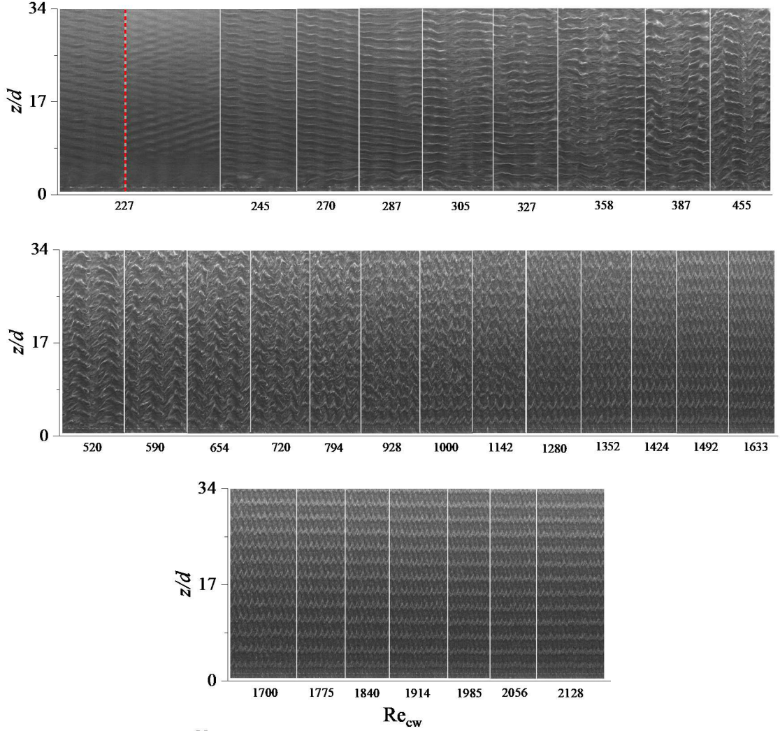
Şekil 4. 13 Farklı Re_{cw} değerlerinde gliserin akışkanına ait uzay-zaman grafiği ( \omega_o=-33rpm ).
