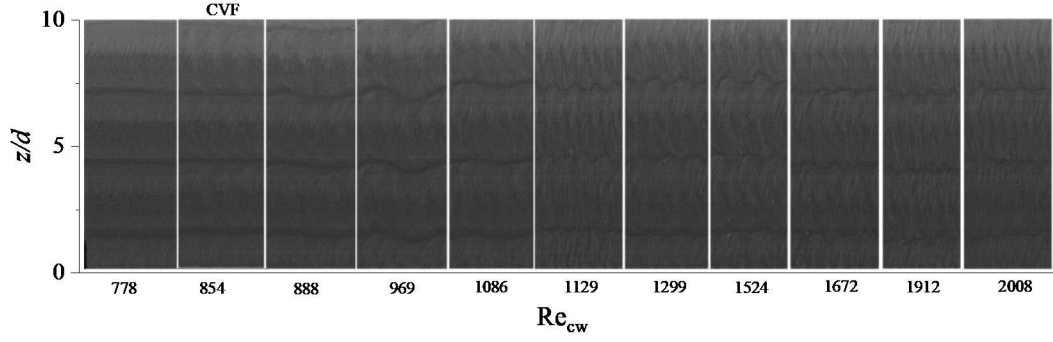
Şekil 3. 10 Farklı Re_{cw} değerlerinde %0,1 xanthan çözeltisi için uzay-zaman grafiği ( \eta=0,643 ).
