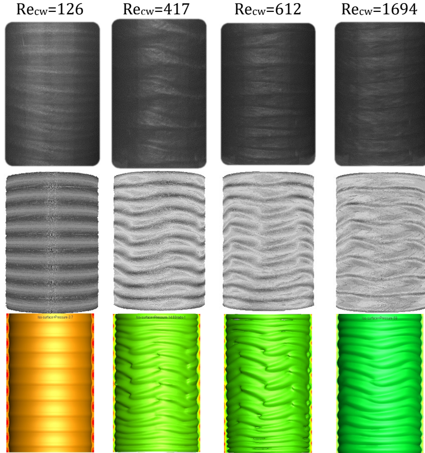
Şekil 7. 10 %0,1 XG çözeltisinin akış yapılarının deneysel, nümerik akış yapıları ve eş basınç çizgileri.
