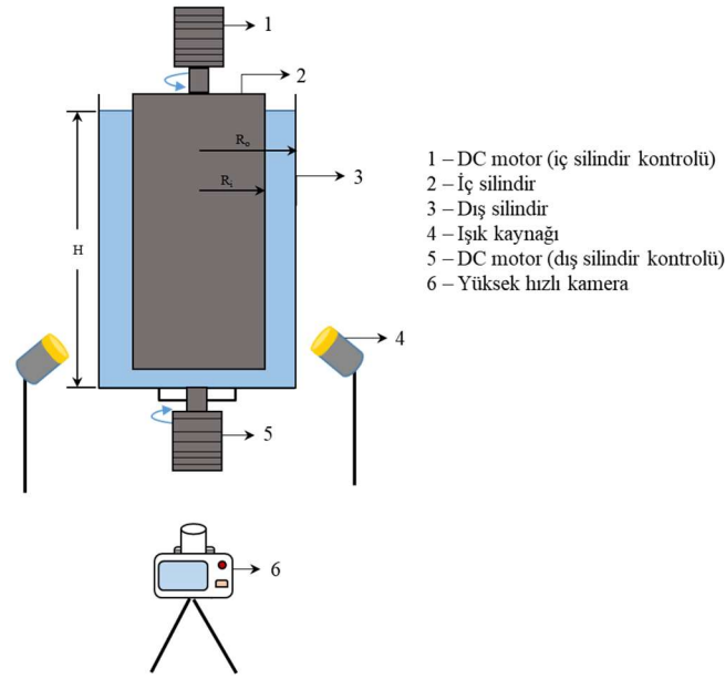
Şekil 8. 1 Deney düzeneğinin şematik gösterimi.
