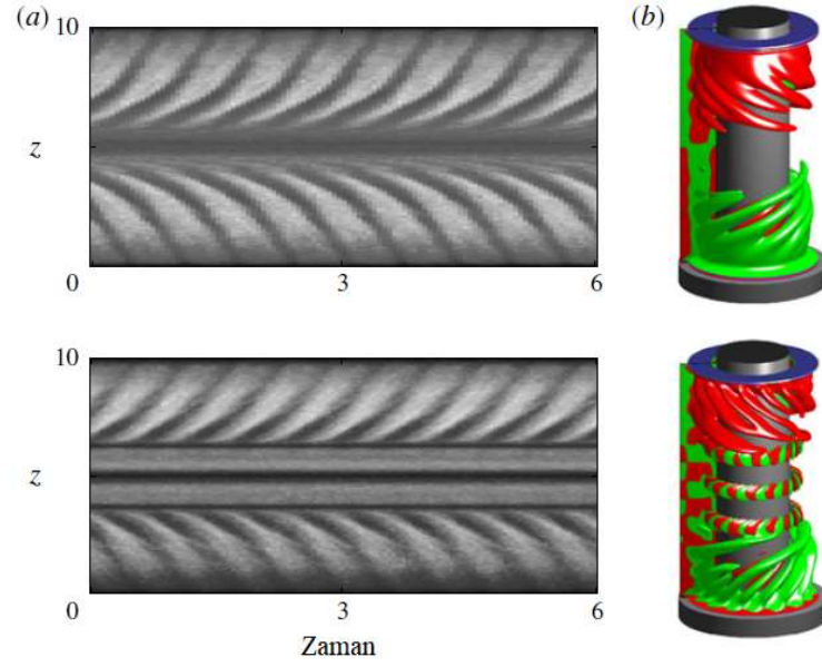
Şekil 4. 2 Heise ve ark. (2013) tarafından gözlemlenen akış yapılarının a) deneysel ve b) nümerik olarak görünümü [125].
