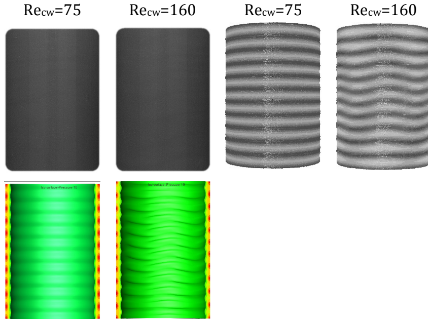
Şekil 7. 14 %0,02 carbopol çözeltisinin akış yapılarının deneysel, nümerik akış yapıları ve eş basınç çizgileri.
