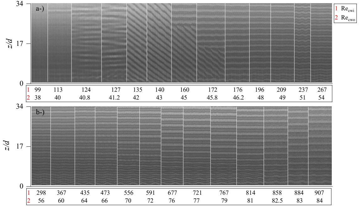
Şekil 4. 17 Farklı Re_{cw} değerlerinde %0,2 xanthan çözeltisi için uzay-zaman grafiği.
