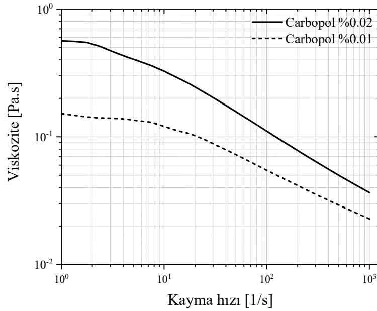
Şekil 6. 1 Deneysel çalışmalarda kullanılan carbopol akışkanının reolojik özellikleri.
