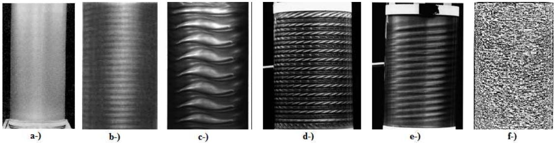
Şekil 1.2 Akış rejimlerinin görsel olarak görünümü a-) Couette akışı b-) TVF c-) WVF d-) bükümlü (twisted) vorteks e-) SVF f-) türbülans.
