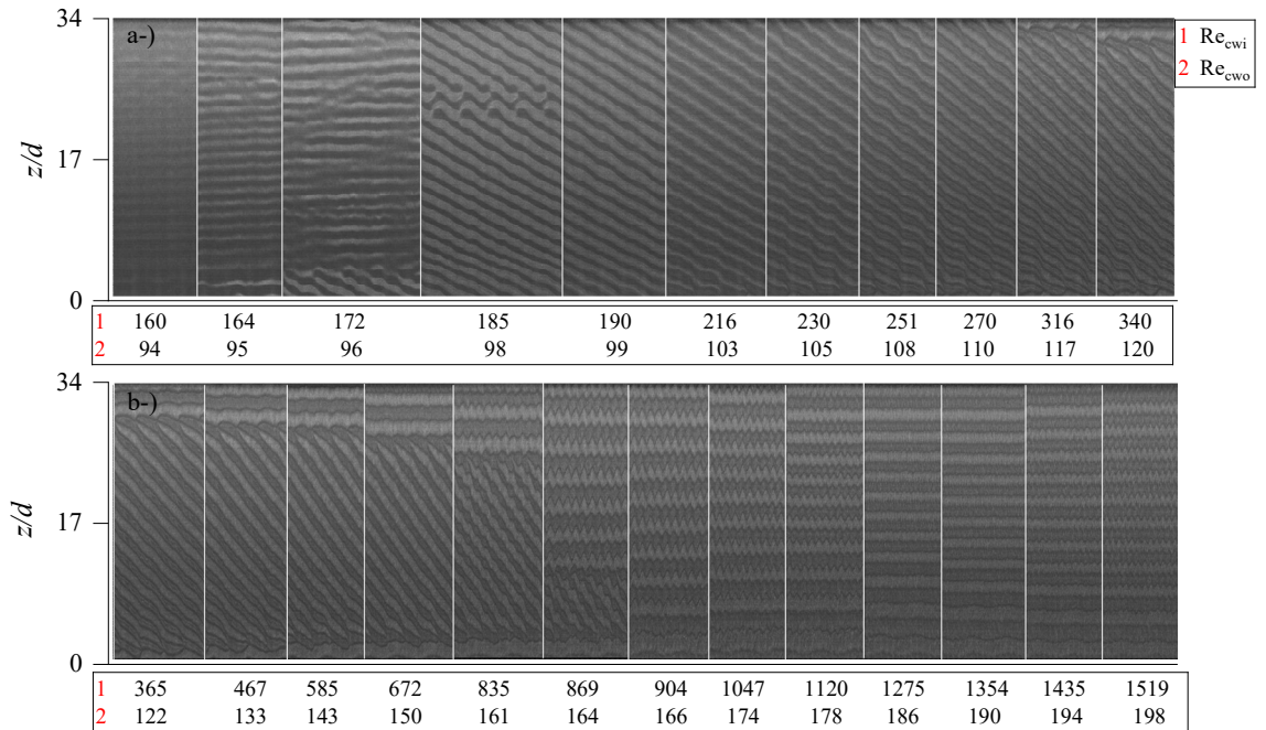
Şekil 4. 22 Farklı Re_{cw} değerlerinde %0,1 xanthan çözeltisi için uzay-zaman grafiği.
