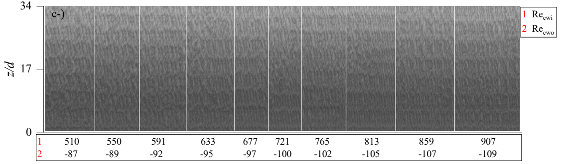
Şekil 4. 27 Farklı Re_{cw} değerlerinde %0,2 xanthan çözeltisi için uzay-zaman grafiği (zıt yön).
