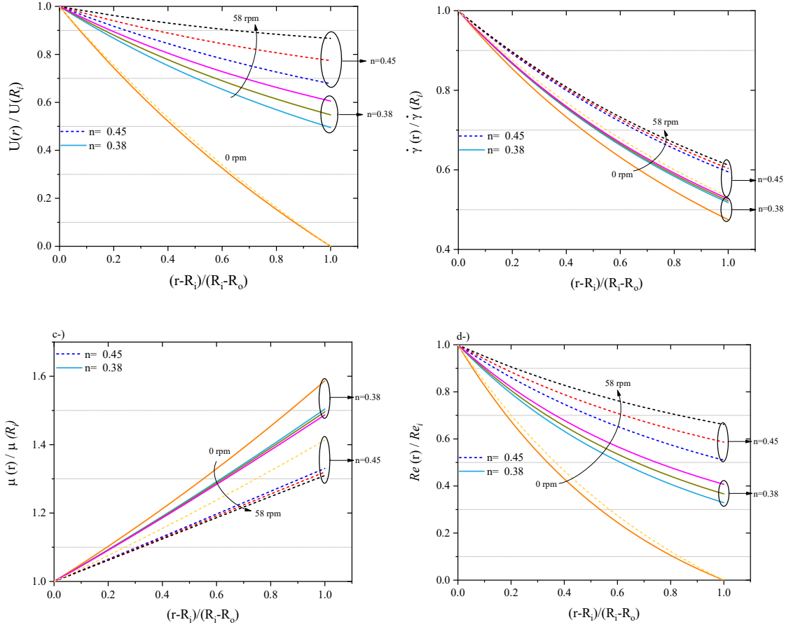
Şekil 4. 15 Hız, kayma hızı, viskozite ve Reynolds profilleri, normalize edilmiş grafikler.
