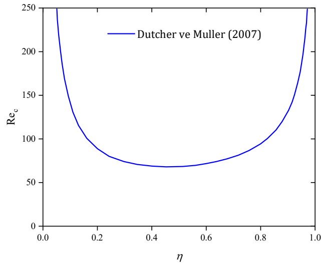
Şekil 1.4 Kritik Reynolds sayısının çap oranına bağlı olarak değişimi [8].
