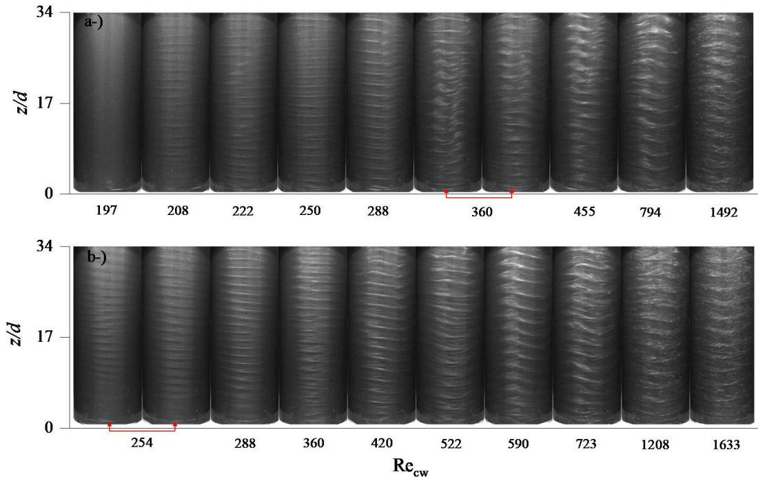
Şekil 4. 11 Farklı Re_{cw} değerlerinde %75 gliserin çözeltisi için akış yapılarının anlık görüntüleri.
