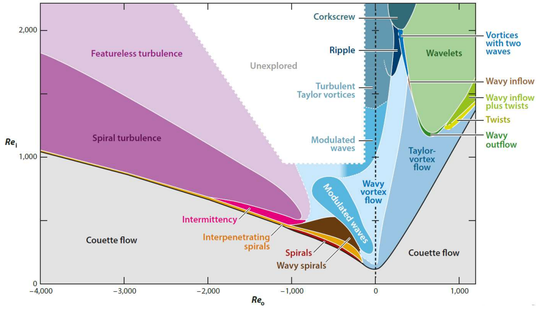
Şekil 1.3 Farklı Reynolds sayılarında tespit edilen akış yapıları ( \eta=0,883 ) [6].
