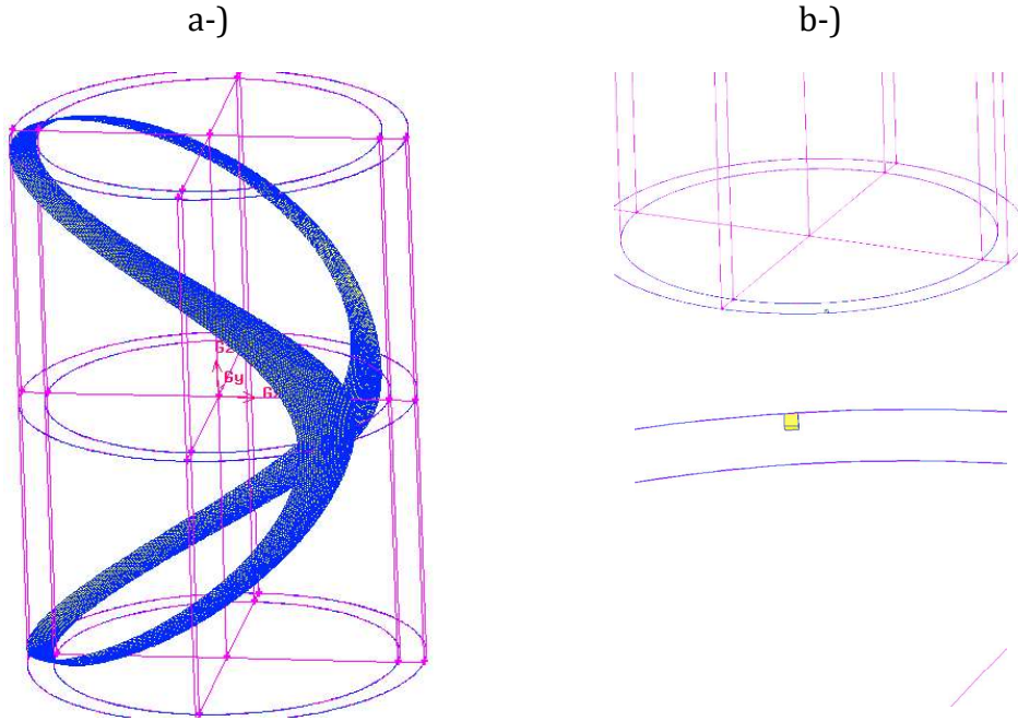
Şekil 7. 7 alışma bölgesindeki ağların büyüklükleri (a) ve en kötü ağ elemanının olduğu yer (b).
