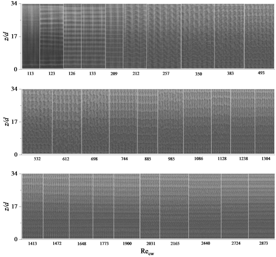
Şekil 5. 11 Farklı Re_{cw} değerlerinde %0,1 xanthan çözeltisi için uzay-zaman grafiği.
