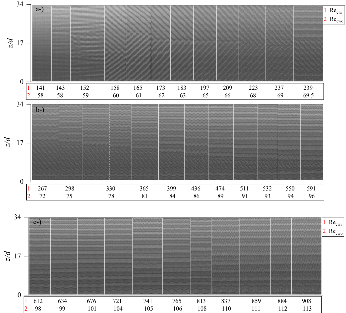
Şekil 4. 20 Farklı Re_{cw} değerlerinde %0,2 xanthan çözeltisi için uzay-zaman grafiği.
