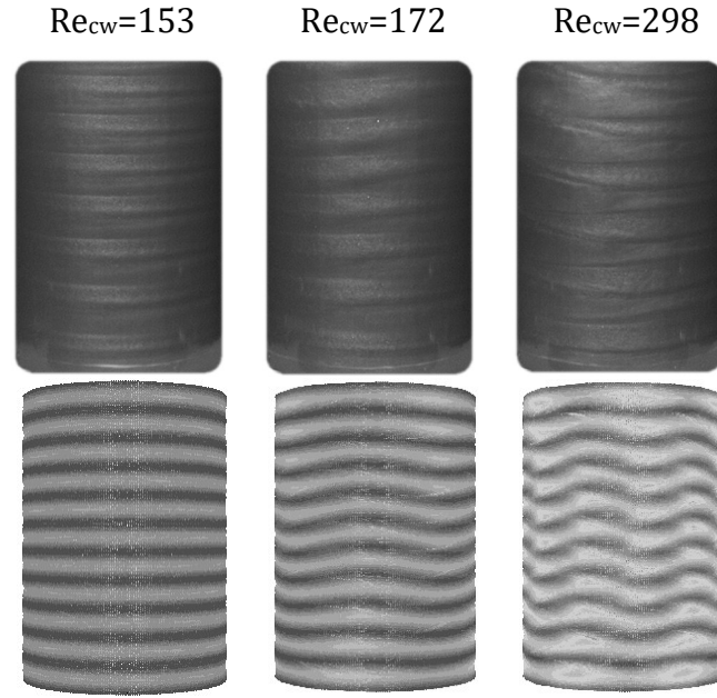
Şekil 7. 11 %0,2 XG çözeltisinin akış yapılarının deneysel ve nümerik görüntüleri.
