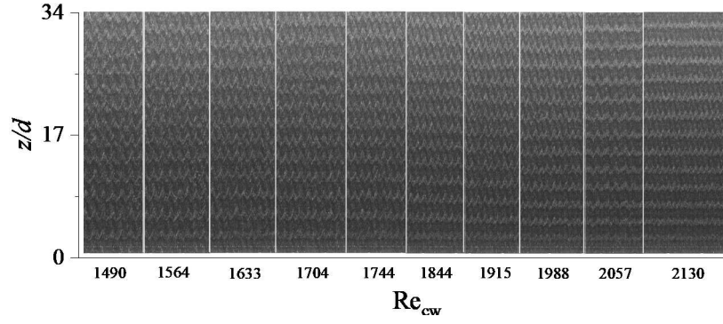
Şekil 4. 14 Farklı Re_{cw} değerlerinde gliserin akışkanına ait uzay-zaman grafiği ( \omega_o=-42\text{rpm} ).
