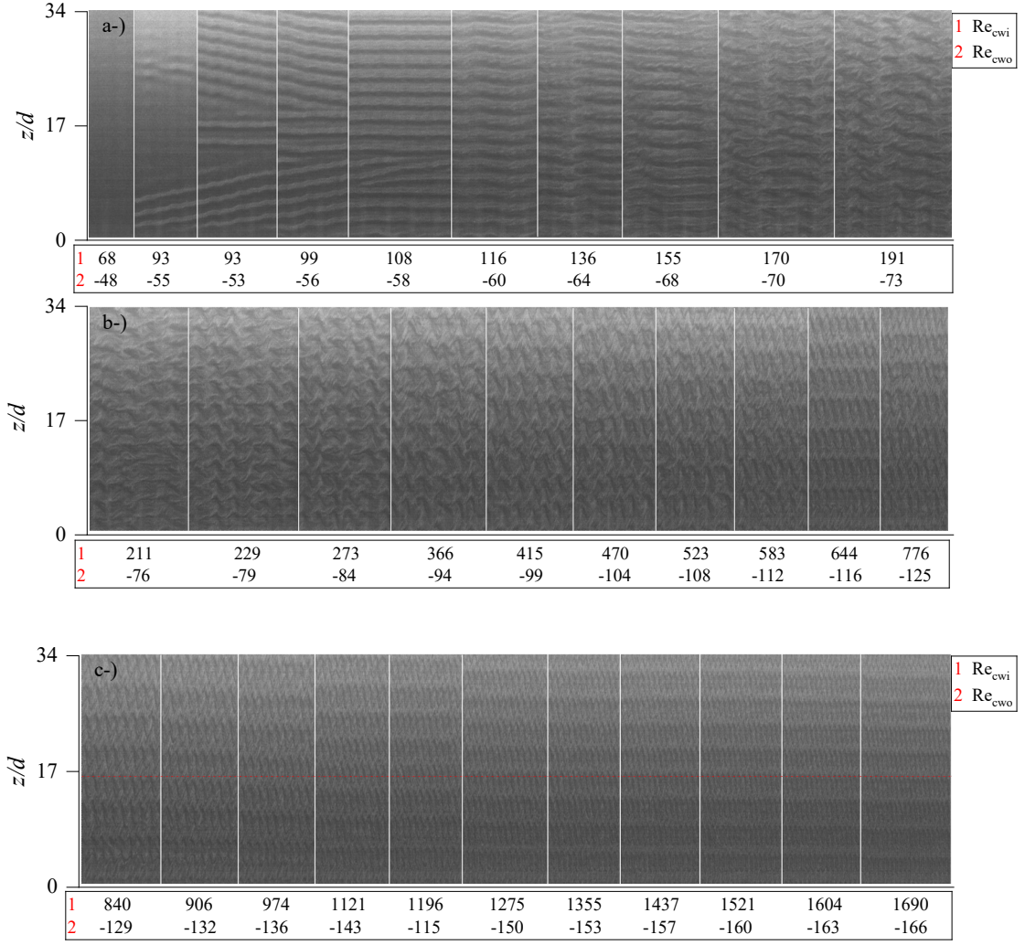
Şekil 4. 30 Farklı Re_{cw} değerlerinde %0,1 xanthan çözeltisi için uzay-zaman grafiği (zıt yön).
