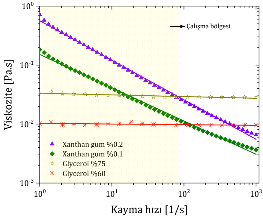
Şekil 5. 5 Deneysel alışmalar kullanılan akışkanlara ait reolojik zellikler
