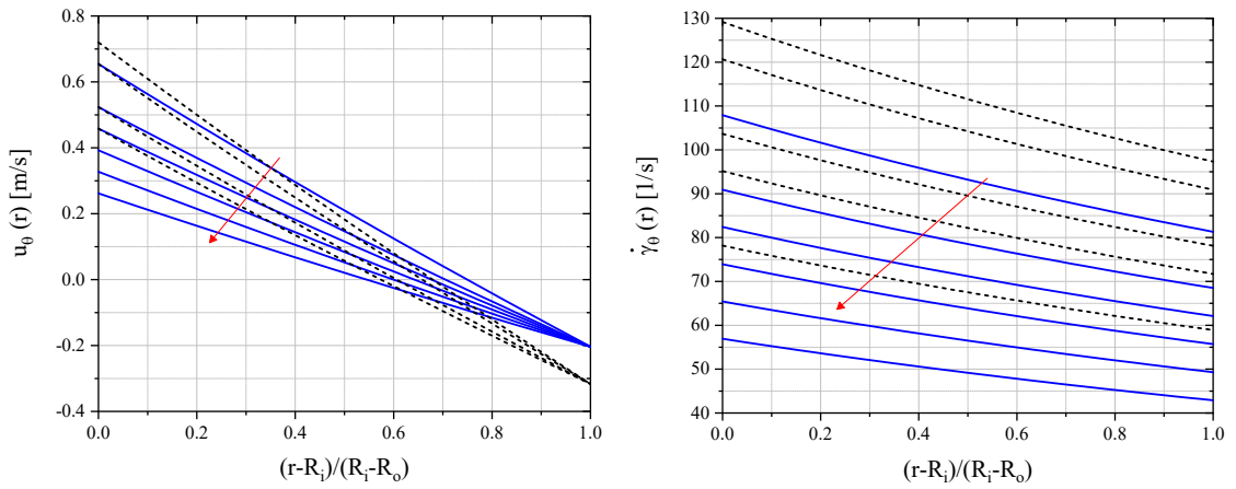
Şekil 4. 10 Silindirler arasındaki boşlukta zıt yöne dönme sonucunda hız ve kayma hızı deđişimleri.
