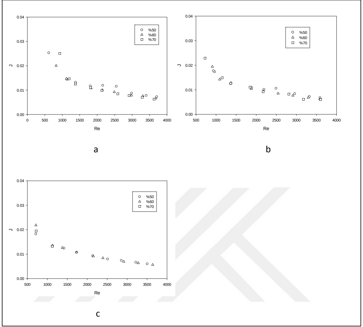
Şekil 5.9 6 sıralı bataryada bağıl nemin Colburn J faktörüne etkisi a. 30°C b.35°C c.40°C
