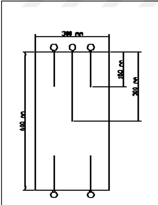
Şekil 3.12 RTD'lerin kanal içindeki yerleşimi
