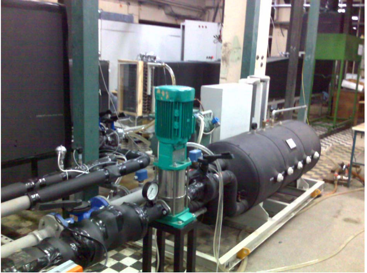
Şekil 3.7 Su soğutucu grubun fotoğrafı
