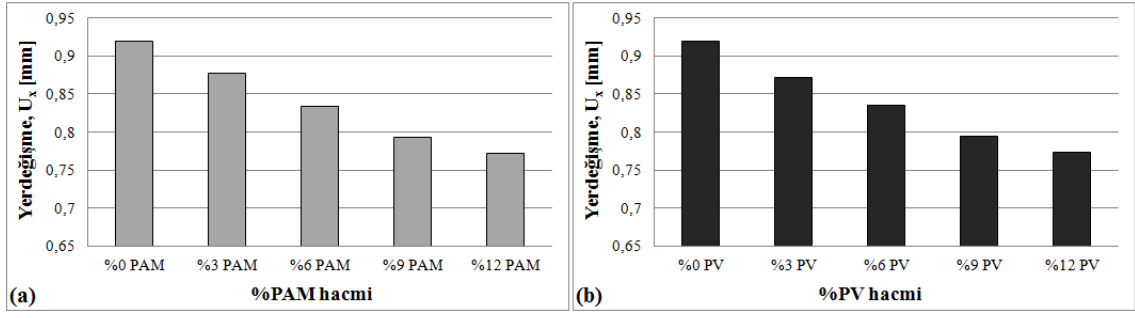
Şekil 3.26 Eğilme momenti (M) altındaki FDPM'den yapılmış tek bindirme bağlantısında, grafit hacim oranının U_x yerdeğiştirmesine etkisi, a) PAM-PAM, b) PV-PV
