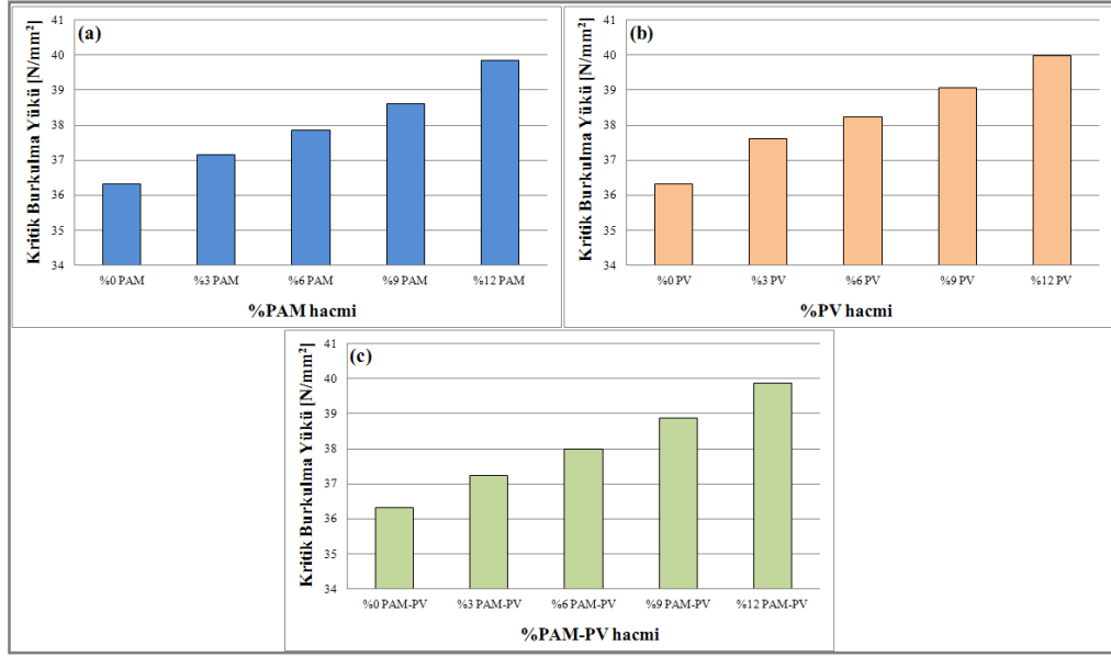
Şekil 3.15 Grafit hacim oranının kritik burkulma yüküne etkisi, doğrusal desteklenmiş FDPM'den oluşan sandviç panel yayılı yük altında, q, a) PAM-PAM, b) PV-PV, c) PAM-PV
