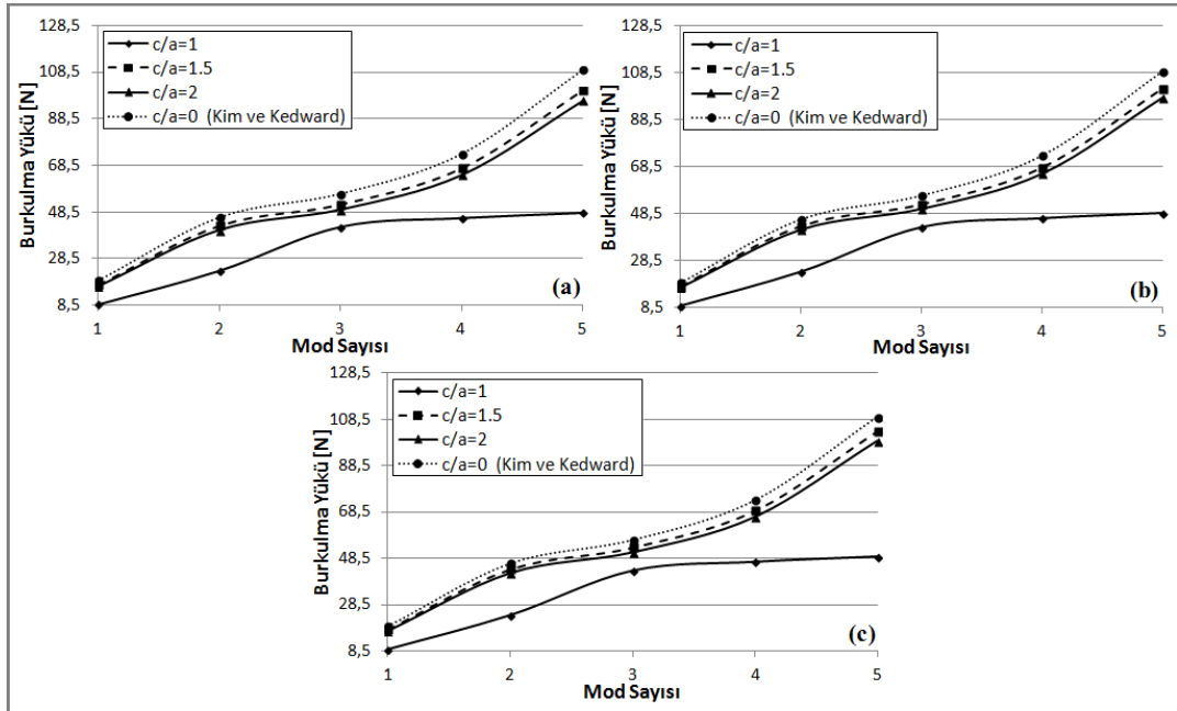
Şekil 4.11 c/a oranına göre burkulma yüklerindeki değişim, (c/a=1, c/a=1.5, c/a=2) a) cam-epoksi, b) grafit-epoksi, c) bor-epoksi
