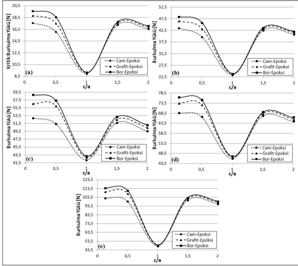
Şekil 4.9 İnküzyon malzemesinin burkulma yüküne etkisi, a) mod 1, b) mod 2, c) mod 3, d) mod 4, e) mod 5
