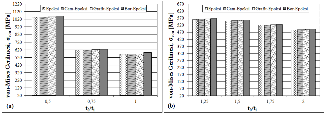
Şekil 4.25 Çekme yükü altındaki, inklüzyon içeren tek bindirme bağlantılarında t_o/t_i oranının von-Mises gerilmesi ( \sigma_{von} ) üzerine etkisi a) 0.5, 0.75, 1, b) 1.25, 1.5, 1.75, 2
