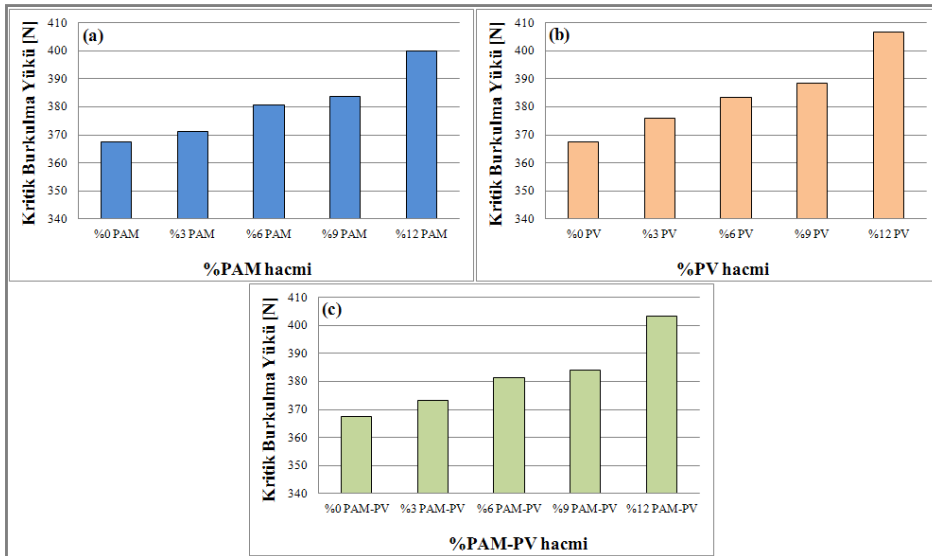
Şekil 3.11 Grafit hacim oranının kritik burkulma yüküne etkisi, noktasal desteklenmiş FDPM'den oluşan sandviç panel düzlem içi normal bası kuvveti altında, N, a) PAM-PAM, b) PV-PV, c) PAM-PV
