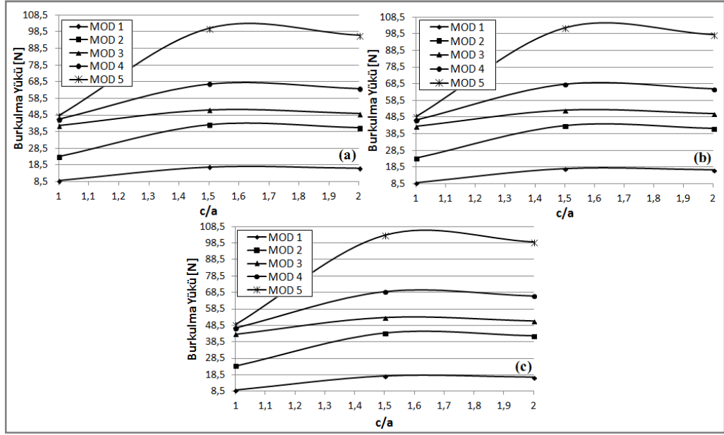
Şekil 4.10 c/a oranının burkulma yüküne etkisi, (c/a=1, c/a=1.5, c/a=2) a) cam-epoksi, b) grafit-epoksi, c) bor-epoksi
