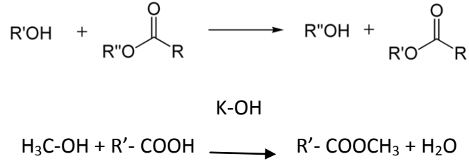
Şekil 2.31 Transesterleşme Reaksiyonu
