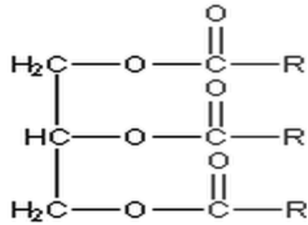
Şekil 2.15 Triaçilgliserol
