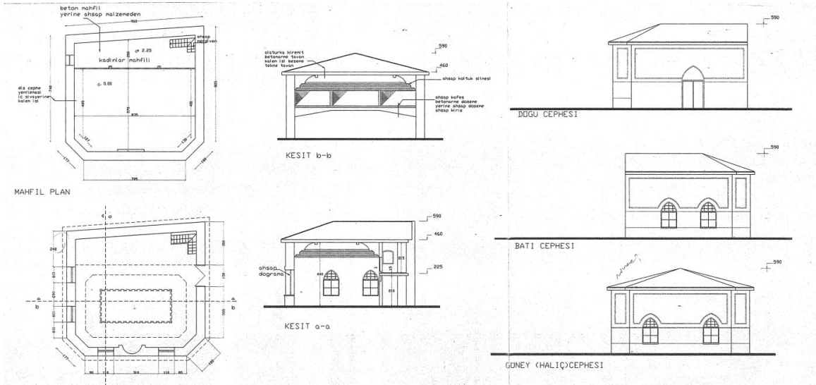
F-7 Bahariye Mevlevîhânesi Mescit Plan, Kesit ve Cephe Restitüsyonu (M. Baha Tanman ve H. Fahrünnisa Ensari Kara)
