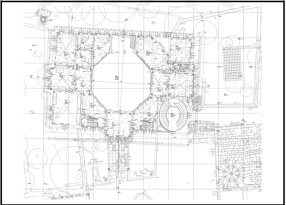
Şekil 3.52 Galata Mevlevîhânesi Rölövesi İkinci Kat Planı [121]
