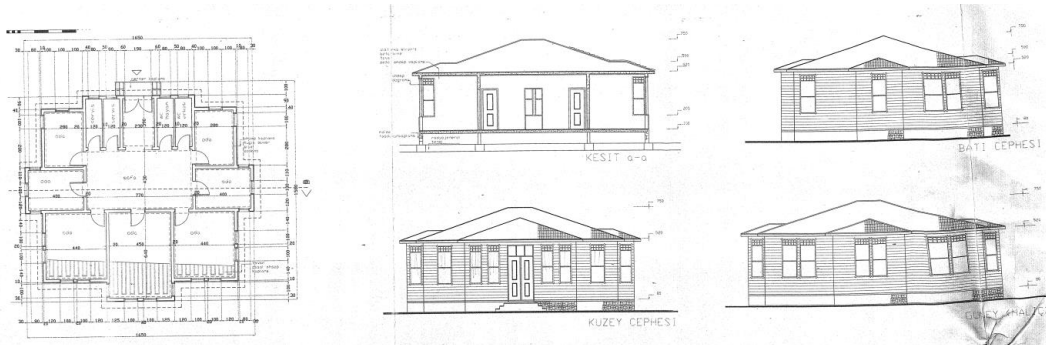
F-4 Bahariye Mevlevîhânesi Selamlık Yapısı Plan, Kesit ve Cephe Restitüsyonu (M. Baha Tanman ve H. Fahrünnisa Ensari Kara)
