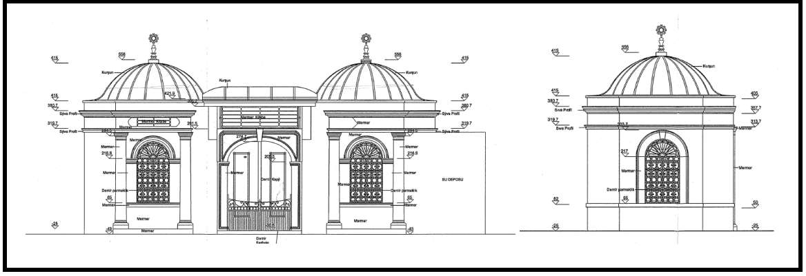
Şekil 3.171 Yenikapı Mevlevîhânesi Muvakkithane (Restitüsyon) Kuzey ve Doğu Cepheleri [121]
