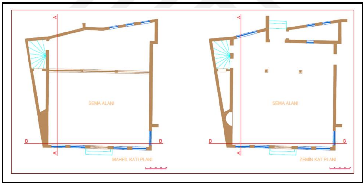
Şekil 4.23 Beşiktaş Mevlevîhânesi (Musahib Abdi Bey Yalısı) Rölövesi Kat Planları – Semahane (Yavuz Bayülken'nin rölövesinden yararlanılarak Gökben PALA AZSÖZ tarafından çizilmiştir)
