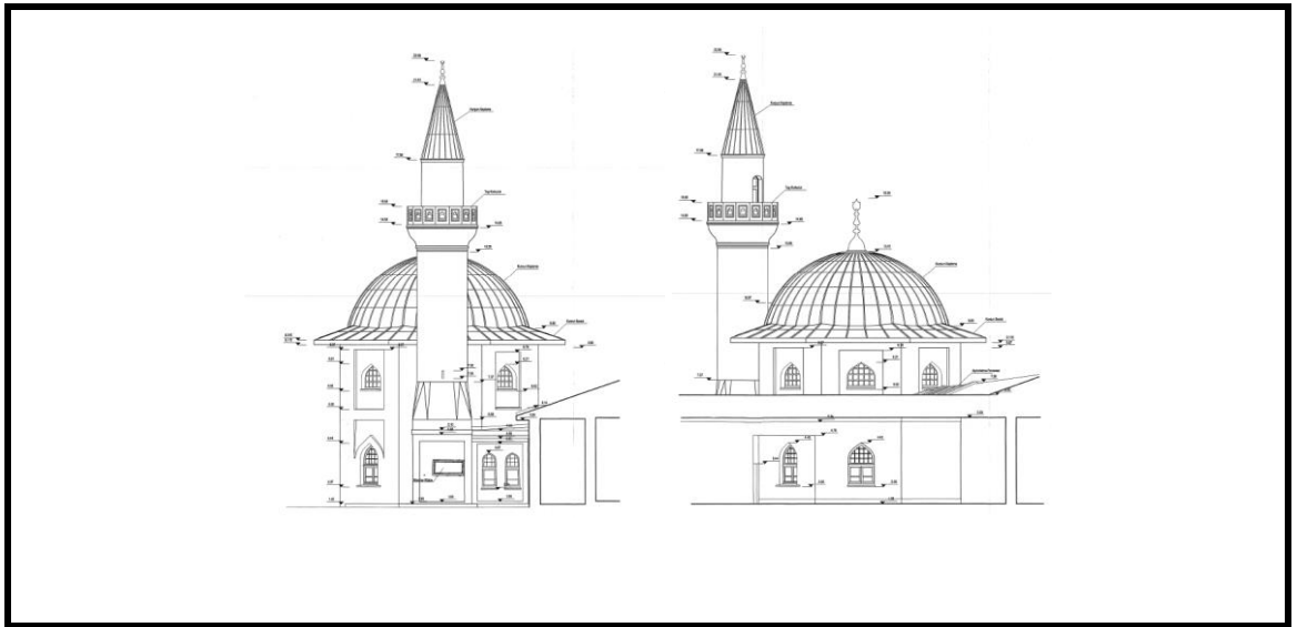
Şekil 3.135 Yenikapı Mevlevîhânesi Mescit (Restitüsyon) Doğu/Güney Cepheleri [121]
