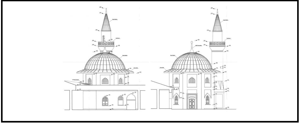
Şekil 3.136 Yenikapı Mevlevihânesi Mescit (Restitüsyon) Batı/Kuzey Cepheleri [121]
