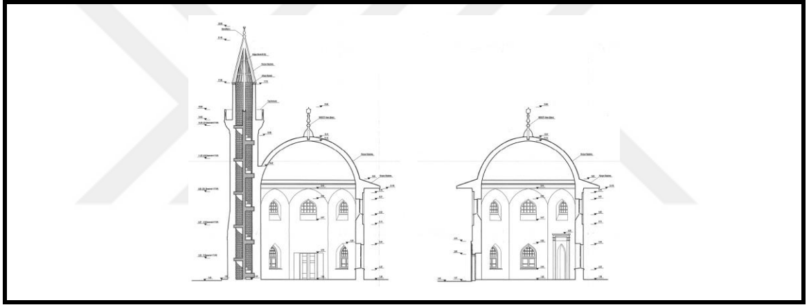
Şekil 3.134 Yenikapı Mevlevîhânesi Mescit (Restitüsyon) A-A ve B-B Kesitleri [121]
