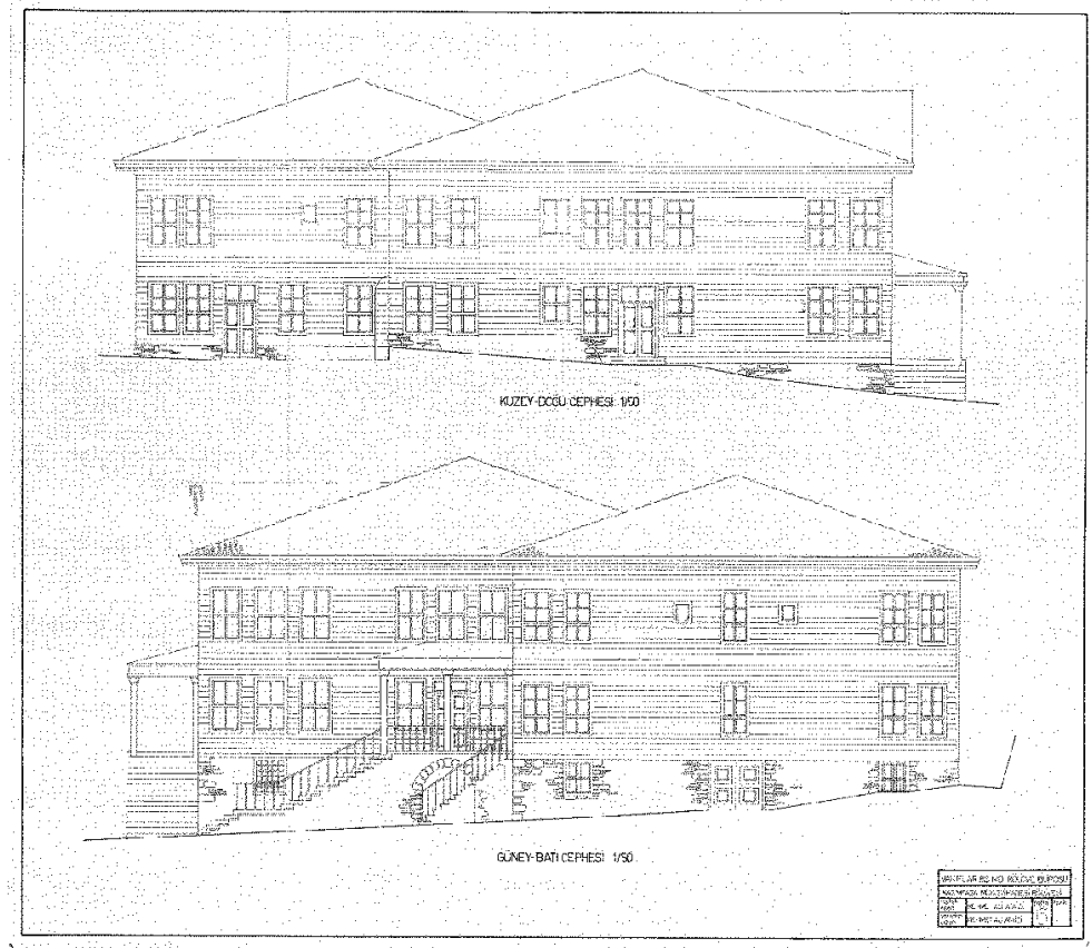
D-9 Kasımpaşa Mevlevîhânesi nin 1966 tarihli Vakıflar Genel Müdürlüğü tarafından çizilen rölövesi Kuzeydoğu ve Güneybatı Cepheleri
