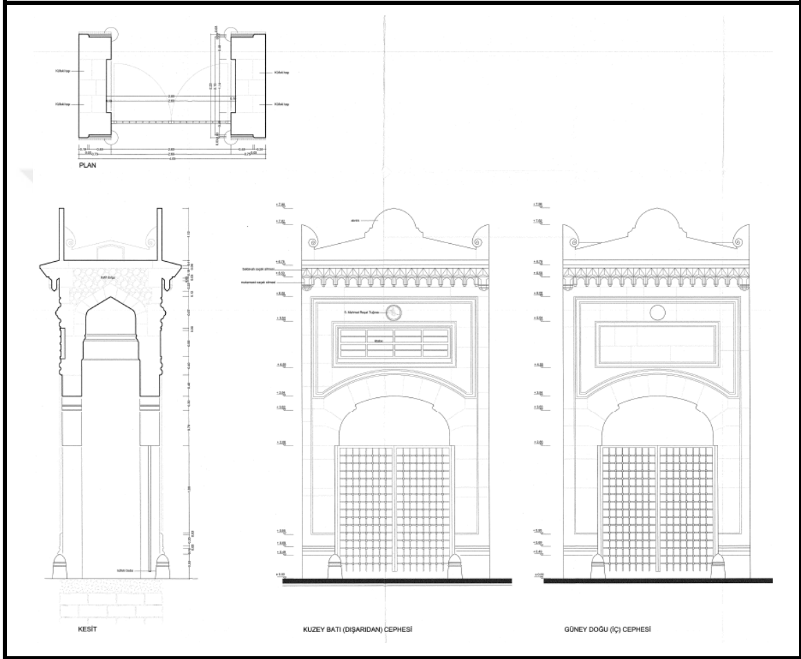
Şekil 3.266 Bahariye Mevlevîhânesi II. Restitüsyon Cümle Kapısı Plan, Kesit ve Cepheleeri
