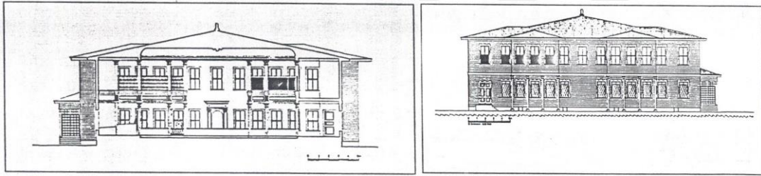
F-7 Bahariye Mevlevîhânesi Mescit Plan, Kesit ve Cephe Restitüsyonu (M. Baha Tanman ve H. Fahrünnisa Ensari Kara)
