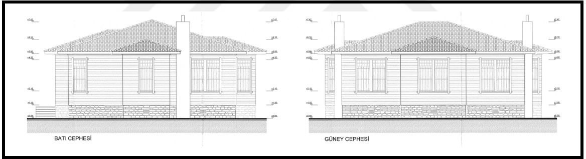
Şekil 3.272 Bahariye Mevlevîhânesi Restitüsyon Selamlık Batı-Güney Cepheleri [121]
