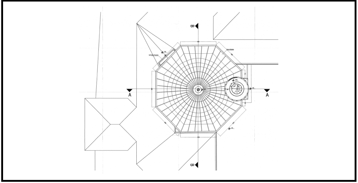
Şekil 3.133 Yenikapı Mevlevîhânesi Mescit +16.00 kodu (Restitüsyon) Planı [121]
