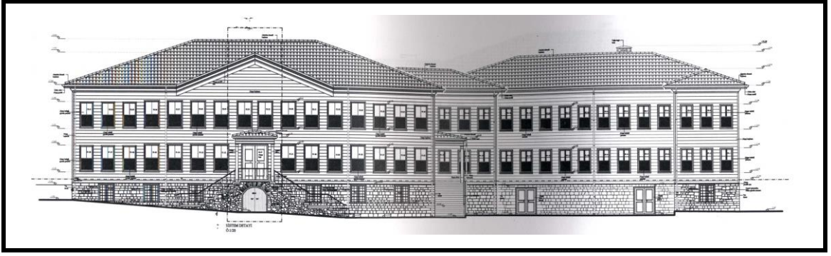
Şekil 3.206 Kasımpaşa Mevlevîhânesi Rekonstrüksiyon Ön Cephe [121]
