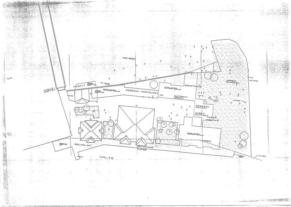
F-3 12/04/1908 tarihli Bahariye Mevlevîhânesi Selamlık Dairesine ait planı
