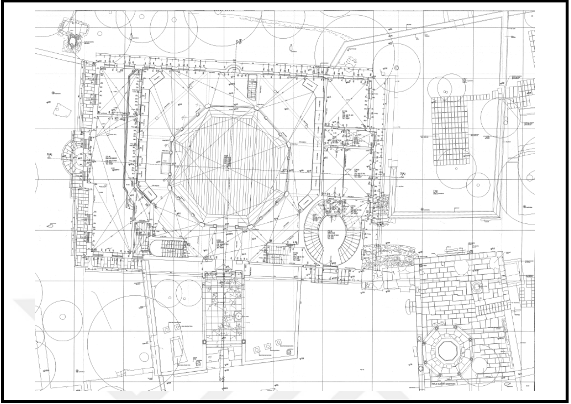
Şekil 3.51 Galata Mevlevîhânesi Rölövesi Birinci Kat Planı [121]
