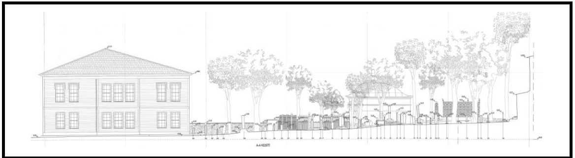
Şekil 3.62 Galata Mevlevîhânesi 2008 Rölövesi Hazire A-A Kesiti [121]
