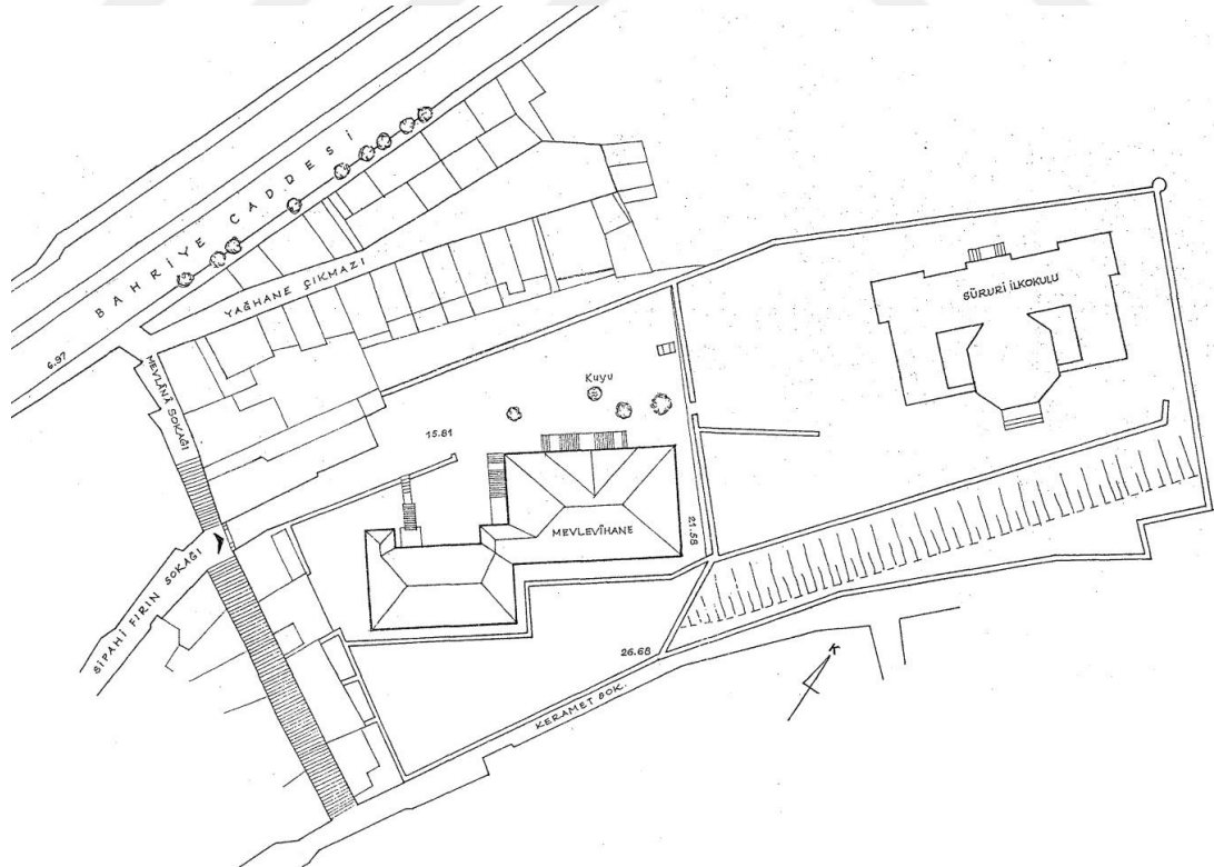
D-3 Kasımpaşa Mevlevîhânesi'nin Nejdet Sargın'a ait vaziyet planı
