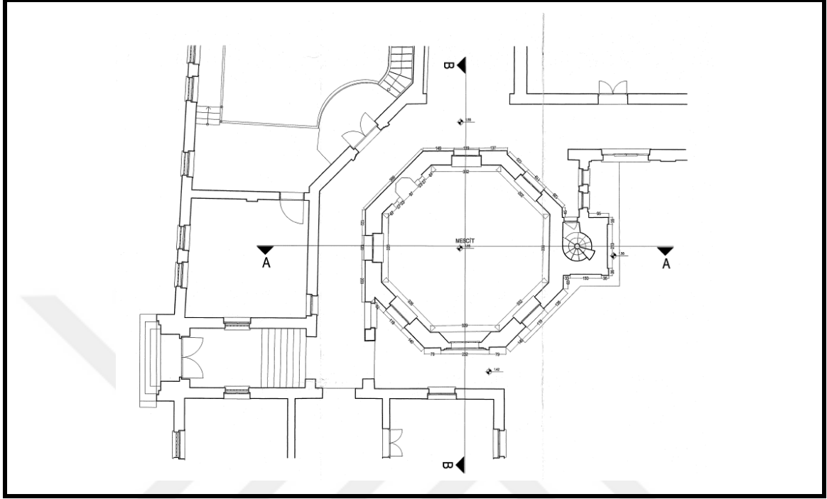
Şekil 3.131 Yenikapı Mevlâhânesi Mescit +3.00 kodu (Restitüsyon) Planı [121]
