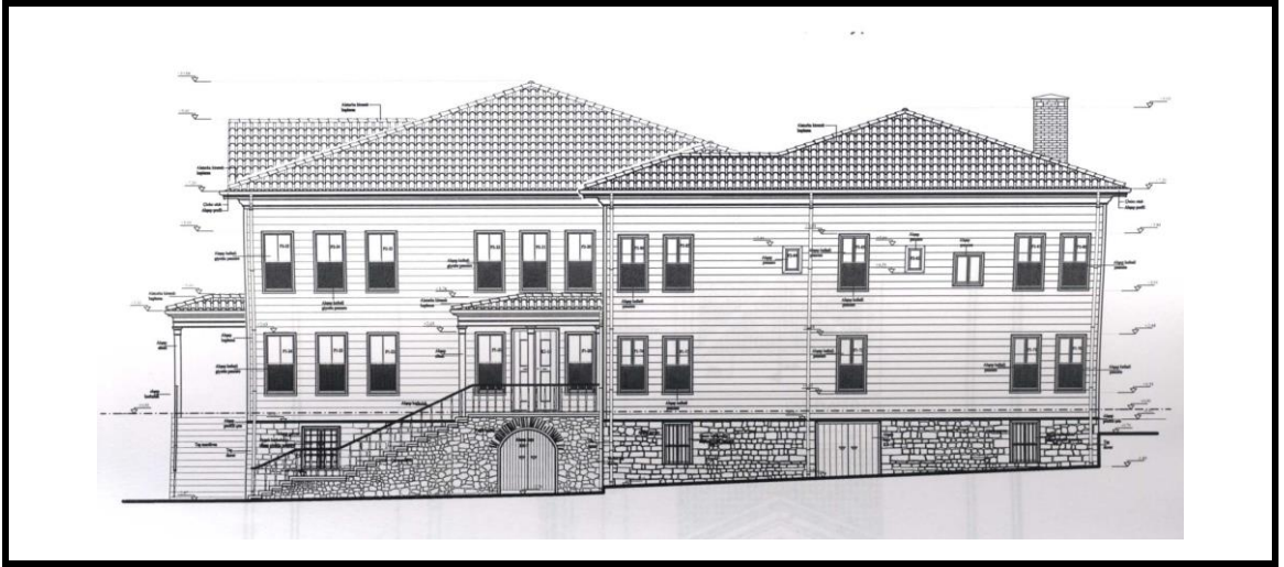
Şekil 3.208 Kasımpaşa Mevlevîhânesi Rekonstrüksiyon Sağ Yan Cephe [121]
