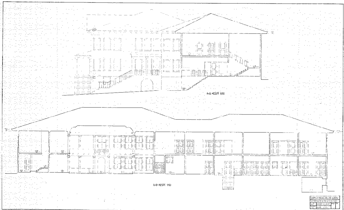
D-7 Kasımpaşa Mevlevîhânesi'nin 1966 tarihli Vakıflar Genel Müdürlüğü tarafından çizilen rölövesi A-A Kesiti ve B-B Kesiti
