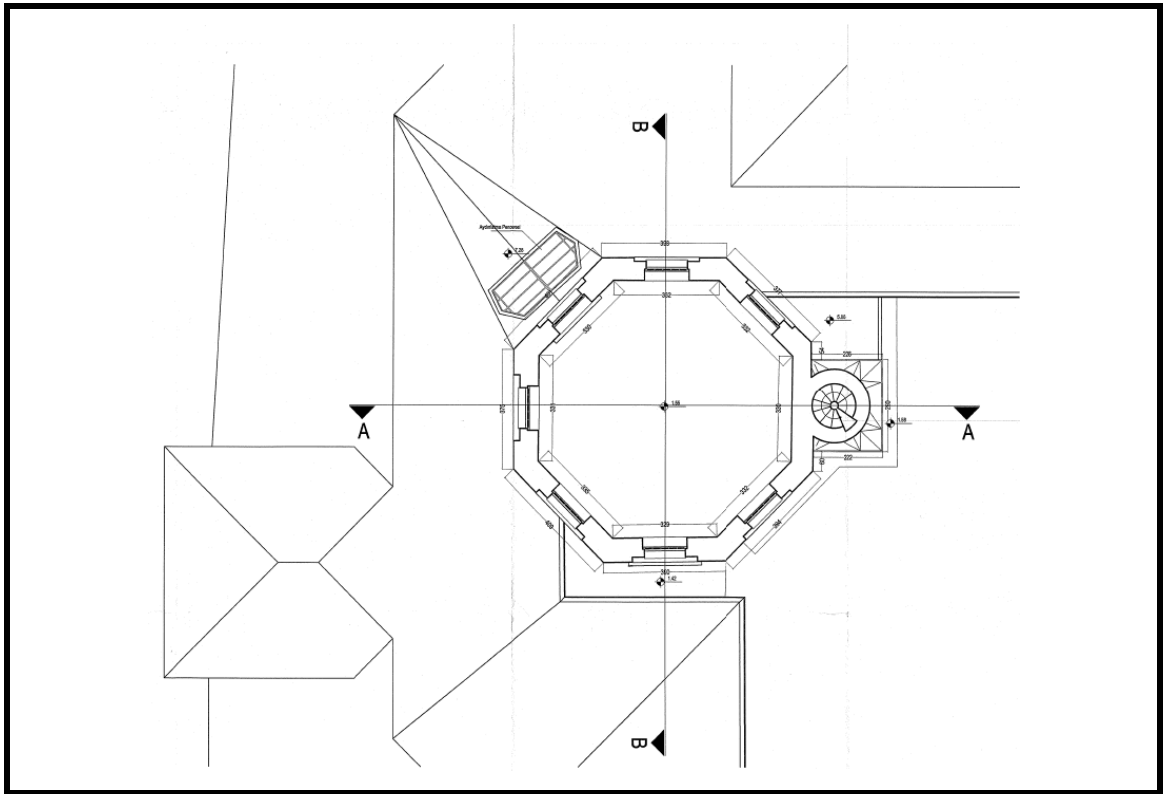
Şekil 3.132 Yenikapı Mevlâhânesi Mescit +12.00 kodu (Restitüsyon) Planı [121]
