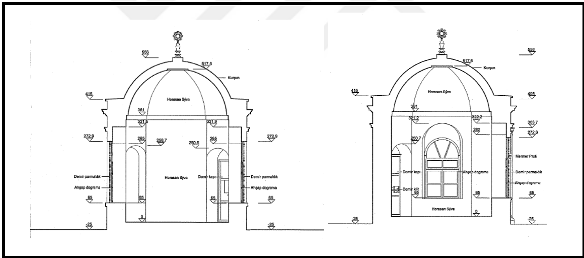
Şekil 3.170 Yenikapı Mevlevîhânesi Muvakkithane (Restitüsyon) A-A ve B-B Kesitleri [121]
