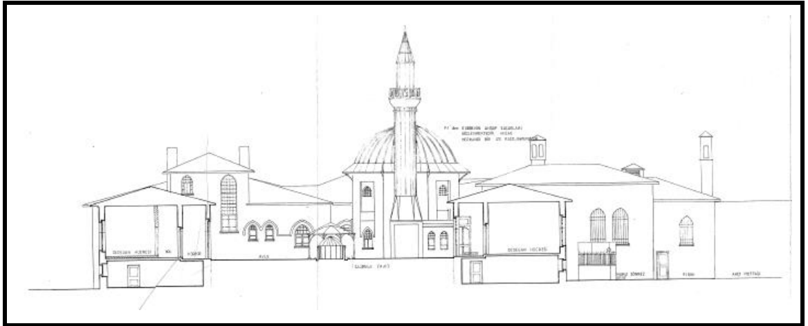
Şekil 3.127 Dedegan Hücreleri (Restitüsyon) A-A Kesiti [121]
