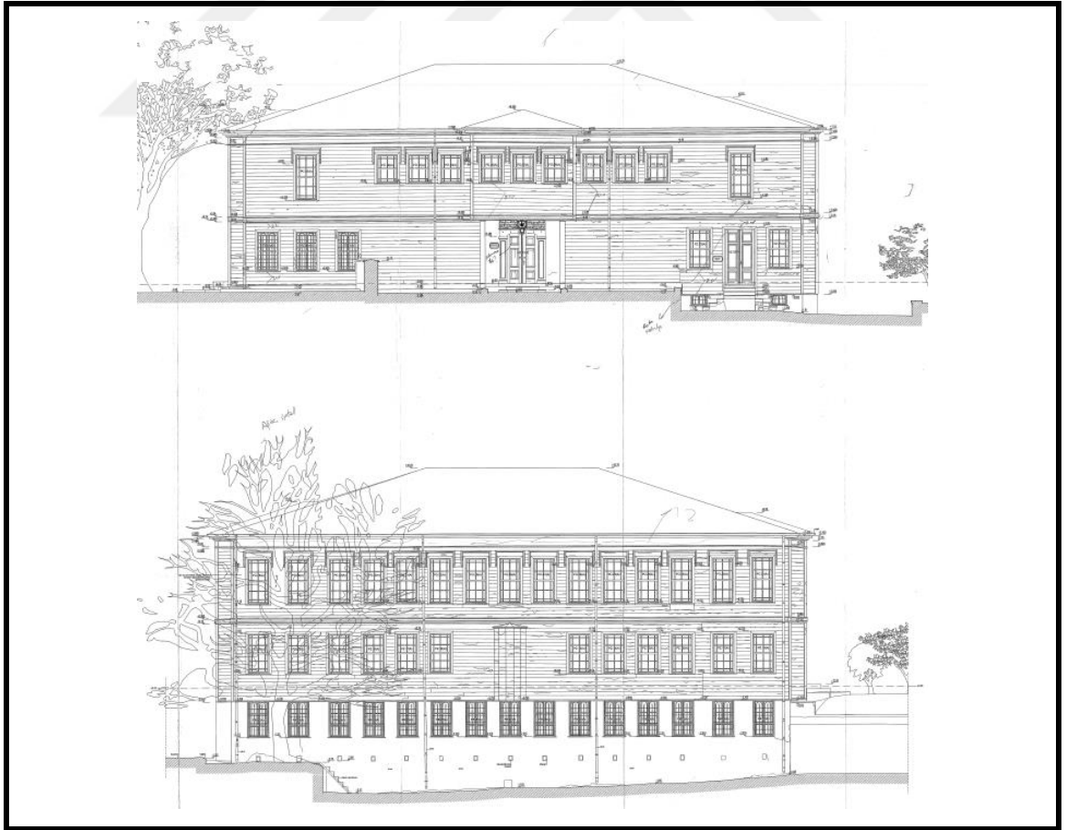
Şekil 3.54 Galata Mevlevîhânesi Rölövesi Semahane Görünüşler [121]
