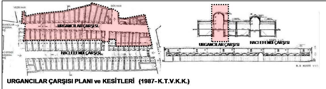
Şekil 3.44 Urgancilar Çarşısı/Arastası plan ve kesitleri
