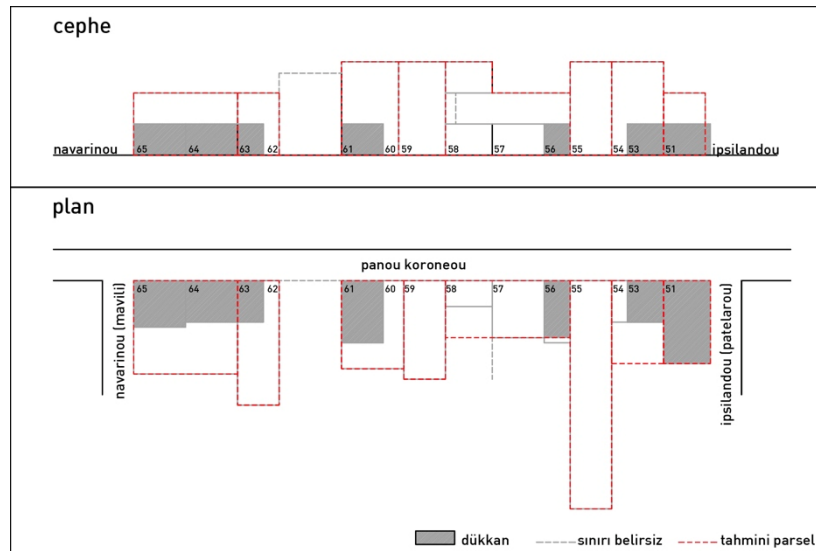
Şekil 6.2.2 Resmo Mülteci Rehabilitasyon Komitesi belgelerine göre Navarinou ve İpsilandou Sokakları arasındaki olası parselasyon
