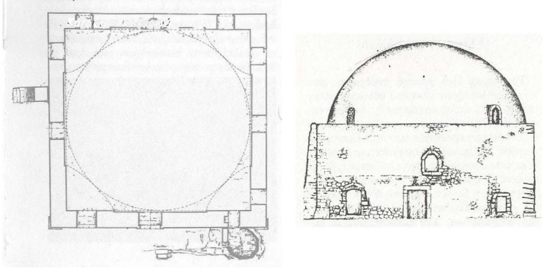
Şekil 2.2 Sultan İbrahim Han Camisi Planı ve Görünüşü [44]
