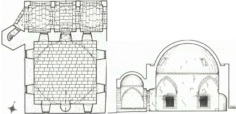
Şekil 2.5 Kara Musa Camisi planı ve kesiti [19]
