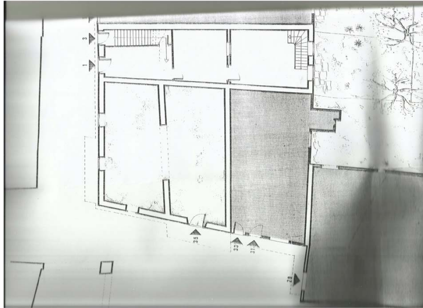
Şekil 6.2.5 Kolokotroni Sokağı, 276 ve 349 numaralı mülklerin giriş kat rölövesi, Resmo eski şehir koruma planı, N. Moutsopoulos, [45]
