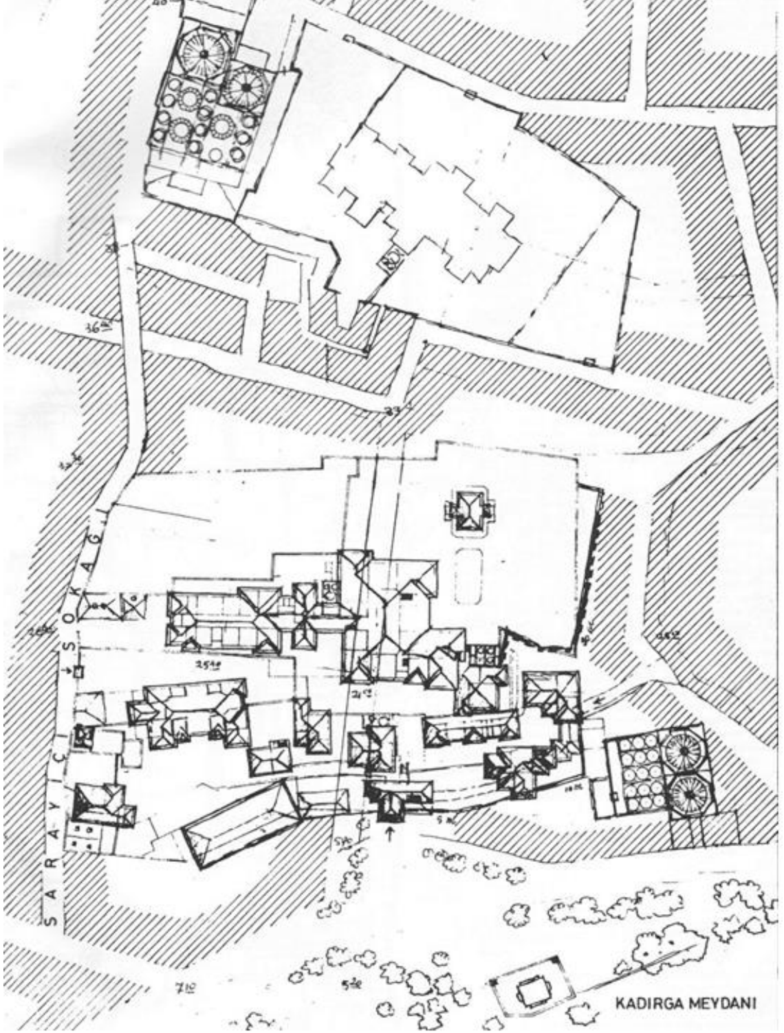
Şekil 4. 1: Esmâ Sultan Sarayı (Sedat Hakkı Eldem) [110]
