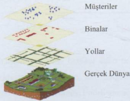
Şekil 5.10 Harita Katmanları
