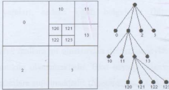
Şekil 6.3 Quad-tree
