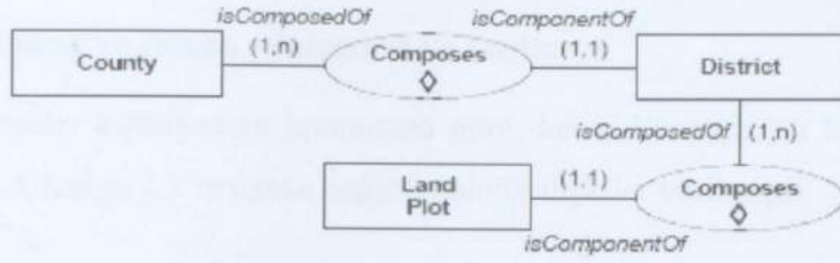
Şekil 3.9 Aggregation ilişkisi
