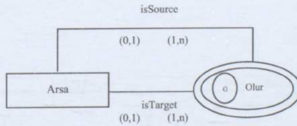
Şekil 3.6 Yaratma yapısı
