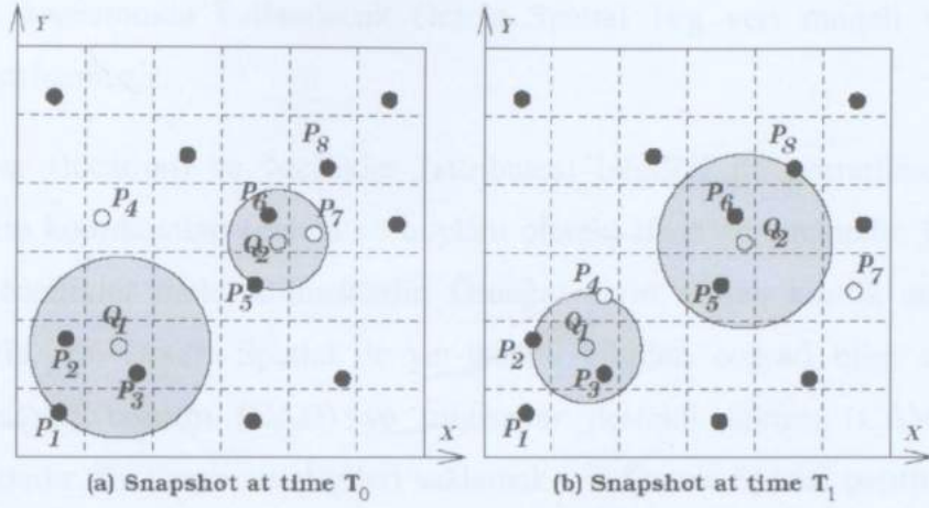
Şekil 4.10 kNN sorgusu
