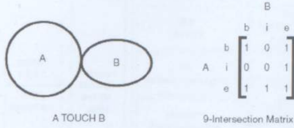
Şekil 5.5 9 Etkileşim modeli
