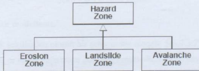
Şekil 3.4 Is-a ilişkisi
