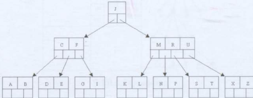
Şekil 6.1 B+tree
