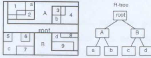
Şekil 6.2 R-tree
