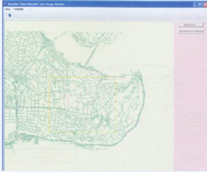
Şekil 5.12 Hareketli nesneler
