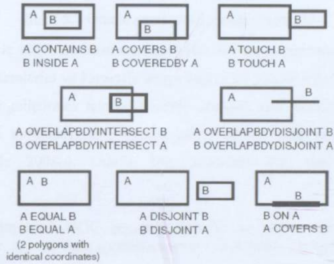
Şekil 5.6 Topolojik ilişkiler
