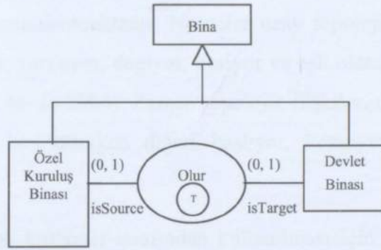
Şekil 3.5 Geçiş yapısı
