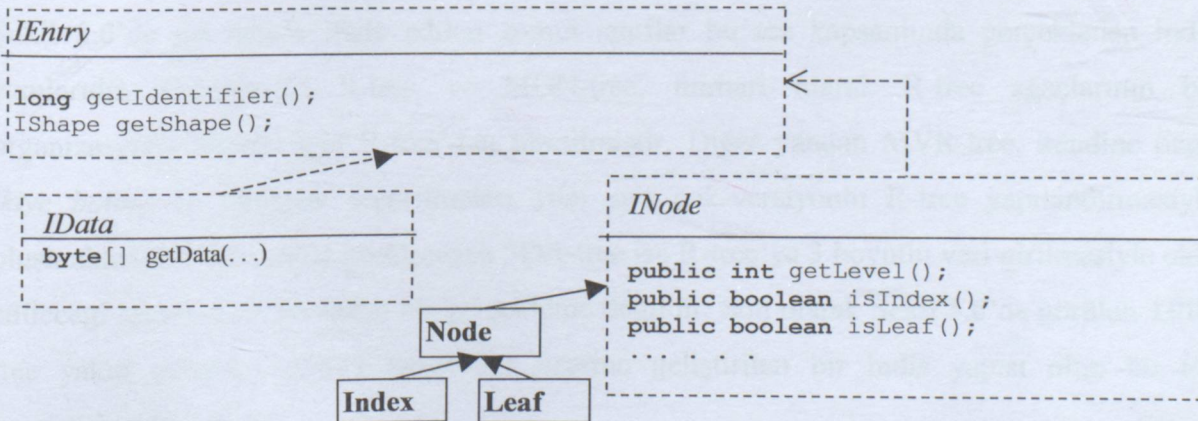
Şekil 5.5 Erişim yapısındaki veri üniteleri için UML diyagramı
