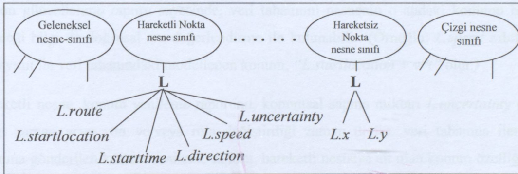
Şekil 2.3 MOST veri modelinde tanımlanan nesne sınıfları
