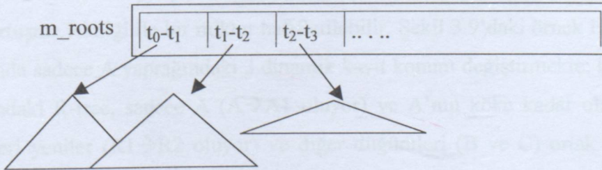
Şekil 3.8 Bir grup R-tree versiyonları
