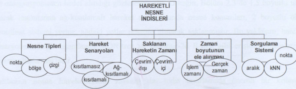
Şekil 3.4 Hareketli Nesnelerin çeşitlenmesi için ele alınan parametreler
