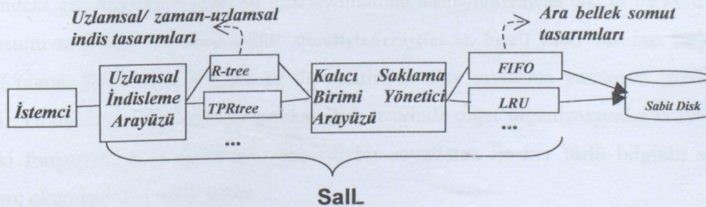
Şekil 5.2 SaIL kütüphanesinin ana mimari yapısı
