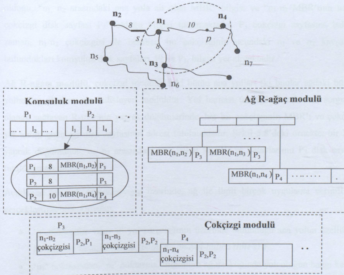
Şekil 5.8 Ağ disk organizasyonu modülleri
