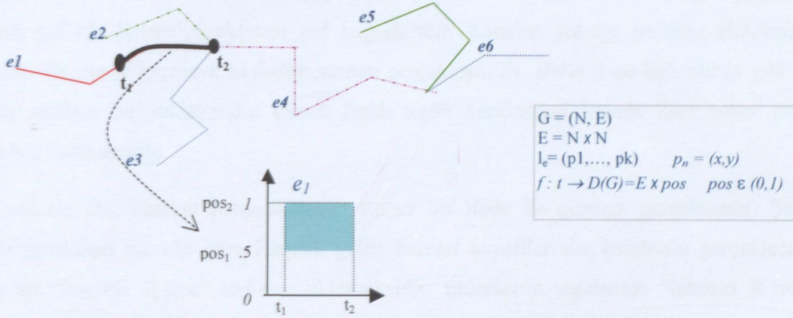
Şekil 3.18 ‘ e1 ’ kenarı üzerindeki nesne hareketinin modellenmesi
