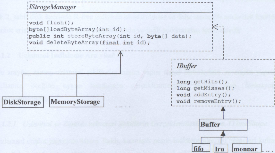
Şekil 5.3 Kalıcı Saklama Birimi ara yüzü UML diyagramı
