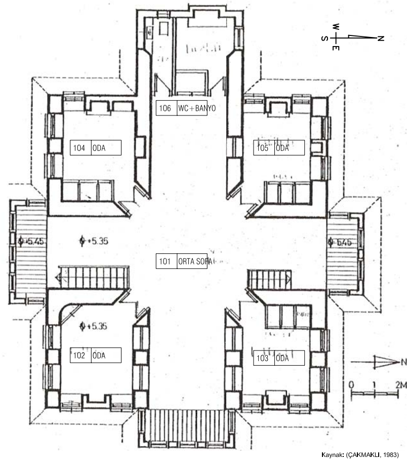
1. KAT PLANI
