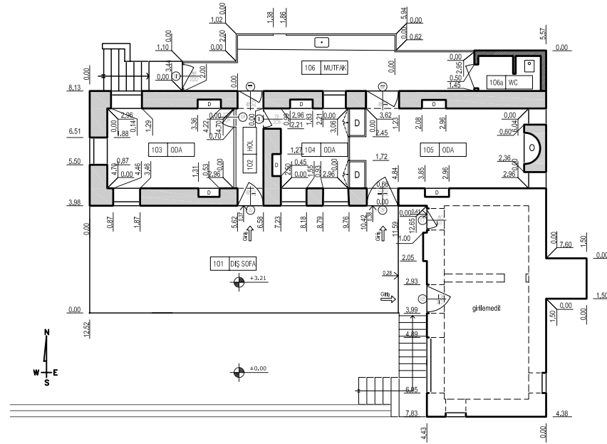
1. KAT PLANI
