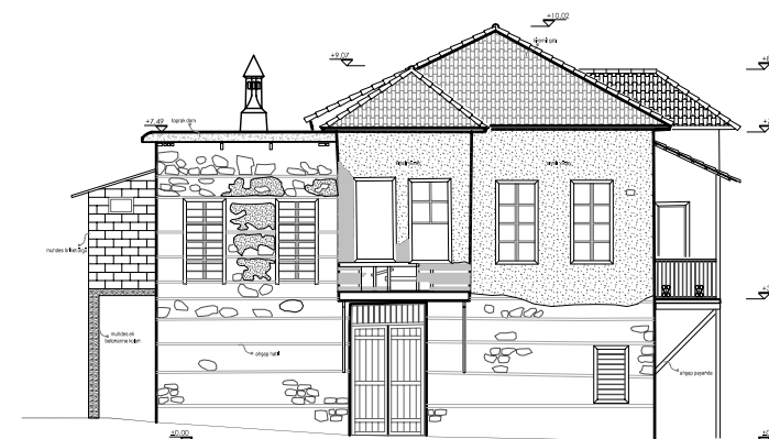
BATI CEPHESİ
