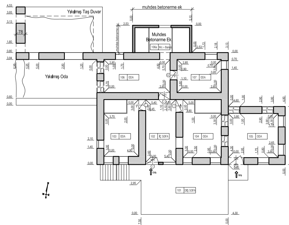
1. KAT PLANI
