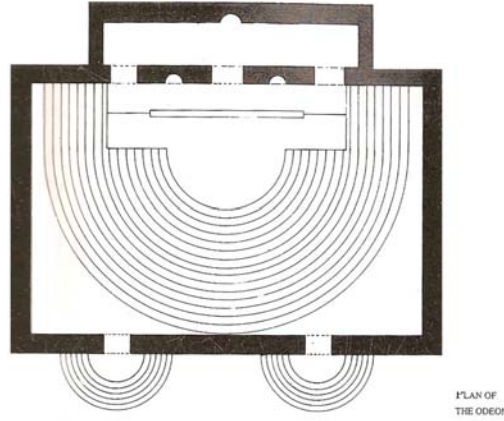
Şekil 2.4 Anemurium'da Yer Alan Odeon Planı (Alan ve Uysal, 2001)
