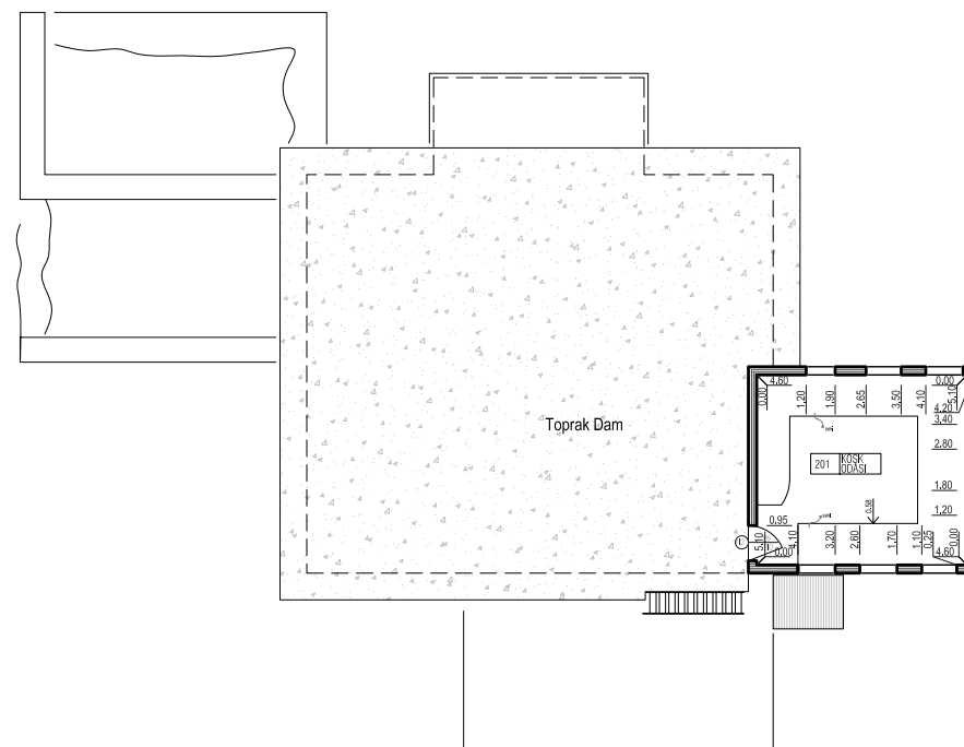
KÖŞK KATI PLANI
