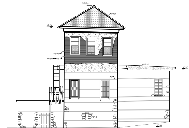
DOĞU CEPHESİ
