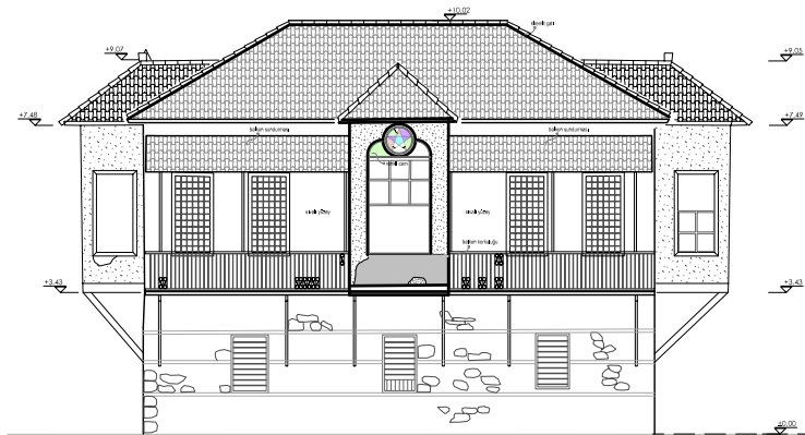
GÜNEY CEPHESİ
