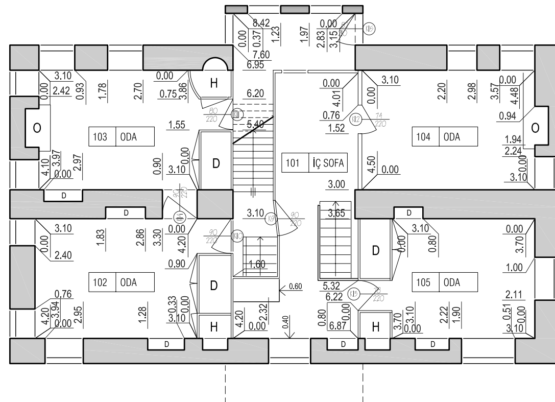
1. KAT PLANI
