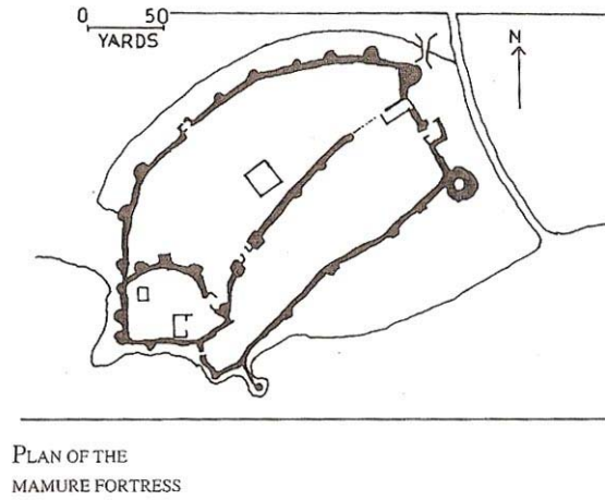
Şekil 2.8 Mamure Kalesi Planı (Alan ve Uysal, 2001)
