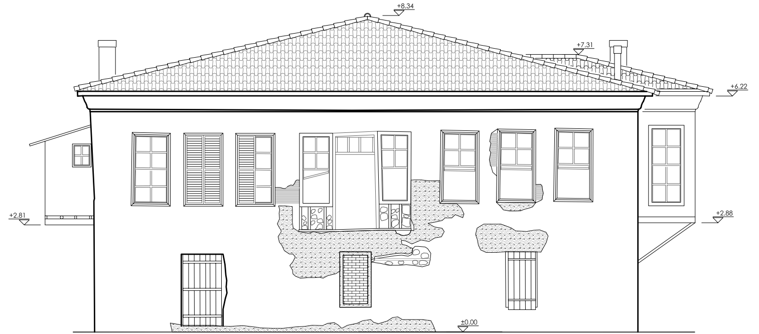
GÜNEY CEPHESİ
