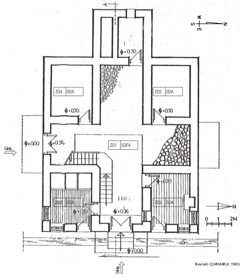
ZEMİN KAT PLANI
