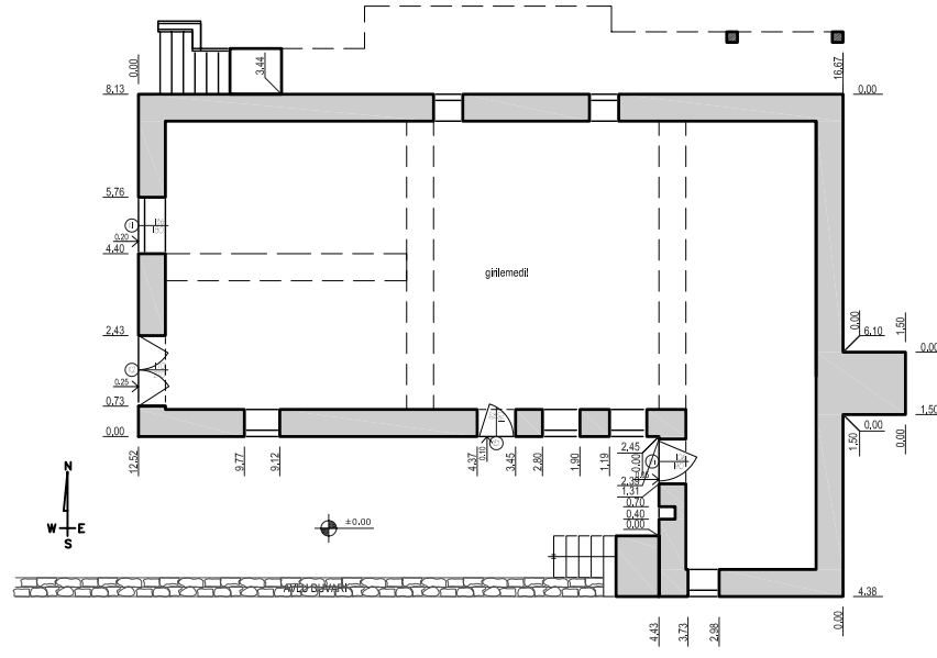
ZEMİN KAT PLANI
