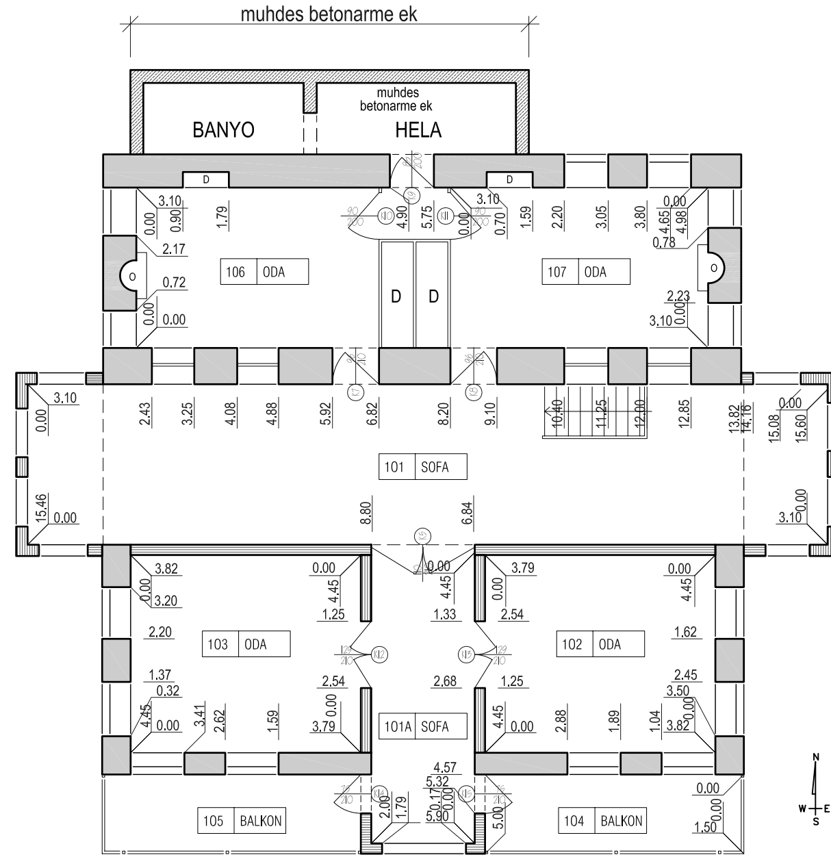
1. KAT PLANI
