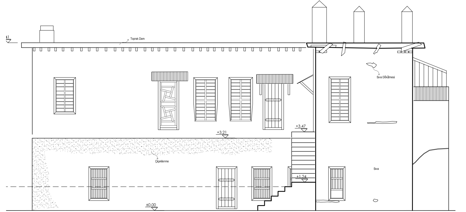
GÜNEY CEPHESİ
