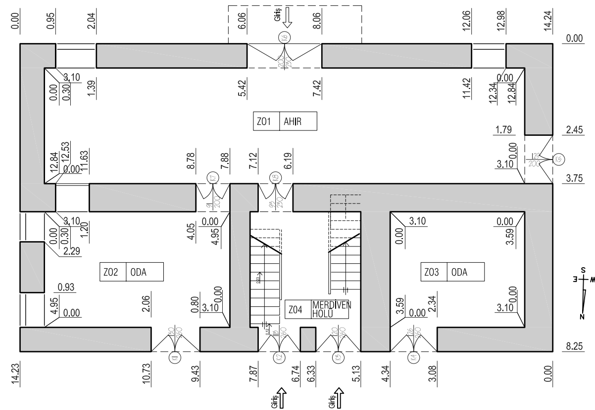
1. KAT PLANI
