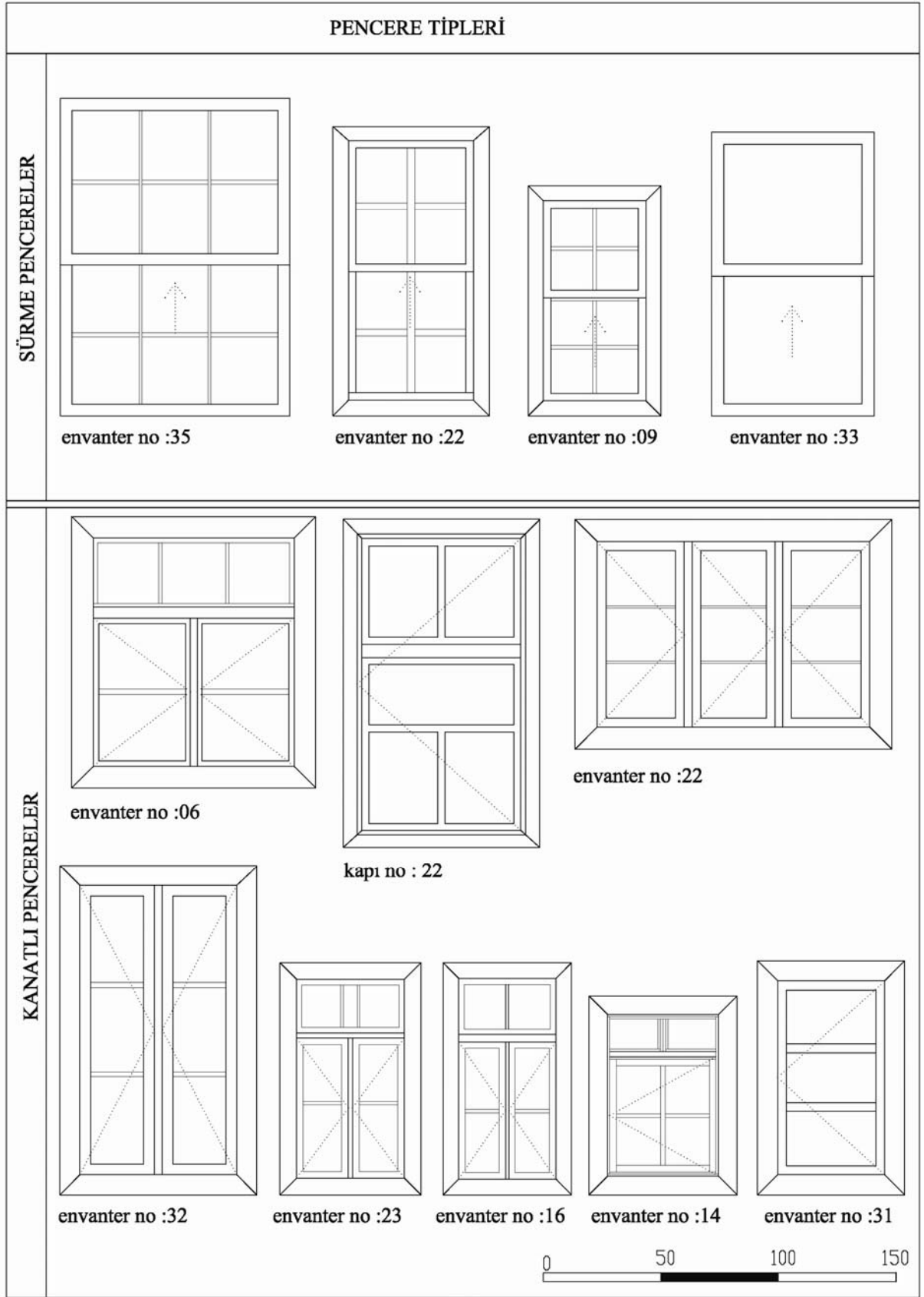
Şekil 4.43 Ürnlü geleneksel evleri pencere tipleri
