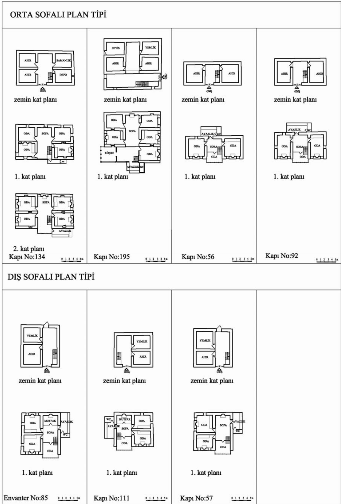
Şekil 4.20 Ürünü geleneksel evleri plan tipleri
