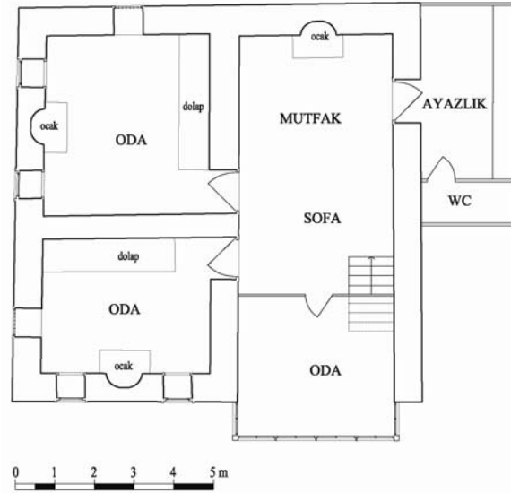
Şekil 4.5 Dış sofalı plan tipine örnek (Yaşar Erman evi)
