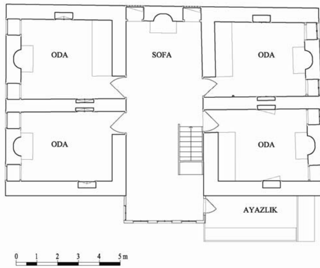
Şekil 4.6 Orta sofalı plan tipine örnek (Ayşe Bayındır evi)
