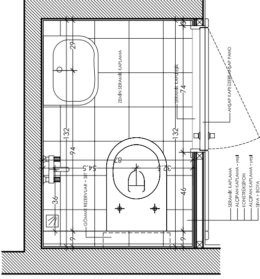
YATAK ODALARI TİP BANYO DETAYI
