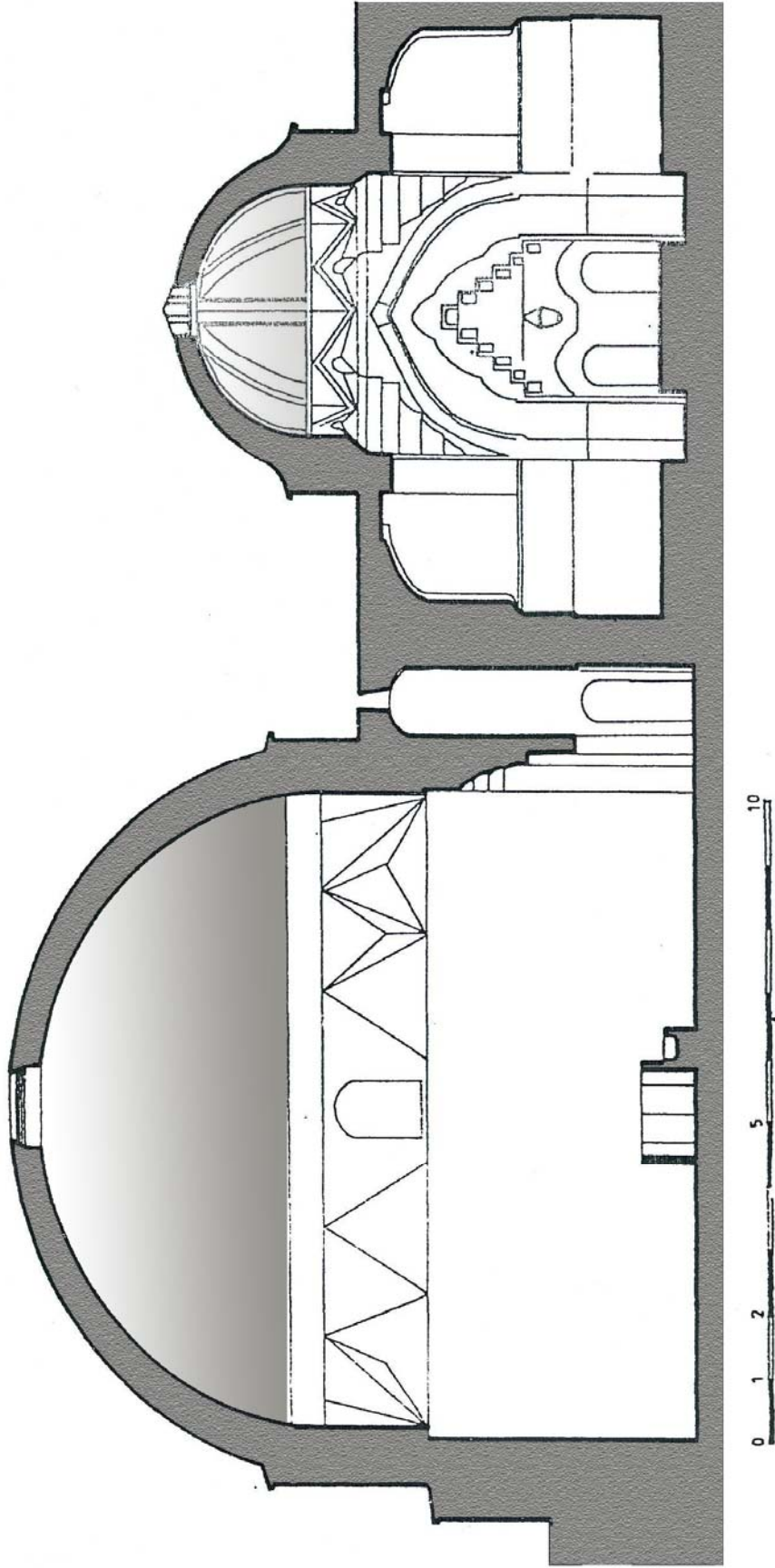
Çizim 3.4 Yıldırım Hamamı Kesiti, E. H. Ayverdi
