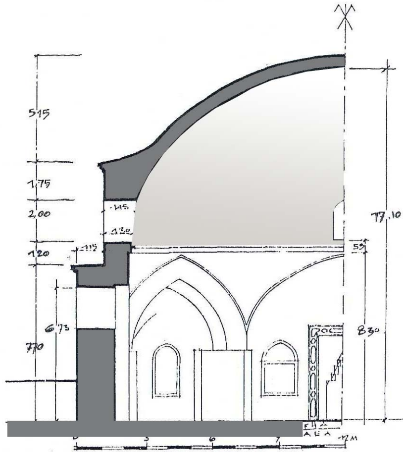
Çizim 3.2 Yıldırım Camii Kesiti, E. H. Ayverdi
