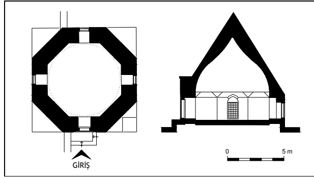
Şekil 2.9 Büyük kümbet plan ve kesit krokisi (Arel, 1962'den tekrar çizim)
