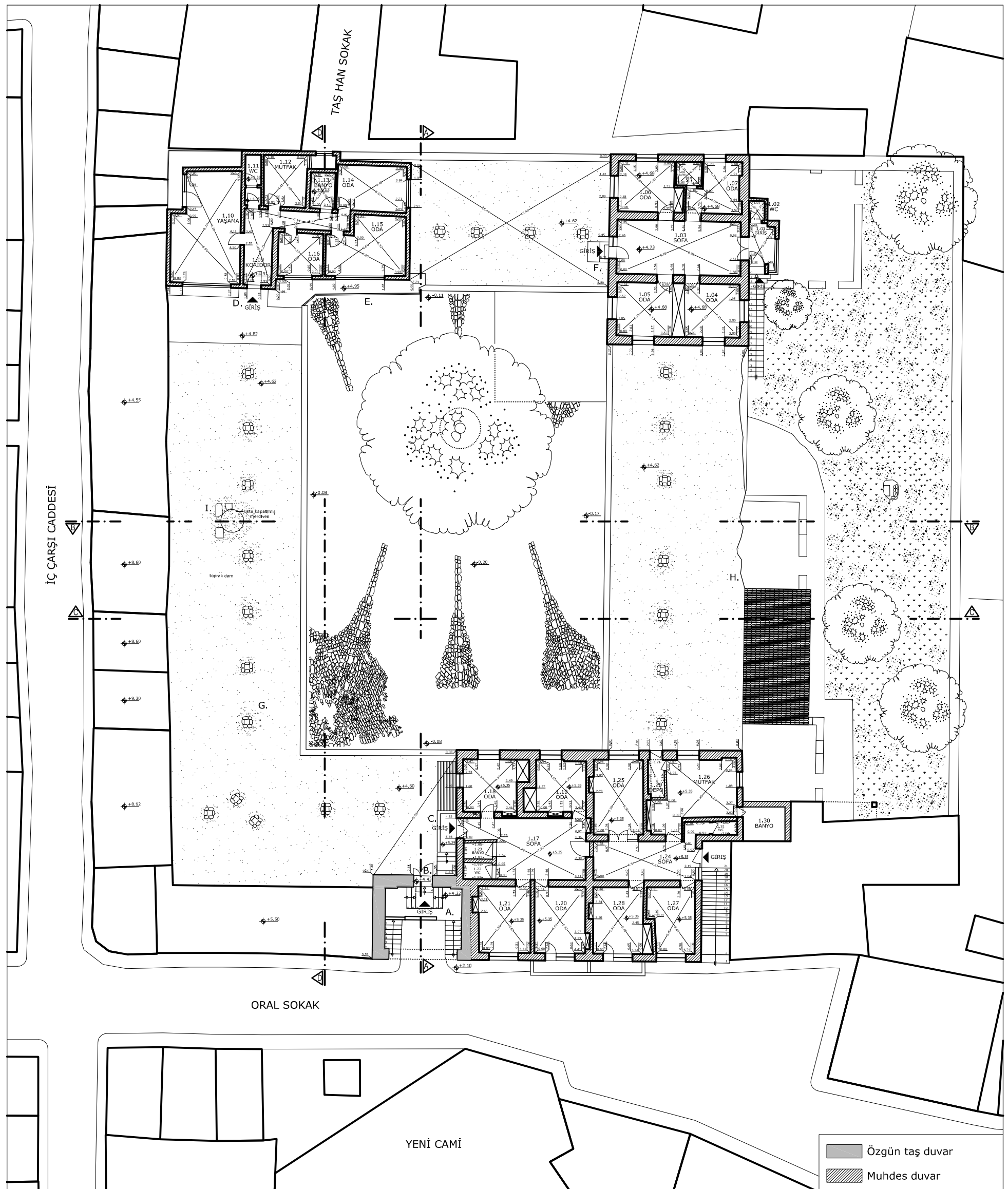
RÖLÖVE - BİRİNCİ KAT PLANI 1/100
