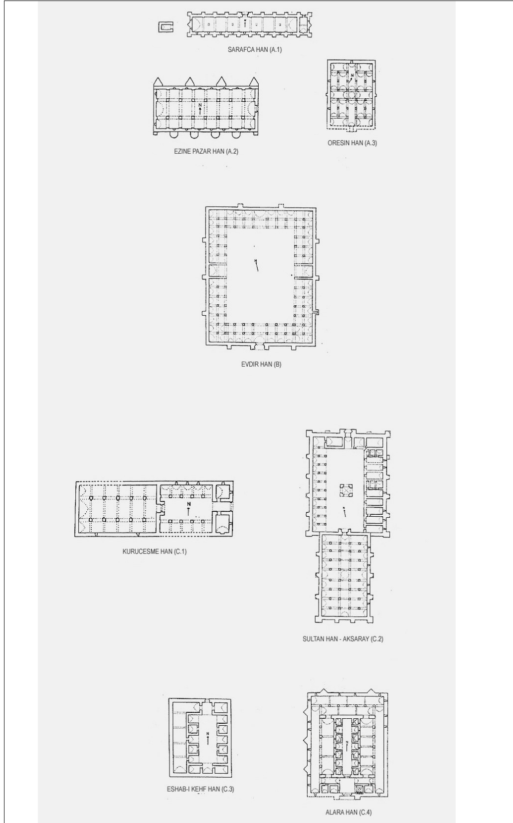
Şekil 3.2 Anadolu Selçuklu Hanları plan tipleri (Bektaş, 1999)
