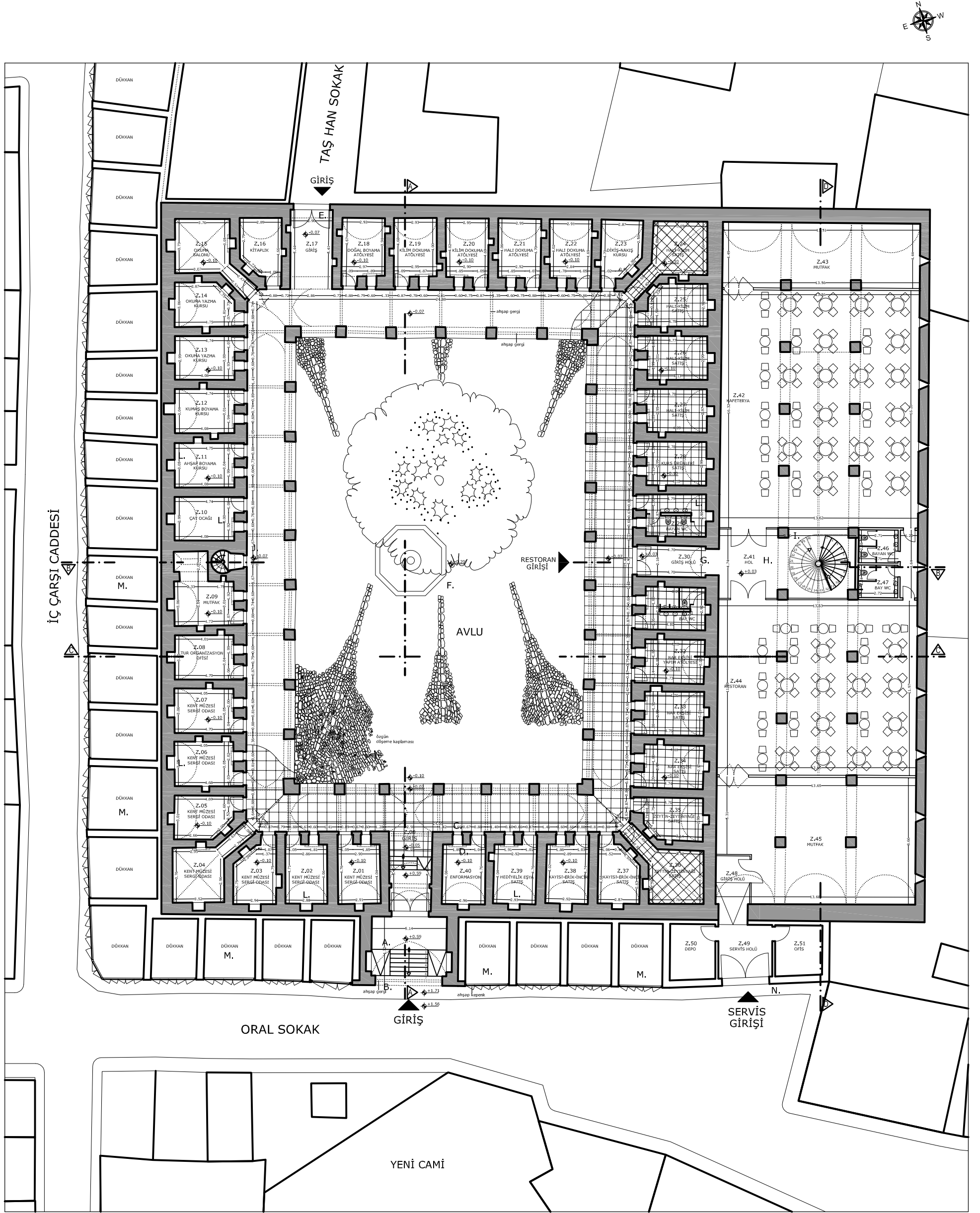
RESTORASYON - ZEMİN KAT PLANI 1/100
