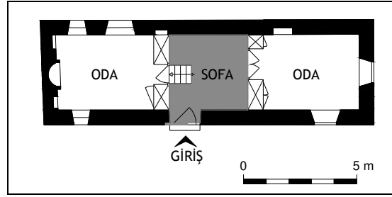
Şekil 2.13 “İki göz bir aralık” olarak adlandırılan plan tipi (Ünal, Yergün; 2007)
