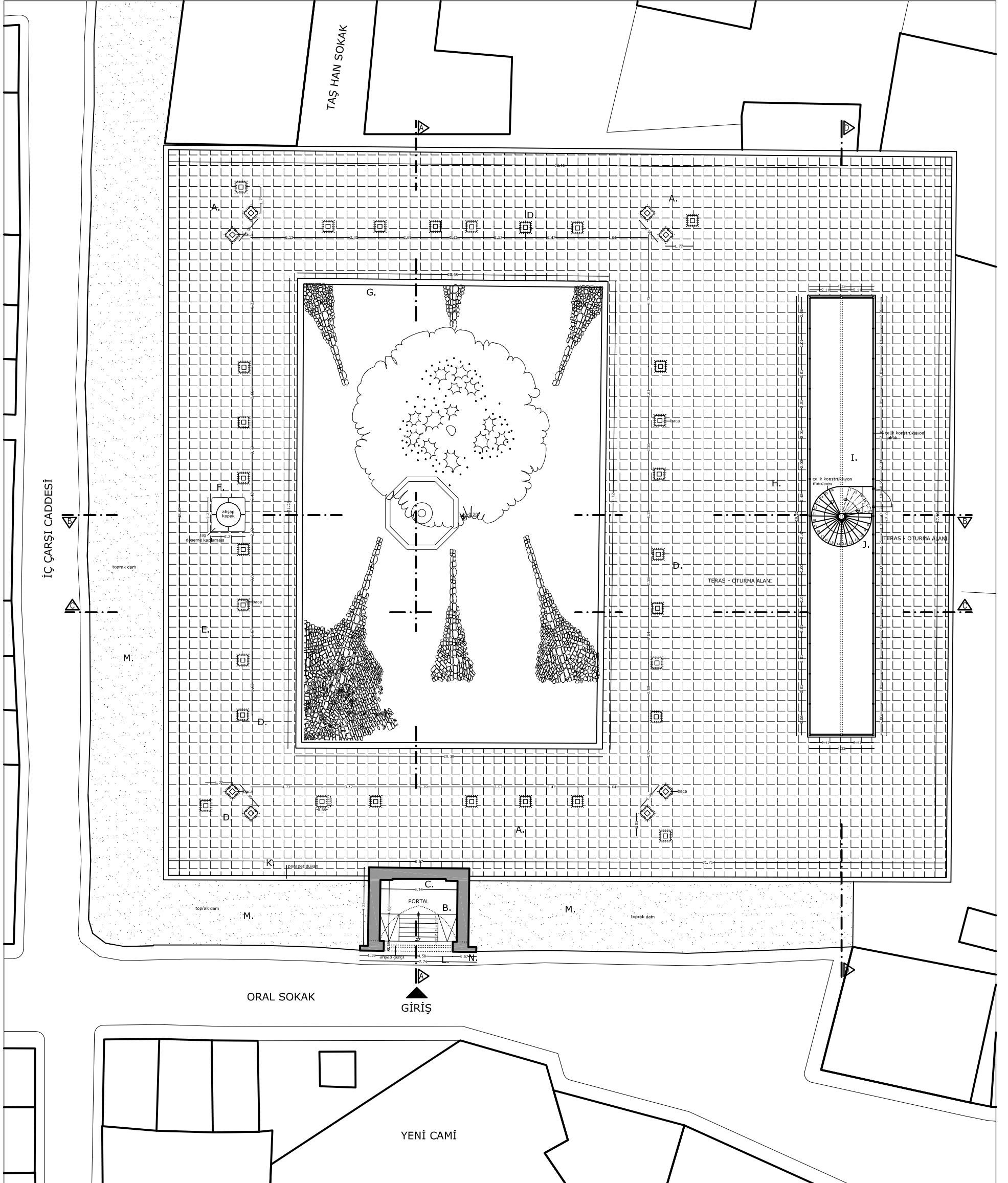
RESTORASYON - BİRİNCİ KAT PLANI 1/100
