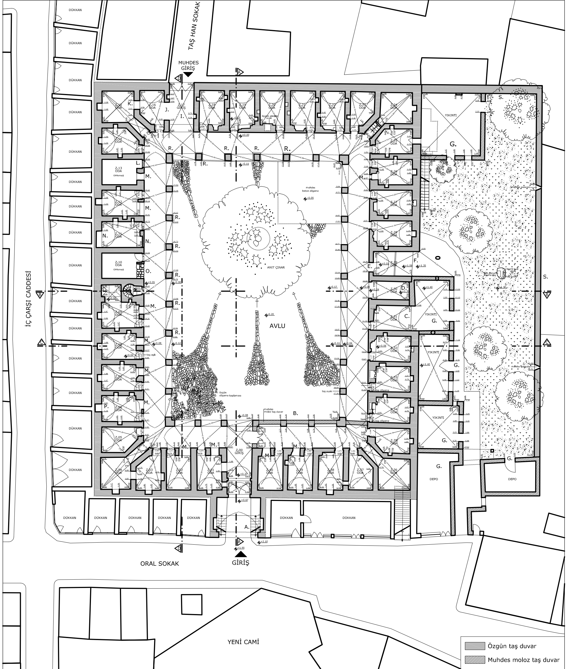
RÖLÖVE - ZEMİN KAT PLANI 1/100
