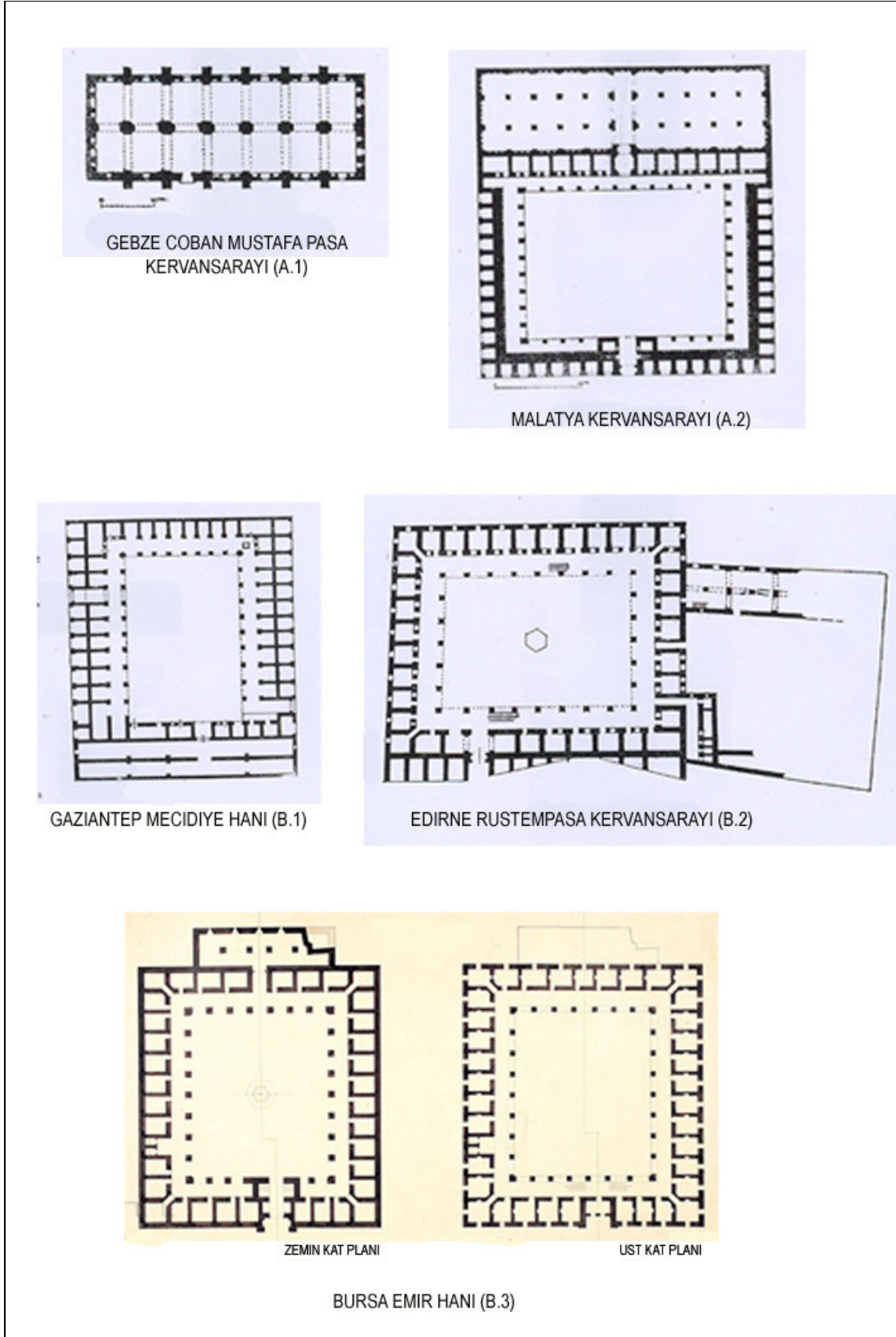
Şekil 3.3 Osmanlı Hanları plan tipleri (Akozan, 1963)
