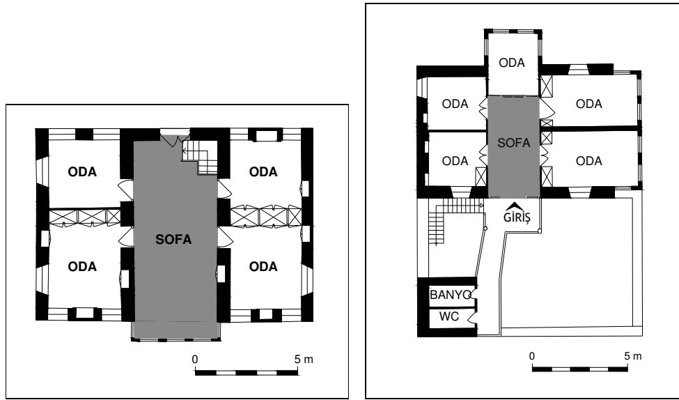
Şekil 2.14 Basit plan tipinden geliştirilmiş plan şemaları (Ünal, Yergün; 2007)
