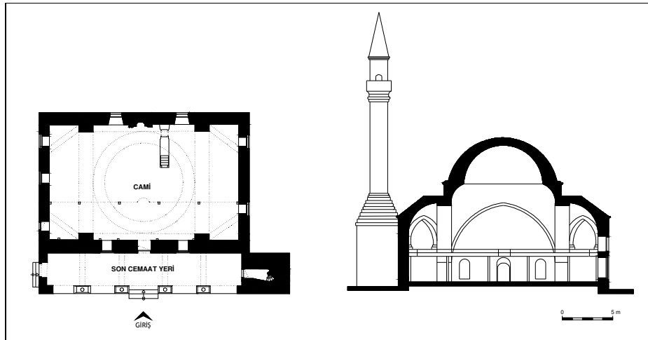
Şekil 2.8 La'lı Paşa Camii plan ve kesit krokisi (Arel, 1962'den tekrar çizim)
