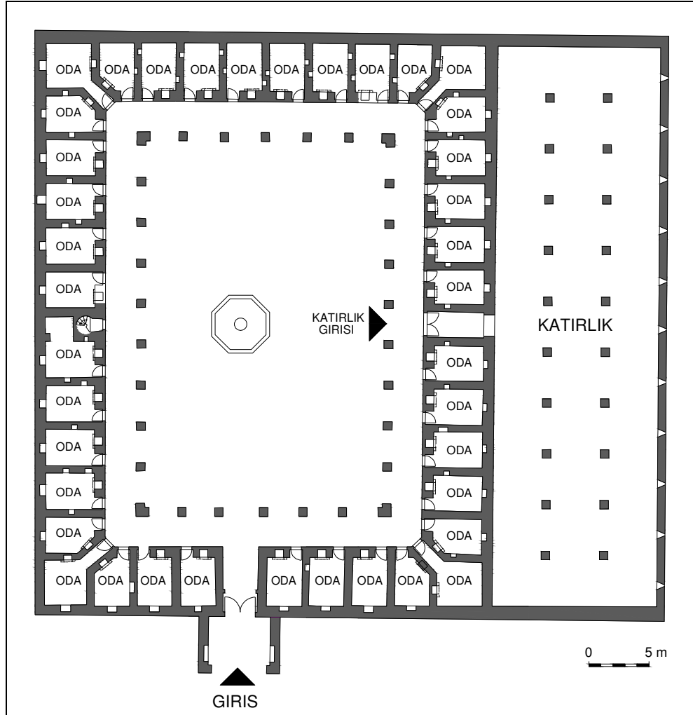
Şekil 4.2 Taş Han'ın özgün plan şeması
