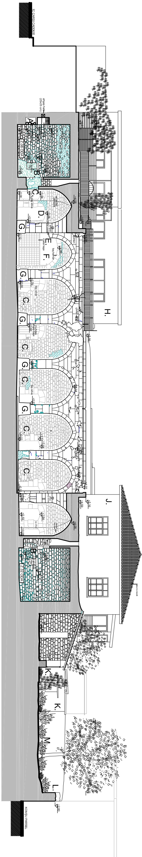
RÖLÖVE - C-C KESİTİ 1/100
