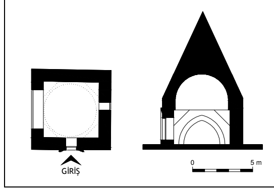
Şekil 2.10 Küçük kümbet plan ve kesit krokisi (Arel, 1962'den tekrar çizim)
