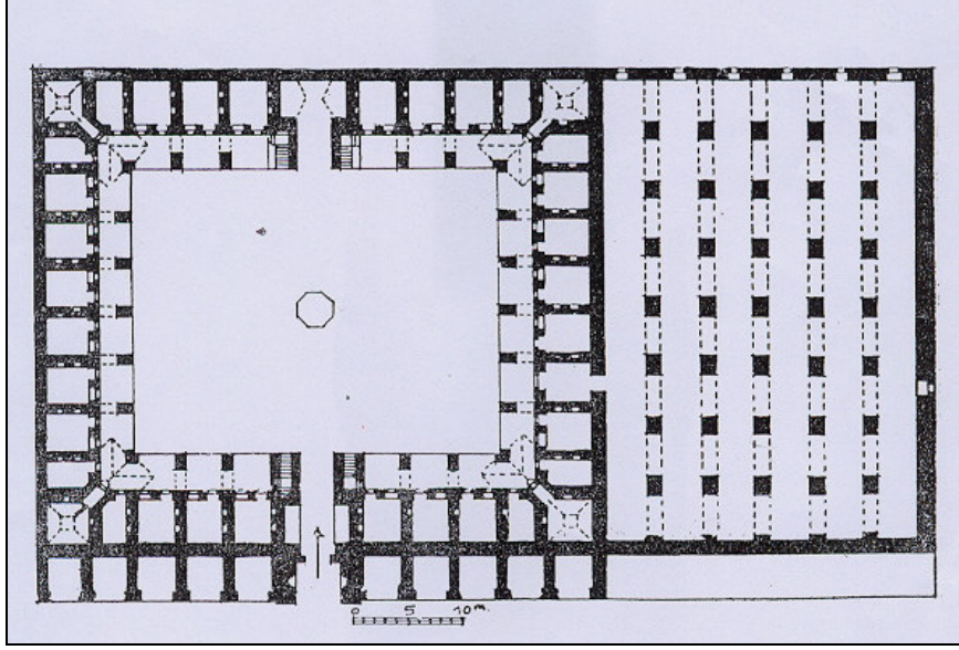
Şekil 4.15 Diyarbakır Hüsrev Paşa (Deliller) Hanı Planı (Akozan, 1963)
