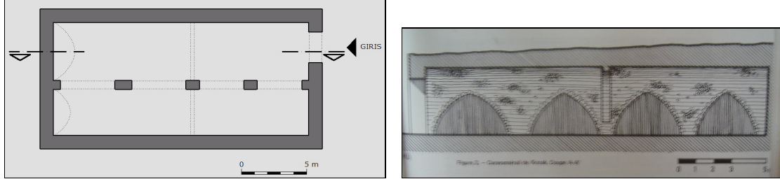
Şekil 4.11 Kozak Hanı plan (Ekim 2004) ve kesiti (Ünal,1993)
