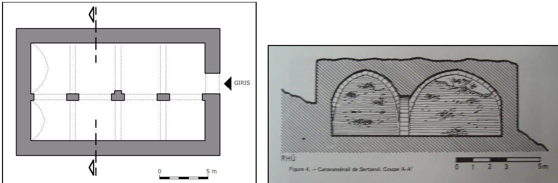
Şekil 4.12 Sertavul Hanı plan (Ekim 2004) ve kesiti (Ünal,1993)
