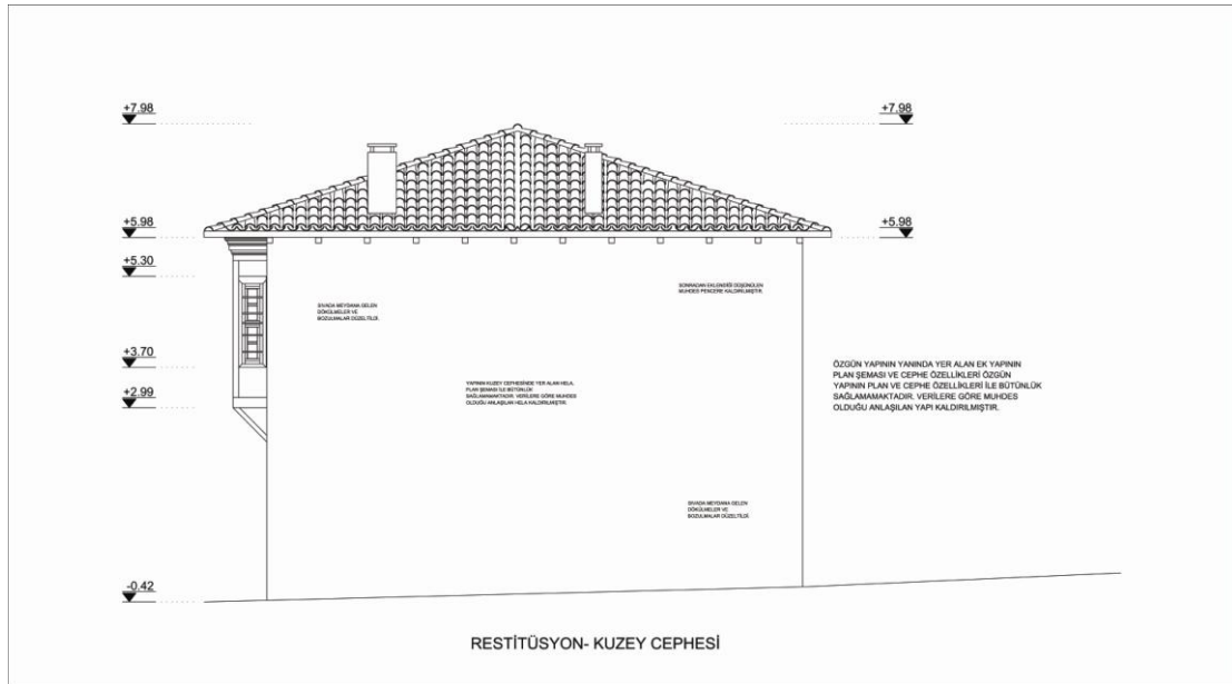
Şekil 6.165 Kuzey cephesi
