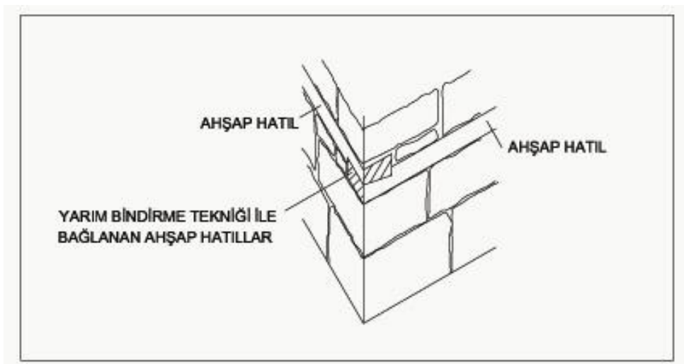
Şekil 5.1 Dış ve iç yüzeyi sıvalı ahşap hatıllı moloz taş duvar çizimi
