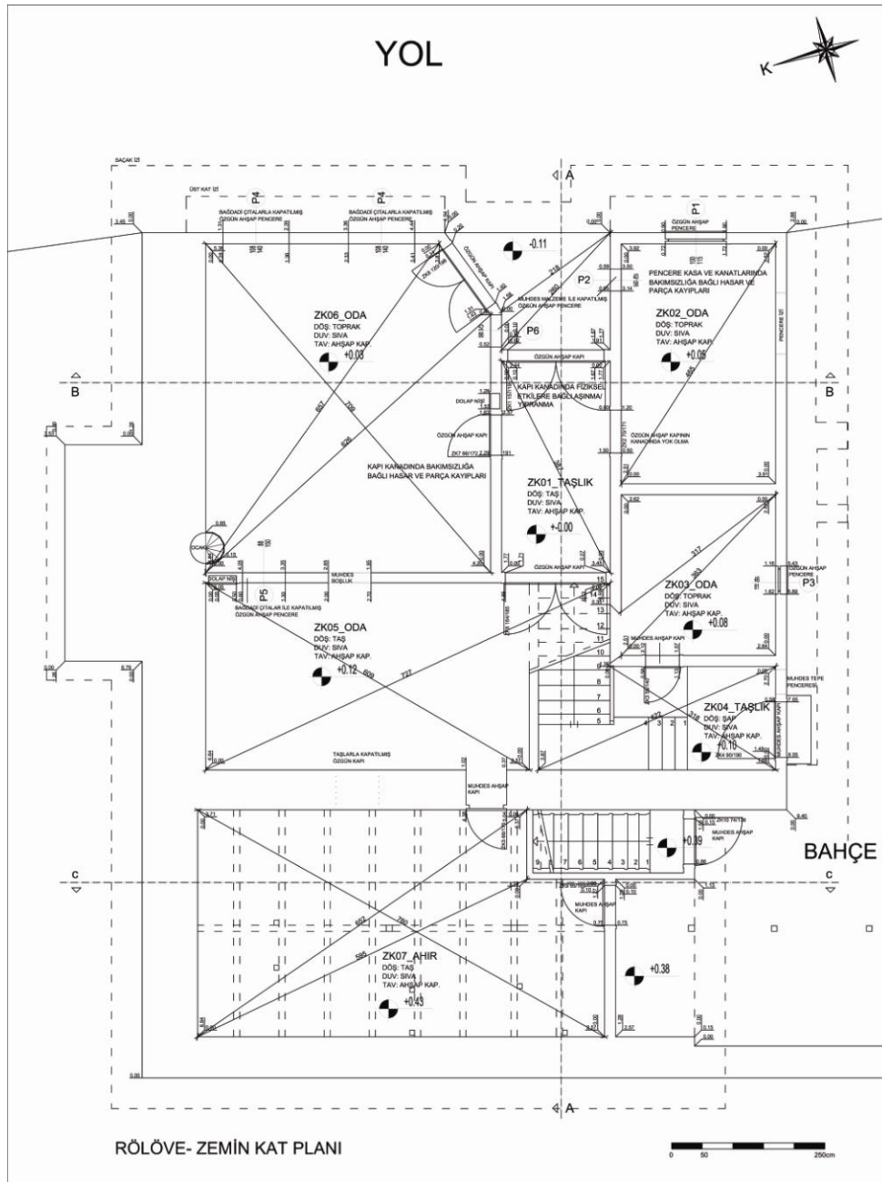
Şekil 6.1 Zemin kat planı
