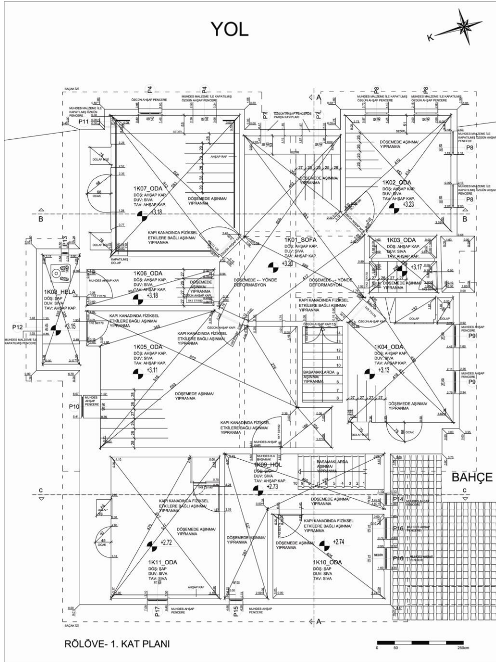
Şekil 6.51 Birinci kat planı
