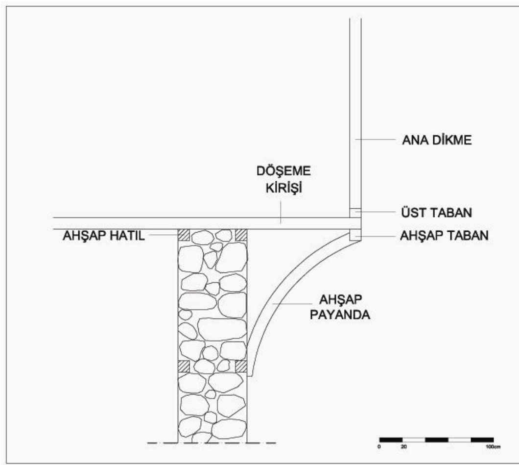
Şekil 4.44 Payandalarla desteklenen çıkmanın şematik çizimi
