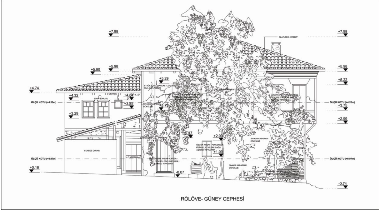
Şekil 6.145 Güney cephesi
