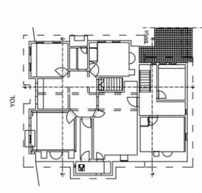
1. KAT PLANI
