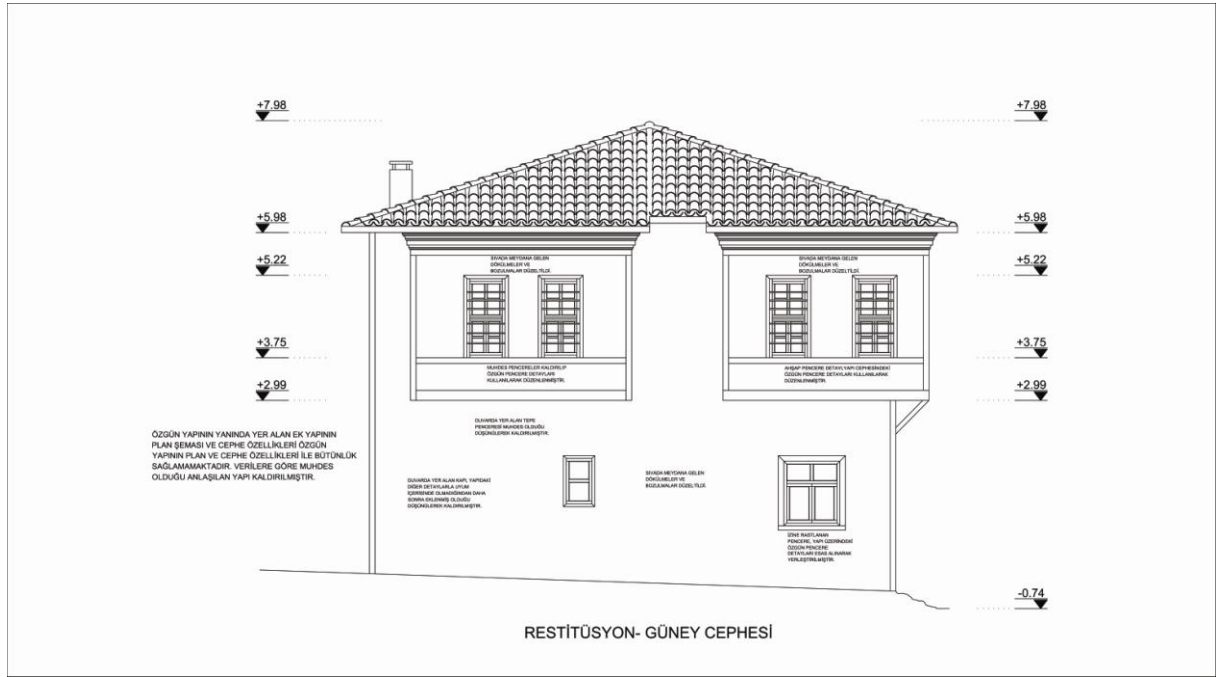
Şekil 6.164 Güney cephesi
