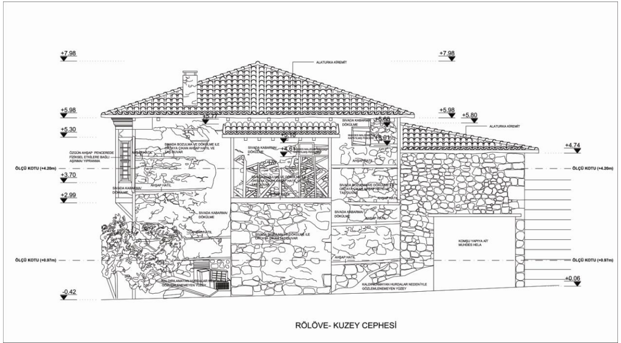
Şekil 6.156 Kuzey cephesi
