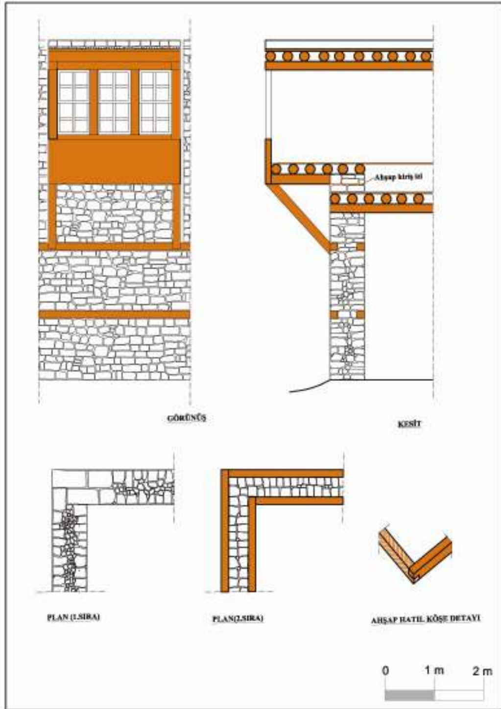
Şekil 4.9. Sistem Kesiti
