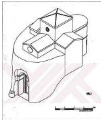
Şekil 4.3. Konacak Mevkii Şapel İzometrik Perspektif, (Mimiroğlu, 2005).
