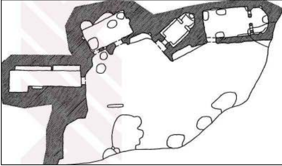
Şekil 4.4. Bayram Hacı İnleri Mevkii'nde bulunan Manastır Planı, (Mimiroğlu, 2005).
