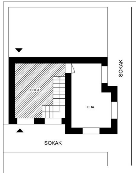
Şekil 4. 39 Dış sofalı çıkmalı tek odalı plan tipi (Envanter no:A-J-3, Ek IV, s.252)
