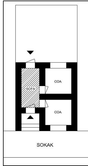
Şekil 4. 35 Dış sofalı tek katlı plan tipi (Envanter no:A-C-8, Ek IV, s.198)
