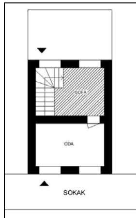
Şekil 4. 41 Dış sofalı tek odalı plan biçimlenişi (Envanter no:G-3, Ek IV, s.590 ve Envanter no:B-K-9, Ek IV, s.394)
