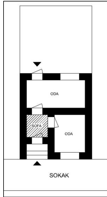
Şekil 4. 36 Dış sofalı tek katlı plan tipi (Envanter no:A-D-2, Ek IV, s.201)
