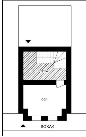
Şekil 4. 42 Dış sofalı tek odalı plan biçimlenişi (Envanter no:A-M-3, Ek IV, s.279 ve Envanter no:D-D-18, Ek IV, s.519)
