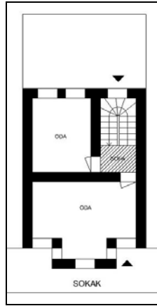
Şekil 4. 43 Dış sofalı iki odalı plan biçimlenişi (Envanter no:A-F-9, Ek IV, s.225 ve Envanter no:A-S-2, Ek IV, s.307)
