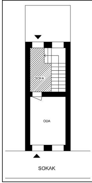
Şekil 4. 40 Dış sofalı tek odalı plan biçimlenişi. (Envanter no:D-E-5, Ek IV, s.531 ve Envanter no:B-O-10, Ek IV, s.434)
