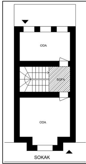
Şekil 4. 50 Orta sofalı iki katlı plan tipi (Envanter no:A-L-11, Ek IV, s.275 ve Envanter no:A-Q-4, Ek IV, s.302)
