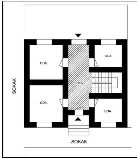
Şekil 4. 48 Orta sofalı iki katlı plan tipi (Envanter no:D-C-1, Ek IV, s.486 ve Envanter no:F-11, Ek IV, s.582)
