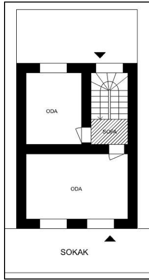
Şekil 4. 44 Dış sofalı iki odalı plan biçimlenişi (Envanter no:B-I-5, Ek IV, s.372 ve Envanter no:B-A-4, Ek IV, s.325)
