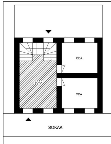
Şekil 4. 37 Dış sofalı iki katlı plan tipi. (Envanter no:A-Q-5, Ek IV, s.303 ve Envanter no:B-O-12 , Ek IV, s.436)
