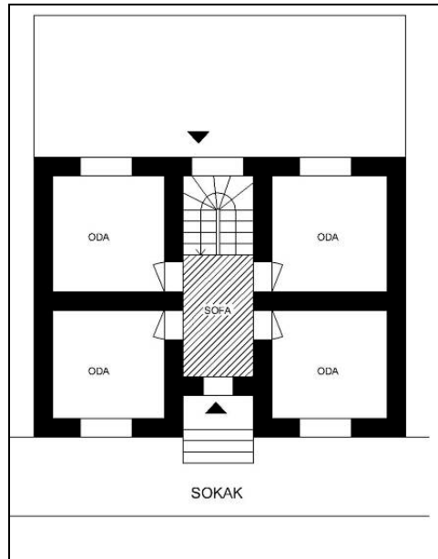
Şekil 4. 47 Orta sofalı iki katlı plan tipi (Envanter no:D-A-1, Ek IV, s.464)
