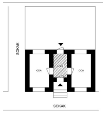
Şekil 4. 45 Orta sofalı tek katlı plan tipi (Envanter no:A-F-7, Ek IV, s.223 ve Envanter no:A-I-4, Ek IV, s.237)
