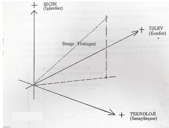
Şekil 4.1 Dengeler yörüngesi.
