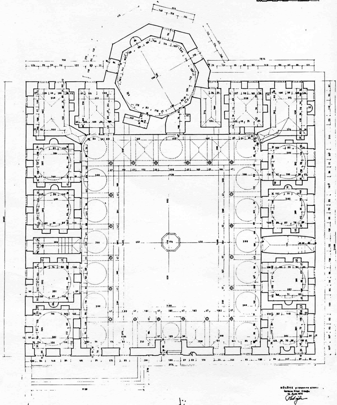
Şekil 5.5 Şeyhülislam Mustafa Efendi Tekkesi Rölövesi, Erkoğlu 1970.
