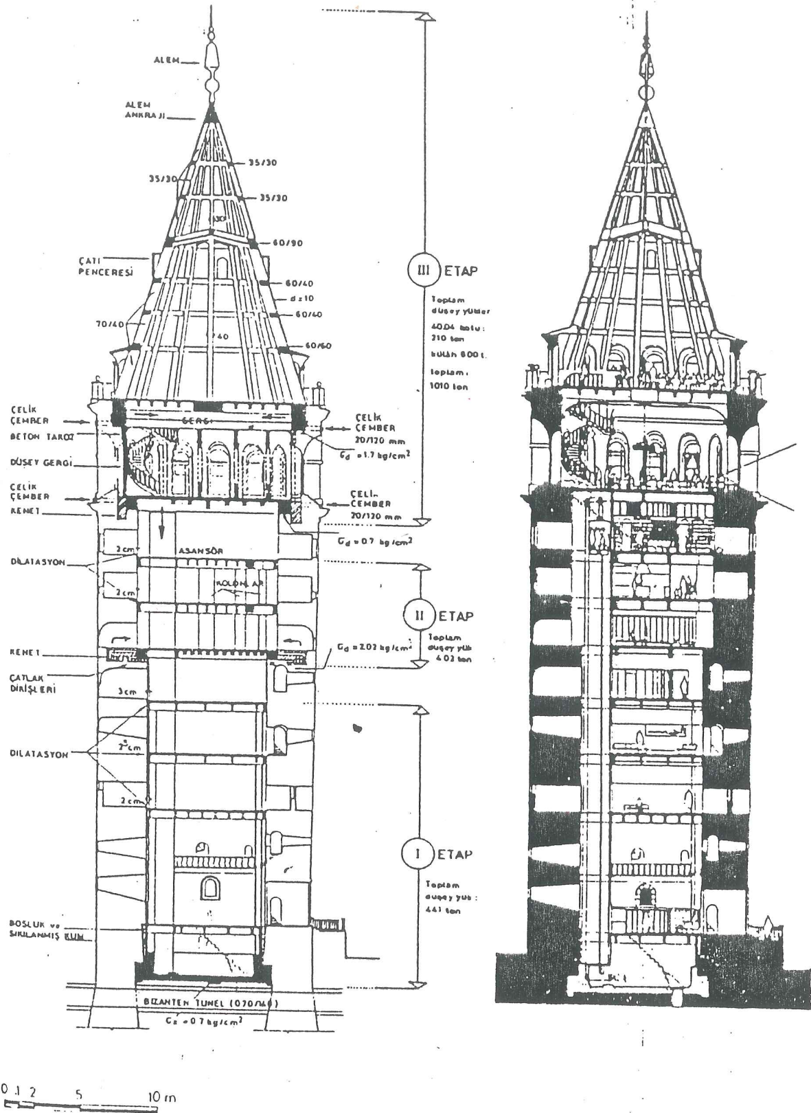
Resim 6: Galata Kulesi, kesitleri.
