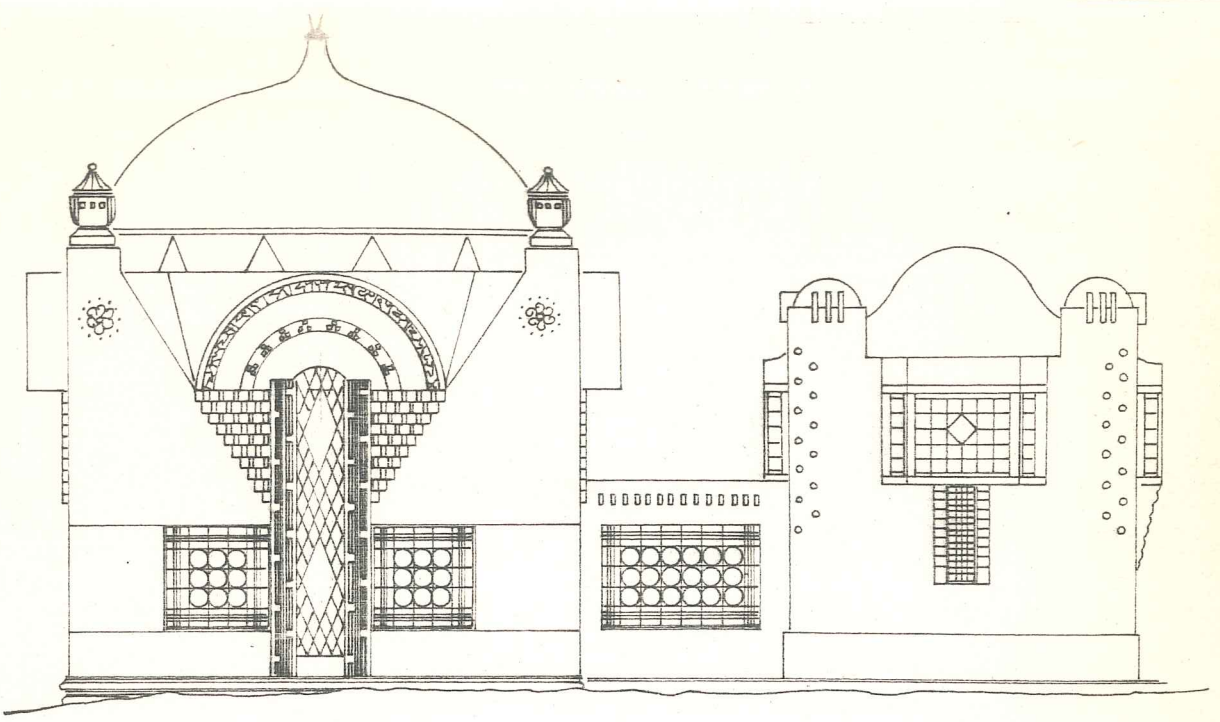
Çizim 6: TÜRBE VE KÜTÜPLÜK BATI CEPHESİ
