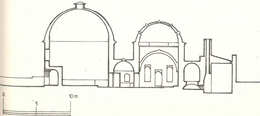
Çizim 13: SİNAN PAŞA HAMAMI KESİT
