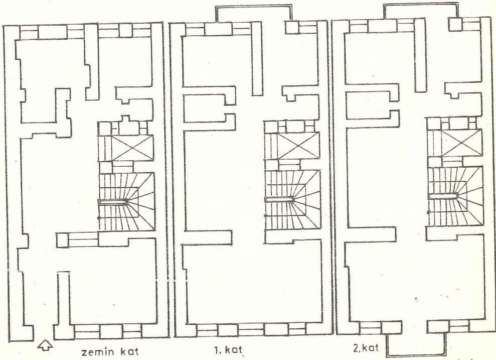
Çizim 22: AKARETLERDE CUMBASIZ VE BALKONLU PLAN TİPİ (Bkz.R.65)
