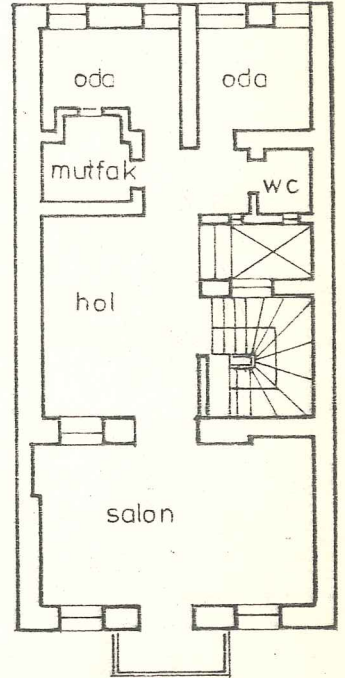
Çizim 20: AKARETLERDE DÜKKÂN KONUT ÖRNEĞİ (Bkz.R. 65)
