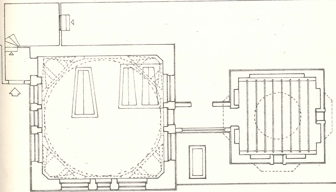
Çizim 5: ŞEYH ZAFİR TÜRBE VE KÜTAPLİĞİ
