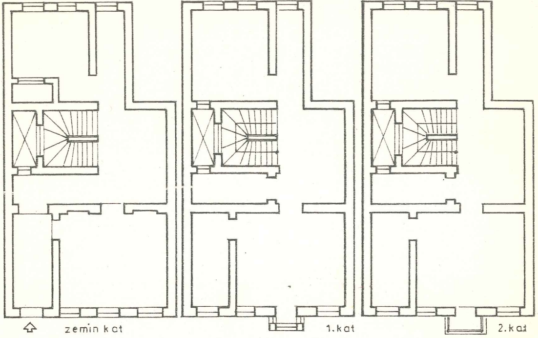
Çizim 19: AKARETLER'DE CUMBALI VE BALKONLU PLAN TİPİ (Bkz. R.66)
