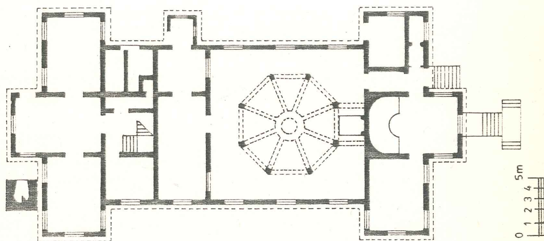
Çizim 3: ERTUĞRUL CAMII
