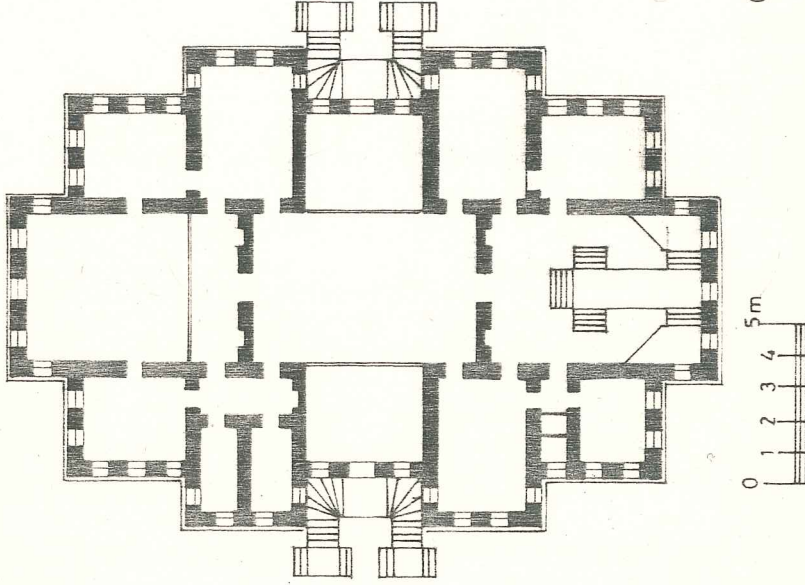
Çizim 18: YILDIZ SARAYI BÜYÜK MABEYN KÖŞKÜ
