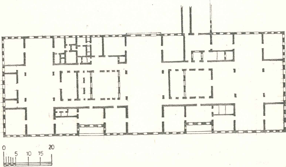
Çizim 17 : ÇİRAĞAN. SARAYI
