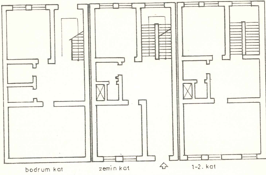
Çizim 21: AKARETLERDEN BİR PLAN TİPİ
